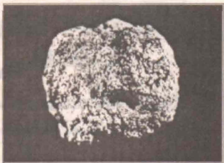
Рис. 69. Полуоплавленная медноколчеданная руда. Мецамор. III—II тыс. до н. э.
