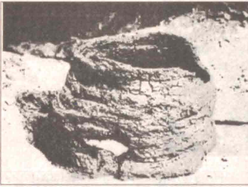
Рис. 53. Домницы. Мецамор. II тыс. до н. э.
