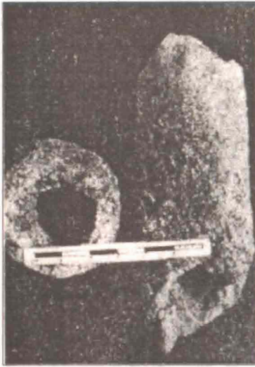
Рис. 64. Сопла (воздухопроводные трубы) доменных печей и металлургический шлак. Мецамор. III—II тыс. до н. э.
