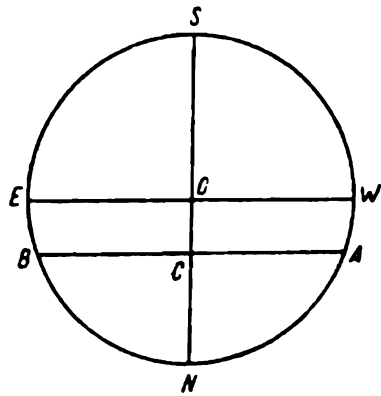
Рис. 168 «Индийский круг».
