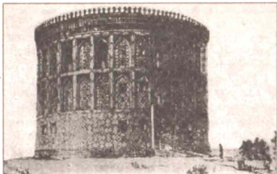
Рис. 169. Самаркандская обсерватория.
