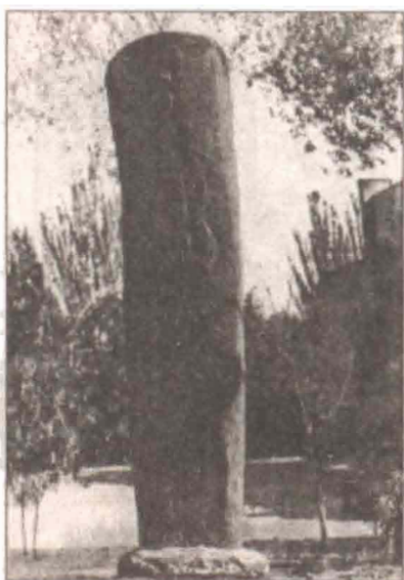
Рис. 133. Гномон «Зангезур-2».
