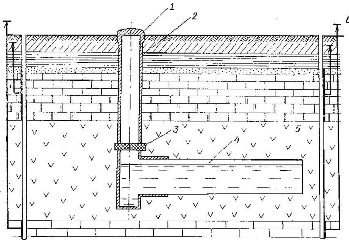
Նկ. 9. Հանքափողային (շախտային) տիպի պահեստարանի երկրաբանաջրաերկրաբանական սխեմատիկ կտրվածքը.
