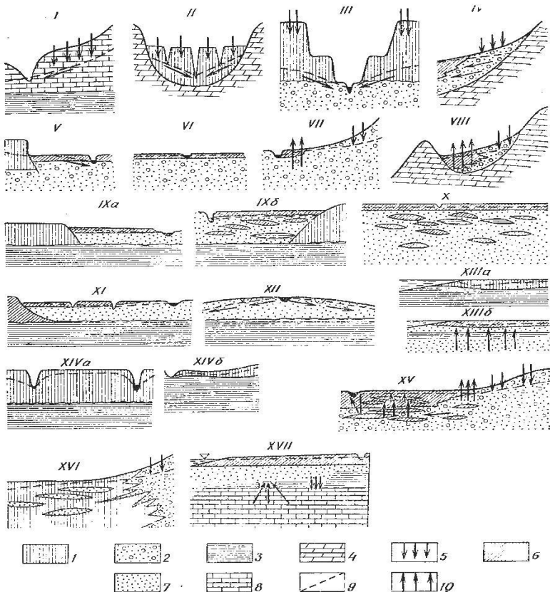
Նկ. 3 Ջրաերկրաբանական պայմանների տիպերը (ըստ Դ. Մ. Կացի)։
