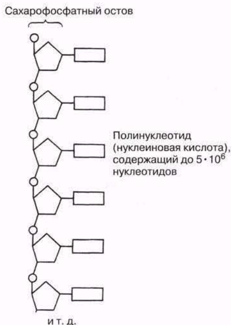
Рис. 3.40. Образование полинуклеотида.
