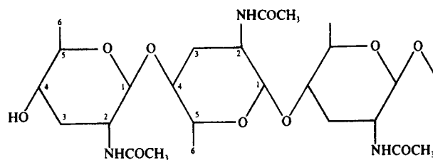
Рис. 3.15. Строение хитина.
