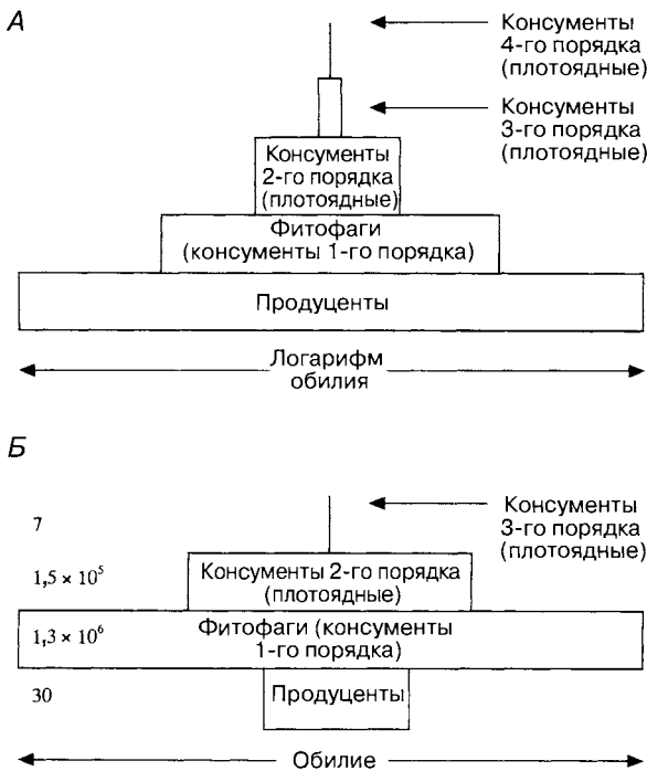
Рис. 10.6. А. Типичная пирамида чисел. Длина каждого прямоугольника пропорциональна обилию организмов каждого трофического уровня. Чаще всего применяется логарифмический горизонтальный масштаб. Консументов высшего порядка принято называть верховными хищниками. Б. Перевернутая пирамида чисел для дубравы Уайтем в Оксфордшире. Горизонтальный масштаб логарифмический. Числа слева отражают обилие организмов на гектар. В качестве продуцентов учитывались только дубы. (Данные из: Varley, 1970.)
