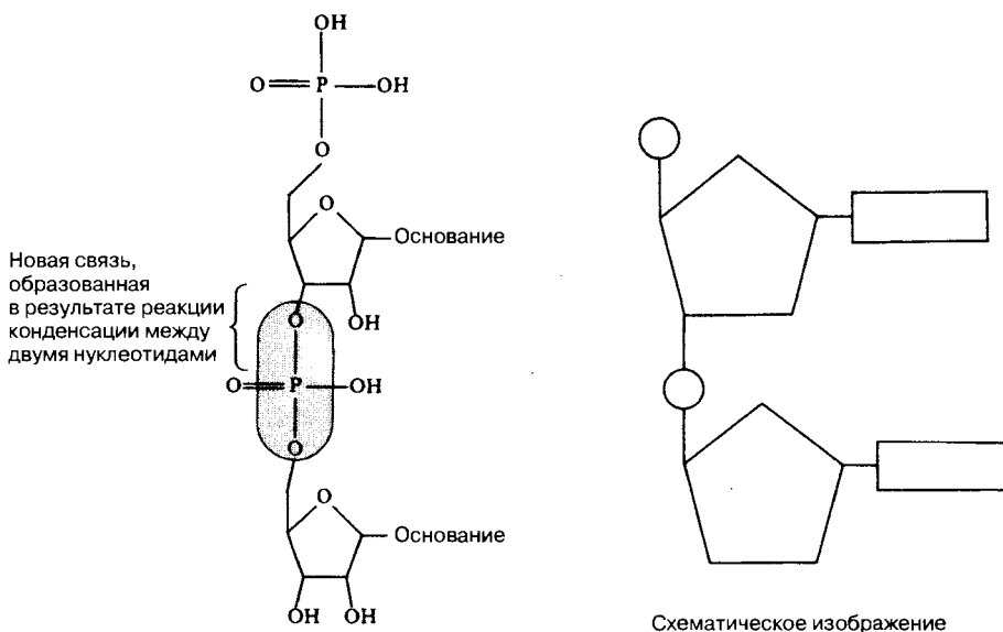
Рис. 3.39. Структура динуклеотида.
