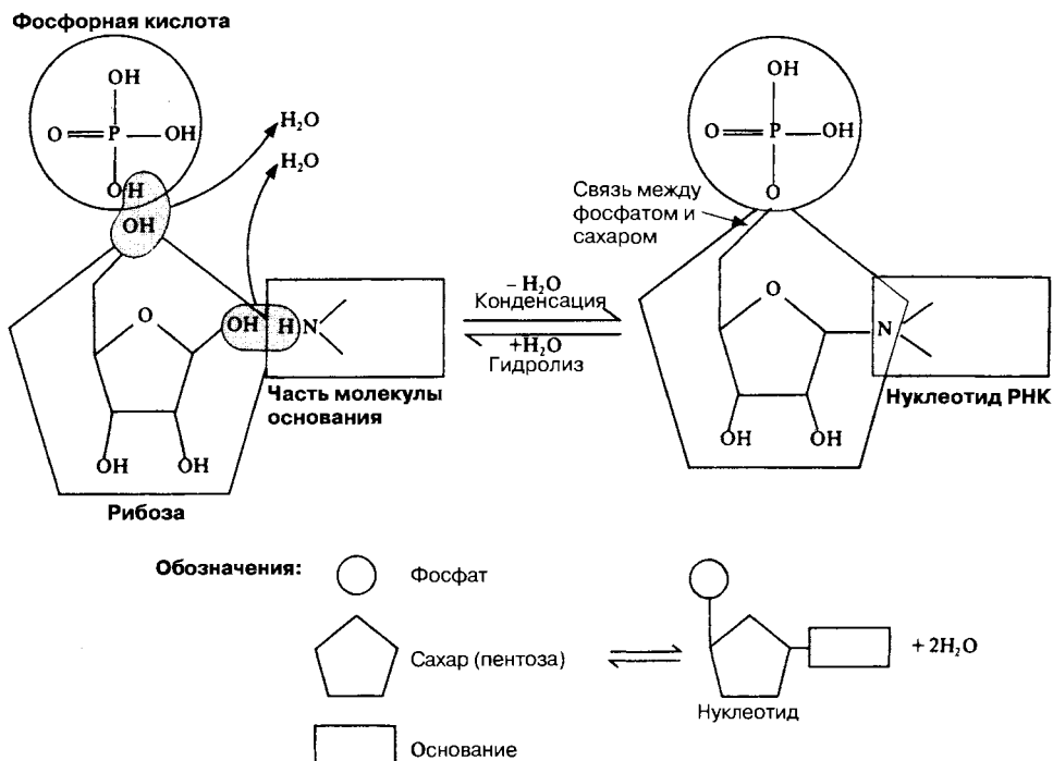
Рис. 3.38. Образование нуклеотида.
