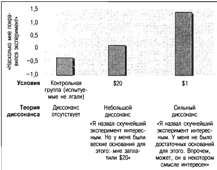
Рис. 4.2. Недостаточное оправдание.
