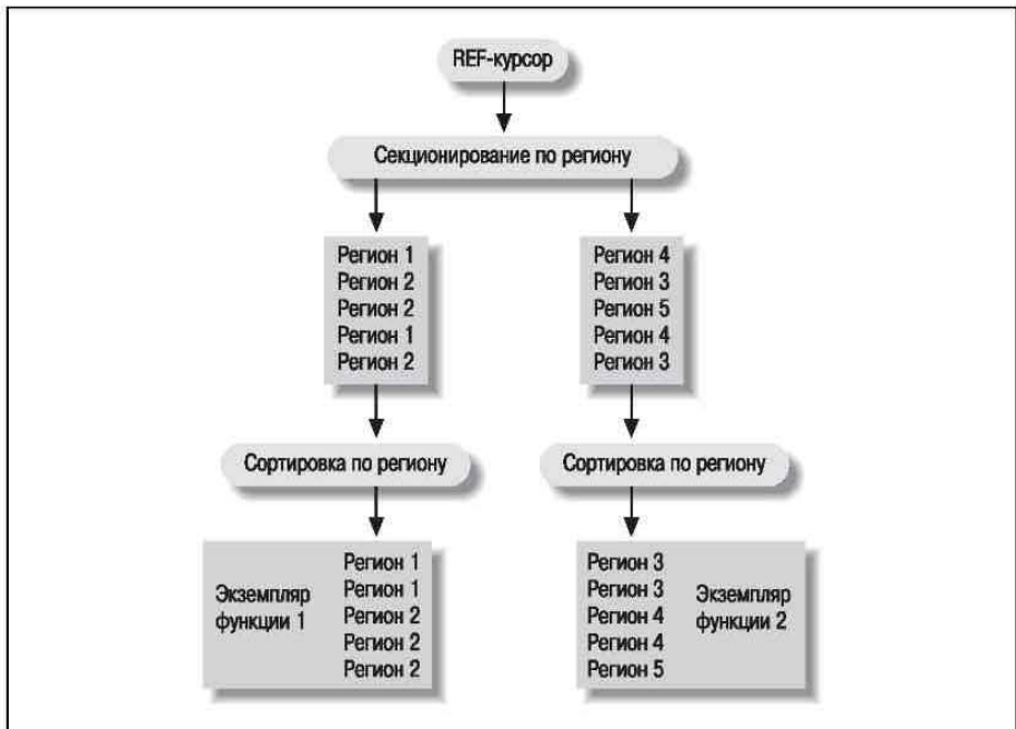
Рис. 3.2. Распараллеленная табличная функция, секционированная и отсортированная по региону
