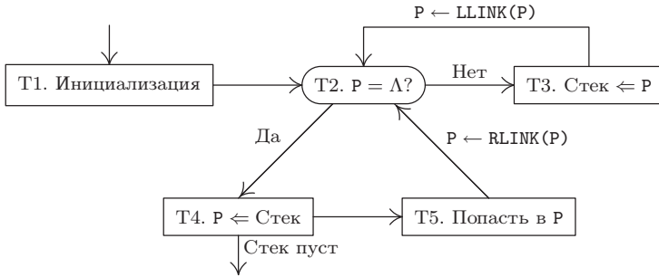
Рис. 23. Алгоритм Т для симметричного обхода.
