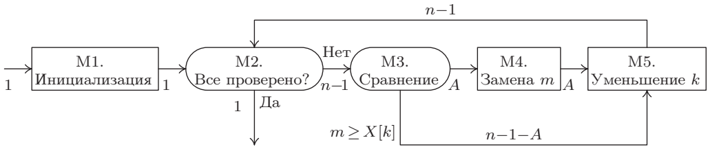
Рис. 9. Алгоритм М. Подписи к стрелкам показывают, сколько раз осуществляется проход каждого пути. Заметьте, что должен выполняться первый закон Кирхгофа, который в данном случае выглядит так: число входов в каждый узел должно равняться числу выходов из него.
