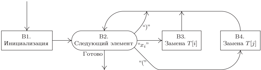
Рис. 21. Алгоритм В: перемножение перестановок.
