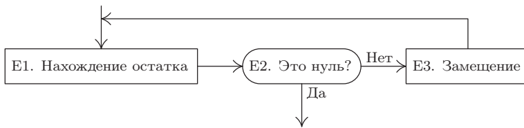
Рис. 1. Блок-схема алгоритма E.
