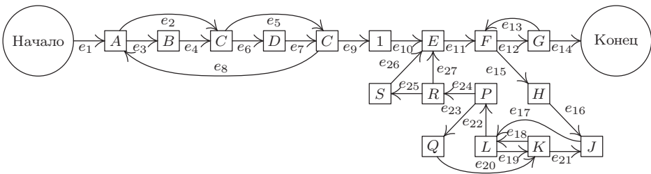
Рис. 31. Абстрактная блок-схема программы 1.3.3А.
