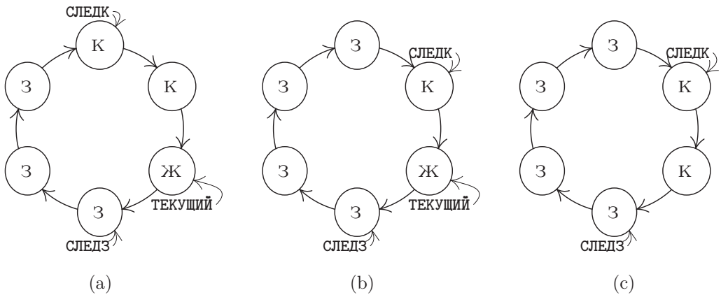
Рис. 24. Состояния буферов: (а) после НАЗНАЧИТЬ , (b) после завершения В/В и (с) после ОСВОБОДИТЬ .
