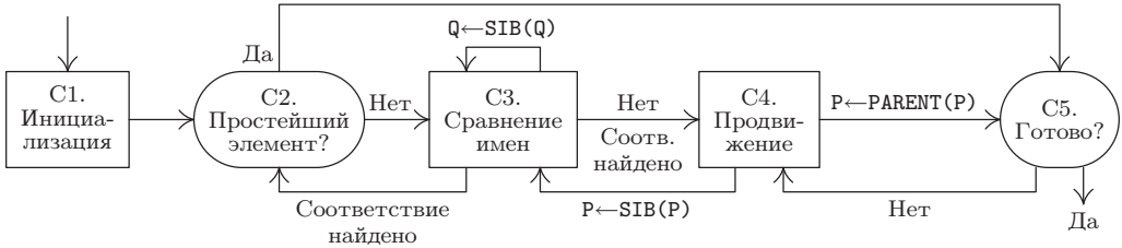
Рис. 41. Алгоритм для выполнения команды MOVE CORRESPONDING.
