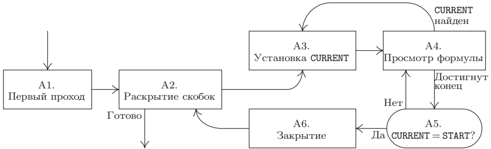
Рис. 20. Алгоритм А (перемножение перестановок).
