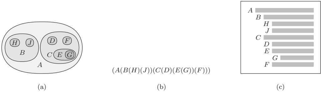
Рис. 20. Способы изображения древовидных структур: (а) вложенные множества; (б) вложенные скобки; (с) список с отступами.
