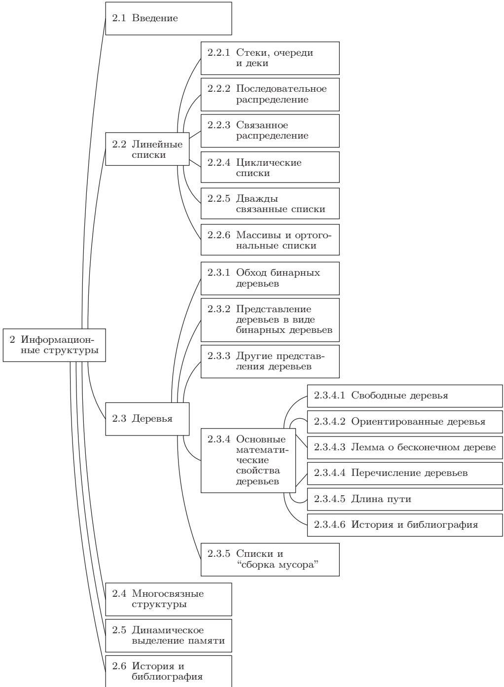
Рис. 22. Структура главы 2.
