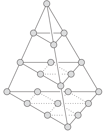
Рис. 8. Геометрическая интерпретация \binom{n+2}{3} , n = 4 .
