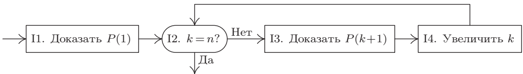
Рис. 2. Алгоритм I: математическая индукция.
