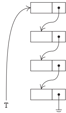
Рис. 5. Связанный стек.
