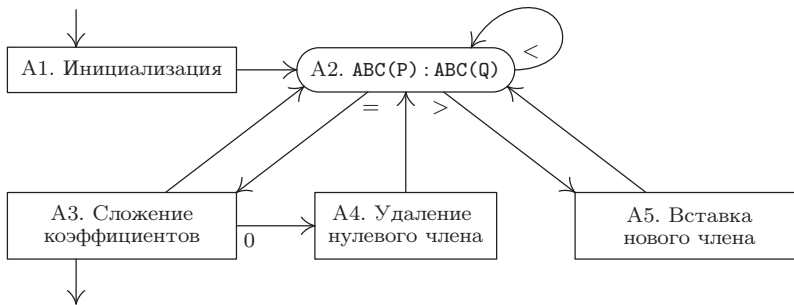
Рис. 10. Сложение многочленов.
