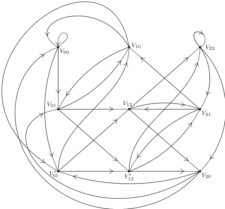
Рис. 37. Диграф с дугами, который соответствует рис. 36 (см. упр. 21).
