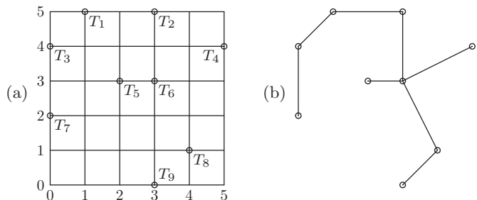
Рис. 33. Свободное дерево с минимальной ценой.
