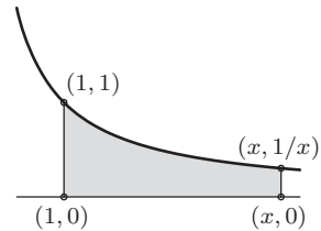
Рис. 6. Натуральный логарифм.
