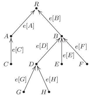
Рис. 34. Ориентированное дерево.
