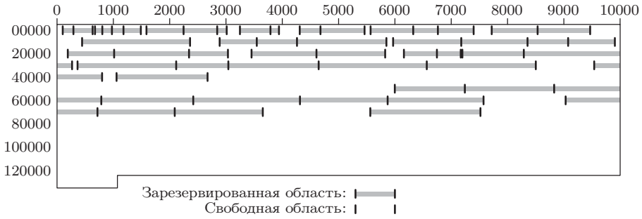
Рис. 42. Карта памяти.
