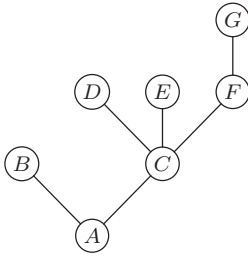
Рис. 15. Пример дерева.
