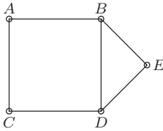
Рис. 29. Граф.
