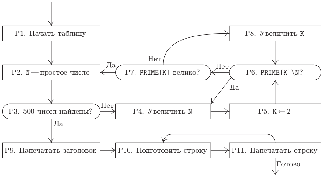
Рис. 14. Алгоритм P.
