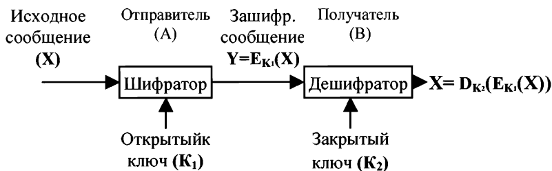
Рис 3.1. Схема асимметричной криптосистемы.
