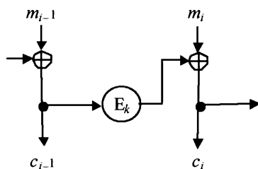
Рис. 2.7. Режим обратной связи по шифрованному тексту.
