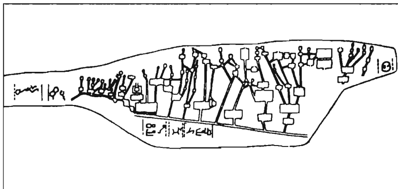
Рис. 58. Схематический план главного сооружения тонкого обогащения («доводки») и иероглифические письма.
