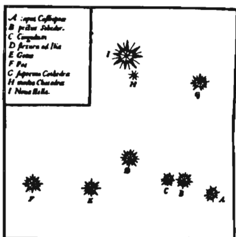
Рис. 179. Новая звезда в созвездии Кассиопеи, обнаруженная Тихо Браге.
