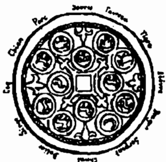
Рис. 159. Китайские и японские астрономические монеты.
