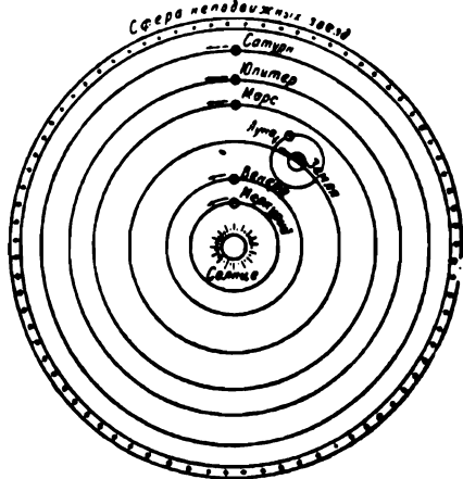
Рис. 177. Система мира по Копернику.
