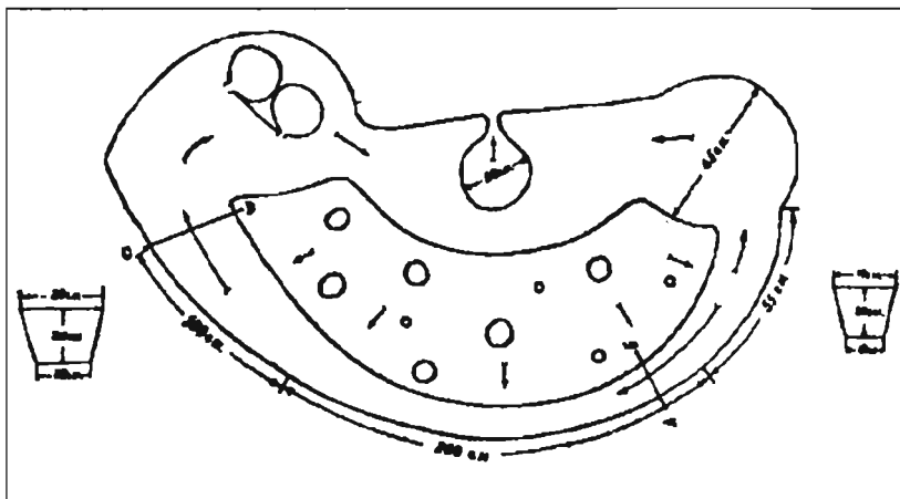
Рис. 60. Комбинированное обогащательное сооружение. Мецамор. III—II тыс. до н. э.
