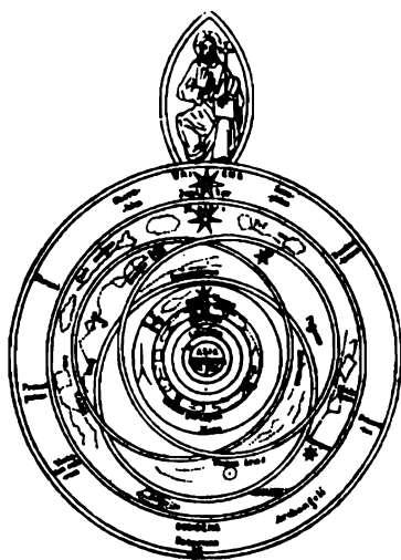
Рис. 174. Изображение планетной системы в средние века.
