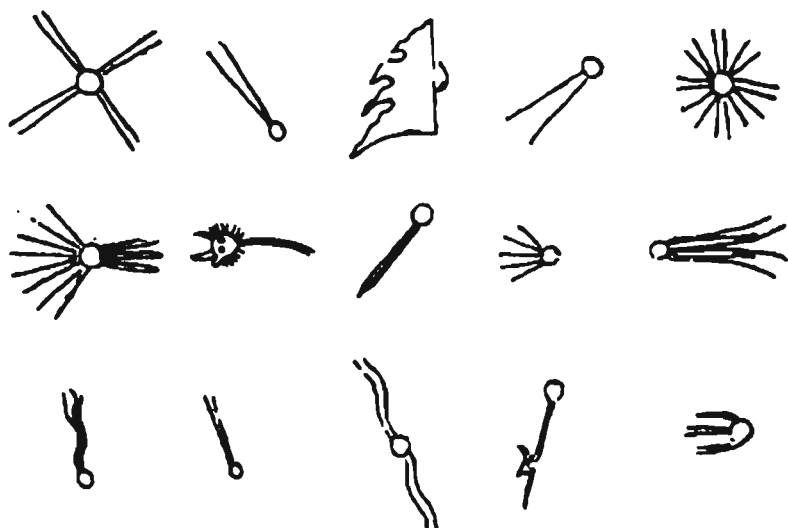
Рис. 110. Изображения комет и падающих звезд (Древний Китай).
