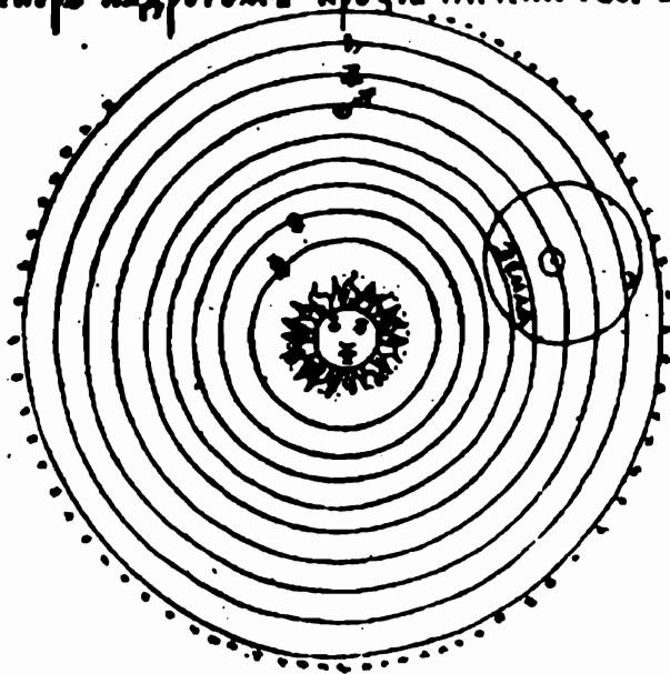
Рис. 181. Изложение теории Коперника в рукописи конца XVII в. «Зерцало всея Вселенная».
