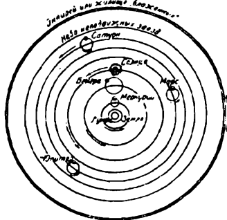
Рис. 152. Птолемеивская система мира.
