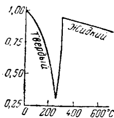
Рис. IX-56. Изменение относительной электропроводности висмута с температурой.
