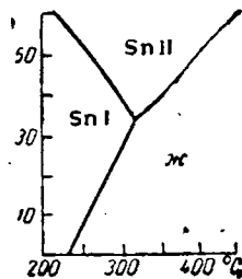
Рис. X-75. Диаграмма состояния олова при высоких давлениях (тыс. ат).
