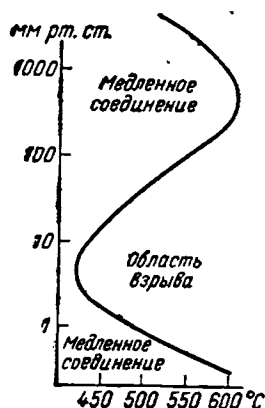
Рис. X-22. Влияние внешних условий на скорость реакции 2\text{H}_2 + \text{O}_2 = 2\text{H}_2\text{O} .
