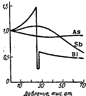
Рис. IX-54. Влияние давления на относительное электропроводность.
