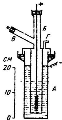
Рис. VII-1. Электролизер для получения фтора.
