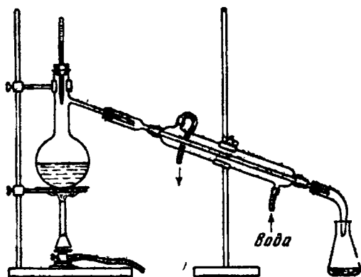
Рис. II-16. Простейшая установка для перегонки жидкостей.
