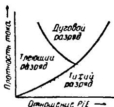
Рис. II-13. Условия возникновения непрерывных электрических разрядов в газах.
