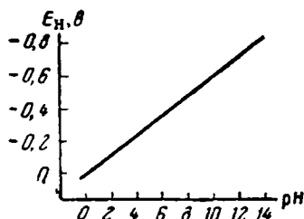
Рис. V-35. Зависимость потенциала водородного электрода от pH среды.
