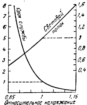
Рис. VIII-35. Относительные характеристики лампы накаливания.
