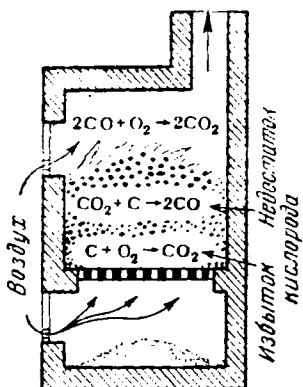
Рис. X-3. Образование и сгорание \text{CO} в печи.
