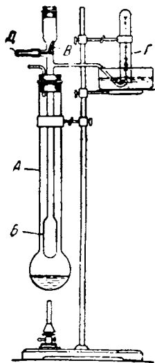
Рис. 1-10. Прибор для определения молекулярного веса.
