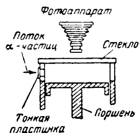
Рис. III-8. Схема конденсационной камеры.
