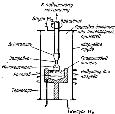
Рис. X-78. Схема установки для выращивания монокристалла германия.
