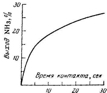
Рис. IX-5. Примерный ход реакции синтеза аммиака.
