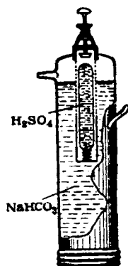
Рис. X-15. Схема получения твердой углекислоты.
