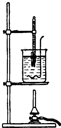
Рис. 11-19. Простейшая установка для определения температур плавления.
