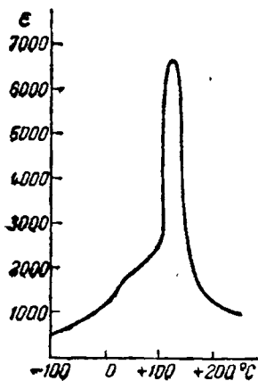
Рис. X-81. Зависимость диэлектрической проницаемости \text{BaTiO}_3 от температуры (в слабых полях).
