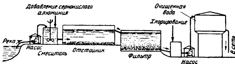
Рис. IV-14. Схема очистки речной воды.
