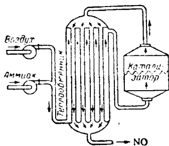
Рис. IX-24. Принципиальная схема установки для каталитического окисления аммиака.
