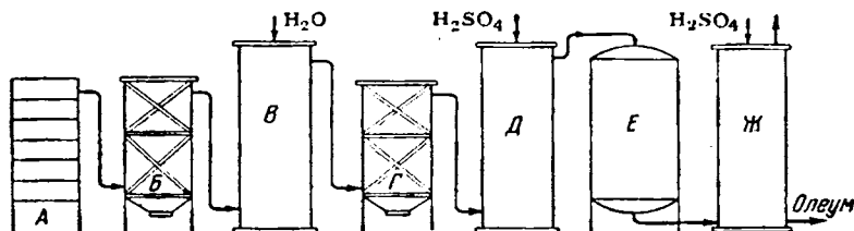
Рис. VIII-26. Схема контактного метода получения серной кислоты.
