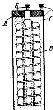
Рис. IX-11. Схема сухого элемента.
