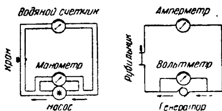
Рис. V-30. Аналогия водной и электрической систем.
