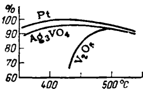
Рис. VIII-27. Выход \text{SO}_3 на катализаторах контактного метода.
