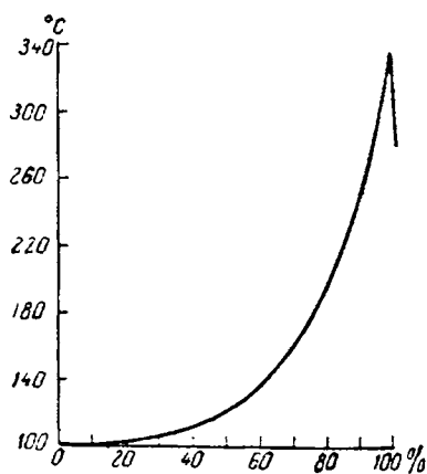
Рис. VIII-21. Температуры кипения растворов \text{H}_2\text{SO}_4 .
