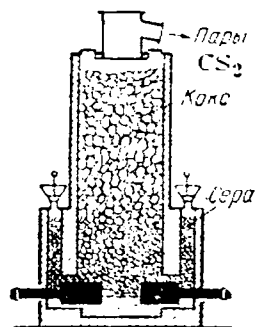
Рис. X-19. Схема электрической печи для получения \text{CS}_2 .
