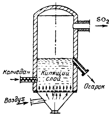
Рис. VIII-24. Схема печи для обжига пирита в кипящем слое.
