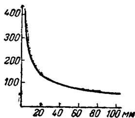
Рис. X-63. Диаметр стеклянного волокна (мк) и его прочность на разрыв (кг/мм²).
