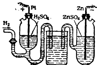
Рис. V-34. Схема определения электродного потенциала цинка.
