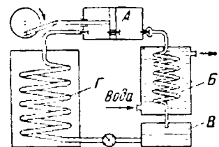
Рис. IX-7. Схема холодильной машины.
