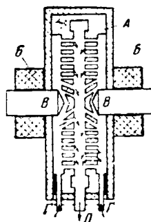
Рис. IX-25. Схема печи для «сжигания воздуха».
