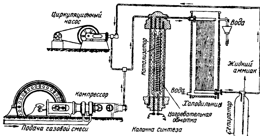
Рис. IX-2. Примерная схема установки для синтеза аммиака.
