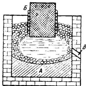
Рис. X-23. Схема электрической печи для получения \text{CaC}_2 .
