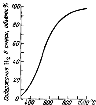
Рис. X-4. Равновесие синтеза метана.
