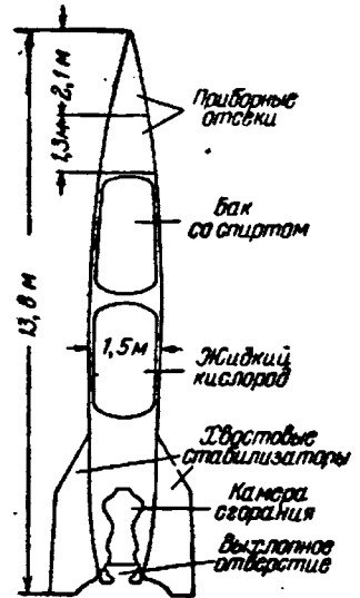
Рис. 11-14. Примерная схема не большой ракеты для высотных исследований.
