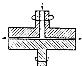
Рис. X-67. Схема коллоидной мельницы.
