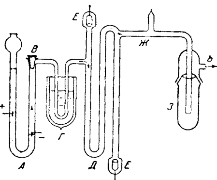
Рис. IV-3. Схема установки для получения атомарного водорода.
