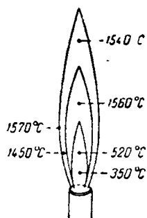
Рис. X-42. Пламя газовой горелки.
