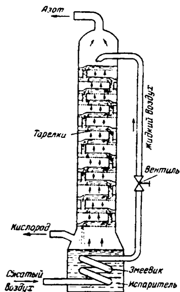
Рис. II-8. Общая схема колонны для разделения воздуха.
