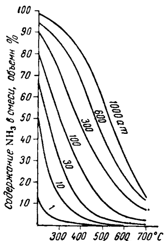
Рис. IX-1. Равновесие синтеза аммиака из элементов.
