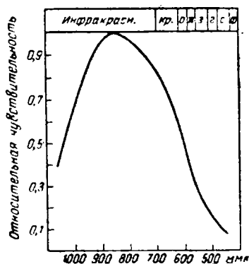
Рис. X-49. Спектральная характеристика кремниевого фотозоэлемента.
