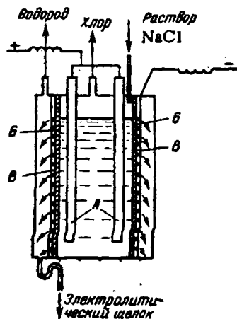
Рис. VII-5. Принципиальная схема электролизера для получения хлора.
