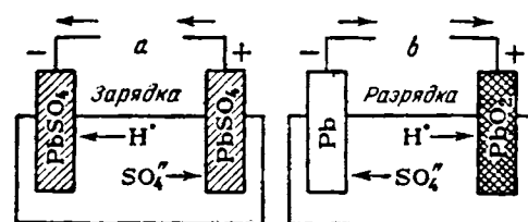
Рис. X-80. Схема работы свинцового аккумулятора.
