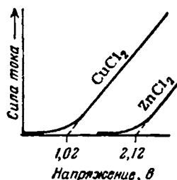
Рис. V-38. Схема приближенного определения потенциала разложения.
