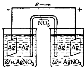
Рис. V-36. Схема концентрационной цепи.
