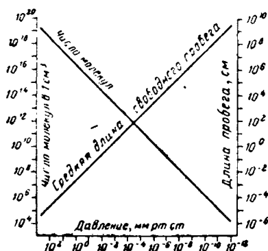
Рис. 11-4. Основные характеристики вакуума.
