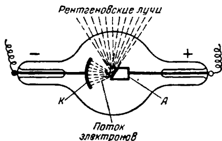
Рис. III-14. Схема рентгеновской трубки.
