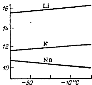
Рис. IX-9. Растворимость щелочных металлов в жидком аммиаке (г-атомов/100 г \text{NH}_3 ).
