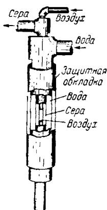
Рис. VIII-7. Схема установки для подземной выплавки серы.
