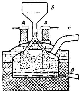
Рис. IX-32. Схема электропечи для получения фосфора.
