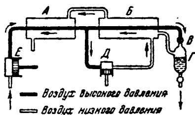
Рис. 11.5. Принципиальная схема установки для получения жидкого воздуха.
