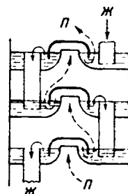
Рис. II-7. Схема работы «тарелок» раздельной колонны.
