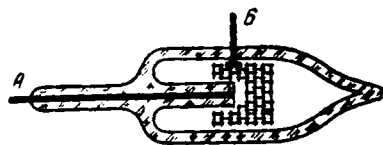
Рис. VII-18. Схема простейшего хемотрона.
