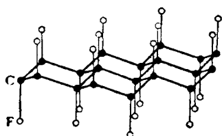
Рис. X-10. Схема структуры слоя \text{CF} .
