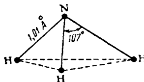
Рис. IX-3. Строение молекулы аммиака.
