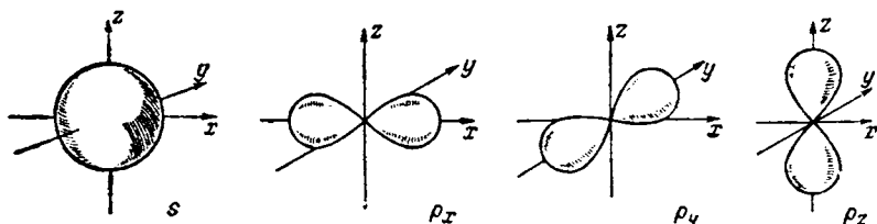
Рис. X-25. Схема направленности орбиталей.
