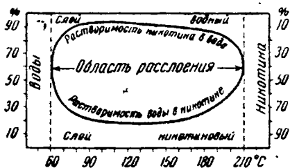
Рис. V-4. Система никотин — вода.
