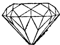
Рис. X-7. Обычная огранка бриллианта.
