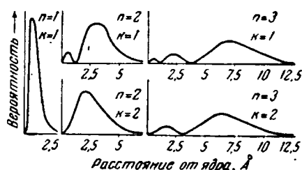
Рис. III-29. Распределение вероятностей нахождения электрона в атоме водорода.
