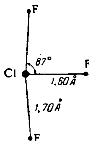
Рис. VII.7. Строение молекулы \text{ClF}_3 .
