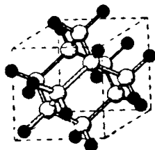
Рис. X-28. Строение молекулы адамантана.
