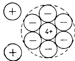
Рис. IX-18. Схема структуры \text{Na}_2[\text{SiF}_6]
