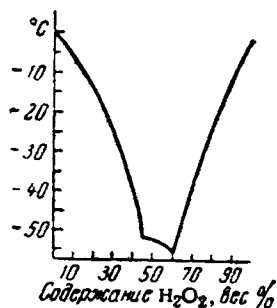
Рис. IV-28. Температуры замораживания водных растворов \text{H}_2\text{O}_2 .
