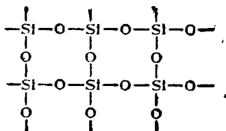
Рис. X-50. Схема структуры двуокиси кремния.
