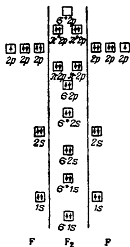
Рис. VI-7. Схема атомных и молекулярной орбит фтора.
