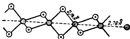
Рис. X-55. Строение кристаллического \text{SiS}_2 .
