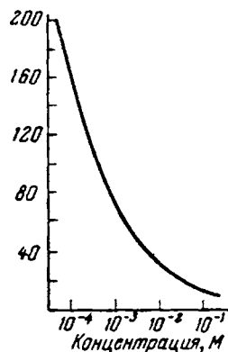
Рис. V-20. Среднее расстояние между растворенными частицами, А.
