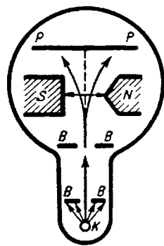
Рис. VI-2. Схема опыта с атомами серебра.
