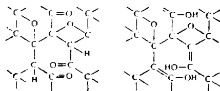
Рис. X-11. Схемы структуры слоев в продуктах окисления графита.
