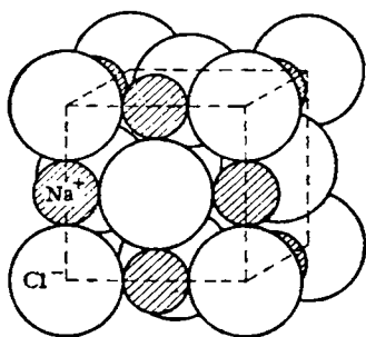
Рис. III-59. Упаковка ионов в кристалле NaCl.
