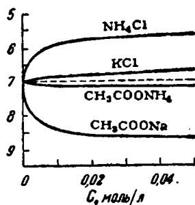
Рис. V-28. Значения pH в разбавленных растворах солей.
