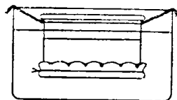
Рис. X-66. Простейший диализатор.
