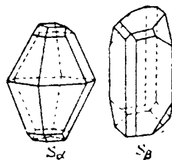
Рис. VIII-11. Характерные формы кристаллов серы.
