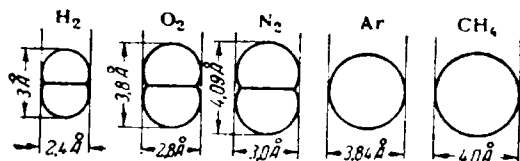
Рис. X-57. Критические размеры некоторых молекул.
