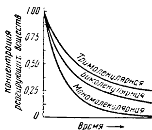
Рис. IV-6. Зависимость хода протекания реакции от ее молекулярности.
