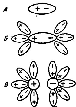
Рис. V-12. Схема перехода полярной структуры в ионную.
