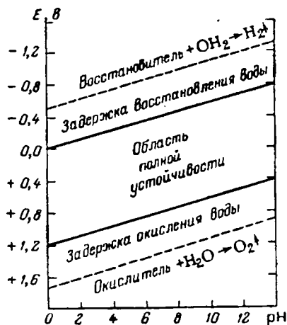
Рис. VII-21. Устойчивость восстановителей и окислителей в водной среде.
