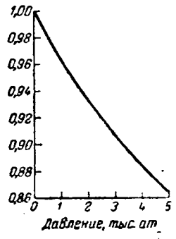
Рис. IV-21. Относительный объем воды.
