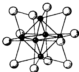
Рис. IX-68. Схема строения группировки \text{Э}_6\text{Cl}_{12} .
