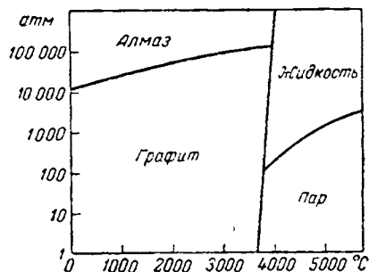
Рис. X-1. Диаграмма состояния углерода.
