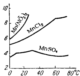
Рис. VII-23. Растворимость солей марганца (моль/л \text{H}_2\text{O} ).
