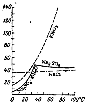
Рис. V-1. Кривые растворимости (г на 100 г \text{H}_2\text{O} ).
