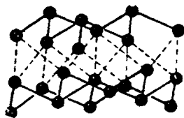
Рис. IX-53. Схема структуры слоя в кристаллах As, Sb и Bi.
