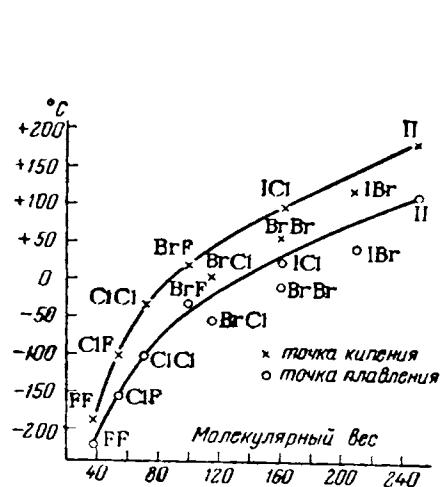
Рис. VII-15. Плавкость и летучесть галидов Г 2 .
