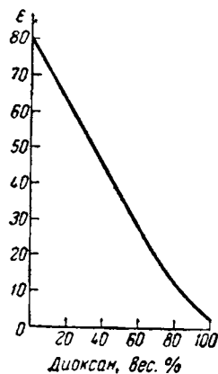
Рис. X-34. Диэлектрические проницаемости в системе вода — диоксид (при 20^\circ\text{C} ).
