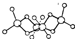
Рис. VIII-33. Схема строения (\text{SeO}_3)_4 .
