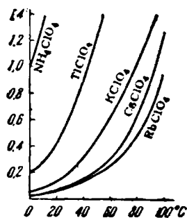
Рис. VII-6. Растворимость некоторых перхлоратов (моль/л \text{H}_2\text{O} ).
