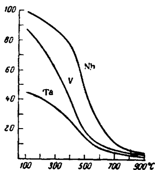
Рис. IX-65. Растворимость водорода в металлах подгруппы ванадия ( см^3/г ).
