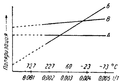
Рис. III-54. Зависимость поляризации молекулы от температуры.
