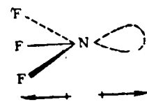
Рис. IX-16. Схема формирования дипольного момента \text{NF}_3 .
