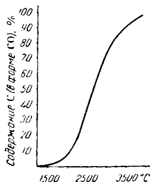
Рис. X-18. Равновесие 2\text{CO} + \text{O}_2 \rightleftharpoons 2\text{CO}_2 .
