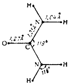
Рис. X-16. Строение молекулы карбамида.
