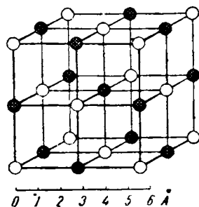
Рис. III-60. Схема строения кристалла NaCl.
