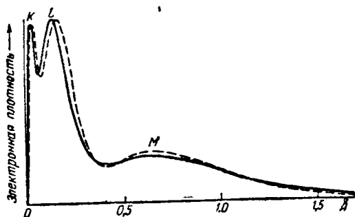
Рис. III-30. Распределение электронной плотности в атоме аргона.
