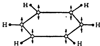
Рис. X-30. Схема строения молекулы бензола.
