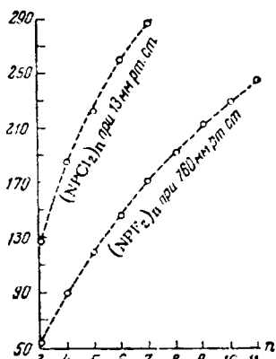
Рис. IX-52. Температуры кипения фосфонитригалогенидов, ^\circ\text{C} .
