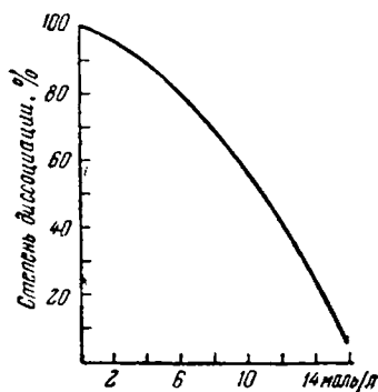
Рис. IX-29. Электролитическая диссоциация \text{HNO}_3 .
