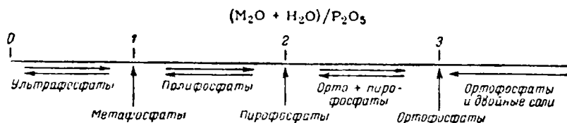
Рис. IX-43. Схема общей классификации фосфатов.
