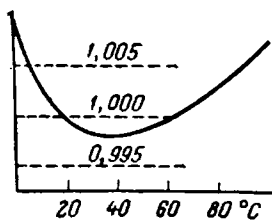
Рис. IV-17. Изменение относительной теплоемкости воды с температурой.
