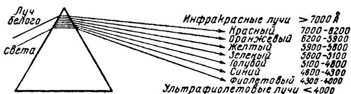
Рис. II-9. Разложение солнечного луча призмой.
