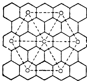
Рис. X-12. Схема координации в \text{C}_8\text{K} .
