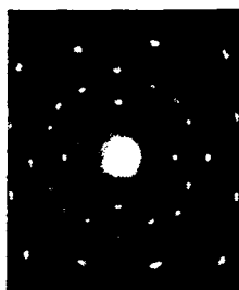
Рис. III-57. Рентгенограмма кристалла MgO .
