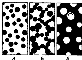
Рис. X-70. Схема последовательных стадий образования геля.
