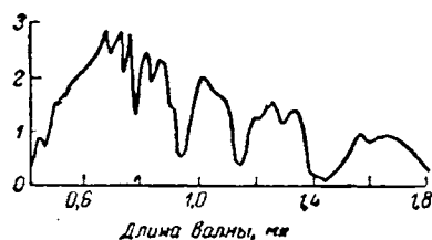
Рис. X-45. Распределение энергии солнечного света на уровне моря (в относительных единицах).
