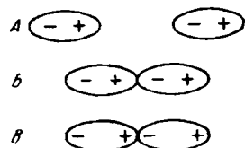
Рис. III-49. Схема взаимодействия двух полярных молекул.
