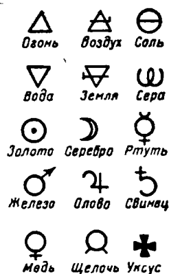
Рис. 1-4. Алхимические обозначения.
