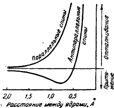
Рис. III-37. Энергия взаимодействия при сближении двух атомов водорода.
