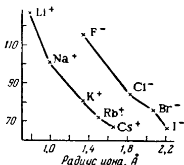
Рис. V-39. Энергии гидратации катионов и анионов (ккал/моль).
