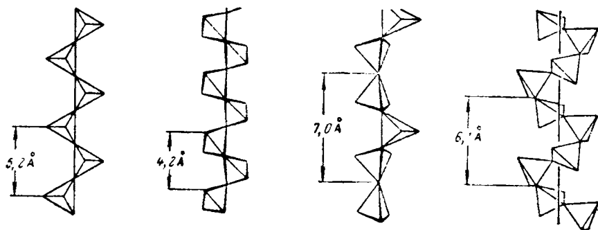
Рис. IX-42. Типы строения цепных полифосфатов.
