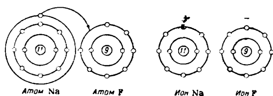
Рис. III-33. Схема образования молекулы \text{NaF} по Косселю.
