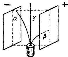
Рис. III-3. Расщепление радиоактивного излучения в электрическом поле.
