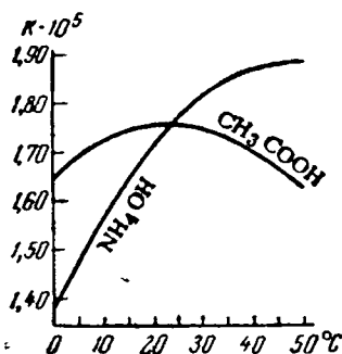
Рис. V-18. Зависимость констант диссоциации от температуры.
