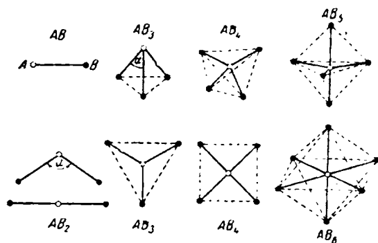
Рис. III-43 Типы пространственных структур молекул AB_n .
