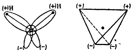
Рис. IV-15. Тетраэдрическая модель молекулы воды.
