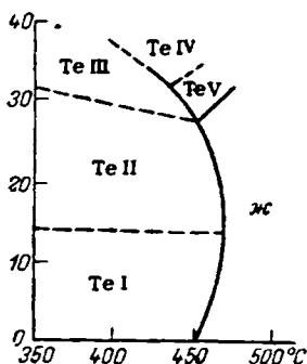
Рис. VIII-31. Диаграмма состояния теллура при высоких давлениях (тыс. ат).
