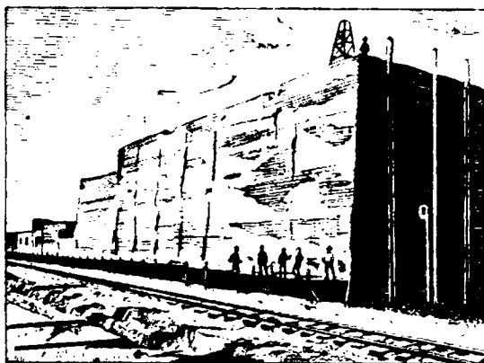
Рис. VIII-8. Массив серы, полученной путем подземной выплавки.
