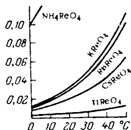
Рис. VII-25. Растворимость некоторых перренатов (моль/л \text{H}_2\text{O} ).
