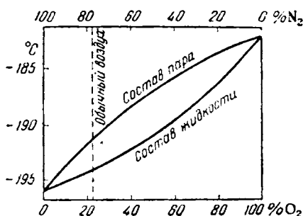
Рис. II-6. Температуры кипения и состав жидкого воздуха.
