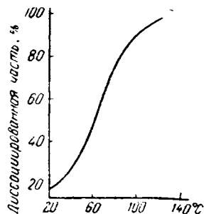
Рис. IX-20. Равновесие системы \text{N}_2\text{O}_4 \rightleftharpoons 2\text{NO}_2 .
