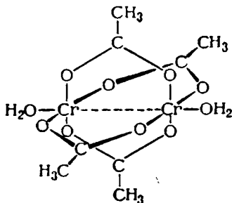
Рис. VIII-39. Схема строения \text{Cr}_2(\text{CH}_3\text{COO})_4 \cdot 2\text{H}_2\text{O} .
