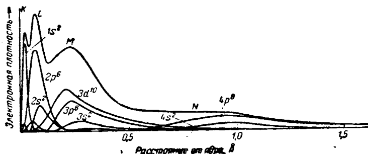
Рис. VI-3. Распределение электронной плотности в атоме рубидия.
