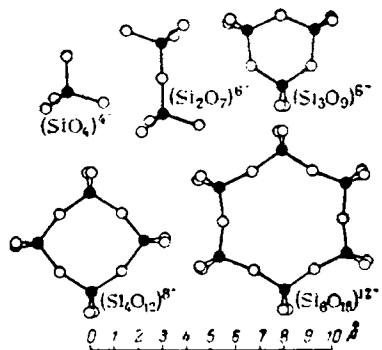
Рис. X-58. Строение простейших силикатных анионов.
