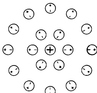
Рис. V-32. Схема гидратации иона.
