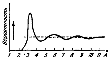
Рис. III-67. Распределение атомов в жидкой ртути.
