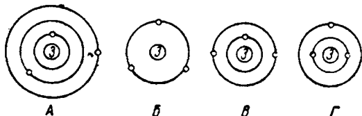
Рис. III-18. Возможные модели атома лития.
