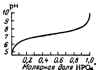
Рис. V-25. Характеристика фосфатного буфера.
