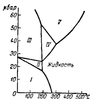
Рис. IX-55. Диаграмма состояния висмута.
