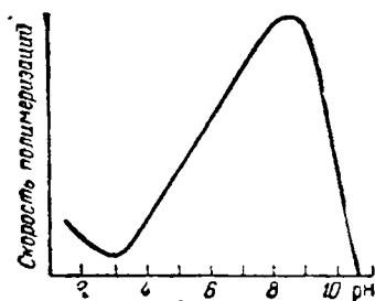
Рис. X-68. Относительная скорость полимеризации кремневой кислоты.
