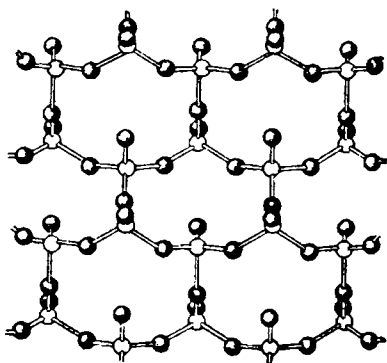
Рис. IX-40. Схема структуры третьей формы \text{P}_2\text{O}_5 .
