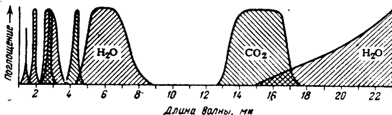
Рис. X-46. Основные области поглощения инфракрасных лучей углекислым газом и водяным паром.
