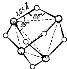
Рис. IX-36. Пространственная структура молекулы \text{P}_4\text{O}_6 .
