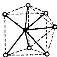
Рис. IX-67. Схема строения иона [\text{NbF}_7]^{2-} .
