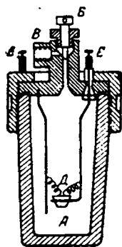
Рис. X-27. Калориметрическая бомба.
