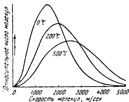
Рис. IV-2. Кривые распределения скоростей молекул водорода.
