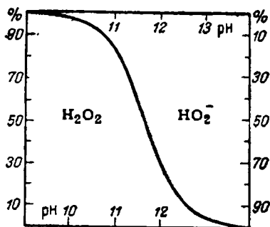
Рис. V-24. Диаграмма электролитической диссоциации \text{H}_2\text{O}_2 .
