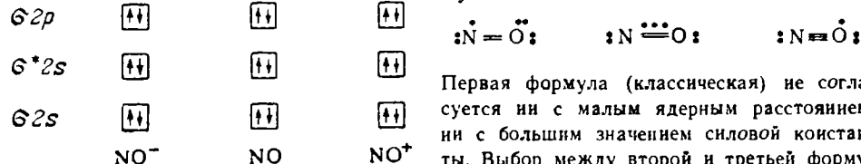
Рис. IX-22 Молекулярные орбиты окиси азота.
