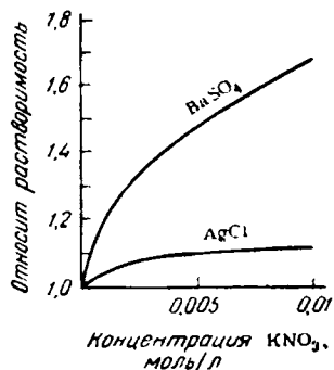
Рис. V-26. Влияние нейтральной соли на растворимость.
