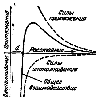
Рис. III-52. Схема сил притяжения и отталкивания.
