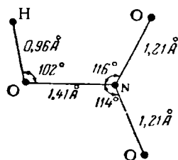
Рис. IX-26. Строение молекулы \text{HNO}_3 .
