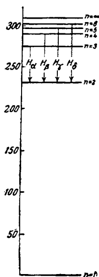
Рис. III-24. Уровни энергии атома водорода (ккал/г-атом).
