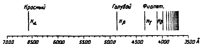
Рис. III-21. Видимый спектр водорода (серия Бальмера).
