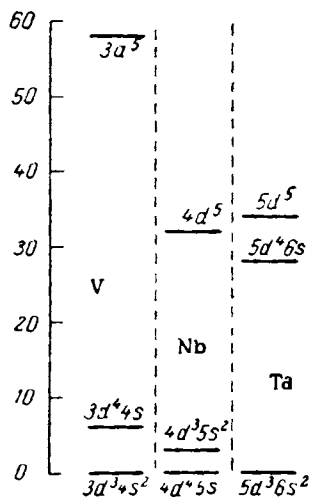
Рис. IX.64. Энергетические уровни атомов V, Nb и Ta (ккал-г-атом).
