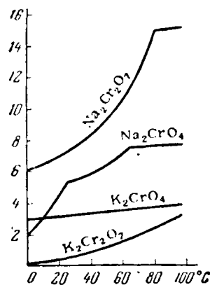
Рис. VIII-34. Растворимость хроматов и бихроматов (моль/л \text{H}_2\text{O} ).
