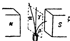
Рис. III-4. Расщепление радиоактивного излучения в магнитном поле.
