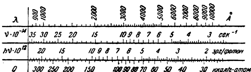
Рис. III-27. Даныи воли и энергии излучения.
