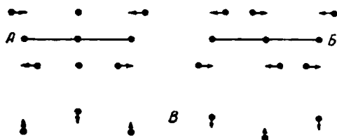
Рис. III-46. Типы колебаний в линейной трехатомной молекуле.
