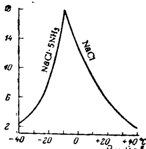
Рис. IX-8. Растворимость \text{NaCl} в жидком аммиаке (г/100 г \text{NH}_3 ).
