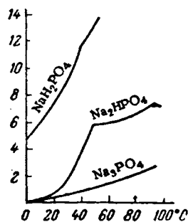
Рис. IX-34. Растворимость фосфатов натрия (моль/л \text{H}_2\text{O} ).
