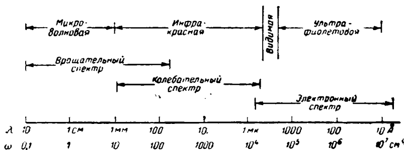
Рис. III-44. Области электромагнитного спектра.
