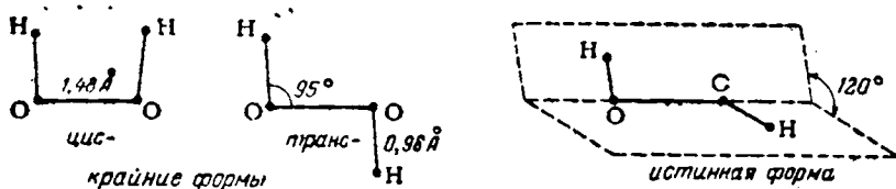
Рис. IV-27. Пространственная структура молекулы \text{H}-\text{O}-\text{O}-\text{H} .
