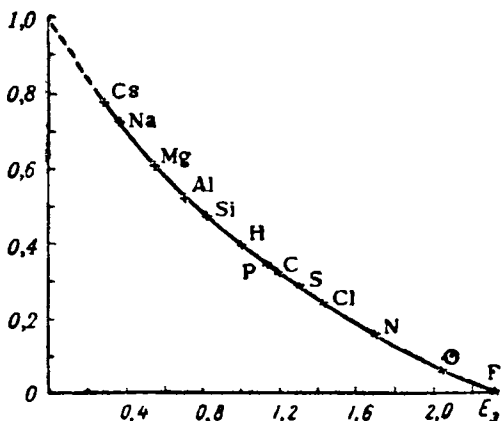
Рис. III-39. Расчетная полярность связей Э—F в молекулах фторадов.
