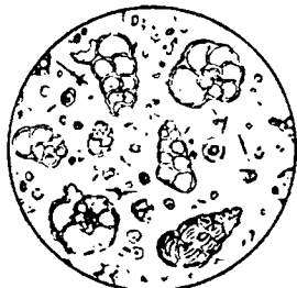
Рис. IV-26. Мел под микроскопом.
