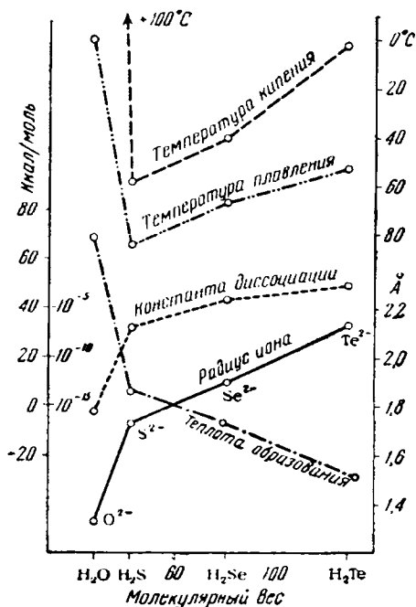
Рис. VIII-28. Свойства водородных соединений элементов VI группы.
