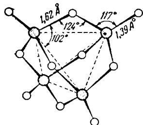
Рис. IX-38. Пространственная структура молекулы \text{P}_4\text{O}_{10} .
