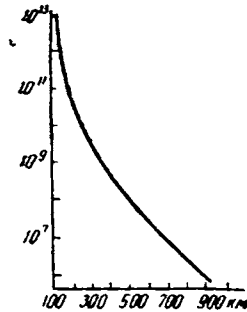
Рис. 11-3. Изменение плотности атмосферы с высотой (атомов/см 3 ).
