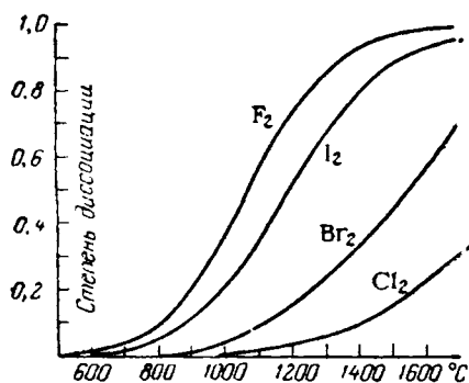
Рис. VII-13. Термическая диссоциация галогенов.
