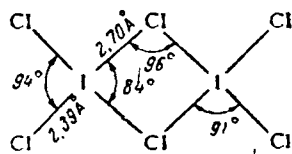
Рис. VII-17. Строение \text{I}_2\text{Cl}_6 .
