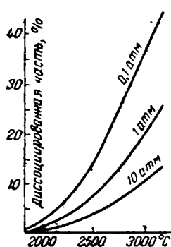
Рис. IV-5. Равновесие термической диссоциации воды.
