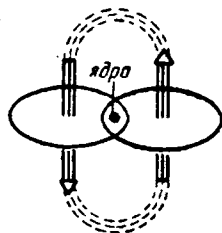
Рис. III-32. Схема замыкания магнитных полей в атоме гелия.
