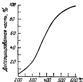
Рис. IX-23. Равновесие термической диссоциации \text{NO}_2 .
