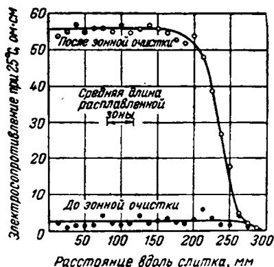
Рис. X-77. Результаты очистки германия зонной плавкой.
