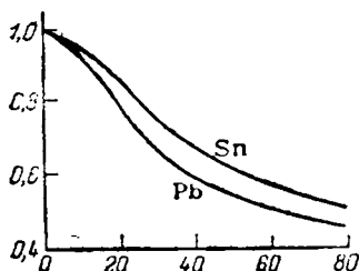
Рис. X-74. Влияние давления (тыс. ат) на относительное электросопротивление олова и свинца.
