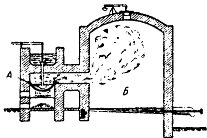
Рис. VIII-1. Печь для перегонки серы.
