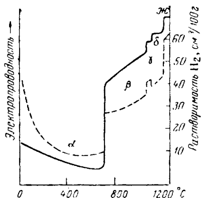
Рис. VII-24. Зависимость электропроводности марганца (сплошная линия) и растворимости в нем водорода (пунктирная линия) от температуры.
