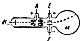
Рис. III-5. Схема установки для исследования катодных лучей.
