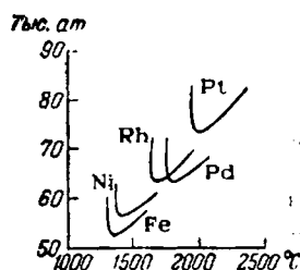
Рис. X-8. Области синтеза алмазов при разных катализаторах.
