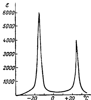
Рис. X-37. Зависимость диэлектрической проницаемости сегнетовой соли от температуры (в слабых полях).
