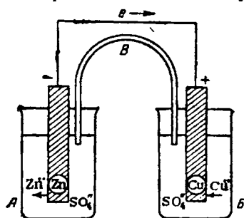
Рис. V-29. Схема гальванического элемента.
