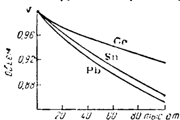
Рис. X-73. Сжимаемость элементов подгруппы германия.
