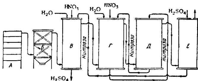
Рис. VIII-25. Схема башенного метода получения серной кислоты.
