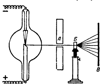
Рис. III-56. Схема рентгеновского исследования кристаллов.
