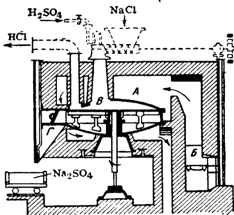
Рис. VII-9. Схема механизированной печи для получения \text{HCl} .
