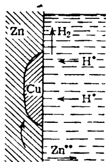
Рис. V-33. Схема действия гальванической пары.
