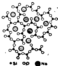
Рис. X-61. Схема структуры натрий-силикатного стекла.
