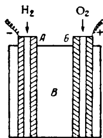
Рис. V-37. Принципиальная схема водородно-кислородного элемента.
