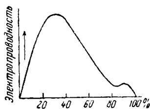
Рис. VIII-4. Электропроводность растворов серной кислоты.
