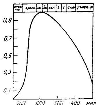
Рис. VIII-30. Относительная спектральная чувствительность селена.
