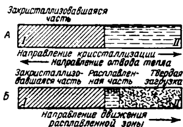
Рис. X-76. Схема очистительной кристаллизации.
