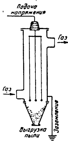
Рис. X-71. Схема электрофильтра.
