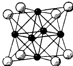
Рис. VIII-40. Схема строения иона [\text{Mo}_6\text{Cl}_8]^{4+} .
