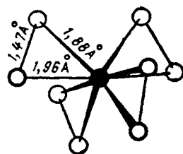
Рис. VIII-37. Строение иона CrO_5^{3-} .
