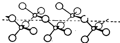
Рис. VIII-17. Схемы цепи (\text{SO}_3)_n .
