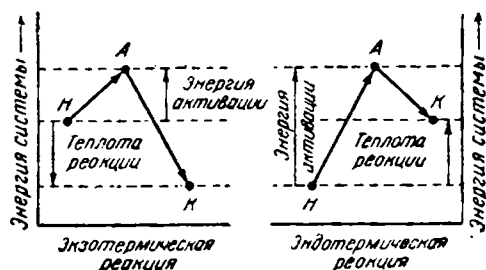
Рис. IV-7. Схема протекания активированных реакций.
