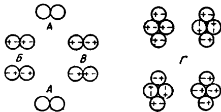
Рис. III-51. Схема модельной трактовки дисперсионного взаимодействия.
