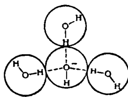
Рис. V-16. Схема строения иона \text{H}_7\text{O}_4^- .
