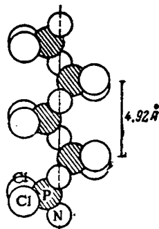
Рис. IX-51. Структура цепи фосфонитрилхлорида.
