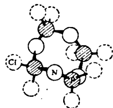
Рис. IX-50. Строение молекулы (\text{NPCl}_2)_4 .
