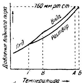
Рис. V-7. Давление пара воды и раствора.
