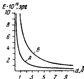
Рис. III-53. Энергия взаимодействия однозарядных (А) и двухзарядных (Б) частиц.
