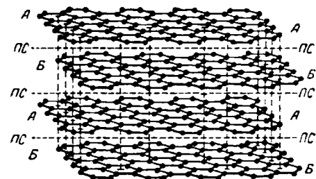
Рис. X-9. Схема расположения атомов C в графите.
