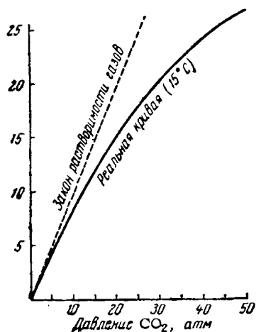
Рис. V-3. Зависимость растворимости углекислого газа от давления (объемы на 1 объем воды).
