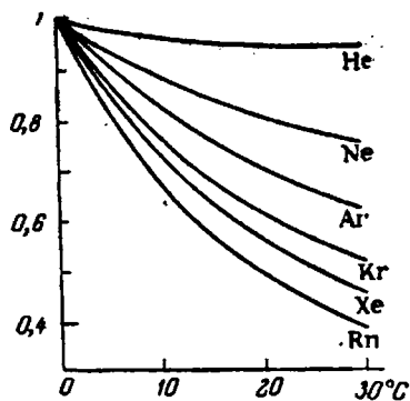
Рис. II-12. Изменение относительной растворимости инертных газов с температурой.
