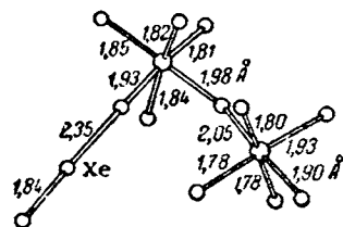
Рис. IX-61. Строение \text{XeF}_2 \cdot 2\text{SbF}_5 .
