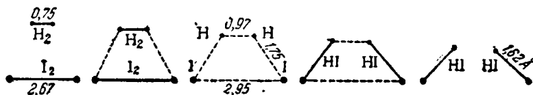
Рис. IV-8. Схема хода реакции H_2 + I_2 \rightleftharpoons 2HI .
