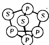
Рис. IX-47. Строение молекулы \text{P}_4\text{S}_3 .
