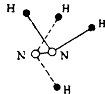
Рис. IX-17. Конформация молекулы гидразина.
