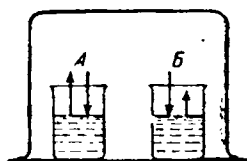
Рис. V-9. Перенос растворителя.
