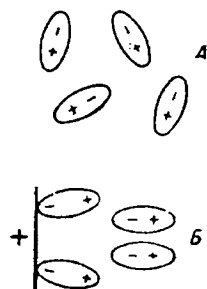
Рис. III-48. Поляризация полярных молекул
