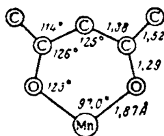
Рис. X-35. Схема координации атомов в ацетилацетонатах Mn и Cr.
