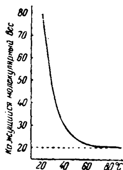
Рис. VII-3. Зависимость ассоциации HF от температуры.
