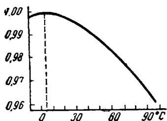
Рис. IV-11. Изменение плотности воды с температурой ( \text{г/см}^3 ).
