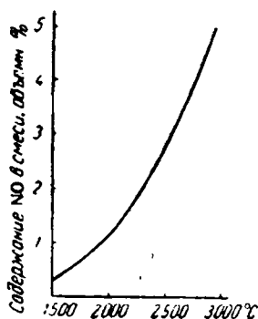
Рис. IX-19. Равновесие синтеза окиси азота.
