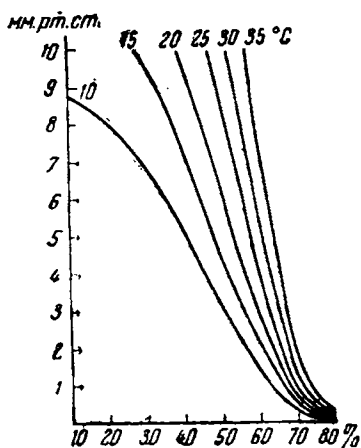
Рис. VIII-20. Давление водяного пара над растворами \text{H}_2\text{SO}_4 .
