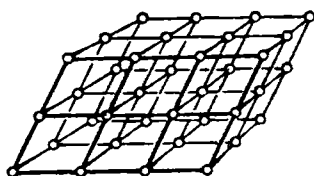
Рис. III-55. Пример пространственной решетки.
