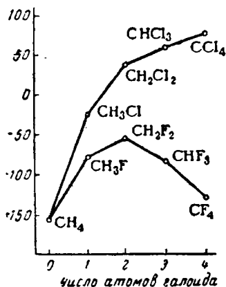
Рис. X-21. Температуры кипения фтор- и хлорметанов, ^\circ\text{C} .
