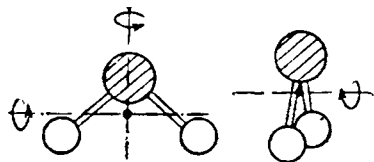
Рис. III-45. Схема типов вращения AB_2
