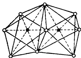
Рис. VIII-38. Схема строения иона [\text{W}_2\text{Cl}_9]^{3-} .
