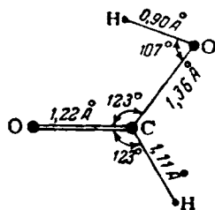
Рис. X-36. Строение молекулы муравьиной кислоты.
