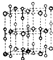
Рис. X-5. Структура кристалла \text{CaC}_2 .
