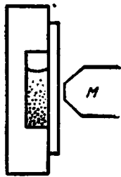
Рис. III-2. Схема опыта Перрена.
