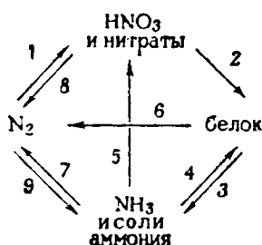
Рис. IX-31. Схема круговорота азота.
