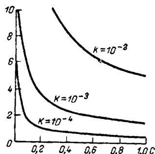
Рис. V-19. Процентная ошибка расчета по формуле [H^+] = \sqrt{K \cdot C} .
