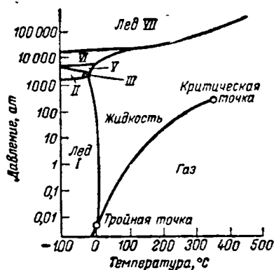
Рис. IV-25. Полная диаграмма состояния воды.
