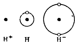
Рис. IV-1. Схема атома и ионов водорода.
