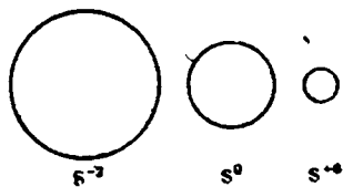
Рис. III-61. Влияние валентного состояния на размеры атома.
