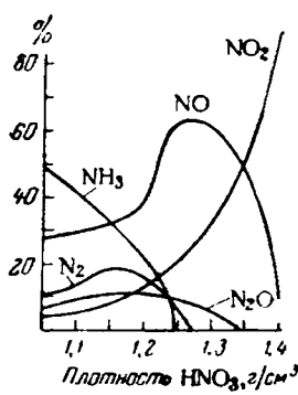
Рис. IX-30. Продукты восстановления \text{HNO}_3 железом.
