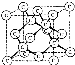
Рис. X-6. Схема расположения атомов C в алмазе.
