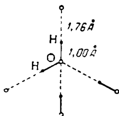
Рис. IV-22. Схема распределения связей в кристалле льда.
