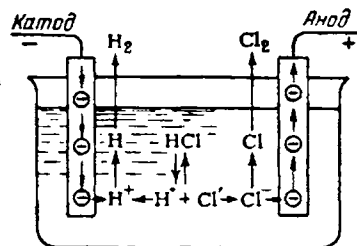
Рис. V-31. Схема электролиза.
