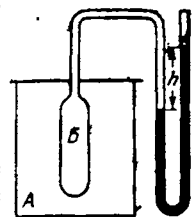
Рис. V-8. Аналогия между осмотическим и газовым давлениями.
