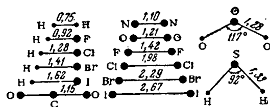
Рис. III-42. Расположение атомных ядер в некоторых простейших молекулах.
