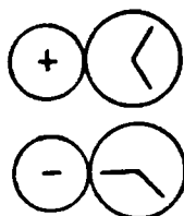
Рис. V-40. Схема ориентации молекул воды.
