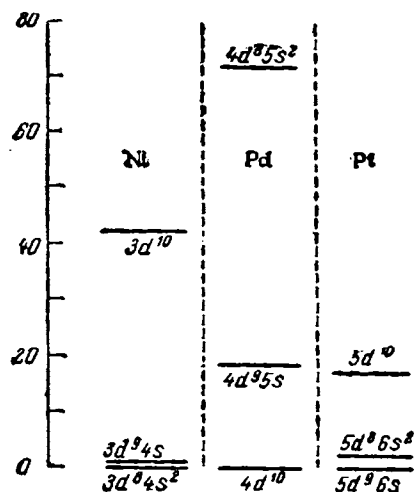
Рис. VI-5. Энергетические уровни атомов Ni, Pd, Pt (ккал/(г-атом)).
