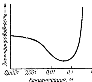
Рис. IX-10. Электропроводность растворов \text{Na} в жидком аммиаке.
