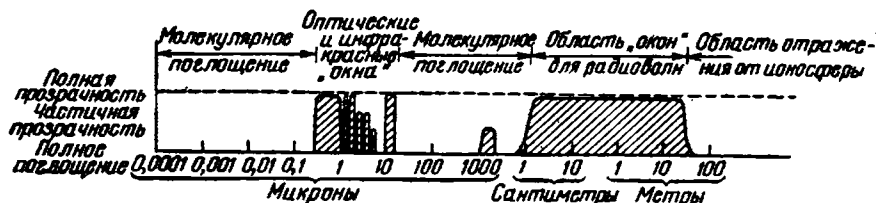
Рис. III-20. Взаимодействие различных волн с атмосферой.
