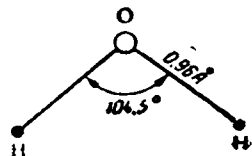
Рис. IV-10. Расположение атомных ядер в молекуле воды.
