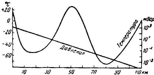
Рис. 11-2. Основные характеристики верхней атмосферы.
