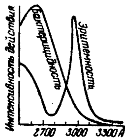
Рис. 11-10. Биологическая активность ультрафиолетовых лучей.
