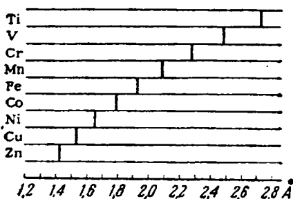
Рис. III-15. Длины волн рентгеновских лучей для элементов от Ti до Zn.
