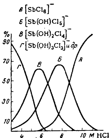
Рис. IX-62. Состав солянокислых растворов \text{SbCl}_5 .
