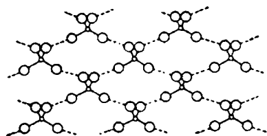
Рис. VIII-18. Схема водородных связей в кристалле \text{H}_2\text{SO}_4 .
