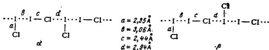
Рис. VII-16. Цепи в кристалле иодхлорида.
