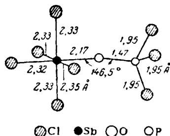
Рис. IX-63. Строение SbCl_5 \cdot OPCl_3 .
