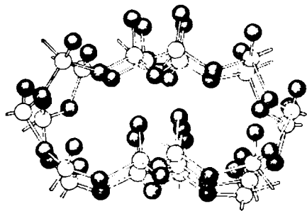
Рис. IX-39. Схема структуры второй формы \text{P}_2\text{O}_5 .
