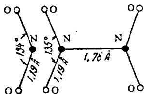
Рис. IX-21. Пространственное строение молекулы \text{NO}_2 и \text{N}_2\text{O}_4 .
