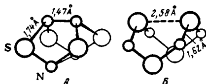
Рис. IX-13. Схемы возможных структур молекулы \text{S}_4\text{N}_4 .
