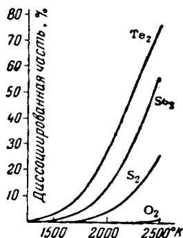
Рис. VIII-32. Термическая диссоциация молекул \text{Te}_2 .
