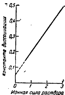
Рис. V-17. Диссоциация иона \text{TiNO}_3^+ .
