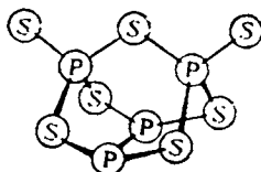
Рис. IX-48. Строение молекулы \text{P}_4\text{S}_7 .
