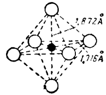
Рис. X-51. Схема координации кремния в стишовите.
