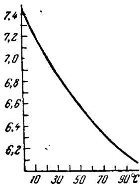
Рис. V-23. Зависимость pH нейтральной среды от температуры.
