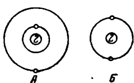
Рис. III-17. Возможные модели атома гелия.
