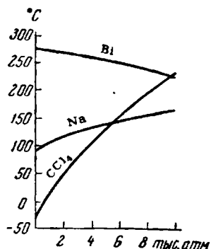
Рис. IX-57. Типичные случаи кризисов плавления.
