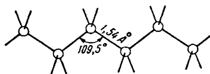
Рис. X-24. Схема строения углеродной цепи.
