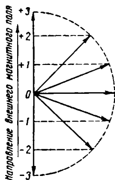
Рис. VI-1. Схема квантования орбитального магнитного момента.
