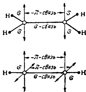
Рис. X-29. Схема валентных связей в этилене и ацетилене.
