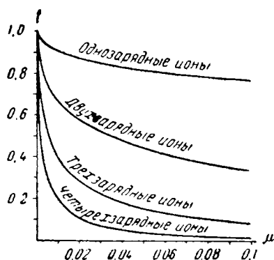
Рис. V-21. Средние коэффициенты активности ионов.
