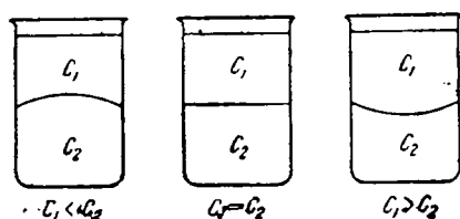
Рис. V-5. Схема осмоса.
