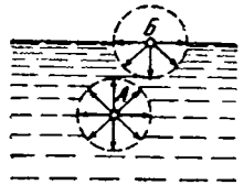
Рис. IV-19. Схема возникновения поверхностного натяжения.
