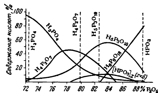
Рис. IX-44. Кислотный состав в системе \text{P}_2\text{O}_5-\text{H}_2\text{O} .
