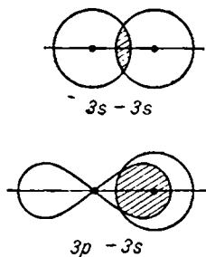
Рис. X-26. Схема перекрывания орбиталей.
