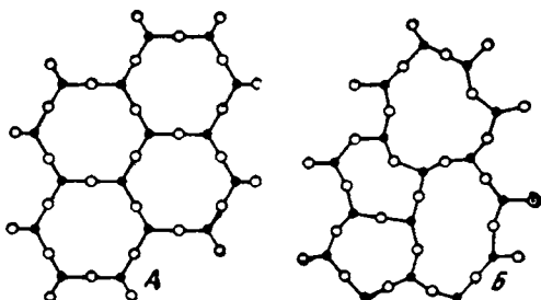
Рис. X-60. Схемы структур \text{Al}_2\text{O}_3 в кристаллическом (А) и стеклообразном (Б) состояниях.
