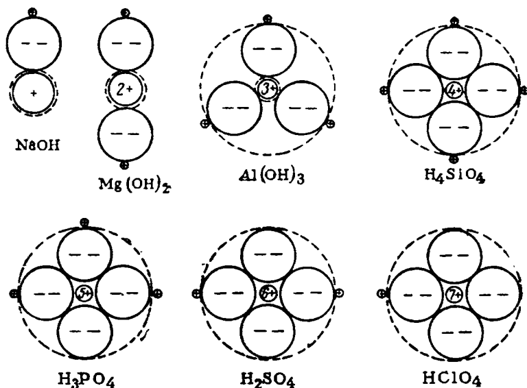
Рис. V-13. Характер диссоциации соединений типа \text{ROH} в зависимости от заряда и радиуса R .
