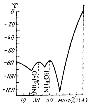
Рис. IX-12. Температуры плавления в системе \text{NH}_3 - \text{H}_2\text{O} .
