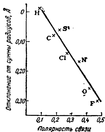
Рис. X-64. Полярность связей Si—X и сокращение ядерных расстояний.
