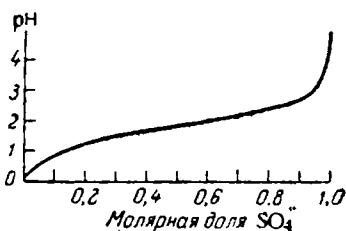
Рис. VIII-22. Характеристика сульфатного буфера.
