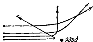
Рис. III-7. Отклонения \alpha -частиц ядром.
