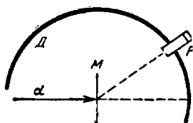
Рис. III-6. Схема опыта Резерфорда.
