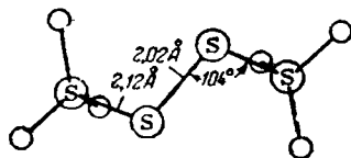
Рис. VIII-15. Строение иона \text{S}_4\text{O}_6^{2-} .
