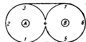
Рис. III-36. Схема модельной трактовки валентных сил.
