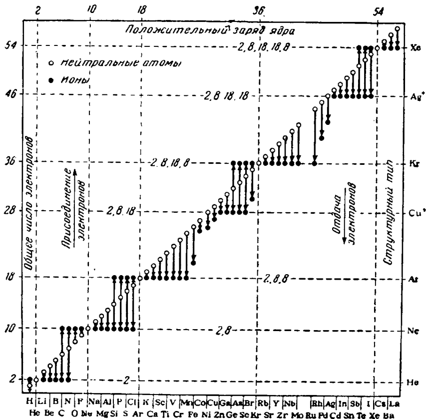
Рис. III-34. Наиболее устойчивые электронные конфигурации.
