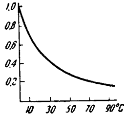
Рис. IV-18. Относительная вязкость воды.
