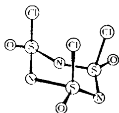
Рис. IX-15. Строение \alpha -формы хлористого сульфамура.
