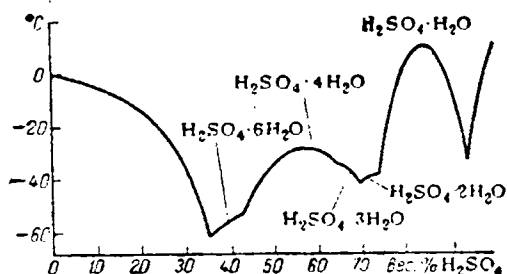
Рис. VIII-19. Температуры плавления в системе \text{H}_2\text{O} \cdot \text{H}_2\text{SO}_4 .
