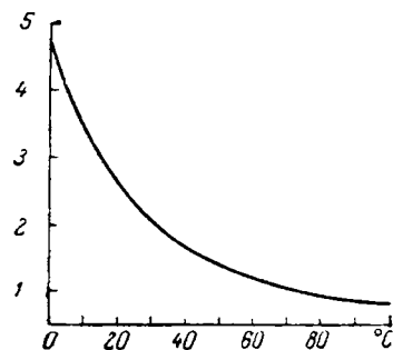
Рис. VIII-2. Растворимость сероводорода (объемы на 1 объем \text{H}_2\text{O} ).
