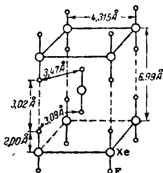
Рис. VII-2. Кристаллическая структура XeF_2 .
