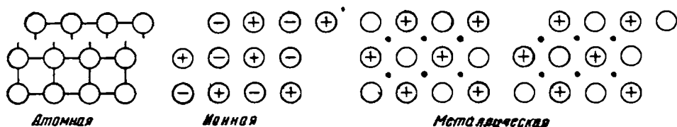
Рис. III-63. Схема сдвига слоев при разных типах структур.
