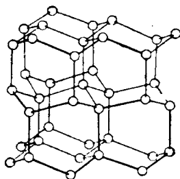
Рис. IV-23. Структурная схема льда.
