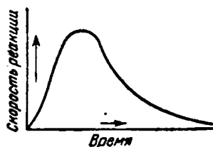
Рис. VII-4. Схема хода аутокаталитической реакции.
