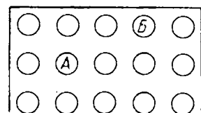
Рис. VII-11. Схема происхождения адсорбционного поля.
