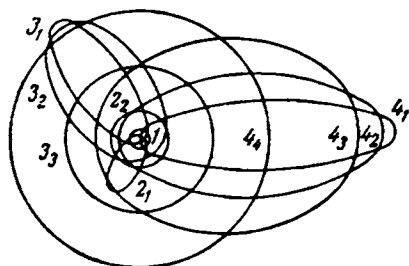
Рис. III-25. Схема возможных электронных орбит атома водорода по Зоммерфельду.
