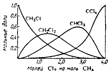
Рис. X-33. Продукты хлорирования метана.
