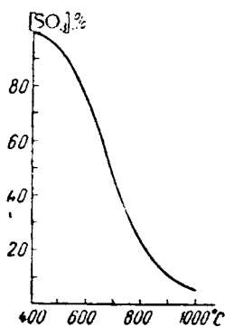
Рис. VIII-3. Равновесные термической диссоциации \text{SO}_3 .
