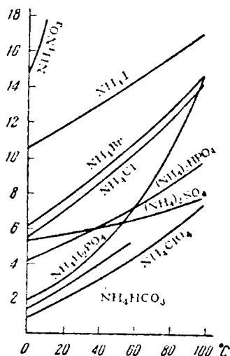
Рис. IX-4. Растворимость солей аммония (моль/л \text{H}_2\text{O} ).
