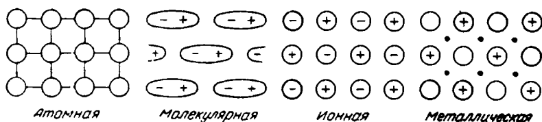
Рис. III-58. Основные типы структур твердого вещества.
