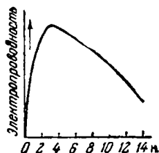
Рис. IX-28. Электропроводность растворов \text{HNO}_3 .
