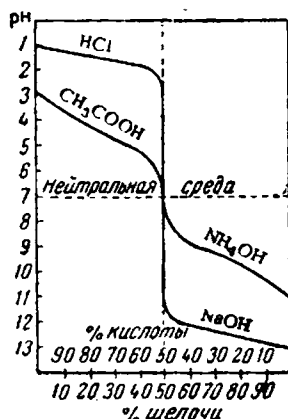
Рис. V-27. Изменение pH при нейтрализации.
