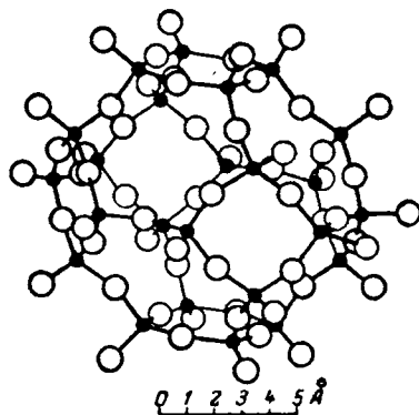
Рис. X-56. Примерная схема цеолитной сетки.
