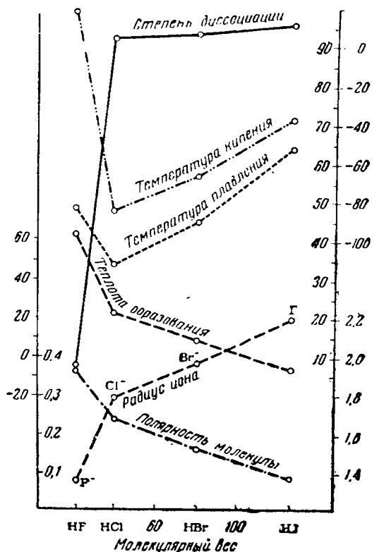
Рис. VII-12. Свойства галоидоводородов.
