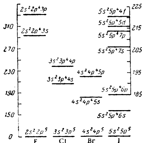
Рис. VII-14. Энергетические уровни атомов галогенов (ккал/г-атом).
