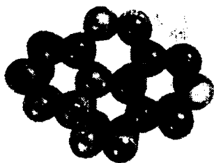
Рис. IV-24. Модель структуры льда.
