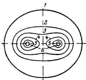
Рис. III-38. Распределение электронной плотности в молекуле \text{H}_2 .
