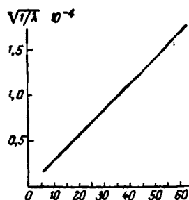
Рис. III-16. Длины волн рентгеновских лучей и атомный номер.
