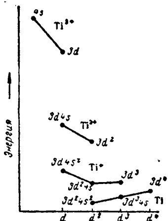
Рис. VI-4. Относительные энергетические уровни атома и ионов титана.
