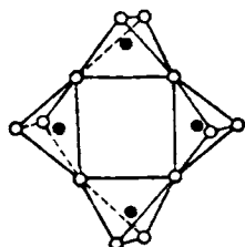
Рис. IX-41. Схема структуры иона \text{P}_6\text{O}_{12}^{4-} .
