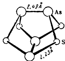
Рис. IX-59. Строение молекулы \text{As}_4\text{S}_4 .
