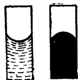
Рис. IV-20. Формы менисков.
