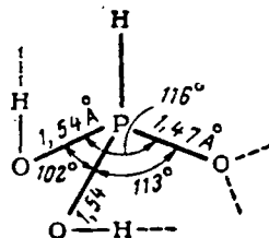
Рис. IX-37. Строение молекулы \text{H}_3\text{PO}_3 .
