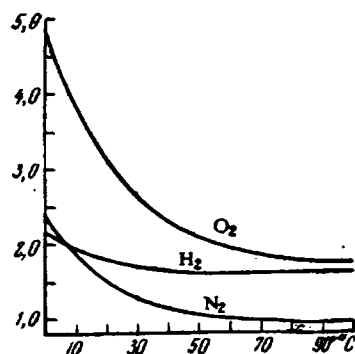
Рис. V-2. Растворимость некоторых газов (объемы на 100 объемов воды)
