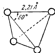
Рис. IX-33. Строение молекулы \text{P}_4 .
