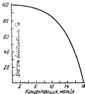
Рис. VII-10 Электролитическая диссоциация \text{HClO}_4 .
