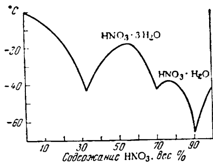
Рис. IX-27. Температуры плавления в системе \text{H}_2\text{O}-\text{HNO}_3 .
