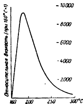
Рис. VIII-12. Изменение вязкости серы с температурой.
