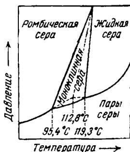
Рис. VIII-10. Диаграмма состояния серы.
