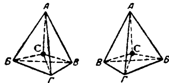
Рис. X-38. Схема стереоизомерии.
