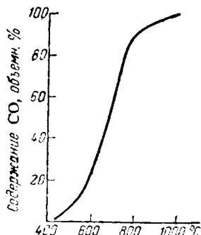
Рис. X-2. Равновесие \text{CO}_2 + \text{C} \rightleftharpoons 2\text{CO} .
