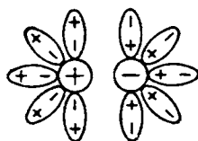
Рис. V-11. Диполи около ионной молекулы.
