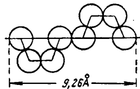
Рис. VIII-13. Вероятное строение цепи S_\mu .
