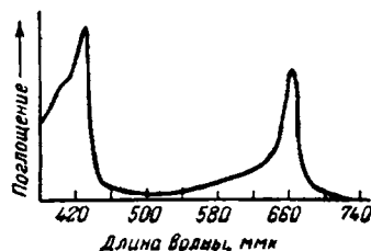
Рис. X-41. Спектр поглощения хлорофилла.
