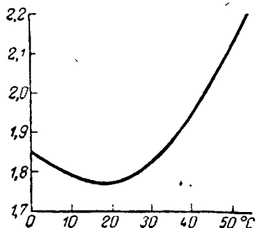
Рис. X-31. Растворимость бензола в воде (г/л).
