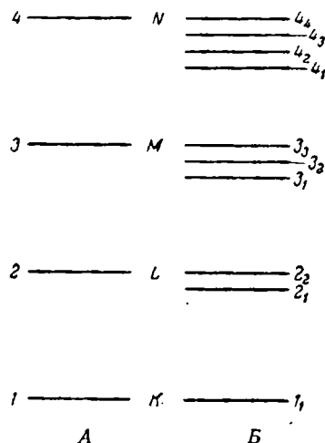
Рис. III-26. Схемы относительных энергетических уровней круговых и эллиптических орбит.
