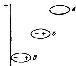
Рис. III-47. Поляризация неполярной молекулы.
