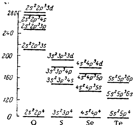
Рис. VIII-29. Энергетические уровни атомов O — Te (ккал/г-атом).
