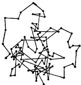
Рис. III-1. Примерный путь частицы газа.
