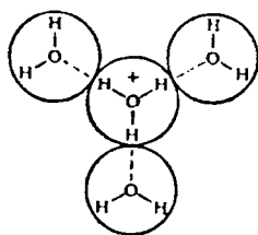
Рис. V-15. Возможная схема строения иона \text{H}_3\text{O}_4^+ .
