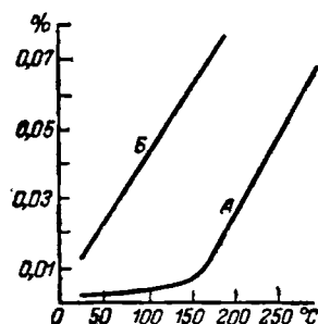
Рис. X-54. Растворимость в воде кварца (A) и аморфного кремнезема (B).
