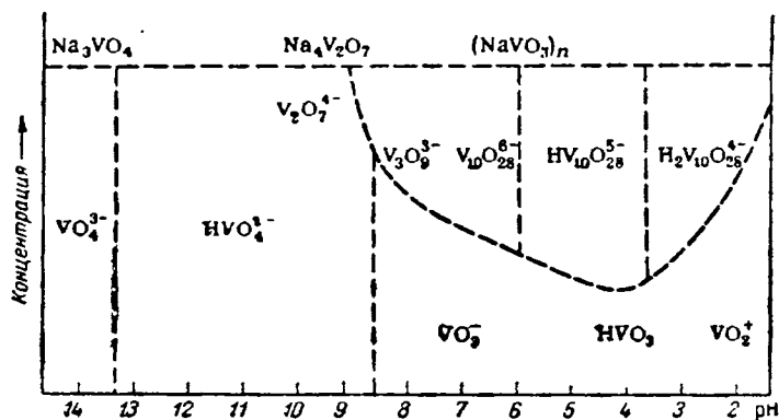
Рис. IX-66. Области существования ванадат-ионов.
