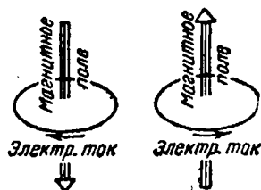
Рис. III-31. Правило буравчика.
