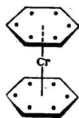
Рис. X-32. Схема строения дибензолхрома.
