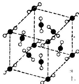
Рис. X-13. Расположение молекул в кристалле двуокиси углерода.
