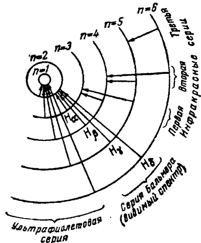
Рис. III-23. Схема происхождения водородного спектра.
