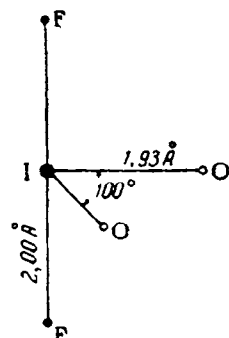
Рис. VII-19. Строение иона \text{IO}_2\text{F}_2^- .
