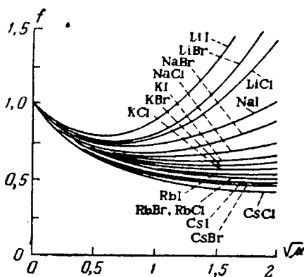
Рис. V-22. Зависимость коэффициентов активности от природы ионов.
