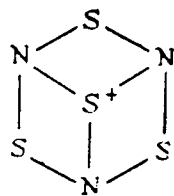
Рис. IX-14. Вероятная структура иона S_4N_3^+ .
