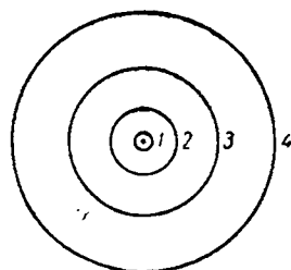
Рис. III-22. Возможные электронные орбиты атома водорода по Бору.
