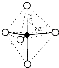
Рис. IX-46. Строение молекулы \text{PCl}_5 .
