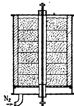
Рис. IX-6. Схема цианамидной печи.
