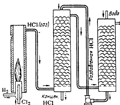
Рис. VII-8. Схема установки для синтеза \text{HCl} .
