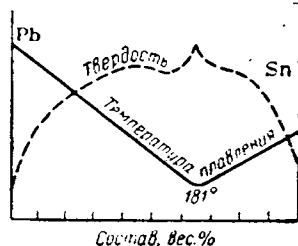
Рис. X-79. Характеристики мягкого припоя.
