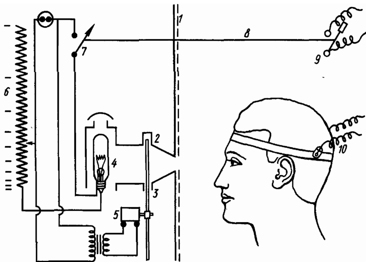
Рис. 103. Установка для исследования изменений основной электрической активности мозга при действии прерывистых раздражений нарастающей интенсивности (по методу М. Н. Ливанова):
