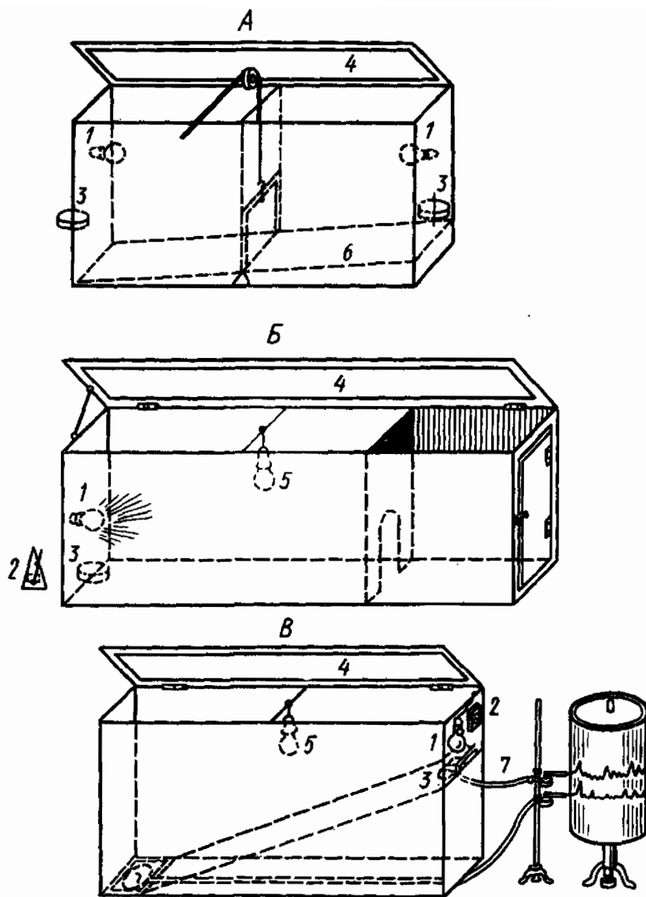
Рис. 91. Камеры для исследования условных рефлексов у мелких грызунов. А — с перекрестным подкреплением (по Ю. П. Фролову); Б — с фиксированным исходным положением животного (по Л. И. Котляровскому); В — с «горкой» у кормушки (по В. К. Фадеевой, А. Ю. Изергиной): 1 — сигнальные лампочки, 2 — звуковые сигналы (звонок, метроном, зуммер), 3 — кормушки, 4 — наклонное зеркало в потолке для наблюдения за животными, 5 — постоянное освещение камеры, 6 — подвижный пол для регистрации перебежек из отделения в отделение, 7 — воздушная передача для регистрации подбегания к кормушке
