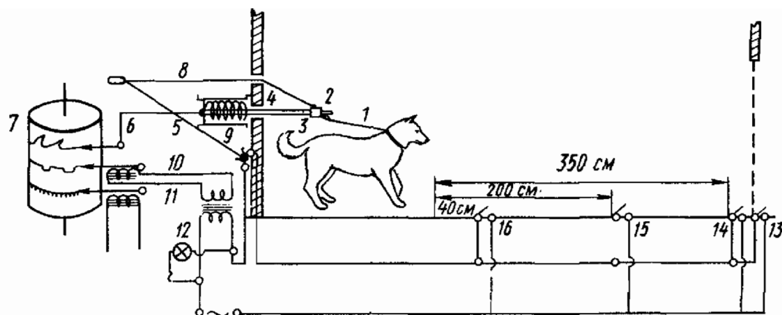
Рис. 58. Установка для быстрой оценки типологических различий служебных собак (по Э. А. Варухе):
