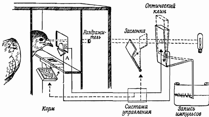
Рис. 25. Схематическое изображение установки для «слежения», применяемой при определении порога восприятия света данной длины волны у голубя [282].
