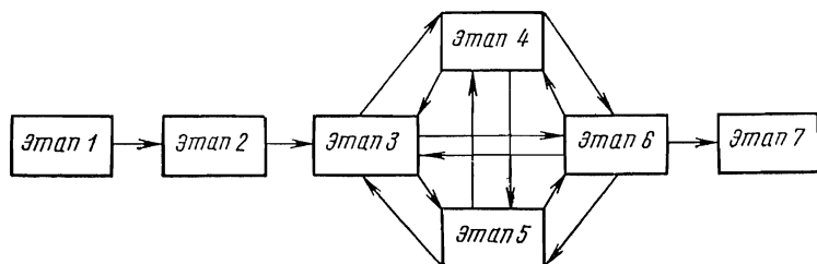
Рис. В.8. Схема хронологически-итерационных взаимосвязей основных этапов статистического исследования зависимостей
