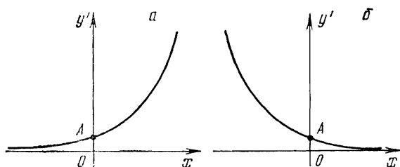
Рис. 6.6. График показательной (экспоненциальной) зависимости вида y' = A e^{bx} : а) случай b > 0 ; б) случай b < 0
