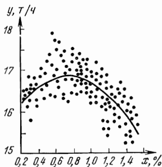
Рис. В.4. Зависимость производительности ( y , т/ч) от процентного содержания углерода ( x , %) в металле до расплавления
