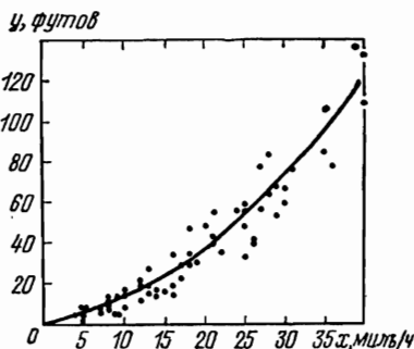
Рис. 6.1. График зависимости тормозного пути автомобиля ( y ) от скорости его движения ( x )
