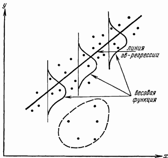
Рис. 7.2. Настройка эв-регрессии на интересующую исследователя часть выборки
