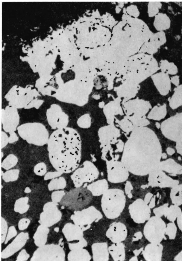
Фото 32. Микрофотография докембрийского пиритово-кварцевого песка из системы Витватерсранд, Южная Африка ( \times 45 ) (гл. XIII, [21]). Зерна пирита — белые, зерна кварца — темные. Вверху — обломок перестроенного более древнего пиритового песка. В этом древнем песчанике еще различимы округлые очертания зерен пирита.
