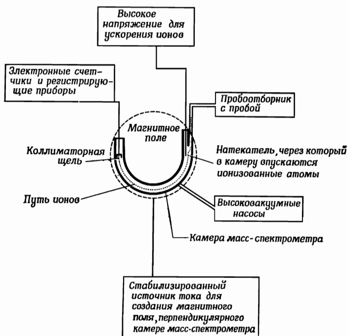
Фиг. 7. Схема газового масс-спектрометра с отклонением на 180^\circ .
