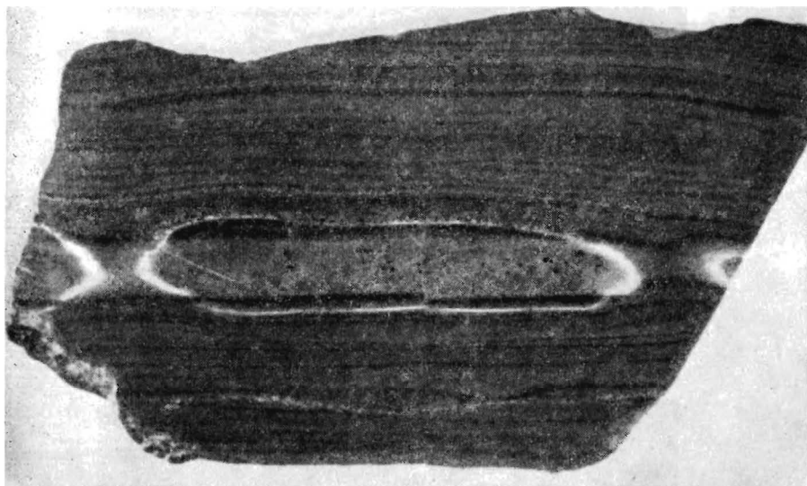
Фото 38. Полированная плитка породы из докембрийской полосчатой железорудной формации вблизи Ишпеминг, на севере штата Мичиган. Очень тонкие прослойки, заметные простым глазом в таких тонкозернистых сланцевых породах, возможно, возникли в результате сезонных изменений процесса седиментации. Более толстый пласт в середине — песчанистая порода. Беловатые прожилки образовались при замещениях, происходивших позднее.
