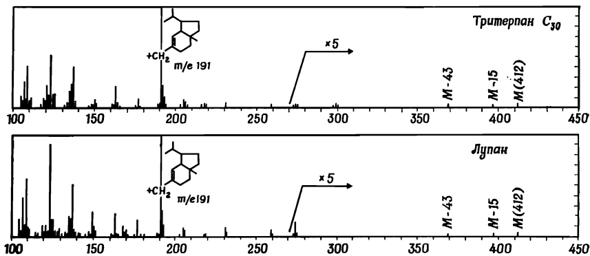
Фиг. 66. Сравнение масс-спектров тритерпанового молекулярного ископаемого C_{30} (мол. масса 412) с масс-спектром синтетического лупана ( C_{30} ) [13].
