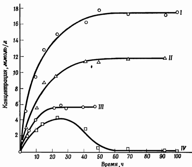
Фиг. 26. Скорость образования аминокислот и других продуктов из водных смесей формальдегида и гидроксиламина [28].
