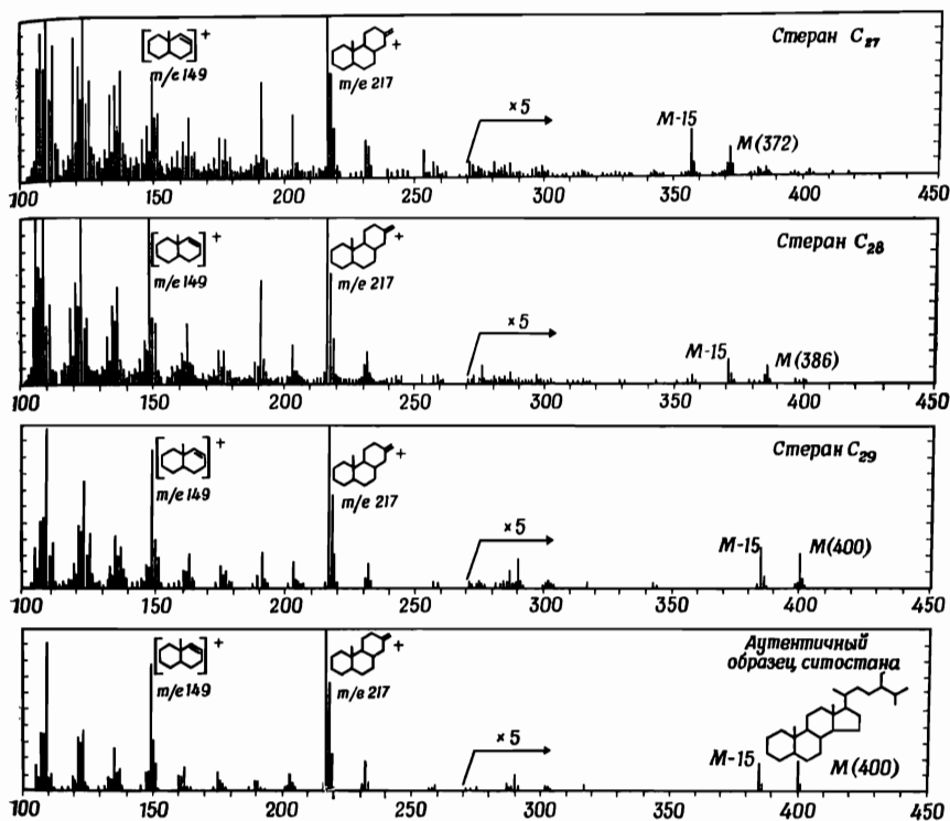
Фиг. 64. Сравнение масс-спектров стерановых молекулярных ископаемых C_{27} (мол. масса 372), C_{28} (мол. масса 386) и C_{29} (мол. масса 400) с масс-спектром стандарта — ситостана ( C_{29} ), синтезированного в лаборатории [13]. Все четыре соединения сначала теряют группу CH_3 ( M-15 ) (мол. масса 15). Образуются довольно стабильные фрагменты с молекулярными массами 217 и 149. Спектры молекулярных ископаемых C_{29} и синтетического ситостана очень сходны, что говорит об их близком родстве.
