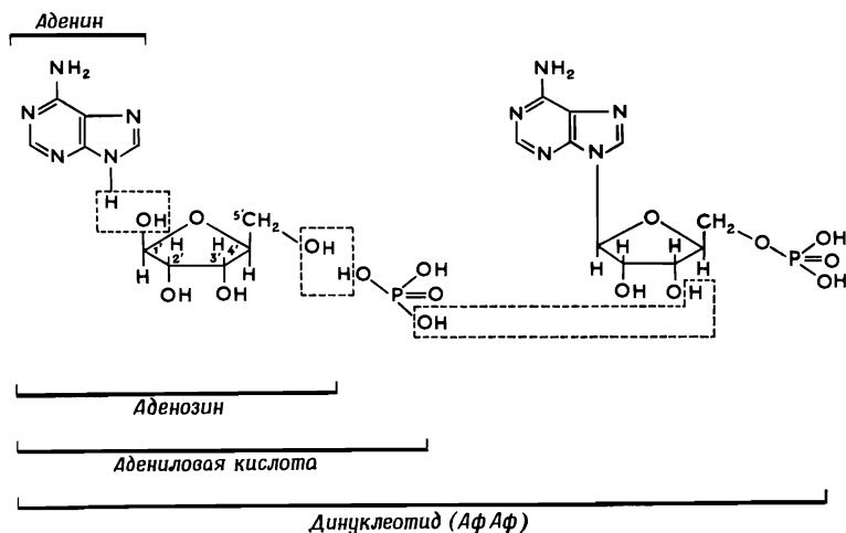
Фиг. 21. Строение цепи нуклеиновой кислоты [3].
