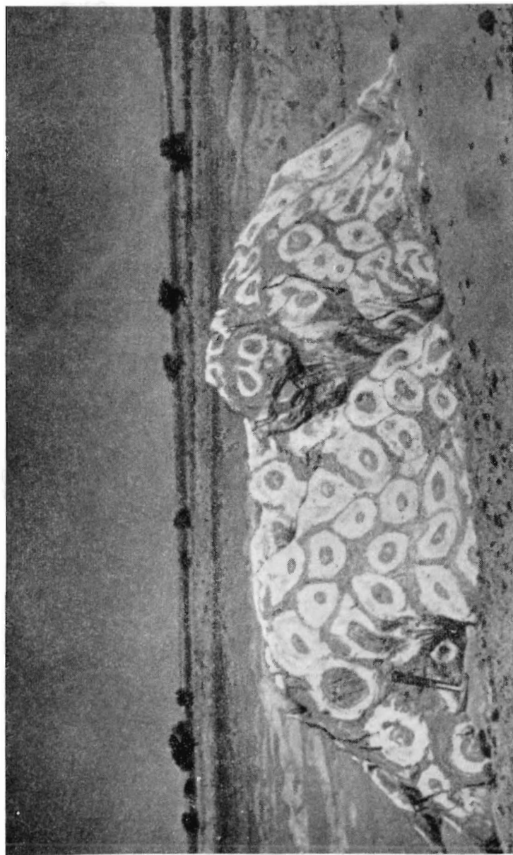
Фото 8. Риф, образованный Sophrhyton (Фарузий); докембрий массива Ахагар, Сахара (гл. XII, [37]).
