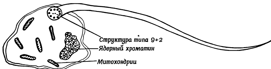
Фиг. 42. Схема первой эукариотической клетки [11].
