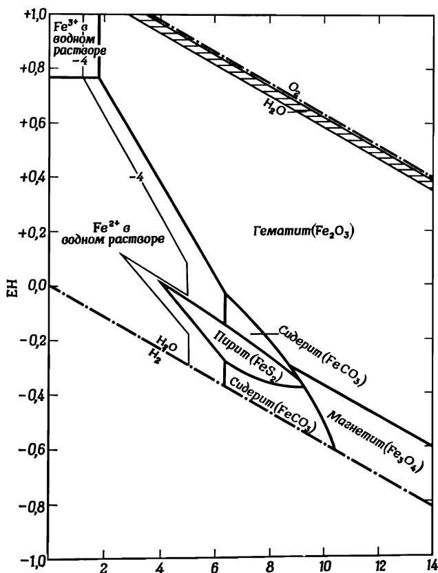
Фиг. 77. Устойчивость окислов, карбонатов, сульфидов и силикатов железа при температуре 25°С и общем давлении 1 атм в присутствии воды [10].
