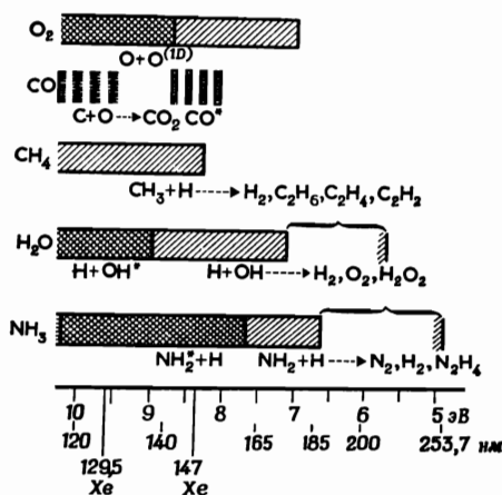
Фиг. 14. Фотохимические реакции, идущие в различных газах при облучении их светом с разной длиной волны.
