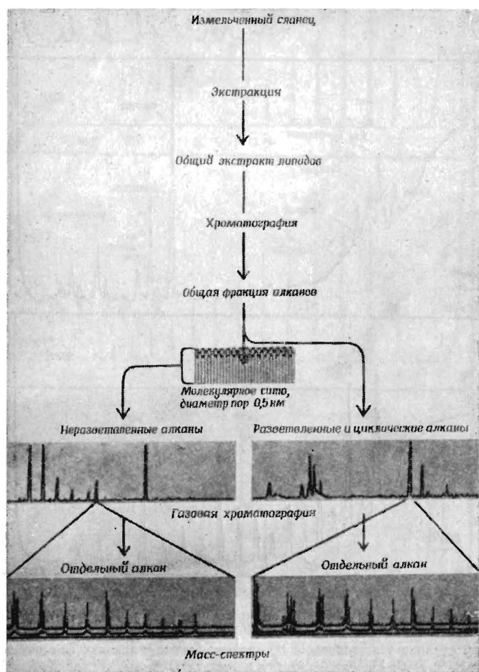
Фиг. 57. Схема анализа химических ископаемых [23].
