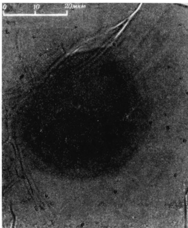
Фото 1. Плеохроичные ореолы.
