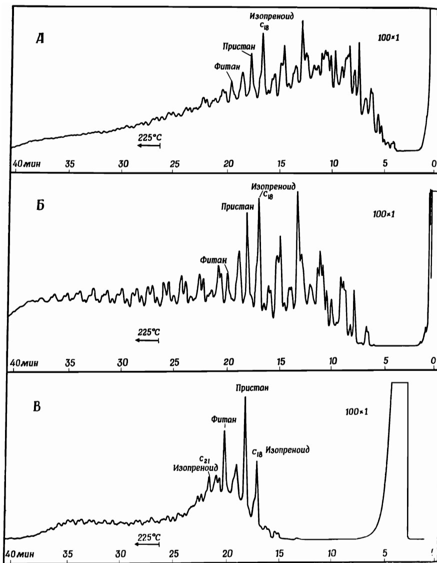
Фиг. 60. Сравнение газовых хроматограмм разветвленных и циклических углеводородов из формаций Антрим (А), Пансач (Б) и Соуден (В) [46]. В этих древних отложениях гораздо беднее, чем в сланце Грин-Ривер, представлены разветвленные и циклические алканы с большой молекулярной массой. Считается, что это результат постседиментационного разрушения этих соединений. Чувствительность 100 \times 1 .
