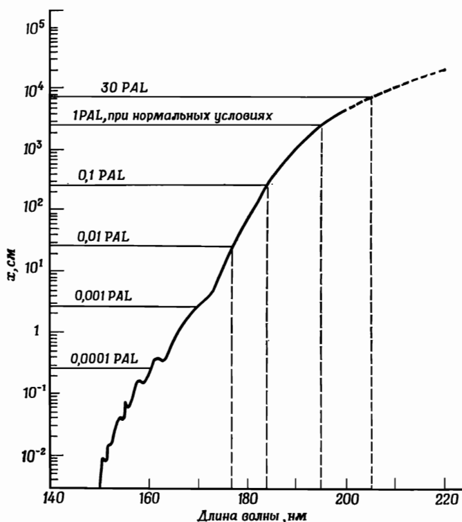
Фиг. 89. Толщина слоя \text{CO}_2 , необходимого для поглощения солнечного ультрафиолета до уровня 1 эрг/(см 2 ·с) при ширине полосы 5 нм (ср. фиг. 88) [1].
