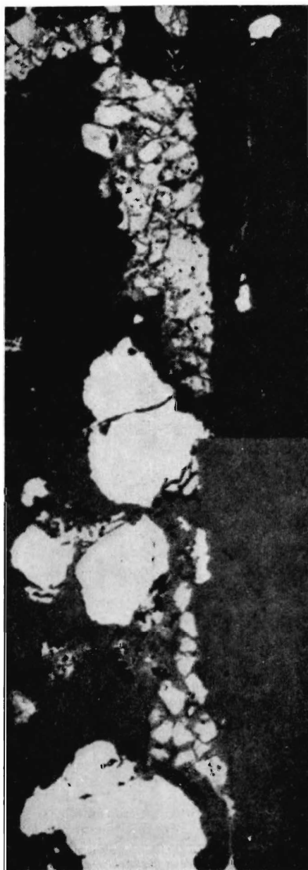
Фото 33. Микрофотография осадочного ритма (кварц — пирит)/(кварц — урановая смолка) в докембрийском песчаннике Блайд-Ривер, Канада ( \times 22,5 ) (гл. XII, [21]). Кварц — черный, границы отдельных зерен на фотографии не видны; пирит — белый; мелкие зерна урановой смолки — серые.
