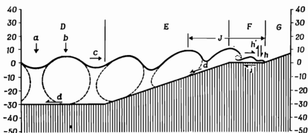
Фиг. 47. Схема циркуляции морской воды вблизи берега. Масштаб не соблюден. Расшифровка обозначений — в подписи к фиг. 45.
