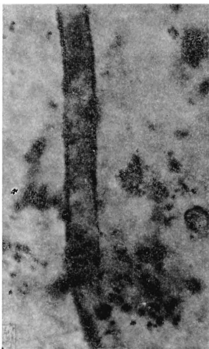
Фото 16. Образцы нитчатого ископаемого организма, названного Баргхоорном Animikiea septata ( \times 1000 ) (гл. XII, [6]). Формация Ганфлинт, Онтарио.
