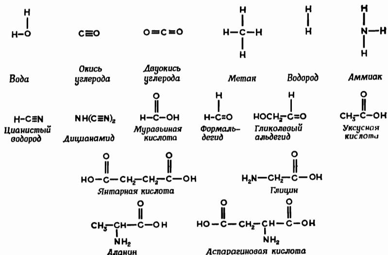
Фиг. 13. Строение малых молекул, которые неизбежно должны присутствовать в любой планетной примитивной атмосфере и гидросфере [6].
