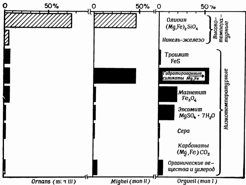
Фиг. 101. Минералогия углистых хондритов.
