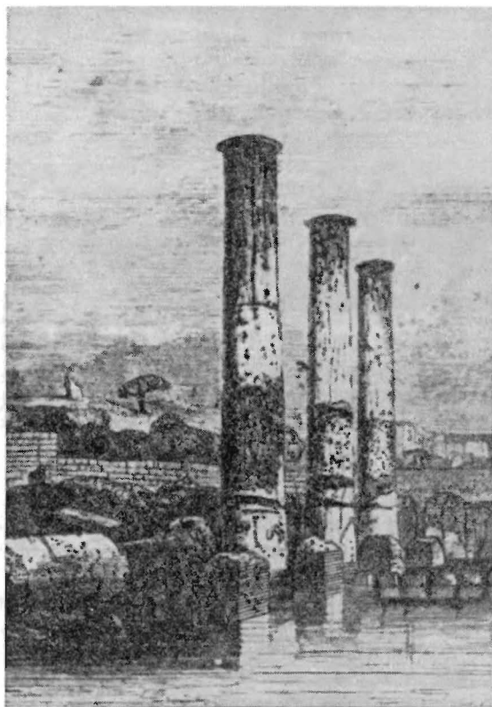
Фиг. 1. Колонны так называемого храма Сераписа в Поццуоли близ Неаполя. На них хорошо видны колебания уровня моря, благодаря чему этим колоннам отведено важное место в труде Чарльза Лийеля [8]. Трансгрессия моря ясно отмечена темными ходами сверлящих моллюсков, расположенными не выше 2—3 м над основанием колонн. Выше сильно истощенной зоны видны отдельные отверстия; они проделаны моллюсками во время более поздней, гораздо более сильной, но краткой трансгрессии. Сейчас уровень моря стоит намного ниже; вода у основания колонн — пресноводный пруд, устроенный городскими властями вокруг развалин.
