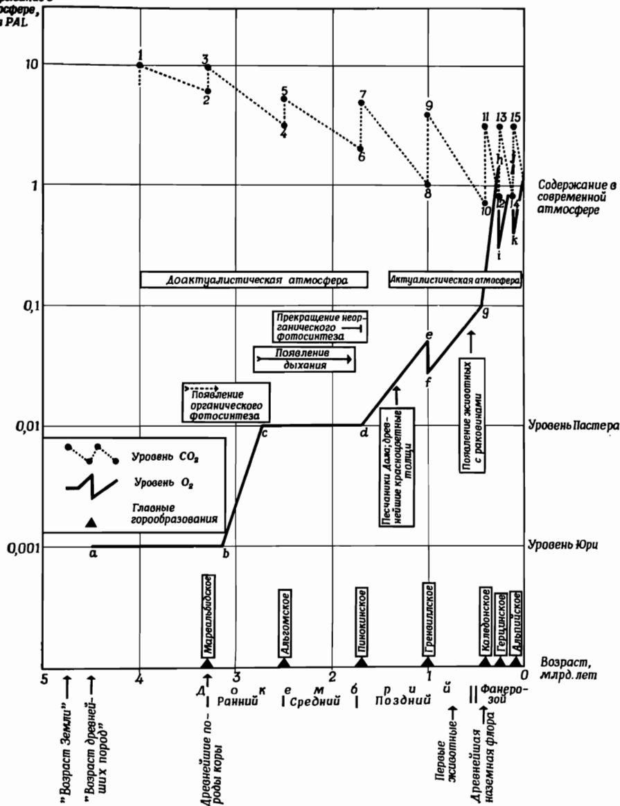
Фиг. 99. Предполагаемая история атмосферного кислорода и двуокси углерода (объяснение см. в тексте).
