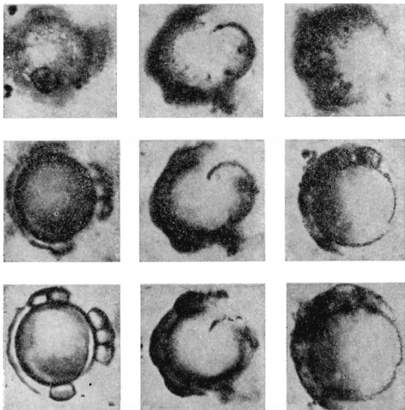
Фото 20. Три образца распространенного в формации Ганфлинт (Онтарио) сферического микроископаемого Eosphaera tyleri [6]. В каждом вертикальном ряду даны три снимка одной и той же особи, сделанные при разной фокусировке микроскопа. Снимки нижнего ряда сделаны при фокусировке на экваториальную плоскость сфер. Можно представить себе объемную морфологию организма. Это двойная сфера, между стенками которой лежат сферические бугорки, прикрепленные к внутренней стенке. Как и в случае рассмотренных выше сегментированных нитевидных ископаемых, столь сложная структура свидетельствует о том, что перед нами довольно высокоорганизованные существа.
