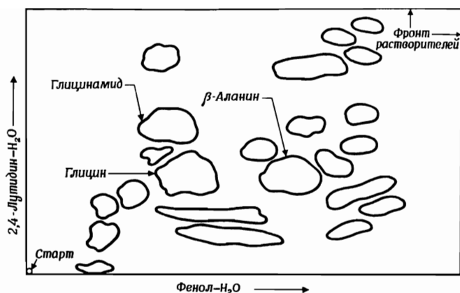
Фиг. 31. Хроматограмма на бумаге (см. разд. 9 этой главы) продуктов, образующихся в системе с формальдегидом и гидроксиламином [28].
