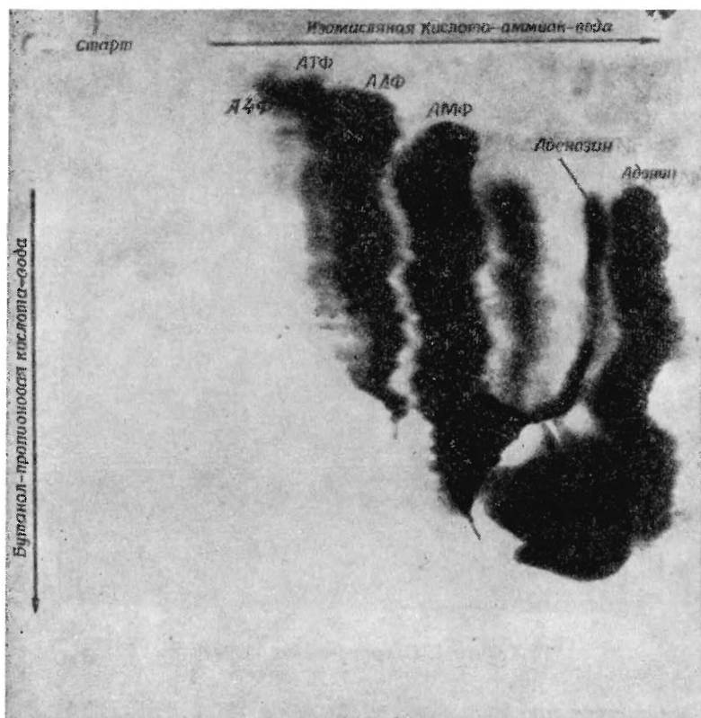
Фото 3. Хроматограмма на бумаге смеси соединений, полученных после облучения аденозинмонофосфата (АМФ) ультрафиолетом (гл. VI, [31]). Среди продуктов синтеза — аденозинтетрафосфат (А4Ф), аденозинтрифосфат (АТФ), аденозиндифосфат (АДФ). В более ранних экспериментах была доказана возможность неорганического синтеза АМФ из аденозина и аденина под действием ультрафиолета. Аденозин и аденин в свою очередь могут быть синтезированы в водных растворах с цианистым водородом под действием несколько повышенной температуры (гл. VI, [28, 29]) или ультрафиолета. Таким образом, в условиях примитивной атмосферы, очевидно, был вполне возможен неорганический синтез небольших органических молекул, на которых основана современная жизнь.
