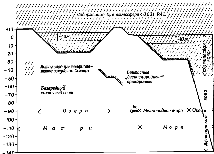
Фиг. 95. Схема распространения жизни в условиях примитивной атмосферы, в которой содержание O_2 составляло 0,001 современного или ниже.
