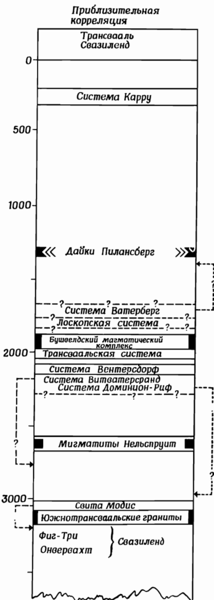
Фиг. 70. Стратиграфическая колонка докембрия Трансвааля.
