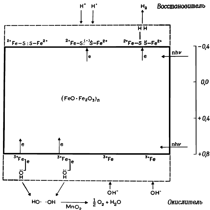
Фиг. 40. «Фотогальваническая модель» Граника [18].
