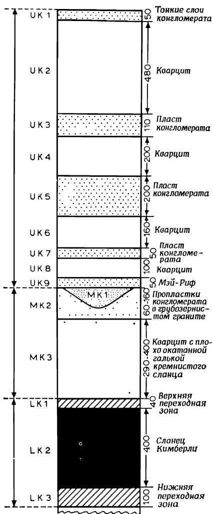
Фиг. 73. Стратиграфическая колонка серии пород Кимберли, входящей в систему Витватерсранд, Южная Африка [27].
