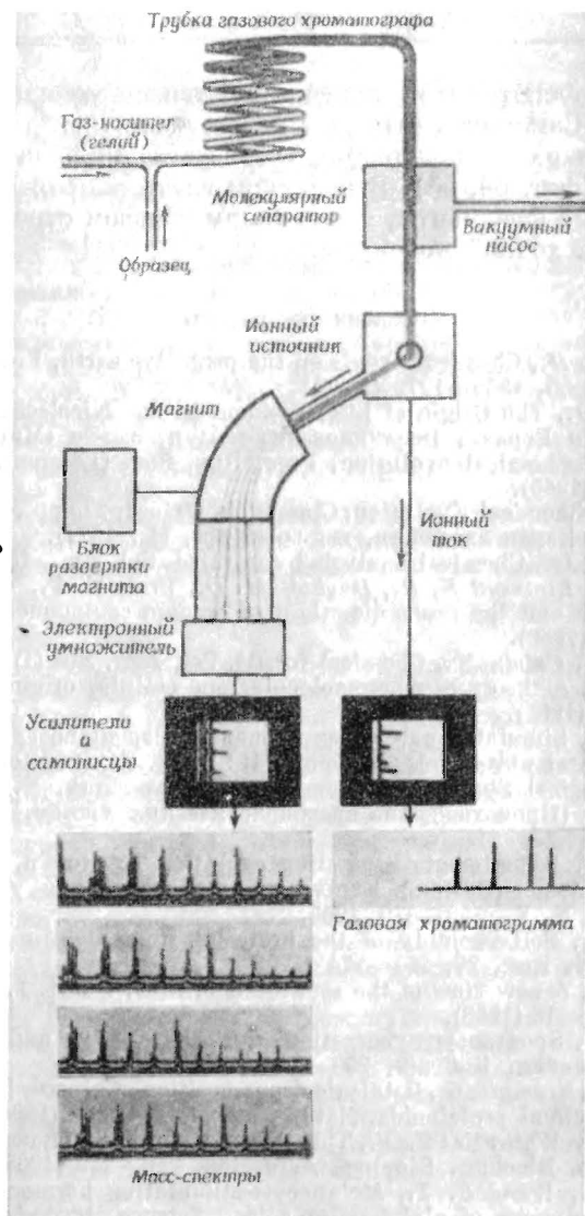
Фиг. 36. Схема комбинированной установки из газо-жидкостного хроматографа с масс-спектрометром [7].
