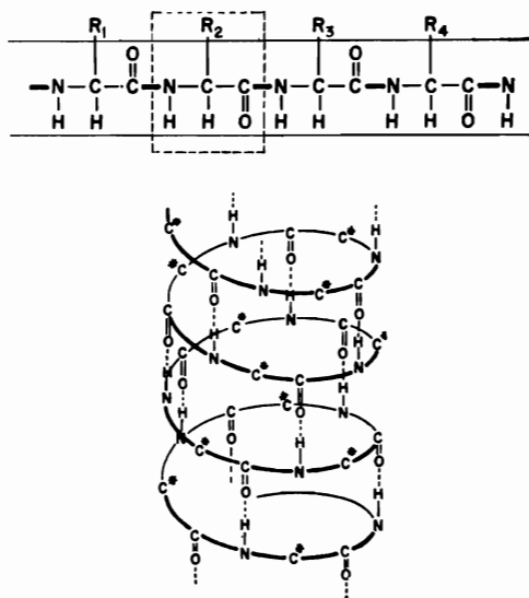
Фиг. 16. Схема строения белка.
