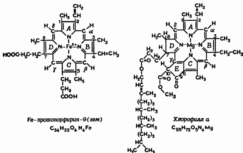
Фиг. 41. Структура гема и хлорофилла [18].
