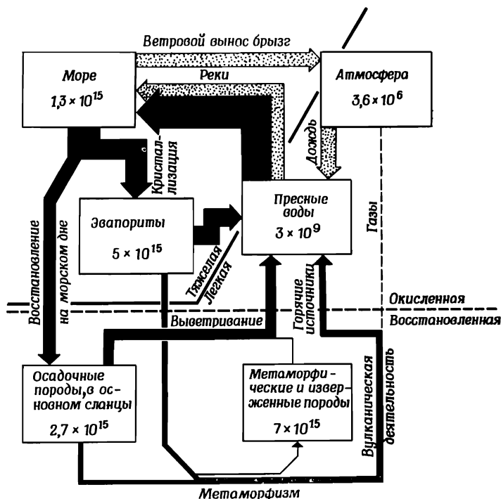
Фиг. 81. Геохимический цикл серы [20]. Массы указаны в метрических тоннах.
