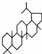
Фиг. 67. Скелет молекулы циклического изопреноида лупана C_{30} .
