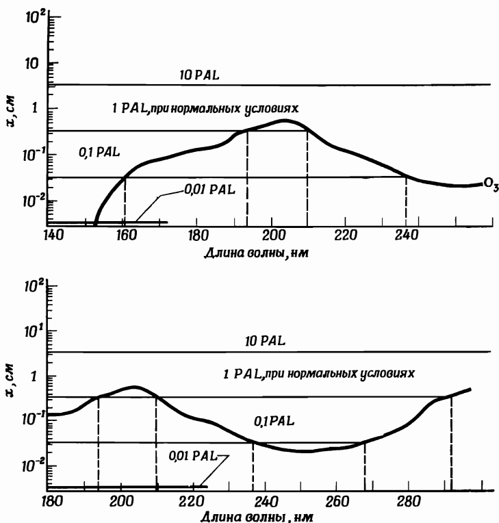
Фиг. 91. Толщина слоя O_3 , необходимого для поглощения солнечного ультрафиолета до уровня 1 \text{ эрг}/(\text{см}^2 \cdot \text{с}) при ширине полосы 5 нм [1].
