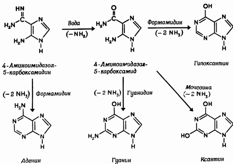
Фиг. 30. Предполагаемый механизм образования пуринов из водной смеси аммиака и цианистого водорода [29]. Промежуточные продукты — 4-аминоимидазол-5-карбоксамидин (АИКАМ) и 4-аминоимидазол-5-карбоксамид (АИКА) — были найдены в растворе.
