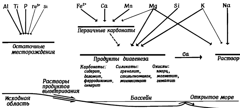
Фиг. 78. Схема латеритного выветривания на материковой низменности и образования железорудной формации в мелководном море в условиях бескислородной атмосферы.
