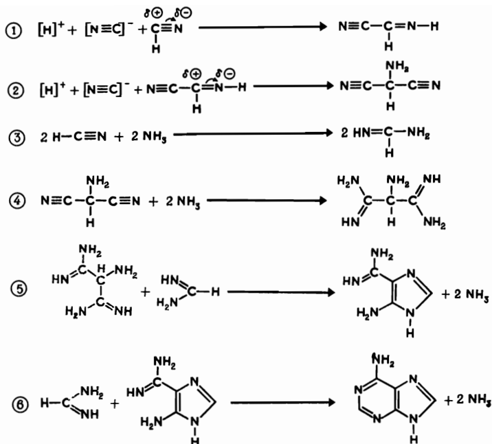
Фиг. 29. Предполагаемый механизм образования аденина из водной смеси аммиака и цианистого водорода (суммарная реакция: 5 \text{HCN} = \text{Аденин} ) [29]. Значки \delta+ и \delta- в уравнениях 1 и 2 означают частичные положительный и отрицательный заряды.
