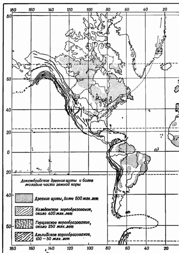
Фиг. 49. Схематическая текто
