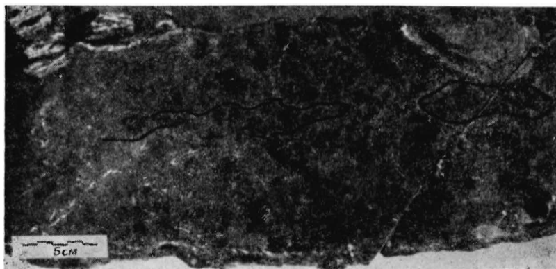
Фото 28. Шлиф докембрийского филлита, слабометаморфизованного глинистого осадка. Видны два экземпляра Corysium enigmaticum Sederholm, Миллинемы, Айтолакти, в 7 км к северо-востоку от Тампере, Финляндия.
