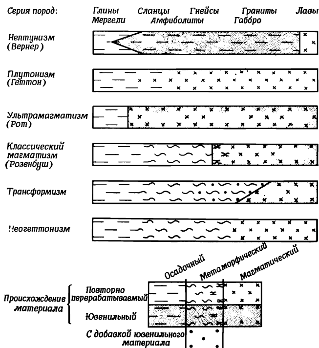
Фиг. 80. Обзор основных петрологических теорий [31].
