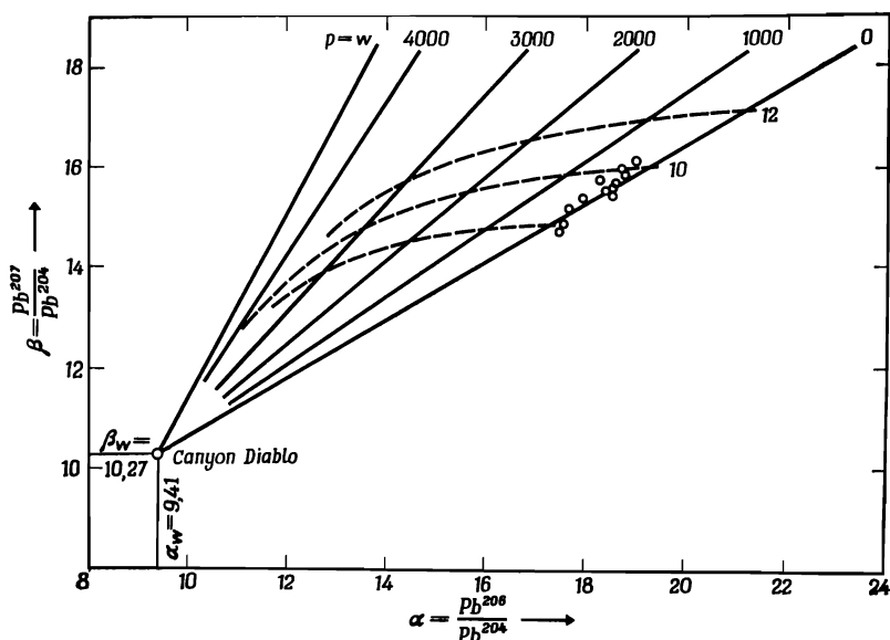
Фиг. 12. История изменения состава обычного свинца согласно модели Холмса — Хоутерманса [9].
