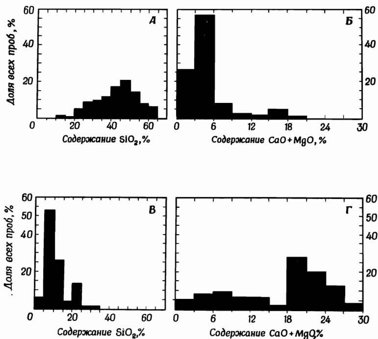
Фиг. 74. Распространенность SiO 2 и CaO + MgO в докембрийских (вверху) и более молодых (внизу) железорудных формациях.
