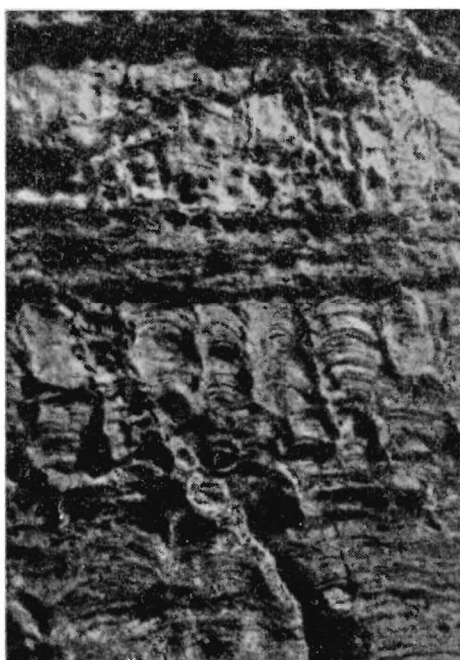
Фото 12. Выветрившаяся поверхность слоистого докембрийского доломита (возраст более 1780 млн. лет) вблизи Оллитерво, Тервола (Финляндия) (гл. XII, [40]). Порода образована строматолитами; биогенные отложения накапливались слой за слоем.
