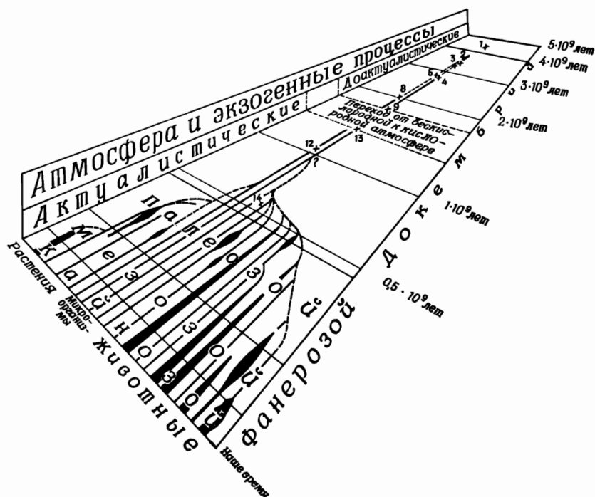
Фиг. 104. Схема истории жизни в целом.
