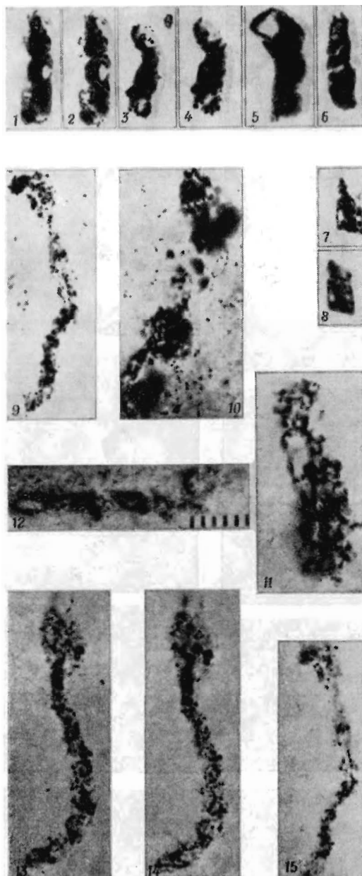
Фото 24. Нитчатые образования из формации Фиг-Три (ранний докембрий, Южная Африка). 1—11 — нитчатые образования разных типов ( \times \sim 375 ); 12 — колония глобулярных образований типа A_2 ( \times \sim 150 ); 13—15 — нитчатые образования разных типов ( \times \sim 375 ).
