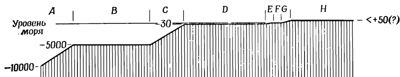
Фиг. 45. Схема ландшафтов, лежащих выше и ниже уровня моря.
