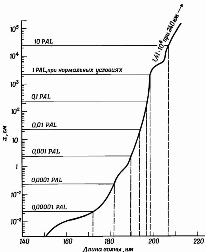
Фиг. 88. Толщина слоя воды, необходимого для поглощения солнечного ультрафиолета разной длины волны до уровня 1 \text{ эрг}/(\text{см}^2 \cdot \text{с}) при ширине полосы 5 \text{ нм} [1].
