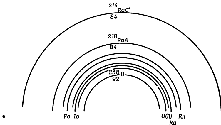
Фиг. 4. Схематическое изображение плеохроичных ореолов вокруг включения урана.
