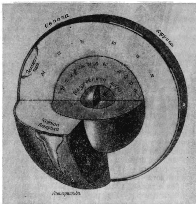
Фиг. 11. Схематический разрез Земли, показывающий материковую кору, мантию и ядро.
