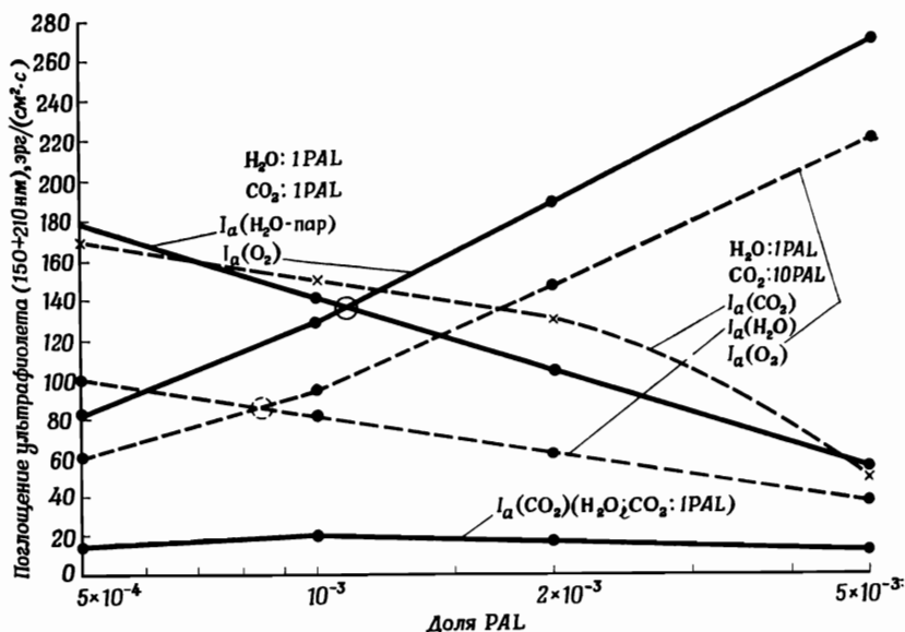
Фиг. 93. Автоматический механизм регуляции неорганического производства кислорода в первичной атмосфере [2].
