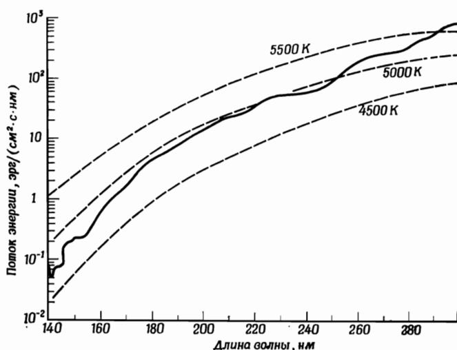
Фиг. 85. Интенсивность солнечного излучения (т. е. его энергия на верхней границе земной атмосферы) в области спектра от 140 до 300 нм [1].
