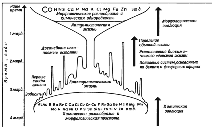
Фиг. 105. Схема возникновения и дальнейшей эволюции жизни [8].
