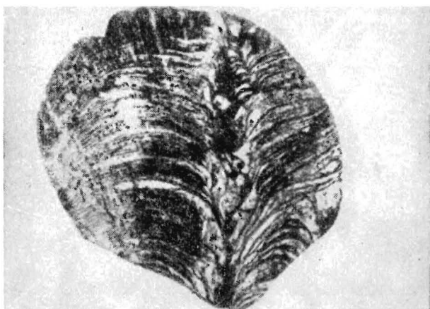
Фото 11. Тонкий шлиф биогенного докембрийского известняка (гл. XII, [51]). Серия Доломит, вблизи Булавайо, Южная Родезия. Несколько уменьшено. Обратите внимание на сложную структуру центральной «колонки», которая типична для биогенных отложений, но не встречается в неорганических известняковых отложениях.
