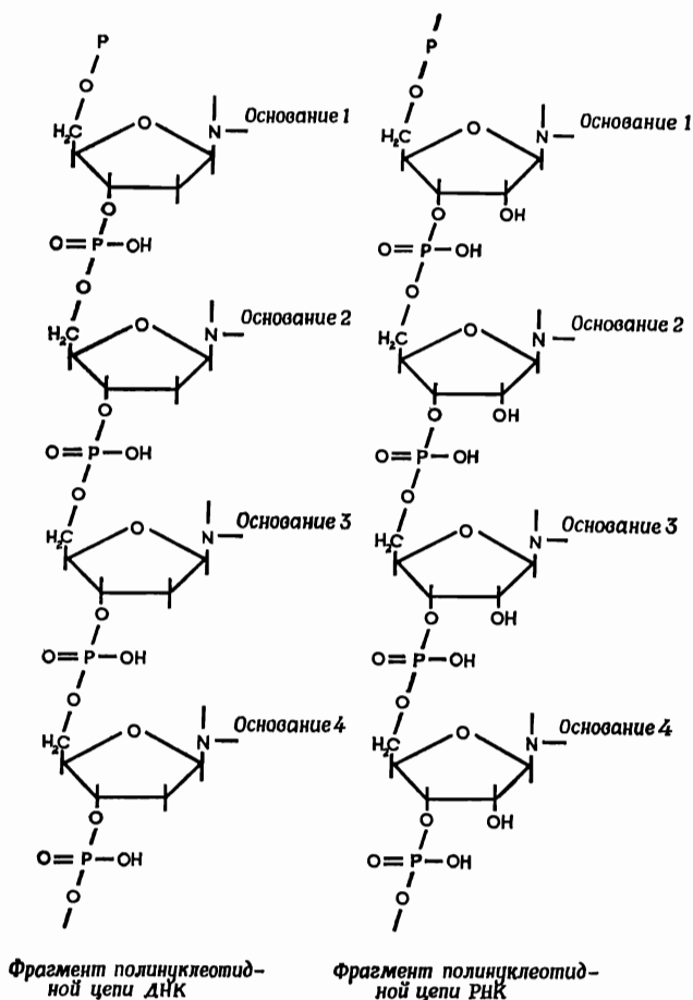
Фиг. 20. Строение полинуклеотидов ДНК и РНК.
