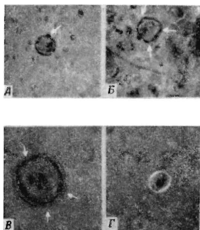
Фото 45. «Организованные элементы» метеорита Orgueil. Обозначения: А—В — «организованные элементы», выделенные из размолотой в порошок пробы; Г — «организованный элемент» на тонком шлифе. Снято при фазо- вом контрасте.
