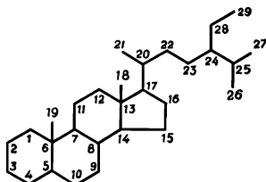
Фиг. 65. Углеродный скелет циклического изопреноида ситостана ( C_{29} ).
