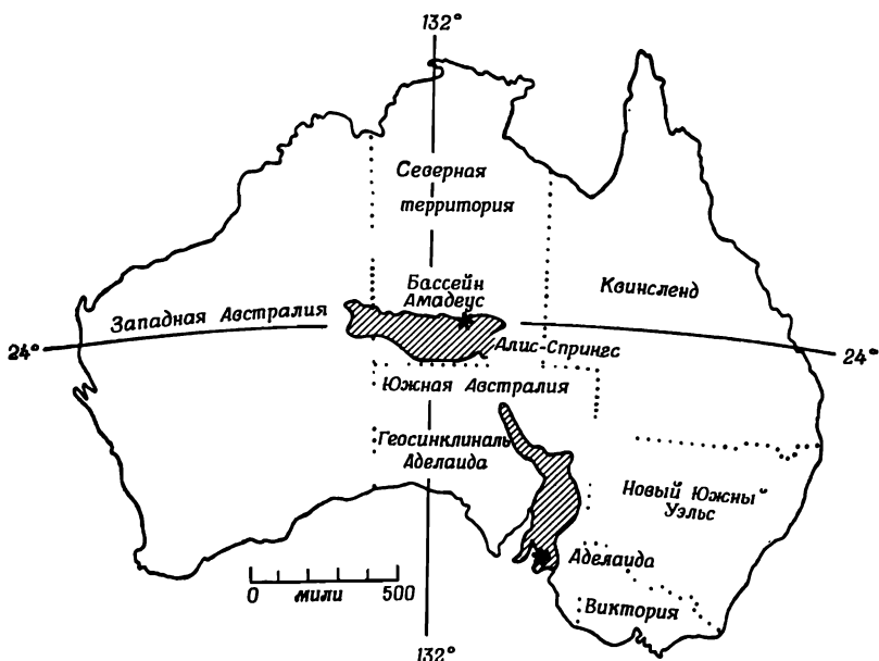
Фиг. 84. Карта Австралии [41].
