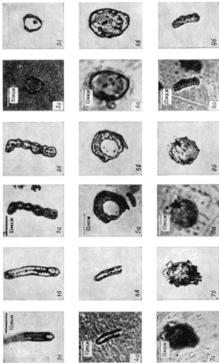
Фото 43. Микрофотографии (а) и рисунки (б) «организованных элементов» из метеорита Orgueil (гл. XV, [32, 33]). Рисунки сделаны человеком, не видевшим фотографий. С помощью сканирования электронным микроскопом показано, что образования 1, 2, 3, 4, 5 и 9 частично минерализованы железом и некоторым количеством хлора. В образовании 6 содержатся железо и никель, а образцы 7 и 8 состоят из силиката магния.
