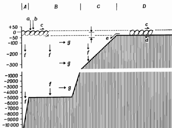
Фиг. 46. Схема циркуляции воды и возможных механизмов концентрирования и сохранения в море.
