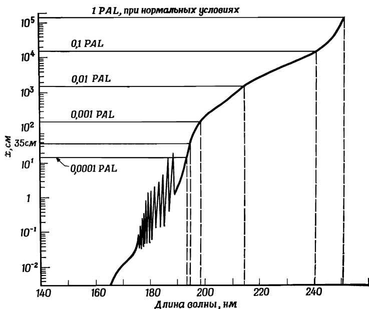
Фиг. 90. Толщина слоя O_2 , необходимого для поглощения солнечного ультрафиолета до уровня 1 \text{ эрг}/(\text{см}^2 \cdot \text{с}) при ширине полосы 5 нм [1].
