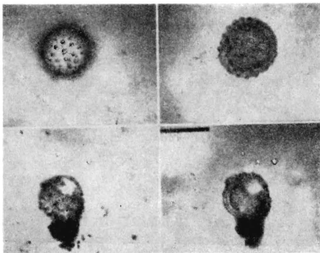
Фото 47. Сравнение «организованного элемента» из метеорита Orgueil (вверху) с пылью Ambrosia ( \times 720 ) (гл. XVII, [13]. В каждой паре фотографии, сделанные с одного объекта, различаются фокусировкой микроскопа. Кажущееся сходство между этими двумя образованиями обусловлено нечеткостью изображения при таком увеличении, но этот недостаток присущ даже лучшим микрофотографиям. Непосредственное изучение под микроскопом показывает, что объекты явно различаются.
