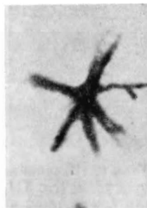
Фото 18. Типичное беспорядочное скопление нитей, главным образом Gunflintia minuta и спороподобных телец Huroniospora (гл. XII, [6]). Снимки ясно говорят об обилии микроископаемых в формации Ганфлинт, Онтарио.
