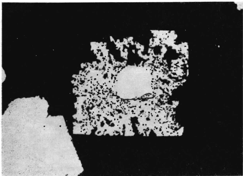
Фото 36. Микрофотография округлого зерна пирита, окруженного более молодыми наростами, обычно повторяющими форму кристаллов пирита (гл. XIII, [15]); Витватерсранд, Южная Африка ( \times 100 ).
