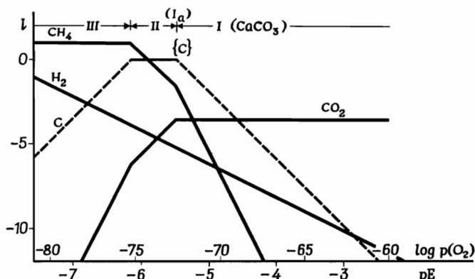
Фиг. 83. Зависимость логарифмов активности ( l ) для \text{C}_{\text{тверд.}} , \text{CH}_{4\text{газ}} , \text{CO}_{2\text{газ}} , и \text{H}_{2\text{газ}} от \log p(\text{O}_2) и pE в силленовской модели морской воды [47]. Можно выделить следующие области: I — присутствует \text{CaCO}_{3\text{тверд.}} ; Ia — переходная между I и II, присутствуют и \text{CaCO}_{3\text{тверд.}} и \text{C}_{\text{тверд.}} ; II — присутствует \text{C}_{\text{тверд.}} ; III — нет ни \text{CaCO}_3 , ни C. Показана только восстановительная часть области I. В современных условиях \log p(\text{O}_2) равен 7 \cdot 10^{-1} , а pE = \pm 12,5 . \text{CH}_4 имеет нулевую химическую активность (т. е. может существовать) только при падении парциального давления кислорода ниже \log p(\text{O}_2) = -75 .
