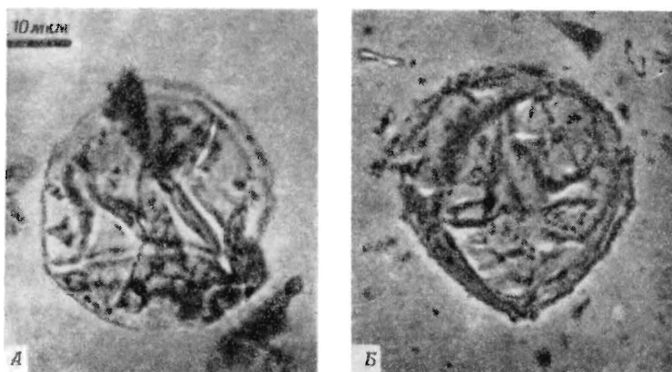
Фото 48. «Организованный элемент» из метеорита Orgueil (А) и ископаемый земной организм, динофлагеллята (Б). Между ними есть некоторое сходство, только следует учесть, что «организованный элемент» увеличен в четыре раза сильнее, чем динофлагеллята. К тому же ультрамикроспектр «организованного элемента» не похож на спектры современного биологического материала. Значит, сходство здесь лишь чисто внешнее. «Организованный элемент» входит в состав метеорита, а не занесен в метеорит на Земле.
