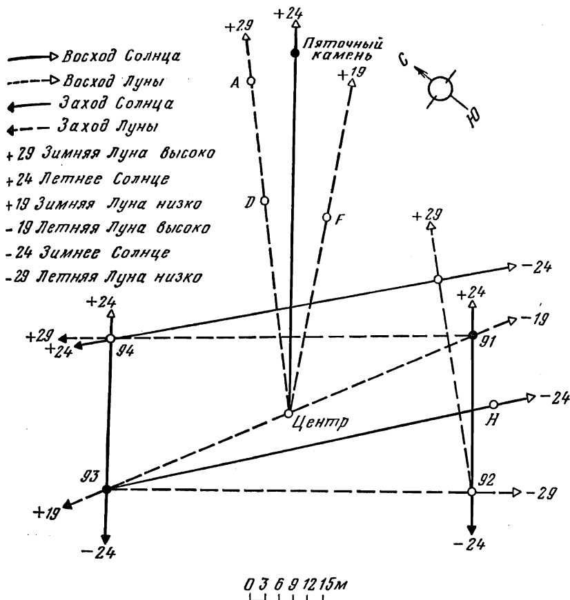
Рис. 11. Первоначальные направления, определенные по Стоунхенджу I. Точные значения азимутов приведены в табл. 1.
