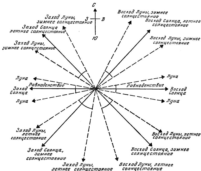
Рис. 3. Азимуты направлений восхода и захода Солнца и Луны в дни солнцестояний и равноденствий для широты Каллениша.
