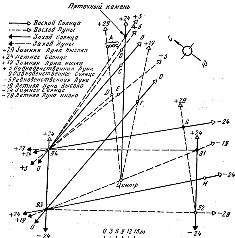
Рис. 14. Все направления, найденные в Стоунхендже I, включая равноденственные линии для Солнца и Луны.
