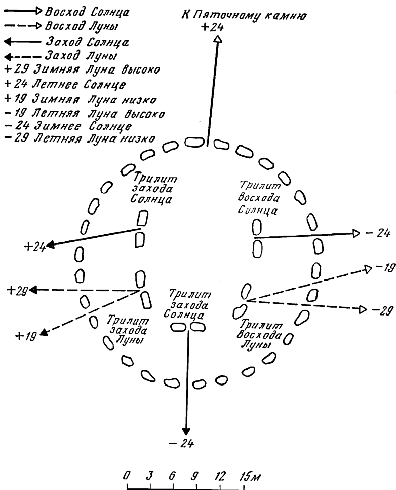
Рис. 12. Направления, определяемые арками Стоунхенджа III. Точные значения азимутов приведены в табл. 1
