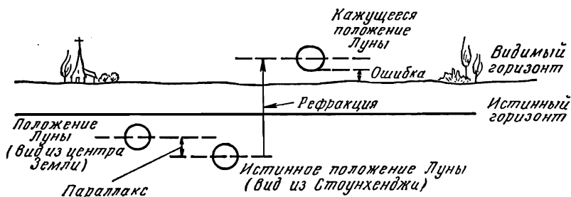
Рис. 13. Условия при восходе или заходе. Сначала астрономические вычисления проводятся для наблюдателя в центре Земли. Чтобы рассчитать условия для наблюдателя на поверхности Земли, надо ввести поправку на параллакс. Затем надо учесть атмосферную рефракцию, из-за которой светило кажется выше над горизонтом, чем на самом деле. Наконец, надо принять во внимание высоту видимого горизонта, который, как правило, бывает выше астрономического горизонта, определяемого горизонтальной плоскостью, находящейся на уровне глаз наблюдателя.
