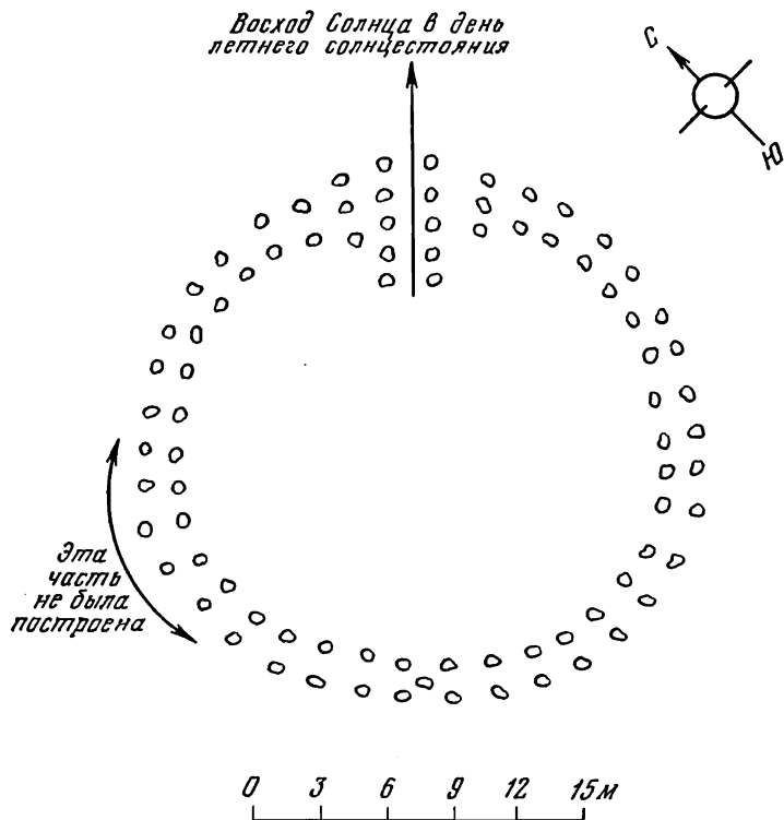
Рис. 4. План Стоунхенджа II.
