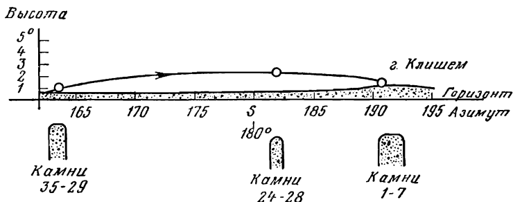
Рис. 4. Вычисленный видимый путь полной Луны в период летнего солнцестояния в Калленише примерно в 1500 г. до н. э.
