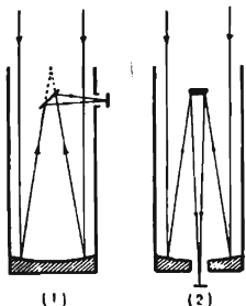
Նկ. 20. Նյութոնի (1) և Կասեգրենի (2) հայելավոր աստղադիտակների օպտիկական սխեմաները:
