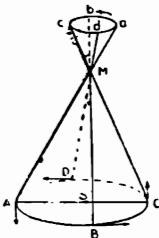
Նկ. 58. Աստղերի պարալաքսային տեղաշարժը:
