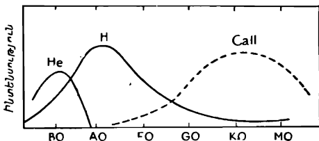
Նկ. 97. Ջրածնի (H), հելիումի (He) և իոնացված կալցիումի (Ca II) կլանման գծերի ինտենսությունները տարբեր ապեկտրալ դասերի աստղերի ապեկտրոններում:
