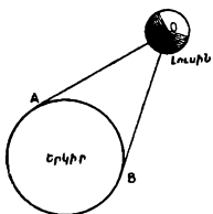
Նկ. 64. Լուսնի պարալաքսային ճոճումը:
