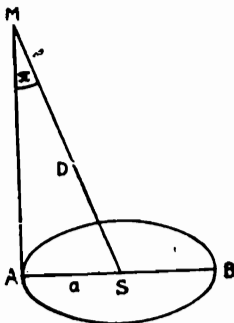
Նկ. 55. Աստղերի տարեկան պարալաքսը:
