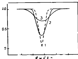
Նկ. 94. Արեգակի խավարման կոորբոր օպտիկական (1), \lambda=1,5 մ (2) և \lambda=4,2 մ (3) ալիքներում։ Մինչև խավարումը ճառագայթման հզորությունն ընդունված է հավասար 1,0-ի։ Պարզ երևում է Արեգակի չափերի աճը երկար ալիքներին անցնելիս։
