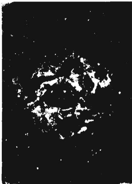
Նկ 159. Միկղշուր I աստղասփյուռը, որը տեսնվորված է Վար- դակ (Մոզես) դիֆուզ միազումածության Մէջ: Աստղասփյուռի կո- րիչը N(C) 2244 աստղակույտն է:
