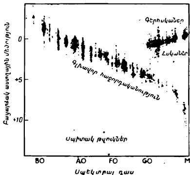
Նկ. 98. Հերցշպրունգ-Ռենսելի (սպեկտր-լուսատվություն) դիագրամը՝ համեմատաբար պայծառ աստղերի համար։ Երևում են գլխավոր հաջորդականությունը, կարմիր հսկաները և գերհսկաները, ինչպես նաև 3 սպիտակ թզուկ։ Սպիտակ թզուկների սակավությունը պայմանավորված է նրանց ցածր լուսատվությամբ, որի պատճառով դիտվում են ամենամոտ թզուկները։ Իրականում նրանց թիվը շատ ավելի մեծ է քան հսկա և գերհսկա աստղերինը։
