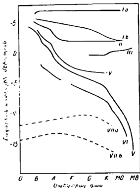
Նկ. 99. Սպեկտր-լուսատվություն դիագրամի սխեմատիկ տեսքը, ըստ MK երկշափ սպեկտրալ դասակարգման. Ia, Ib—պայծառ և թույլ գերհսկաներ, II, III—պայծառ և թույլ հսկաներ, IV—ենթահսկաներ, V—գլխավոր հաջորդականություն, VI—ենթաթղուկներ, VIIa, VIIb—պայծառ և թույլ սպիտակ թղուկներ:
