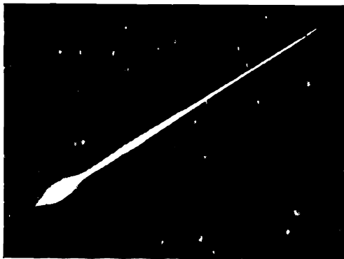
Նկ. 82. Բոլիդի անկումը:
