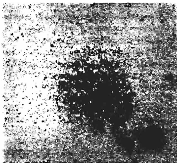
Նկ. 121. M 92 գնդաձև աստղակույտը Կենտավրոսի համաստեղությունում:
