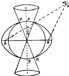
Նկ. 57. Պրեցեսիոն շարժումը։
