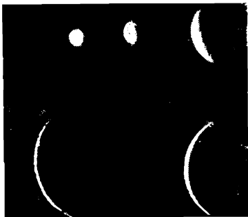
Նկ. 71. Վեներայի փուլերը:
