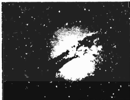
Նկ. 150. Կենտավրոս Ա (NGC 5128) ուղիղ գալակտիկան, ուի կենտրոնում գտնվող փոշե զանգվածն այն բաժանում է երկու կեսի :
