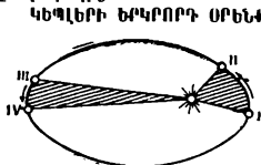
Նկ. 40. Կեպլերի երկրորդ օրենքի բացատրությունը:
