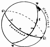
Նկ. 3. Հասարակածային կոորդինատներ:
