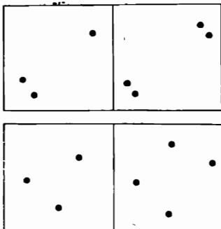
Նկ. 135. Սովորական տիպի (վերևում) և Օրինի Տրապեցիայի տիպի (ներքևում) եռակի և քառակի համակարգեր:
