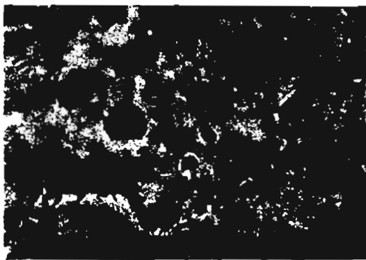
Նկ. 76. Մարսի մակերևույթը:
