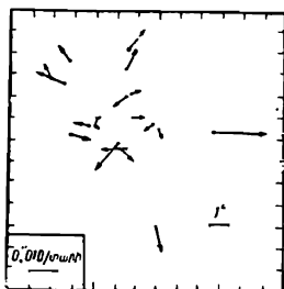
Նկ. 136. Հ Պերսեուսի աստղի շուրջը գտնվող Պերսեու II աստղասփյուռի լայնացման սխեման: Սլաքները ներկայացնում են աստղերի սեփական շարժումները աստղաափյուռի կենտրոնի նկատմամբ: Նրանց երկարությունը համեմատական է սեփական շարժման մեծությանը:
