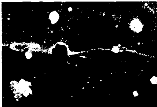
Նկ. 127. Փչիու գլուխ մութ միգամածությունը, որը կաղմված է հիմնականում փոշահատիկներից. ոտներ ցրում են իրենց վրա ընկած լույսը: Այդ է պատճառը, որ միգամածության ուղղությամբ աստղեր գրեթե չեն երևում:
