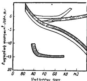
Նկ. 130. I և II տիպերի աստղային բնակչությունների սպեկտր-լուսատվություն համեմատական դիագրամը: Սպիտակ շերտերը ներկայացնում են II տիպի աստղային բնակչությունը, իսկ կարտված շերտերը՝ I տիպի աստղային բնակչությունը:
