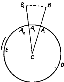
Նկ. 56. Վախր ընկնող մարմինների շեղվելը դեպի արևելք (Երկրի հասարակածում):
