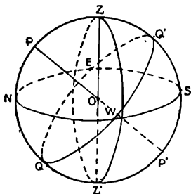
Նկ. 1. Երկնոլորտի հիմնական կետերն ու շրջանները:
