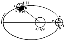
Նկ. 62. Լուսնի ճոճումն ըստ երկայնության:
