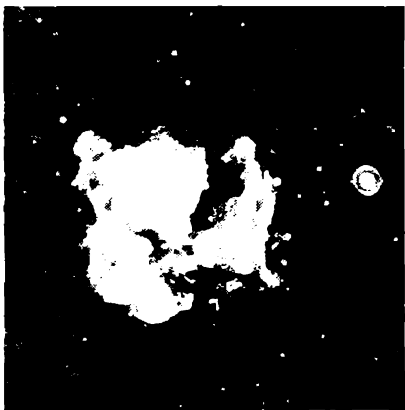
Նկ. 124. Տրիֆիդ (M 20) դիֆուզ միզամածությունը Աղեղնավորի համաստեղությունում:
