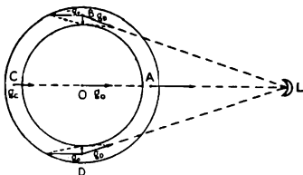
Նկ. 47. Մակընթացությունների և տեղափոխությունների առաջացումը:
