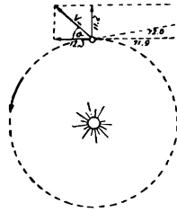
Նկ. 84. Երրորդ տիեզերական արագության որոշումը:
