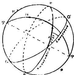
Նկ. 12. Խավարածրային կոորդինատներ
