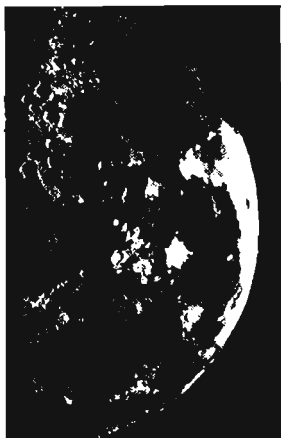
Նկ. 73. Լուսիս ատաշին բառուղում
