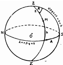
Նկ. 2. Հորիզոնական կոորդինատներ:
