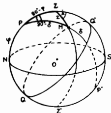
Նկ. 14. Պարալակտիկ եռանկյուն:
