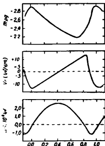
Նկ. 106. Ճ Ցեֆեոսի պայծառության ( M_{pg} ), տեսողական արագության ( V_r ) և շառավղի ( R ) փոփոխությունների կորերը՝ կախված պարբերության փուլից:
