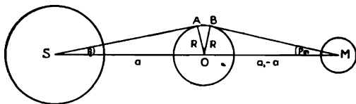
Նկ. 53. Արեգակի պարալաքսի որոշելը:
