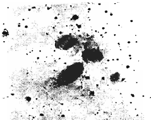
Նկ. 156. Գալակտիկաների ֆիզիկական խումբ (Ստեֆանի կվիետերը)։
