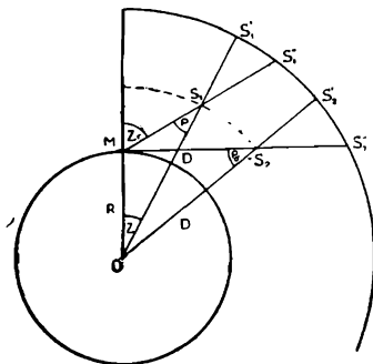
Նկ. 51. Կապ պարալաքսի և հորիզոնական պարալաքսի միջև
