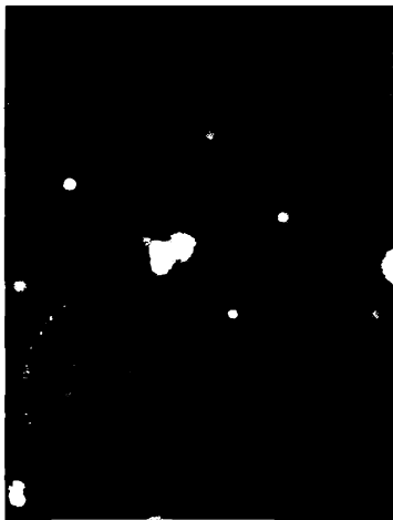
Նկ. 149 Կարապ A ռադիոգալակտիկայի կրկնակի կորիզը:
