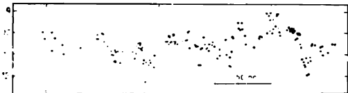
Նկ. 114. T Ցուլի տիպի փոփոխական աստղ, RW Կառավարի պայծառության կորի մի կտոր:
