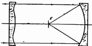
Նկ. 22. Շմիդտի համակարգի աստղադիտակի օպտիկական սխեման։
