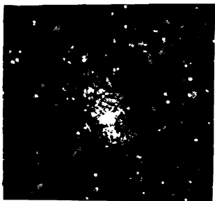
Նկ. 140. NGC 148 էլիպսաձև գալակտիկան:
