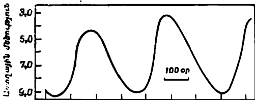
Նկ. 108. Ծրկարպարբերական փոփոխական Կետի Զարմանալի աստղի (օ Կետի) պայծառության փոփոխության կորը՝ 1946—48 թվականներին:
