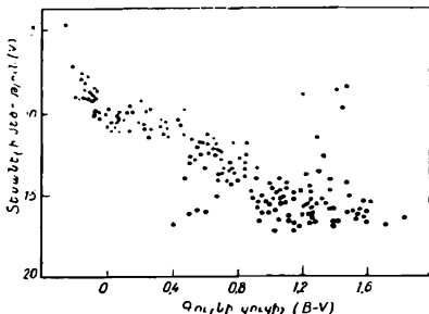
Նկ. 100. NGC 2264 բաց աստղակույտի տեսանելի աստղային մեծություն-գույնի ցուցիչ դիագրամը, որ լիովին փոխարինում է նրա Հերցշպրունգ-Ռեյսի դիագրամին, աստղակույտի բոլոր աստղերը գործնականորեն նույն հեռավորության վրա գտնվելու շնորհիվ:
