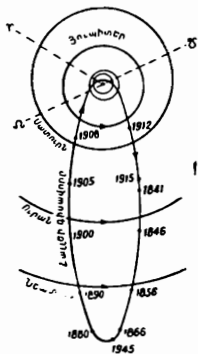
Նկ. 81. Հալլեյի գիսավորի ուղեծիրը (ներառիվ ուղեծրի վրա՝ տարբեր թվականներին):
