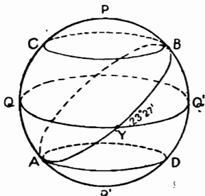
Նկ. 9. Արեգակի տեսանելի շարժումը:
