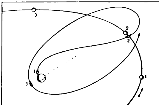
Նկ. 86. Սովետական երրորդ տիեզերական հրթիռի շարժման պեման: Սխեմայի վրայի թվերը նշանակում են լուսնի և հրթիռի դիրքերը. 1—հրթիռի արձակման պահին, 2—նրանց ամենամոտ մոտենցման պահին, 3—հրթիռը Երկրի մոտով անցնելու պահին:
