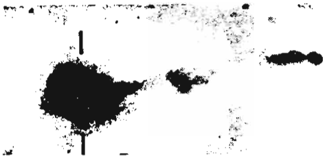
Նկ. 152. NGC 1182 գալակտիկան, միջուկից արտավիժված նյութի խտացումների հետ:
