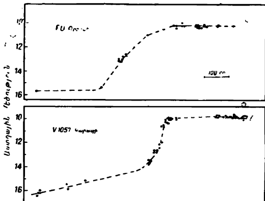
Նկ. 116. FU Օրիոնի և V 1057 Կարապի պայծառության կորերը: Հորիզոնական առանցքի վրա տրված ժամանակը, իսկ ուղղահայաց առանցքի վրա՝ աստղային մեծությունը:
