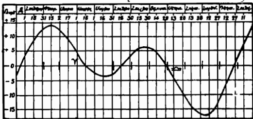
Նկ. 17. Ժամանակի հավասարման գրաֆիկը:
