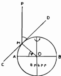
Նկ. 4. Տեղի աշխարհագրական լայնության և բևեռի բարձրության կապը:
