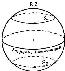
Նկ. 5. Լուսատուների օրական շարժումը քննենք:
