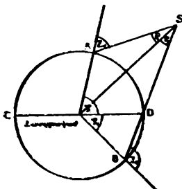
Նկ. 52. Հորիզոնական պարալաթսի բրոշեյու
