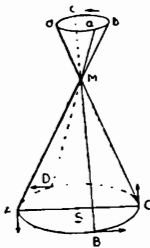
Նկ. 59. Աստղերի աբերացիայի տեղաշարժը:
