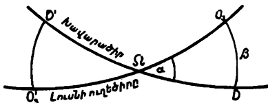
Նկ. 68. Արեգակը խավարելու գոտին:
