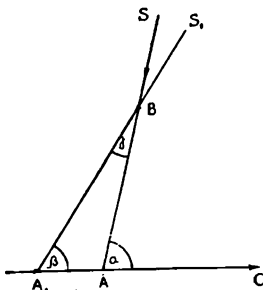
Նկ. 60. Արեռացիայի բացատրման սխեման:
