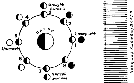
Նկ. 61. Լուսնի փուլերի առաջացումը:
