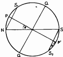
Նկ. 8. Մայր շմտնող, շժագող, ծագող ու մայր մտնող լուսատուները:
