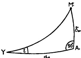
Նկ. 15. Գարնանային գիշերահավասարի կետի դիրքի որոշելը:
