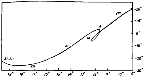
Նկ. 36. Մերկուրու տեսանելի ուղին 1976 թ. օգոստոս-դեկտեմբեր ամիսներին:
