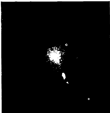
Նկ. 148. Կուլս A (NGC 4486) ռադիոգալակտիկան, որի կորիզից դուրս է շարտվել գալակտիկաների գանգվածների կարգի խտացումներ պարունակող նյութի մի շիթ:
