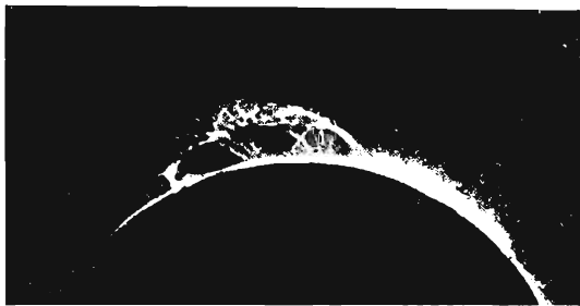
Նկ. 93. Հսկայական հրվիժակ:
