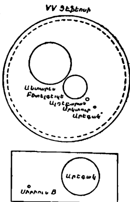
Նկ. 103. Արեգակի և մի քանի աստղերի համեմատական չափերը, գծիկներով նշված շրջանագծերը հավասար է Սատուրնի ուղեծրին՝ Արեգակի շուրջը:
