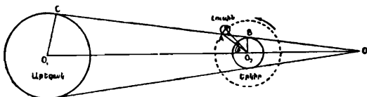
Նկ. 67. Լուսնի դիրքը Արեգակի խավարումը սկզբնու պահին:
