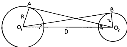
Նկ. 54. Լուսատուների շառավղի որոշելը:
