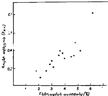
Նկ. 123. Աստղերի բեկոացման աստիճանի կախումը նրանց զույնի ավելցուկից ( E_B - V ):
