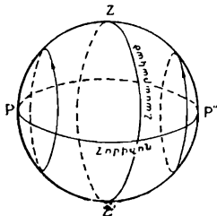
Նկ. 6. Լուսատուների օրական շարժումը հասարակածում:
