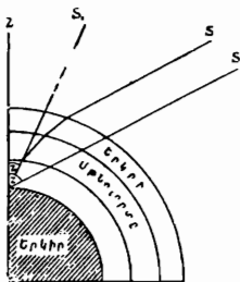
Նկ. 16 ա. Ստեղագիտական ռեֆրակցիա:
