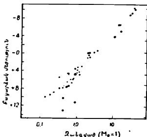
Նկ. 104. Զանգված-լուսատվություն էմպիրիկ առնչությունը: Զանգված-նրն արտահայտված են Արեգակի զանգվածի միավորներով:
