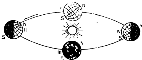
Նկ. 10. Տարվա եղանակների առաջացումը:
