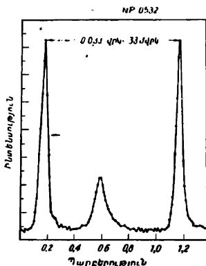
Նկ. 105. Խեցգետնածև միգամածության մեջ գտնվող NP 0532 բարախիչի (պուլսարի) պայծառության փոփոխության կարը սղեկարի օդափական տիրւթում՝ մի փուլի ընթացքում:
