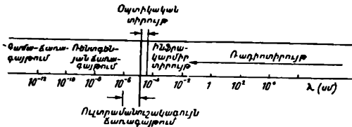
Նկ. 18. Էլեկտրամագնիսական ճառագայթման ալիքի երկարությունների սանդղակը:
