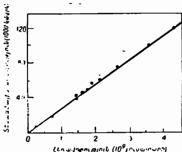
Նկ. 146. Գալակտիկաների տեսագծային արագությունների կախումը նրանց հեռավորությունից (Հաբլի օրենք): Կախումը ստացված է ավելի քան 1000 գալակտիկաների սպեկտրների չափումներից:
