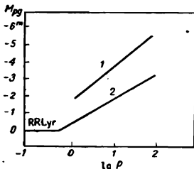
Նկ. 107. Ճ Ցեֆեոսի և RR Փնարի տիպի փոփոխականների պարբերություն-լուսատվություն առնչությունը: Հորիզոնական առանցքի վրա արված է պարբերությունը ( P ), իսկ ուղղահայաց առանցքի վրա՝ բացարձակ լուսանկարչական աստղային մեծությունը ( M_{pg} ):
