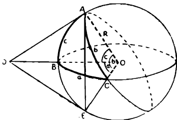
Նկ. 13. Սֆերիկ եռանկյուն:
