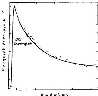
Նկ. 109. Հերկուլեսի համաստեղության մեր 1934 թ. դիտված նորի (DQ Հերկուլեսի) պայծառության կորը:
