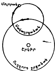
Նկ. 37. Մակաշրջանակ և ուղղորդ շրջանակ:
