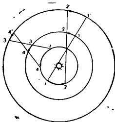
Նկ. 38. Արտաքին մոլորակների տեսանելի շարժումների բացատրությունը:
