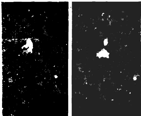
Նկ. 126. Հարյի գիսավորաձև միգամածությունը (NGC 2261) Միեղջյուրի համաստեղության մեջ: Միգամածության զազաթում գտնվում է R Միեղջյու- րի փոփոխական աստղը: Միգամածության տարբեր ժամանակներում ստաց- ված լուսանկարները վկայում են, որ ինքը՝ միգամածությունը, և ույնպես փոփոխական է:
