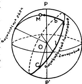
Նկ. 119. Գալակտիկական կոորդինատների համակարգը: P և P'-ը աշխարհի հյուսիսային և հարավային բևեռներն են, C-ն Գալակտիկայի կենտրոնը, l-ը գալակտիկական երկայնությունը, իսկ b-ն գալակտիկական լայնությունը (հաստ սղլաքները):
