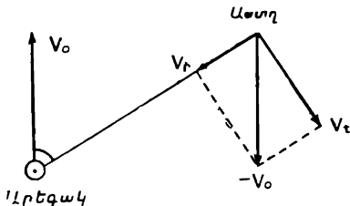
Նկ. 132. Արեգակի տարածական շարժման ազդեցությունը աստղի դիտվող շարժման վրա:
