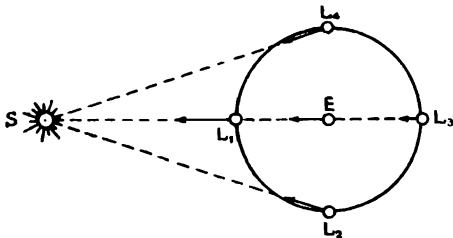
Նկ. 46. Լուսնի շարժման խանգարող ուժեր
