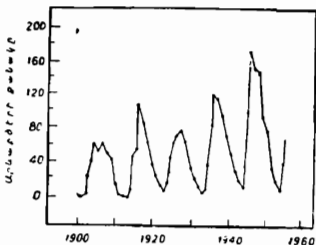
Նկ. 92. Արեգակի ակտիվության պարբերականությունը, որն արտահայտվում է արևաբծերի քանակի փոփոխությամբ:
