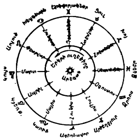
Նկ. 11. Արեգակի տեսանելի շարժումը Կենդանաշրջանով:
