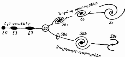
Նկ. 139. Գալակտիկաների դասերի հաջորդականությունն ըստ Հաբլի:
