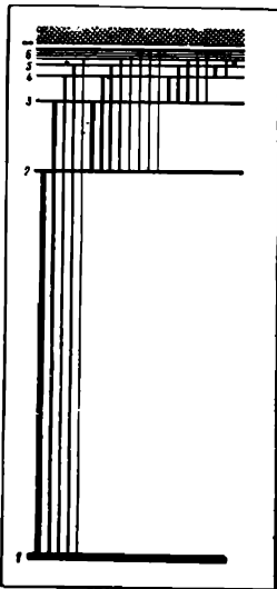
Նկ. 32. Ջրածնի ատոմի էներգետիկ մակարդակները: Ձախից ներշնչված են մակարդակների համարները՝ հիմնական մակարդակից (1) մինչև իոնացման մակարդակը ( \infty ):
