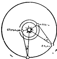
Նկ. 39. Ներքին մոլորակների տեսանելի շարժումների բացատրությունը:
