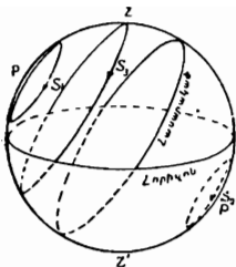
Նկ. 7. Լուսատուների օրական շարժումը միջին աշխարհագրական լայնություններում:
