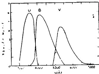
Նկ. 95. U, B և V աստղային մեծությունների ղգայնության կորերը:
