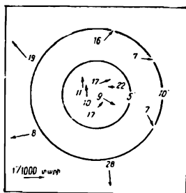
Նկ. 137. Օրիոնի աստղասփյուռի կենտրոնական մասի լայնացման սխեման: Տրված են աստղերի միջին դիրքերը և միջին շարժումները վեց հավասար սեկտորների համար՝ Տրապեցիայի շուրջը 5 անկյունային րոպե շառավղով շրջանի ներսում և վեց սեկտորների համար՝ այդ շրջանից դուրս: Բերված թվանշանները ցույց են տալիս, թե քանի աստղի վերաբերյալ տրվել են չափումներ և օգտագործված:
