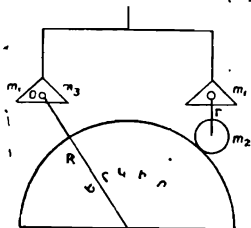
Նկ. 42. Երկրի զանգվածի որոշելը:
