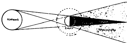
Նկ. 66. Լուսնի խավարման սխեման:
