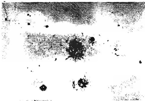
Նկ. 151. 3C273 քվազարը. ծրեում է կորիզից արտավիժված էլուքի շիթը:
