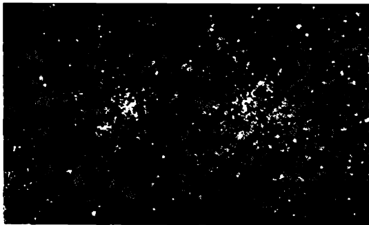
Նկ. 122. Պերսեուս 1 աստղասփյուռը, որի կորիզներն են ի և չ Պերսեուսի կրկնակի աստղակույտը:
