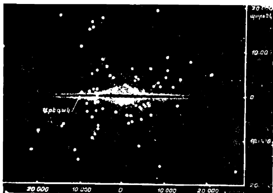
Նկ 122 Գալակտիկայի սխեմատիկ պատկերը։
