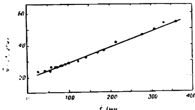
Նկ. 138. Երիտասարդ Օ—B դասերի աստղերի միջին տարածական արագության կախումը՝ աստղասփյուռների կորիզներից, նրանց ունեցած հեռավորությունից, որը աստղասփյուռների լայնացման հետևանք է:
