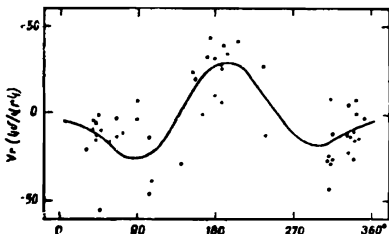
Նկ. 134. O—B դասերի աստղերի տեսագծային արագությունների կախումը նրանց գալակտիկական երկայնությունից (1): Այն բավարար կերպով ներկայացվում է Օորտի տեսական բանաձևով (հոծ գիծ):
