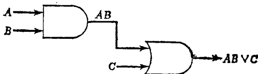
Рис. 6.12. Упрощенная схема.
