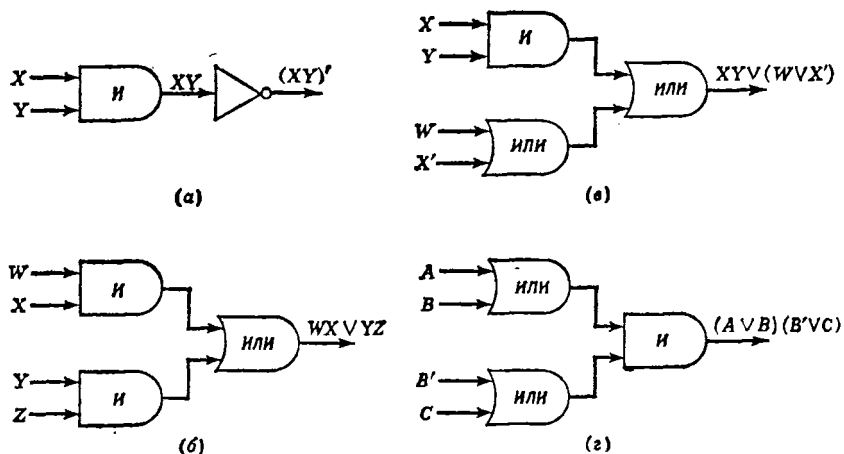
Рис. 5.4. Примеры вентильных схем.
