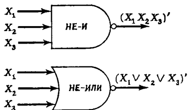
Рис. 6.13. Универсальные элементы.
