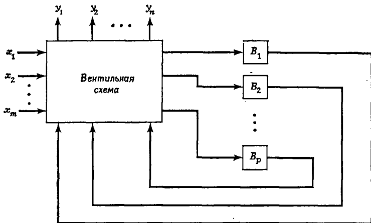
Рис. 6.20. Логическая схема последовательностной машины.
