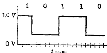
Рис. 3.1. Уровни постоянного тока и соответствующие двоичные значения.
