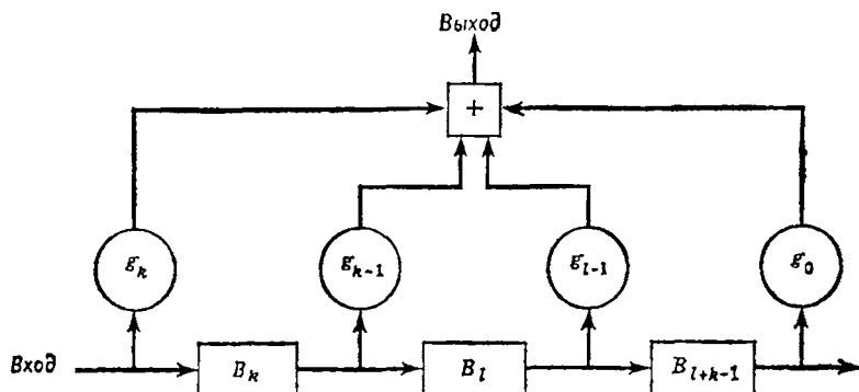
Рис. 11.2. Логическая схема, реализующая умножение на фиксированный многочлен g(x) .
