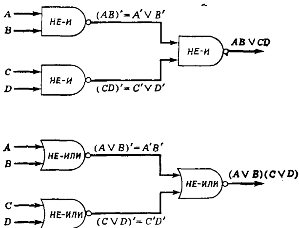
Рис. 6.14. Универсальная схема.
