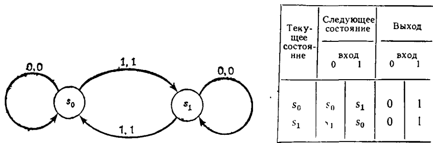
Рис. 3.6. Автомат для проверки четности.
