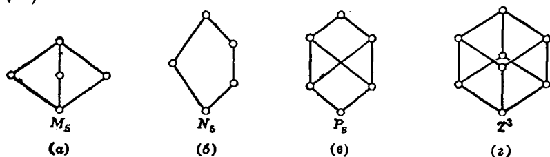
Рис. 9.1. Примеры частично упорядоченных множеств.
