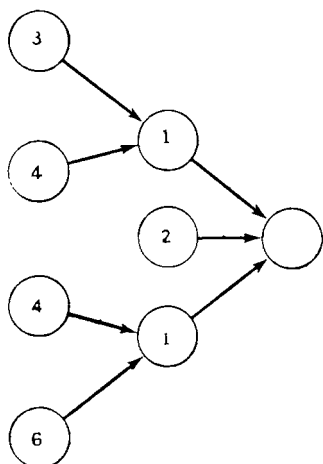
Рис. 6.3. Граф для отыскания функции M от стадии 3.
