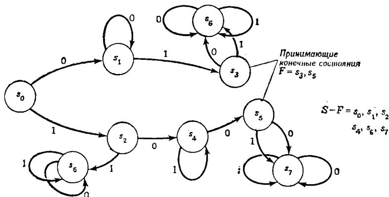
Рис. 14.3. Конечный акцептор.
