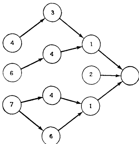
Рис. 6.4. Граф для отыскания функции M от стадии 2.
