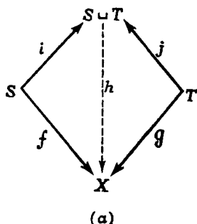
Рис. 1.2. Диаграмма универсальных отображений.
