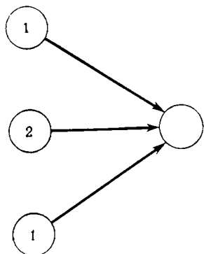
Рис. 6.2. Граф для отыскания функции M от стадии 4.
