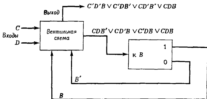
Рис. 6.23. Двоичный сумматор.
