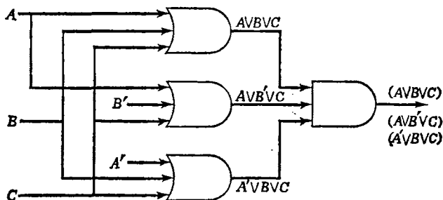
Рис. 6.11. Схема типа ИЛИ—И.
