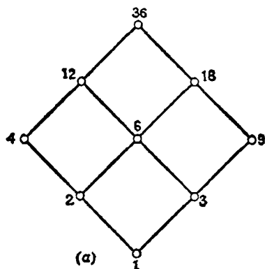
Рис. 9.2. Прямые произведения. а) делители 36; б) 2 \times M_3 .
