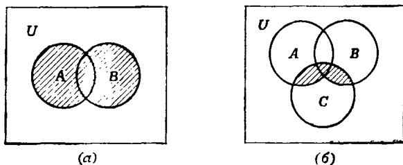
Рис. 1.1. Диаграмма Венна.
