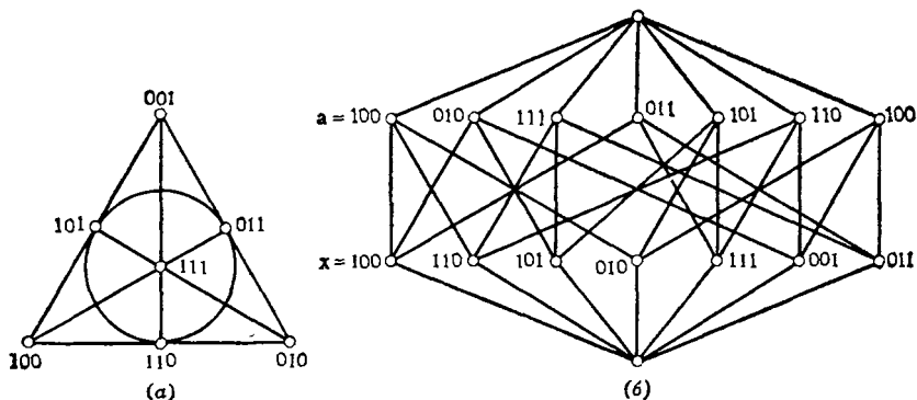
Рис. 9.5. Решетка подгрупп \Delta_4 .
