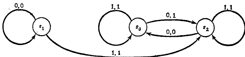
Рис. 3.5. Диаграмма с недостижимыми состояниями.
