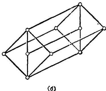
Рис. 9.2. Прямые произведения. а) делители 36; б) 2 \times M_3 .
