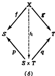
Рис. 1.2. Диаграмма универсальных отображений.
