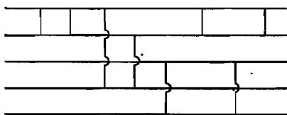
Рис. XIII.3. Двусвязная диаграмма.
