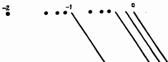
Рис. XII.8. \sigma(H_0(\theta)) .
