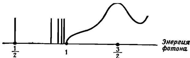
Рис. XII.4. Схематическое изображение сечения поглощения в процессе \text{He} + \gamma .
