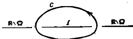
Рис. XIII.4. Контур интегрирования.
