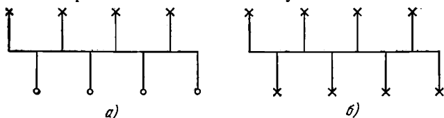
Рис. 7. Винтовая ось второго порядка (а) и плоскость скольжения (б).
