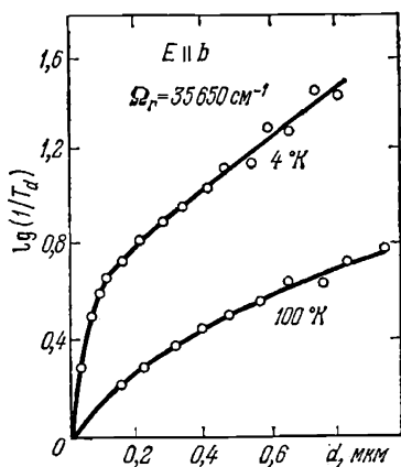
Рис. 70. Зависимость \lg(1/T_d) от толщины кристалла парадихлорбензола при температурах 4°K и 100°K.
