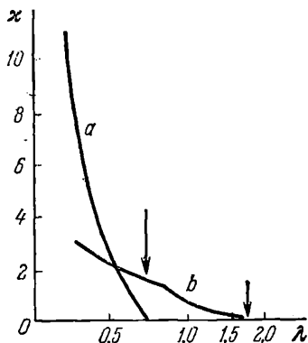
Рис. 54. Коэффициент поглощения \alpha , обусловленный прямыми (а) и не прямыми (б) переходами в Ge.
