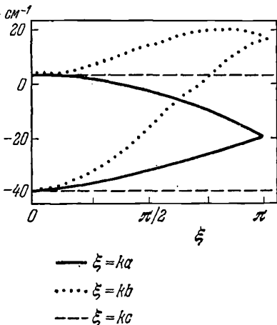
Рис. 77. Структура энергетических полос триплетных экситонов в кристалле антрацена.
