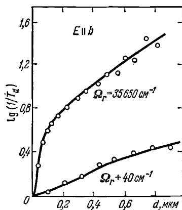
Рис. 71. Зависимость \lg(1/T_d) от толщины кристалла парадихлорбензола при температуре 4°K для двух частот.
