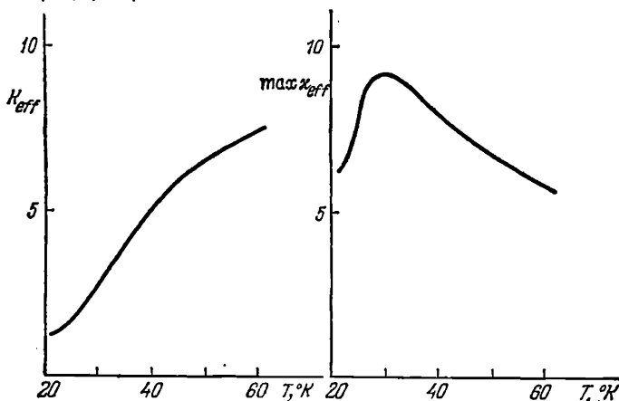
Рис. 76. Относительное изменение с температурой интегрального коэффициента поглощения и максимума кривой поглощения электронной полосы в парадихлорбензоле.
