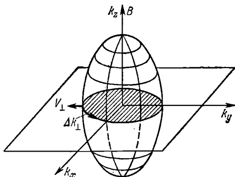
Рис. 33. Траектория движения электрона в k -пространстве, образуемая пересечением плоскости, перпендикулярной магнитному полю, и поверхностью Ферми.
