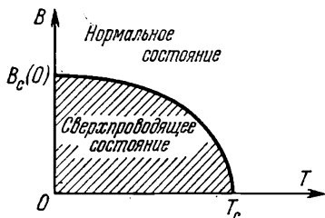
Рис. 49. Фазовая диаграмма сверх проводящего состояния в плоскости B - T .
