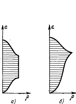
Рис. 29. Плотность одноэлектронных состояний.
