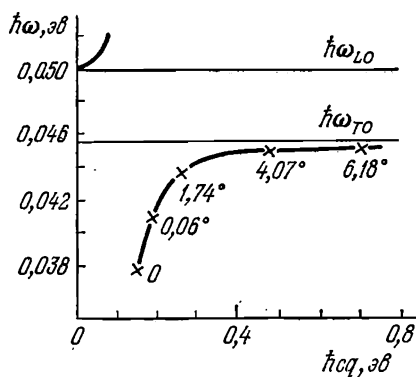
Рис. 18. Поляритонные ветви для кристалла СаР.
