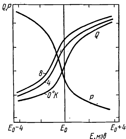
Рис. 84. Зависимости от энергии поляритонов скорости их радиационной гибели P и скорости Q перехода в состояния с другой энергией при комбинационном рассеянии в кристалле сернистого кадмия.
