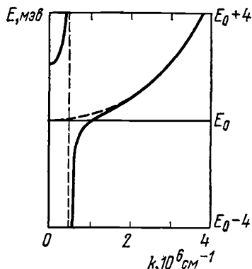
Рис. 83. Дисперсия двух поляритонных ветвей в кристалле сернистого кадмия.
