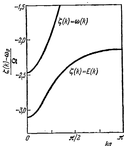
Рис. 48. Изменение энергии одноэлектронных электронных состояний при их взаимодействии с оптическими фононами.
