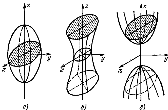
Рис. 22. Изоэнергетические поверхности в \mathbf{k} -пространстве.
