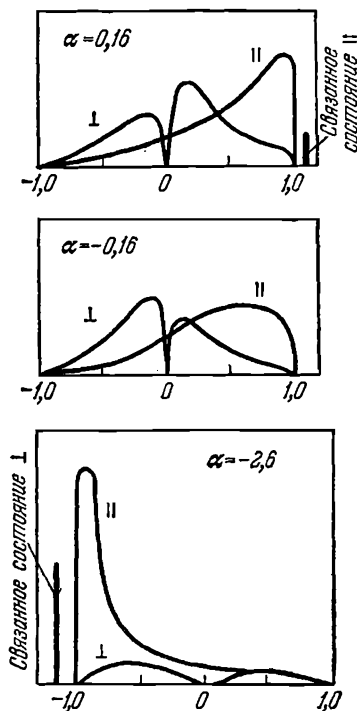
Рис. 82. Кривые поглощения поляризованного света парными экситонами при разных значениях отношения \alpha = V/|\mathcal{L}_a| .
