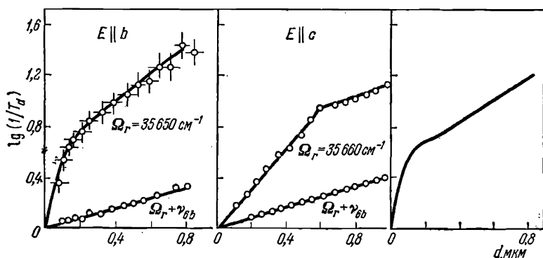
Рис. 69. Зависимость \lg(1/T_d) от толщины кристалла парадихлорбензола при 4^\circ \text{K} в области чисто электронного \Omega и вибронного \Omega_r + \gamma_{ab} переходов для разных поляризаций света.
