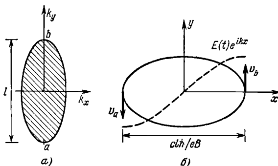
Рис. 38. Траектория движения электронов в k -пространстве (а) и в координатном пространстве (б).
