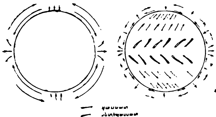
Նկ. 16. Մթնոլորտի շրջապատայտի սխեման
