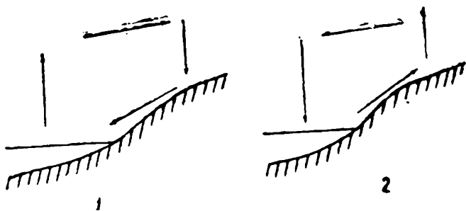
Նկ. 16. Մուստոնների ուղղաքման սխեման:
