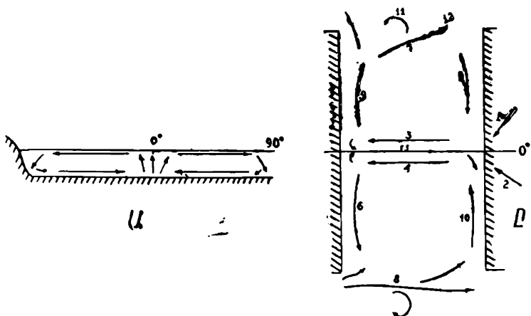
Նկ. 20. Օվկիանոսային հոսանքների սխեման: Ա — ուղղաձիգ կտրվածքում, Բ — վերեկից դիտելիս:
