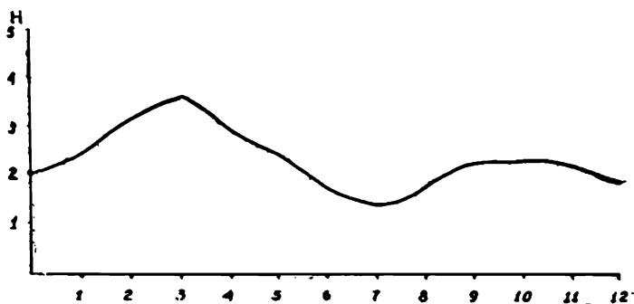
9. Լճի մակարդակի տատանումների գրաֆիկը:
