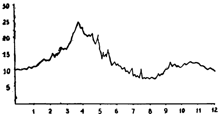
Նկ. 8. Գետի ծախսի գրաֆիկը:
