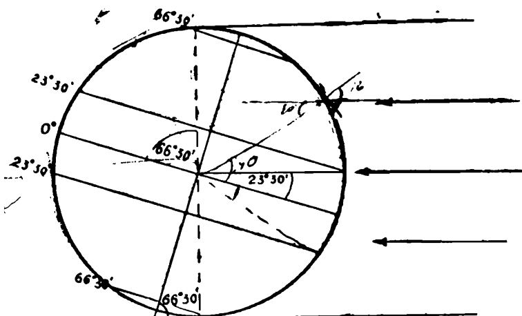
Նկ. 24. Տարվա եղանակների առաջացումը. Երկրագնդի դիրքը և Արևի ճա- ռագայթների ուղղությունը հունիսին:
