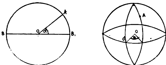
Նկ. 22. Աշխարհագրական լայնության և երկայնության պատկերացումը:
