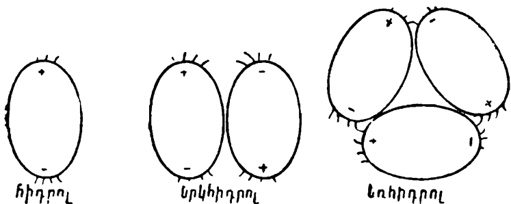
Նկ. 5. Զրի տարրեր ագրեգատային վիճակներում մոլեկուլների դասավորությունը:
