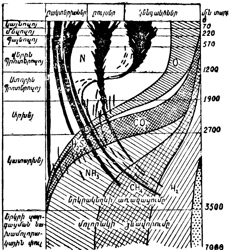
Նկ. 25. Երկրի երկրաբանական փուլերի սահմանակ (ըստ Կ. Կ. Մարկովի 1978)
