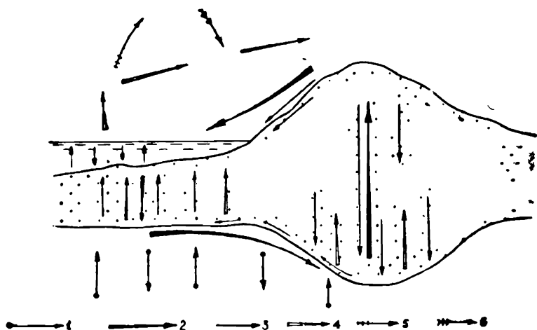
Նկ. 13. Նյութերի համաշխարհային շրջապտույտի սխեման: 1— մանթիայի նյութ, 2— պինդ նյութեր, 3— ջուր, 4— շրային գալոր- չիներ, 5— նյութի արտահոսում դեպի տիեզերք, 6— նյութի մուտք տիե- զերքից:
