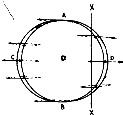
Նկ. 21. Մակրնթացության-տեղափոխության սխեման:
