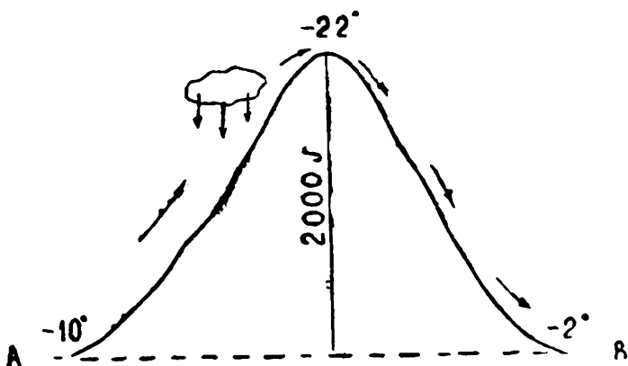
Նկ. 17. Ֆյուն քամիների առաջացման սխեման:
