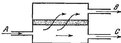
Рис. 8.1. Схема ячейки каскада разделения изотопов: А — на вход поступает смесь изотопов; В — обогащенная легким изотопом смесь, прошедшая через пористую перегородку, подается на вход следующей ступени каскада; С — обогащенная тяжелым изотопом смесь возвращается на вход ячейки предыдущего каскада
