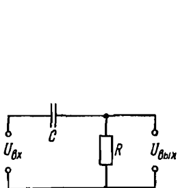
Рис. 13.5. Схема RC -цепочки
