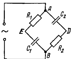
Рис. 15.1. К точкам A и B подается синусоидальное напряжение
