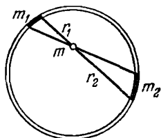
Рис. 17.2. Силы тяготения, действующие на массу m со стороны участков m_1 и m_2 , уравновешиваются
