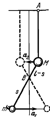
Рис. 6.2. Если верхняя нить остается вертикальной, то центр масс шаров B не перемещается по горизонтали
