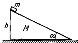
Рис. 8.1. В начальный момент брусок и клин неподвижны
