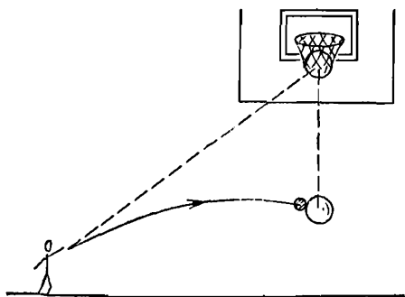
Рис. 4.1. Падающий мяч
