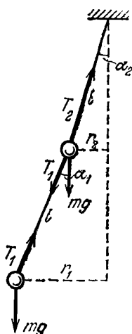
Рис. 8.3. Силы, действующие на шарик в двойном маятнике
