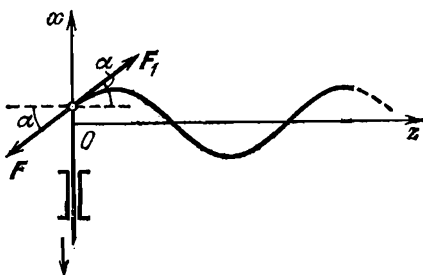
Рис. 14.2. Со стороны стержня на конец струны действует сила F
