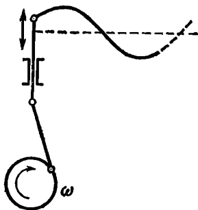
Рис. 14.1. Конец струны приводится в движение по гармоническому закону
