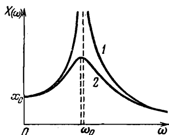
Рис. 9.3. Амплитуда вынужденных колебаний при резонансе тем меньше, чем больше затухание
