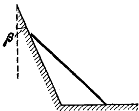
Рис. 1.1. Лестница у наклонной стенки
