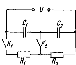
Рис. 11.1. Напряжения на конденсаторах C_1 и C_2 зависят от положения ключей K_1 и K_2
