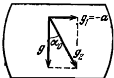
Рис. 10.2. В системе отсчета, связанной с цистерной, действует эффективное поле тяжести g_2
