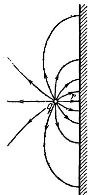
Рис. 4.1. Точечный заряд вблизи проводящей стенки
