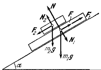
Рис. 4.2. Действующие силы при условии, что нижняя доска выскальзывает из-под верхней
