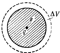
Рис. 10.1. К расчету уменьшения электростатической энергии при увеличении радиуса заряженной капли
