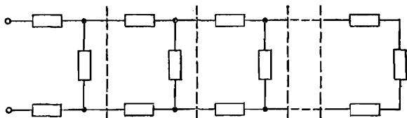
Рис. 3.1. Штриховыми линиями показаны отдельные одинаковые звенья цепочки
