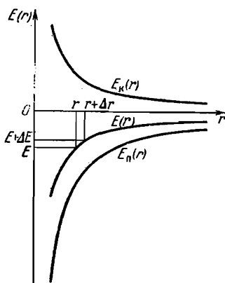
Рис. 18.1. Зависимость кинетической, потенциальной и полной энергий спутника Земли от радиуса орбиты
