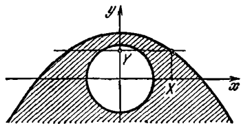
Рис. 9.3. «Мокрая» область заштрихована
