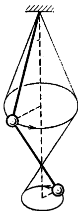
Рис. 8.4. Другое возможное движение двойного маятника
