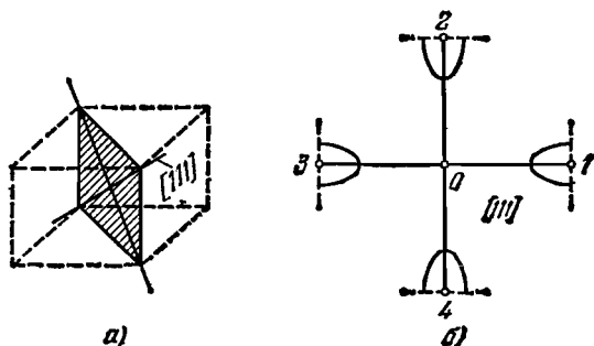
Рис. 3.6. а) Две (из четырех) пространственные диагонали куба [111] . б) Положение изоэнергетических поверхностей электронов в зоне Бриллюэна (Ge). Сечение плоскостью (110) . Пунктир — границы зоны Бриллюэна.
