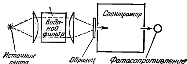
Рис. 9.4. Наблюдение рекомбинационного излучения при оптическом возбуждении.
