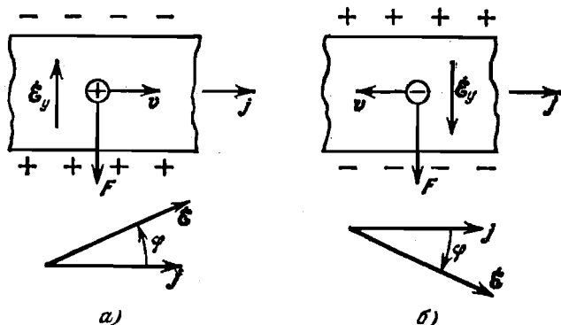
Рис. 1.2. Знак угла Холла: а) \varphi > 0 ; б) \varphi < 0 .
