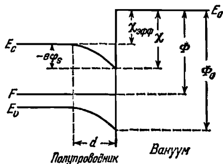
Рис. 10.16. Влияние изгиба зон у поверхности на электронную эмиссию. \Phi — термоэлектронная работа выхода, \Phi_0 — оптическая работа выхода, \chi — электронное сродство, \chi_{\text{эфф}} — эффективное электронное сродство.
