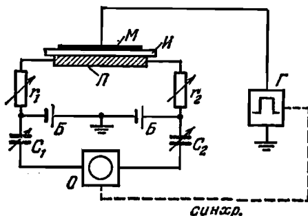
Рис. 10.11. Наблюдение релаксации проводимости в эффекте поля. \Pi — полупроводник, M — металлическая обкладка, И — изолятор, \Gamma — генератор прямоугольных импульсов, O — осциллограф, B — источники постоянного тока.
