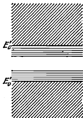
Рис. 19.3. Области непрерывного и дискретного спектров в сильно легированном полупроводнике. Горизонтальная штриховка указывает область дискретного спектра, косая — непрерывного.
