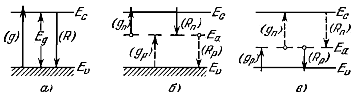
Рис. 7.3. Различные типы оптической генерации: а) собственная генерация пар; б) примесная генерация электронов; в) примесная генерация дырок.
