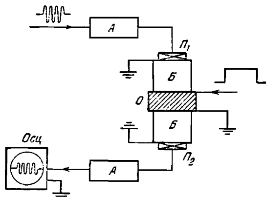
Рис. 15.5. Измерение электронного поглощения и усиления упругих волн в полупроводниках. А — аттенуаторы, Осц — осциллограф.
