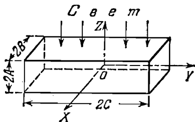
Рис. 10.19. К расчету фотопроводимости в тонких пластинках.
