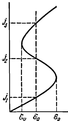
Рис. 16.11. Вольтамперная характеристика S -типа.
