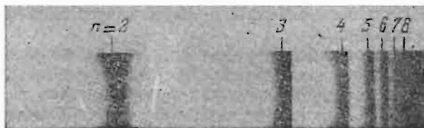
Рис. 17.1. Спектрограмма желтой серии экситона в \text{Cu}_2\text{O} при T = 1,3 К.
