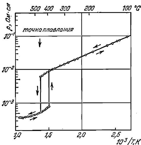
Рис. 2.15. Зависимость удельного сопротивления теллура от температуры. Смещение скачка сопротивления при охлаждении обусловлено переохлаждением расплава.
