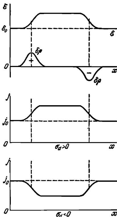
Рис. 16.12. Флуктуации напряженности поля, объемной плотности заряда и плотности тока при положительной и отрицательной дифференциальной проводимости. Через \epsilon_0 и j_0 обозначены средние значения напряженности поля и плотности тока.
