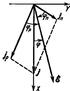
Рис. 1.8. Эффект Холла при смешанной проводимости.
