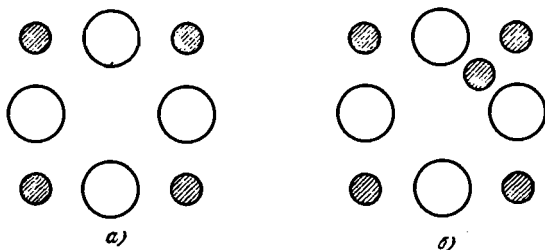
Рис. 2.21. а) Вакансия. б) Вакансия с междоузельным атомом.
