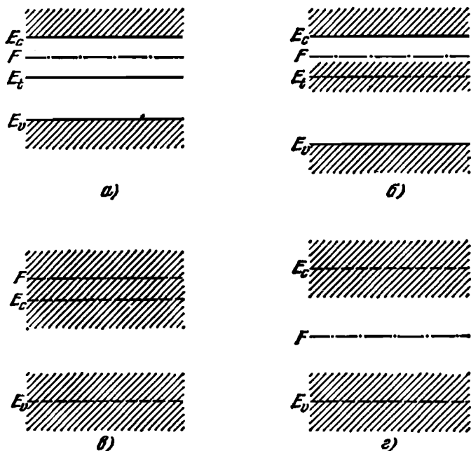
Рис. 19.1. Энергетический спектр полупроводника n -типа в зависимости от уровня легирования (заштрихованы области дозванных значений энергии). а) Слабо легированный полупроводник. Штрихпунктиром указано положение уровня Ферми при низких температурах. б) Промежуточно легированный полупроводник. Пунктирная линия указывает положение бывшего уровня примеси, штрихпунктирная — положение уровня Ферми при низких температурах. в) Сильно легированный полупроводник. Пунктирными линиями указаны бывшие границы зон проводимости и валентной, штрихпунктирной — уровень Ферми в отсутствие компенсации. г) Сильно легированный компенсированный полупроводник.
