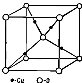
Рис. 2.12. Элементарная ячейка куприта Cu_2O .
