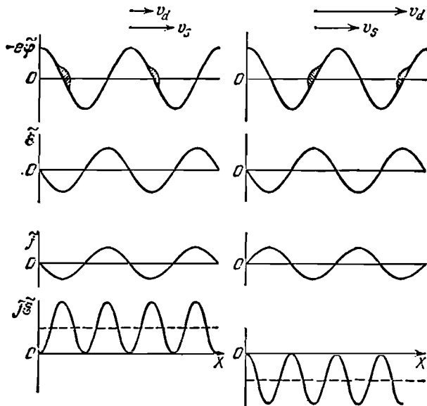
Рис. 15.4. Колебание потенциала \tilde{\phi} , поля \tilde{\mathcal{E}} , тока \tilde{j} и мощности \tilde{j}\tilde{\mathcal{E}} при v_d < v_s (слева) и v_d > v_s (справа).
