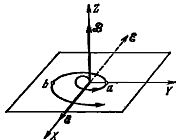
Рис. 4.2. К объяснению диамагнитного (циклотронного) резонанса.
