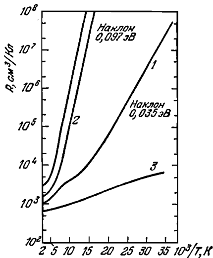
Рис. 5.15. Зависимость постоянной Холла от температуры для различных образцов германия, содержащих цинк, частично компенсированный сурьмой. 1 — N_{\text{Sb}} < N_{\text{Zn}} (p-тип); 2 — N_{\text{Zn}} < N_{\text{Sb}} < 2N_{\text{Zn}} (p-тип); 3 — N_{\text{Sb}} > 2N_{\text{Zn}} (n-тип).
