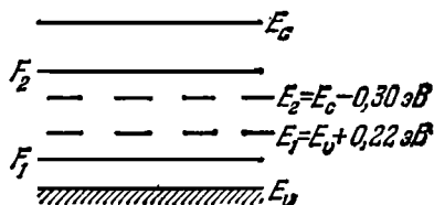
Рис. 9.8. Энергетические уровни никеля в германии.
