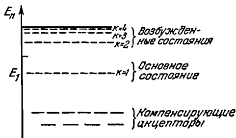
Рис. 5.5. Энергетический спектр связанного электрона при наличии возбужденных состояний.
