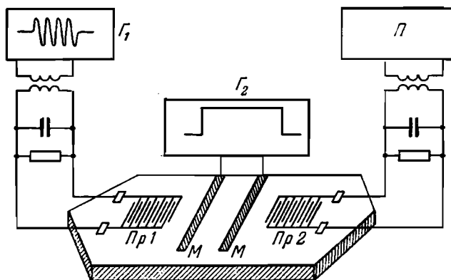
Рис. 15.10. Усиление поверхностных упругих волн дрейфом электронов. G_1 — импульсный генератор высокой частоты, G_2 — генератор прямоугольных импульсов ускоряющего напряжения, P — радиоприемник, Пр1 и Пр2 — электромеханические преобразователи, M, M — металлические ускоряющие электроды.
