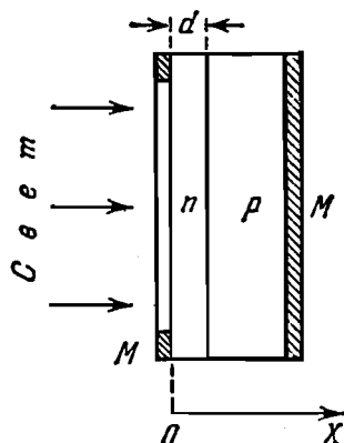
Рис. 11.9. К диффузионной теории вентильного фотоэлемента.
