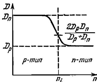
Рис. 7.16. Зависимость коэффициента амбиполярной диффузии от концентрации электронов.
