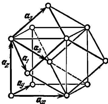
Рис. 2.2. Прямоугольная элементарная ячейка объемноцентрированной кубической решетки (основные векторы a_x , a_y , a_z ) и ромбоэдрическая ячейка решетки Браве (основные векторы a_1 , a_2 , a_3 ).
