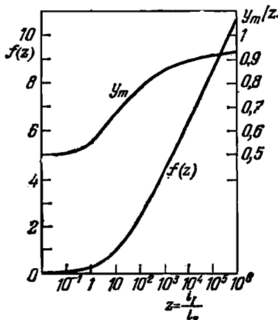
Рис. 11.10. Зависимость оптимального тока фотоэлемента y_m = i_m/i_s от светового тока z = i_l/i_s и функции f(z) .
