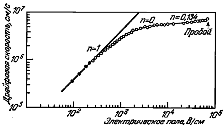
Рис. 16.1. Зависимость дрейфовой скорости от напряженности электрического поля в n -Ge при T = 300 К. Число n характеризует зависимость v_d \sim E^n .
