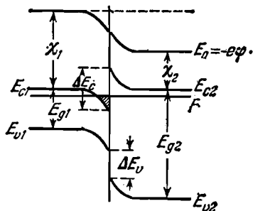
Рис. 8.11. Пример энергетической диаграммы изотипного n-n -гетероперехода. Заштрихованная часть вырождена.
