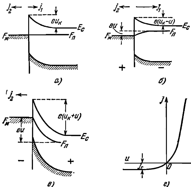
Рис. 6.15. Выпрямление в контакте металл — полупроводник: а) внешнее напряжение u = 0 ; б) проходное направление тока; в) запиорное направление тока; г) вольтамперная характеристика (схематически).
