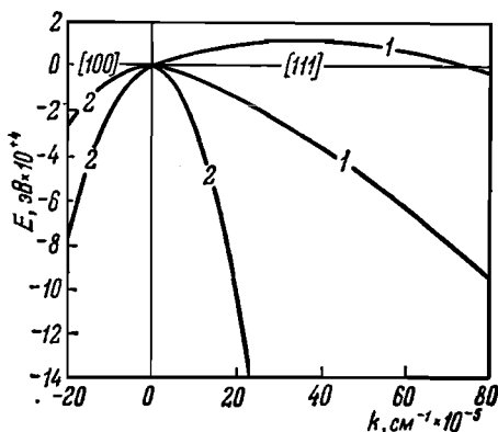
Рис. 3.10. Законы дисперсии для верхних валентных подзон в InSb. По оси абсцисс отложены значения квазиволнового вектора k = p/h в направлениях [111] (справа) и [100] (слева). Цифры у кривых указывают степени вырождения зон. Две верхние кривые в правой части рисунка отвечают зоне тяжелых дырок, нижние — зоне легких дырок.
