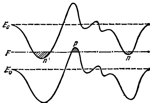
Рис. 19.7. Сильное флуктуационное искривление зон. Буквами n и p отмечены заштрихованные области, в которых при низких температурах образуются «капли» электронов и дырок.
