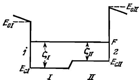
Рис. 6.7. Энергетическая диаграмма двух контактирующих металлов.
