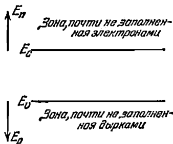
Рис. 4.1. Направления отсчета энергий электронов проводимости E_n(p) и дырок E_p(p) .
