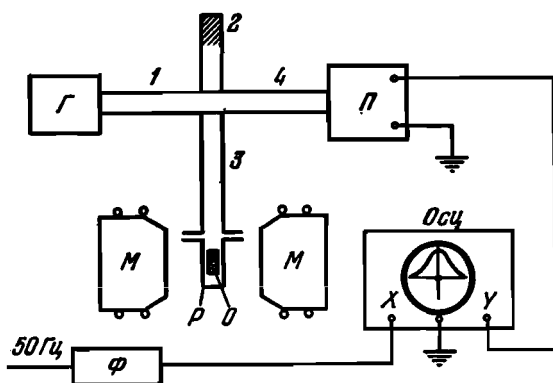
Рис. 4.4. Схема наблюдения диамагнитного резонанса. Г — генератор СВЧ колебаний, П — приемник, Ось — осциллограф, Р — резонансная полость с образцом О, ММ — электромагнит, Ф — фазовращатель.
