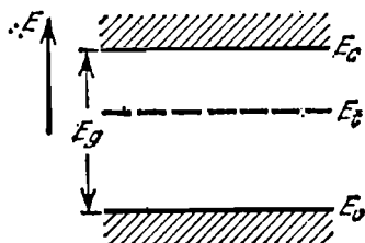
Рис. 2.19. Уровни энергии электронов в кристалле при наличии простых доноров или акцепторов.
