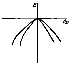
Рис. 3.5. Пример вырождения зон в точке максимума.
