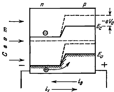
Рис. 11.6. Происхождение вентильной фотоэдс. Пунктиром показаны края энергетических зон в темноте.
