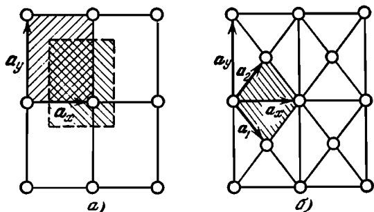
Рис. 2.1. Двумерная прямоугольная решетка: а) простая; б) центрированная. a_1 , a_2 — основные векторы решетки Браве.
