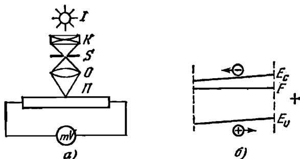
Рис. 11.3. а) Наблюдение объемной фотоэдс. I — источник света, K — конденсор, S — щель, O — объект, П — полупроводник, mV — милливольтметр. б) Направления движения фотоэлектронов и фотодырок.
