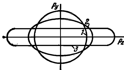
Рис. 16.4. Контуры постоянной функции распределения в пространстве квазимпульсов. Ось Z направлена вдоль вектора напряженности электрического поля; оси Y и X (последняя не показана) эквивалентны. Кривая 1 изображает контур при \xi = 0 ; кривые 2 и 3 отвечают слабо и сильно неупругому рассеянию ( \eta \ll 1 и \eta \approx 1 ).
