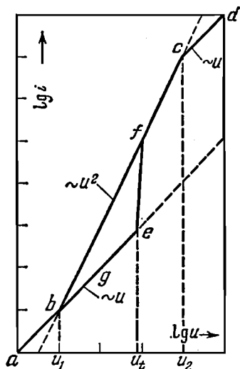
Рис. 6.14. Зависимость тока от напряжения (пронзвольные единицы) для ТОПЗ. abcd — без ловушек; abefcd — при равномерном распределении глубоких ловушек.
