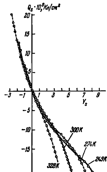
Рис. 10.10. Пример зависимости заряда поверхности от поверхностного потенциала для образца германия.
