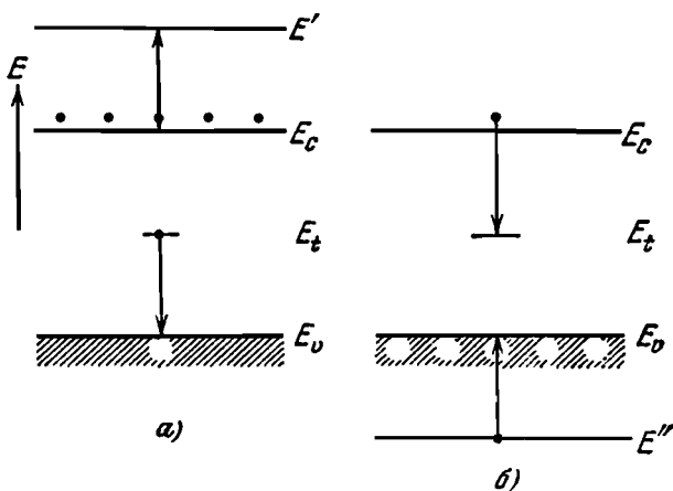
Рис. 17.3. Схема ударного процесса захвата неосновного носителя заряда на ловушку: а) захват дырки в полупроводнике n -типа, б) захват электрона в полупроводнике p -типа.
