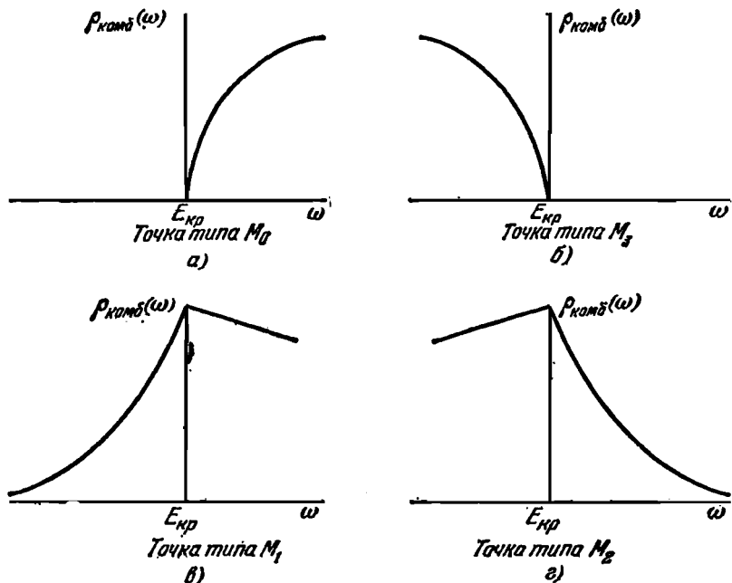
Рис. 18.9. Комбинированная плотность состояний вблизи критических точек (схематически).
