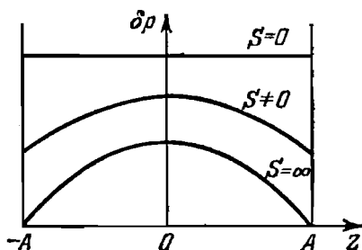
Рис. 10.20. Стационарное распределение фотодырочек в тонкой пластинке при разной скорости поверхностной рекомбинации. Однородная генерация в объеме.
