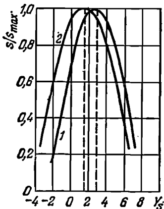
Рис. 10.21. Пример зависимости скорости поверхностной рекомбинации s/s_{\max} от поверхностного потенциала в германии. 1 — вакуум, 2 — сухой кислот; 300 K [1].
