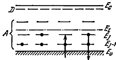
Рис. 5.14. Частично компенсированные многоядерные акцепторы. Полупроводник p -типа.
