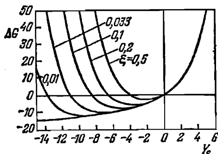
Рис. 10.7. Зависимость изменения проводимости \Delta G германия n -типа (произвольные единицы) от поверхностного потенциала Y_s = e\phi_s/kT .
