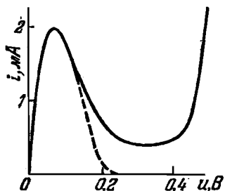
Рис. 8.5. Экспериментальная вольтамперная характеристика германиевого туннельного диода. 300 К, \Delta p = 6 \text{ кТ} , \Delta n = 8 \text{ кТ} . (Пунктирная кривая соответствует схеме рис. 8.4.)
