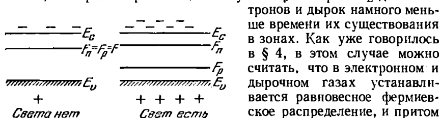
Рис. 7.6. К понятию квазиуровней Ферми.
