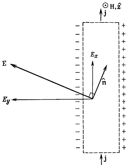
Фиг. 12.11. Схематическое изображение тока \mathbf{j} в проводнике, перпендикулярном магнитному полю \mathbf{H} , в случае, когда в реальном пространстве в направлении \hat{n} , перпендикулярном полю, лежит открытая орбита.
