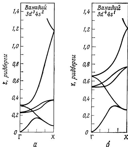
Фиг. 11.1. Энергетические зоны ванадия, рассчитанные для двух возможных способов выбора кристаллического потенциала U(r) . (Из работы [3].)
