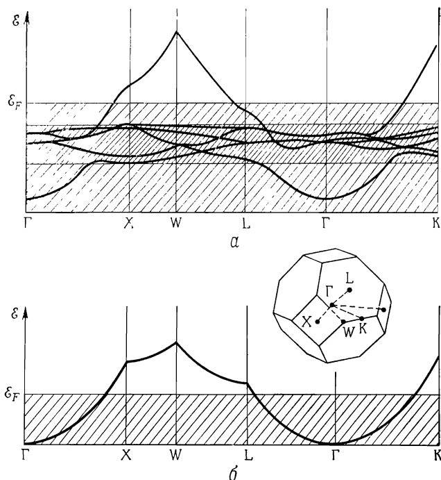
Фиг. 15.4. a — рассчитанные энергетические зоны в меди. (По работе [3].)
