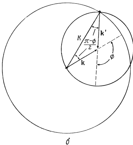
Фиг. 6.10. Построение Эвальда для порошкового метода.
