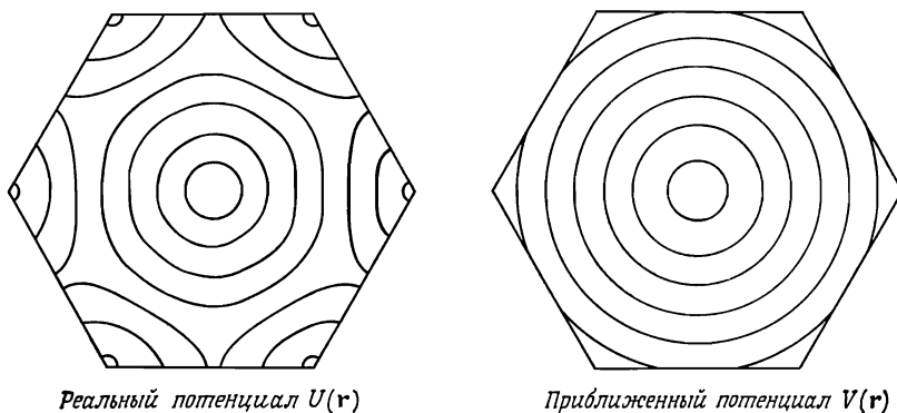
Фиг. 11.3. Эквипотенциали [т. е. кривые постоянного значения потенциала U(\mathbf{r}) ] внутри элементарной ячейки.
