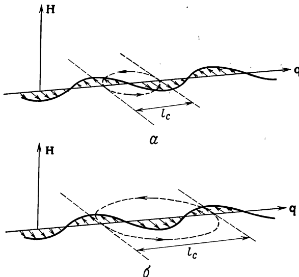
Фиг. 14.7. a — электронная орбита с диаметром l_c , равным половине длины волны. Орбита расположена таким образом, что электрическое поле, сопровождающее звуковую волну, вызывает ускорение электрона во всех точках орбиты.
