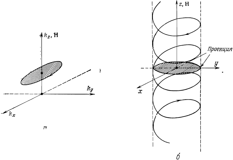
Фиг. 12.7. Проекция орбиты в r -пространстве (б) на плоскость, перпендикулярную полю, получается из орбиты в k -пространстве (а) путем изменения масштаба в отношении \hbar c / eH и поворота на 90^\circ вокруг оси, определяемой вектором \mathbf{H} .
