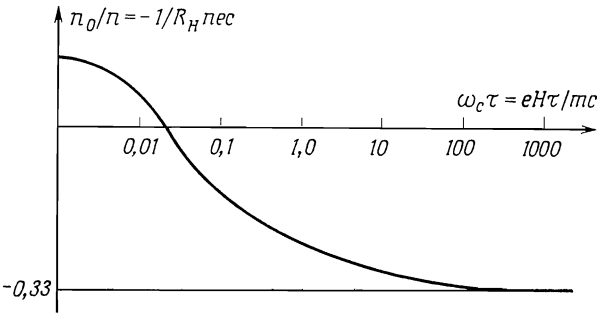
Фиг. 1.4. Зависимость величины n_0/n = -1/R_H пес от \omega_c \tau для алюминия. (Из работы [5].)
