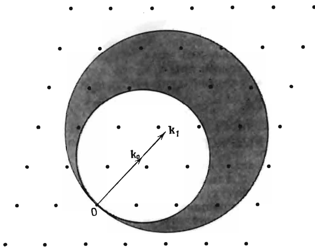
Фиг. 6.8. Построение Эвальда для метода Лауэ.
