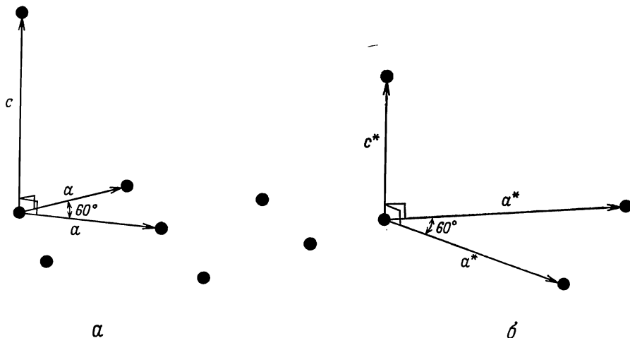
Фиг. 5.1. a — основные векторы для простой гексагональной решетки Бравэ; b — основные векторы для решетки, обратной той, которая порождена основными векторами решетки a .
