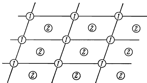
Фиг. 7.6. Центрированная моноклинная решетка Бравэ при наблюдении вдоль c -оси.
