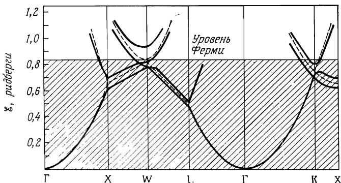
Фиг. 11.9. Сравнение рассчитанных валентных зон для алюминия (три электрона над конфигурацией неона с заполненными оболочками) с зонами свободных электронов (штриховые линии).
