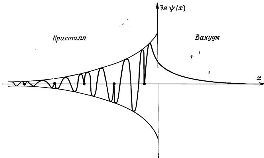
Фиг. 18.9. Волновая функция одноэлектронного поверхностного уровня, изображенная в направлении x , перпендикулярном поверхности.
