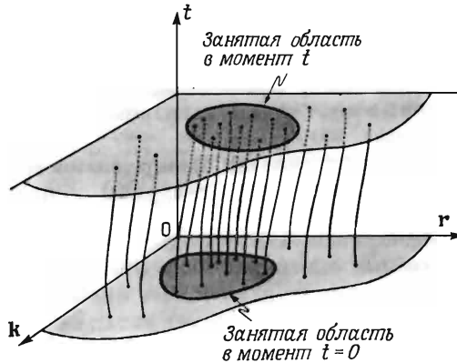
Фиг. 12.5. Схематическое изображение временной эволюции орбит в полуклассическом фазовом пространстве ( \mathbf{r} и \mathbf{k} представлены как одна координата).
