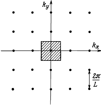
Фиг. 2.2. Точки двумерного k -пространства, имеющие координаты k_x = 2\pi n_x/L , k_y = 2\pi n_y/L .
