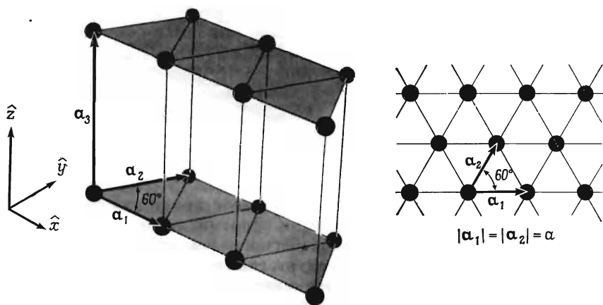
Фиг. 4.19. Простая гексагональная решетка Браве.
