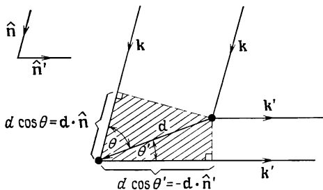
Фиг. 6.4. Построение, показывающее, что разность хода лучей, рассеянных на двух точках, находящихся на расстоянии \mathbf{d} друг от друга, определяется выражением (6.3) или (6.4).
