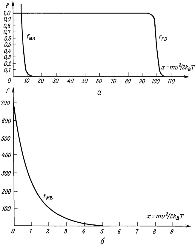
Фиг. 2.1. a — распределения Максвелла — Больцмана f_{MB} и Ферми — Дирака f_{FD} при типичных металлических плотностях и комнатной температуре.
