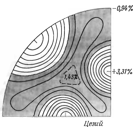
Фиг. 15.1. Определенные экспериментально поверхности Ферми в щелочных металлах. (Из работы [1].)
