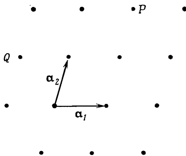
Фиг. 4.1. Произвольная двумерная решетка Бравэ, не обладающая никакой дополнительной симметрией (косая сеть).
