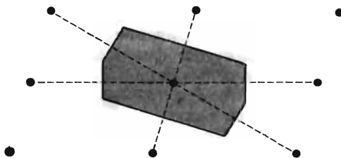
Фиг. 4.14. Ячейка Вигнера — Зейтца для двумерной решетки Бравэ.
