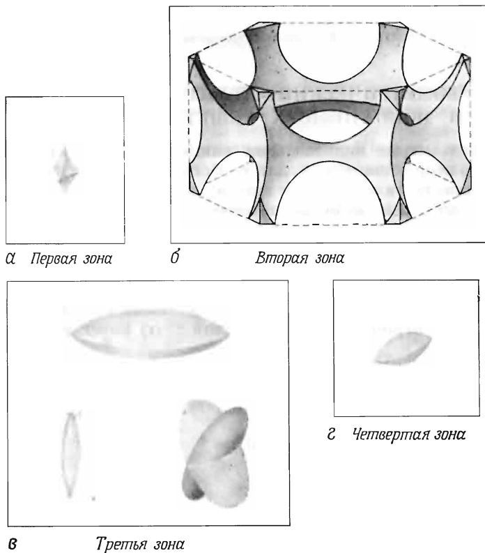
Фиг. 9.11. Поверхность Ферми для свободных электронов в двухвалентном г. п. у. металле с идеальным отношением c/a = 1,633 . (Из работы [5].)
