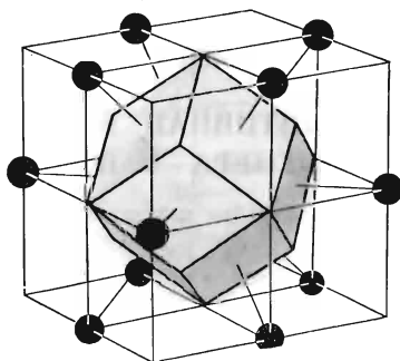
Фиг. 4.16. Ячейка Вигнера — Зейтца для г. ц. к. решетки Бравэ («ромбический додекаэдр»).
