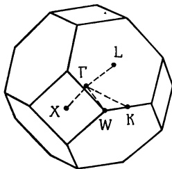
Фиг. 10.5. Первая зона Бриллюэна для г. ц. к. кристаллов.
