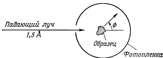
Фиг. 6.13. Схематическое изображение камеры Дебая — Шеррера. Дифракционные максимумы регистрируются на полоске фотоленки.
