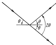
Фиг. 6.2. Брэгговский угол \theta , равный половине полного угла отклонения падающего луча.
