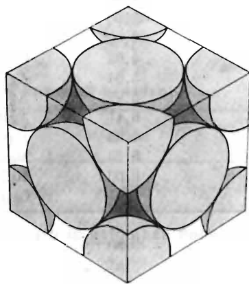
Фиг. 4.23. Вырезанная в форме куба часть пространства, заполненная сферами с гранецентрированной кубической плотной упаковкой.
