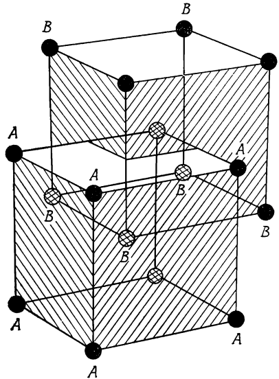
Фиг. 4.5. Несколько узлов объемноцентрированной кубической решетки Бравэ.
