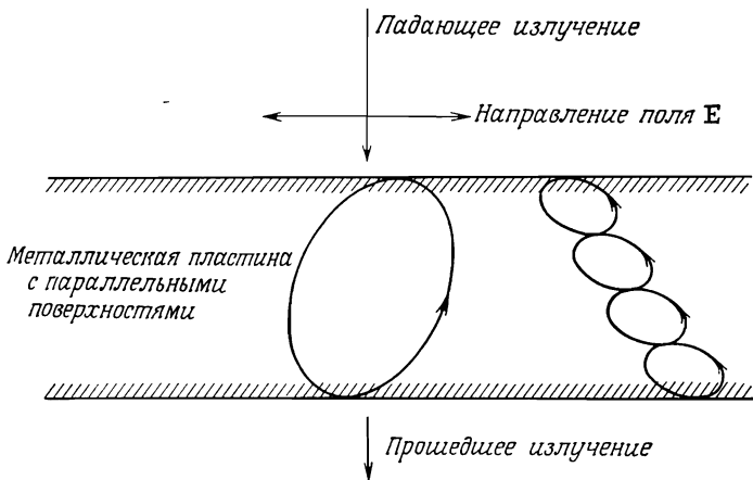
Фиг. 14.10. Эффект Гантмахера в параллельном поле.
