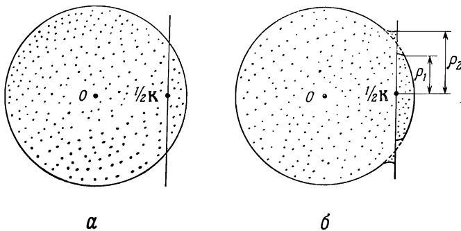
Фиг. 9.6. а — сфера свободных электронов, пересекающая брэгговскую плоскость, удаленную на 1/2 K от начальной точки ( U_k = 0 );
