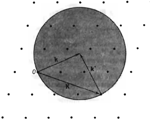
Фиг. 6.7. Построение Эвальда.
