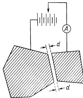
Фиг. 18.5. Измерение контактной разности потенциалов.
