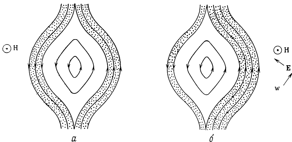
Фиг. 12.10. Сечение поверхностей постоянной энергии плоскостью, перпендикулярной магнитному полю H ; показаны занятые открытые (в областях с точками) и замкнутые (в светлых областях) орбиты.
