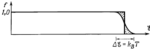
Фиг. 2.4. Функция Ферми при не равной нулю температуре T .
