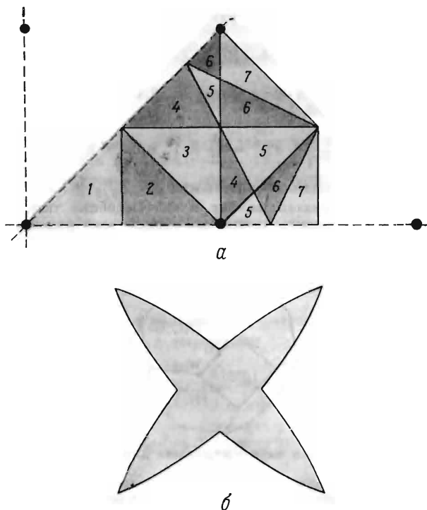
Фиг. 9.15. a — первые семь зон Бриллюэна для двумерной квадратной решетки.
