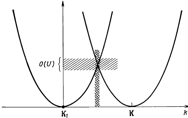
Фиг. 9.1. Для значений k , лежащих в заштрихованных интервалах, уровни свободных электронов \mathcal{E}_{k-K_1} и \mathcal{E}_{k-K} отличаются на величину O(U) .
