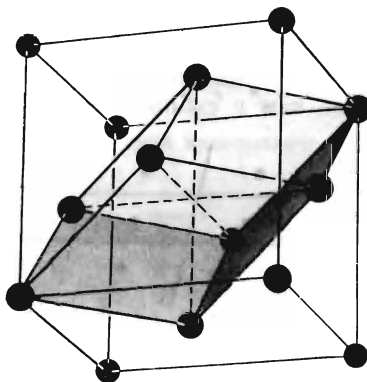
Фиг. 4.12. Примитивная и условная ячейки для г. ц. к. решетки Бравэ.
