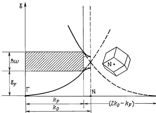
Фиг. 15.9. Определение пороговой энергии межзонного поглощения в модели свободных электронов для щелочных металлов.
