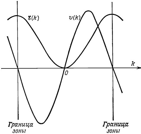
Фиг. 12.4. Зависимость величин \mathcal{E}(k) и v(k) от k [или от времени с учетом формулы (12.17)] в одномерном случае.
