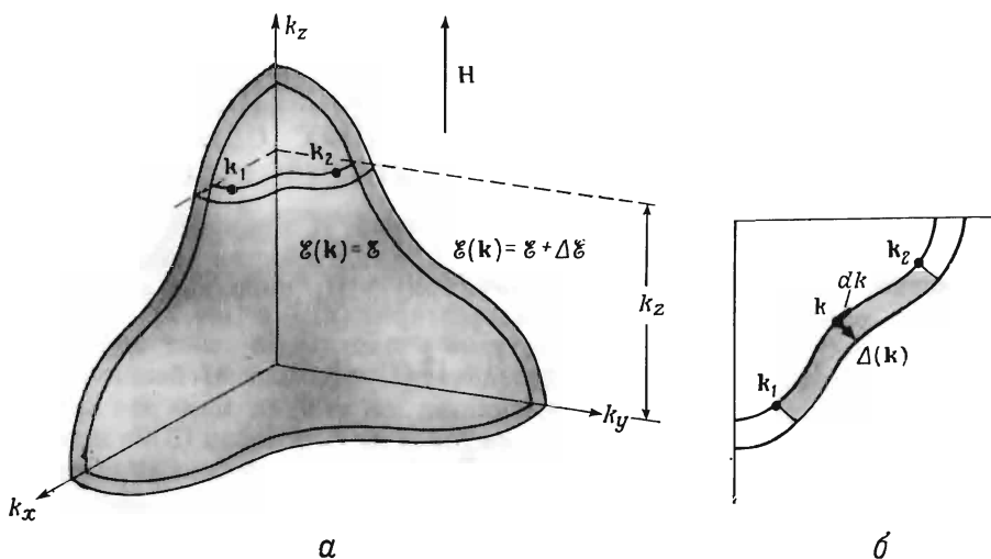
Фиг. 12.9. Изменение геометрии орбит (магнитное поле \mathbf{H} направлено вдоль оси z ).
