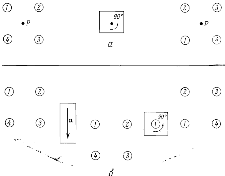
Фиг. 7.1. a — построение, показывающее, что простая кубическая решетка переходит в саму себя при повороте на 90^\circ вокруг оси, не содержащей точек решетки. Ось поворота перпендикулярна плоскости чертежа; показаны только четыре точки решетки, лежащие ближе всего к оси в одной атомной плоскости.
