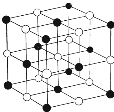
Фиг. 4.24. Структура типа хлорида натрия.
