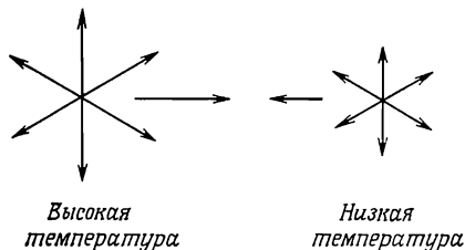
Фиг. 1.6. Схематическое изображение соотношения между градиентом температуры и потоком тепла.
