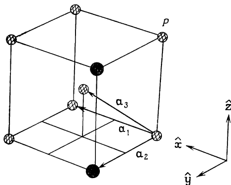
Фиг. 4.6. Тройка основных векторов (4.3) для о. ц. к. решетки Бравэ. Чтобы получить эту решетку, необходимо взять все линейные комбинации основных векторов с целыми коэффициентами. Для точки P , например, P = -a_1 - a_2 + 2a_3 .
