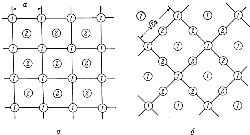
Фиг. 7.4. Два способа представления центрированной тетрагональной решетки Бравэ (вид вдоль c -оси).
