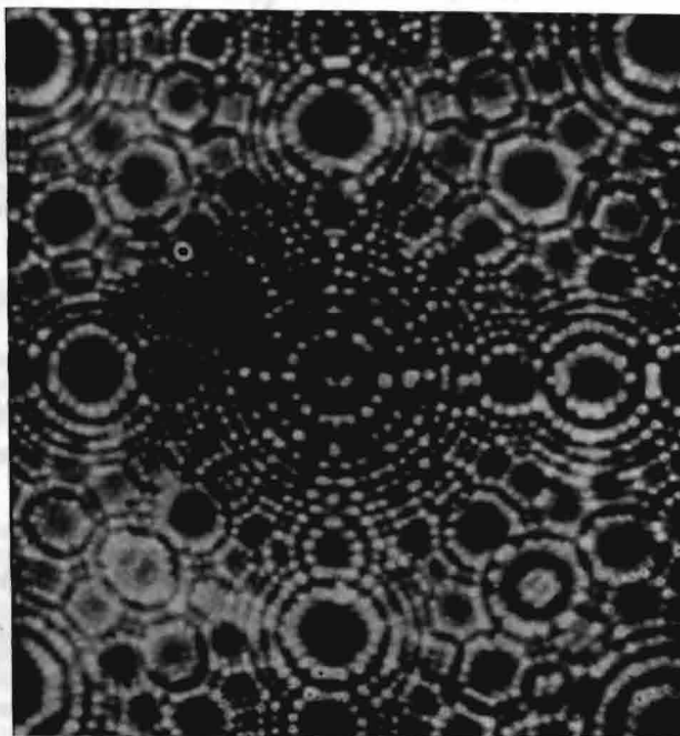
Фиг. 18.8. Ионная микрофотография острия, изготовленного из золота (для получения изображения был использован неон, а не гелий). (Из работы [2].)
