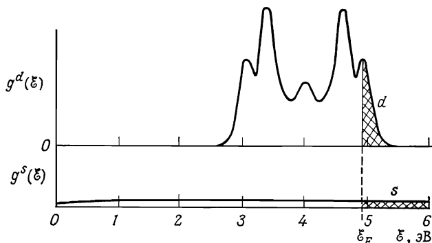
Фиг. 15.19. Качественные особенности вкладов d - и s -зон в плотность уровней переходного металла. (По работе [16].)
