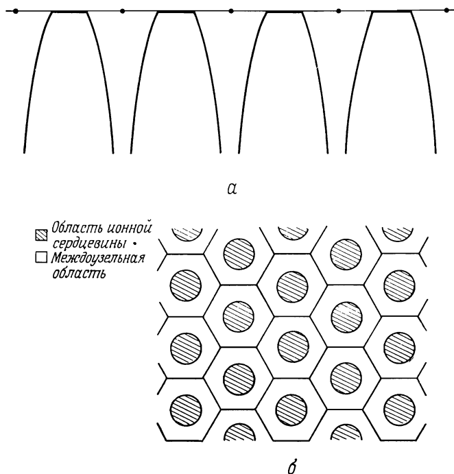
Фиг. 11.6. а — MT-потенциал, изображенный вдоль линии ионов; б — MT-потенциал постоянен (равен нулю) в области между узлами и соответствует изолированному иону в областях ионной сердцевинки.
