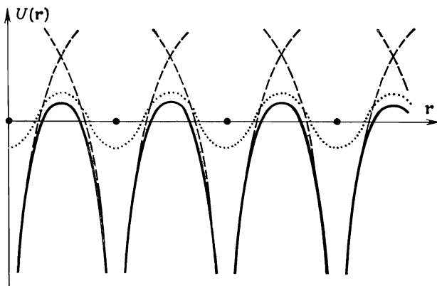
Фиг. 8.1. Типичный кристаллический периодический потенциал, изображенный вдоль линии местонахождения ионов и вдоль линии, проходящей посередине между плоскостями ионов.
