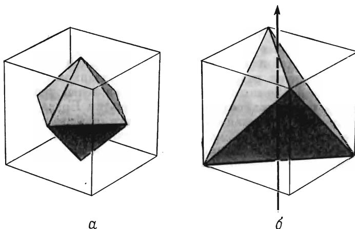
Фиг. 7.2. а — всякая операция симметрии куба является также операцией симметрии правильного октаэдра, и наоборот, поэтому группа симметрии куба идентична группе октаэдра. б — не всякая операция симметрии куба является операцией симметрии правильного тетраэдра; например, поворот на 90^\circ вокруг указанной вертикальной оси переводит в себя куб, но не тетраэдр.
