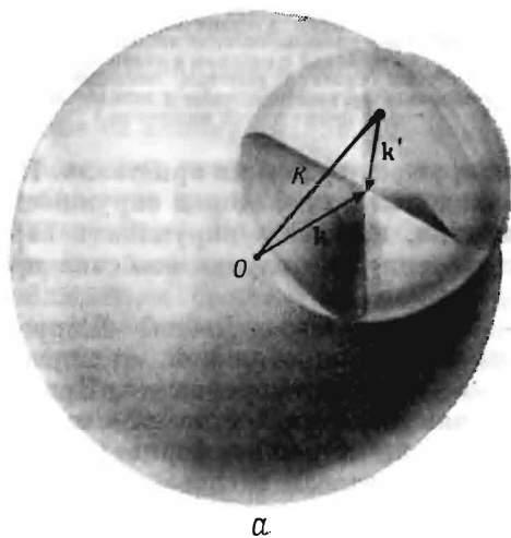
Фиг. 6.10. Построение Эвальда для порошкового метода.
