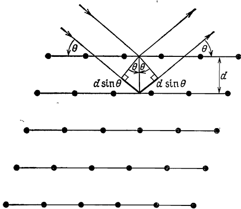
Фиг. 6.1. Брэгговское отражение от определенного семейства атомных плоскостей, отстоящих на расстоянии d .
