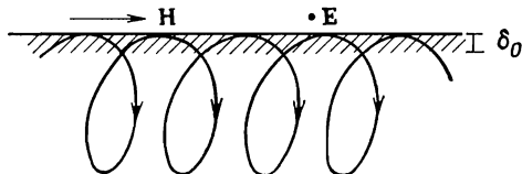
Фиг. 14.8. Геометрия эффекта Азбеля — Канера в параллельном магнитном поле.
