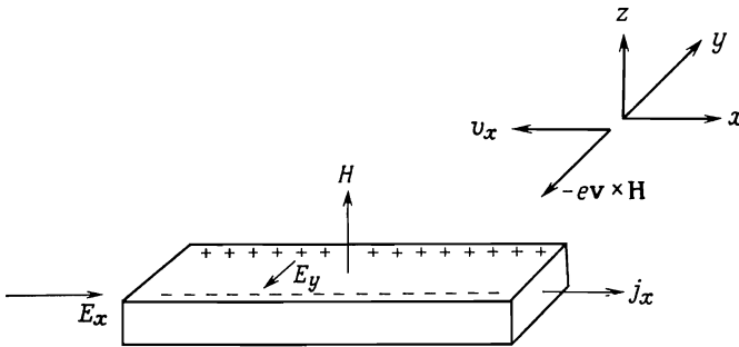
Фиг. 1.3. Схема эксперимента Холла.
