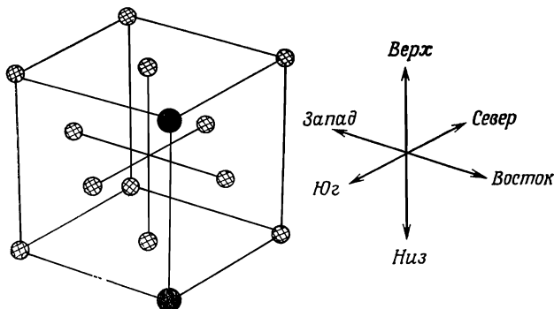
Фиг. 4.8. Некоторые точки г.ц.к. решетки Бравэ.
