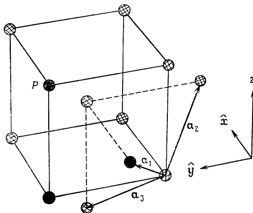
Фиг. 4.7. Более симметричная тройка основных векторов (4.4) для о. ц. к. решетки Бравэ. Для точки P , например, P = 2a_1 + a_2 + a_3 .
