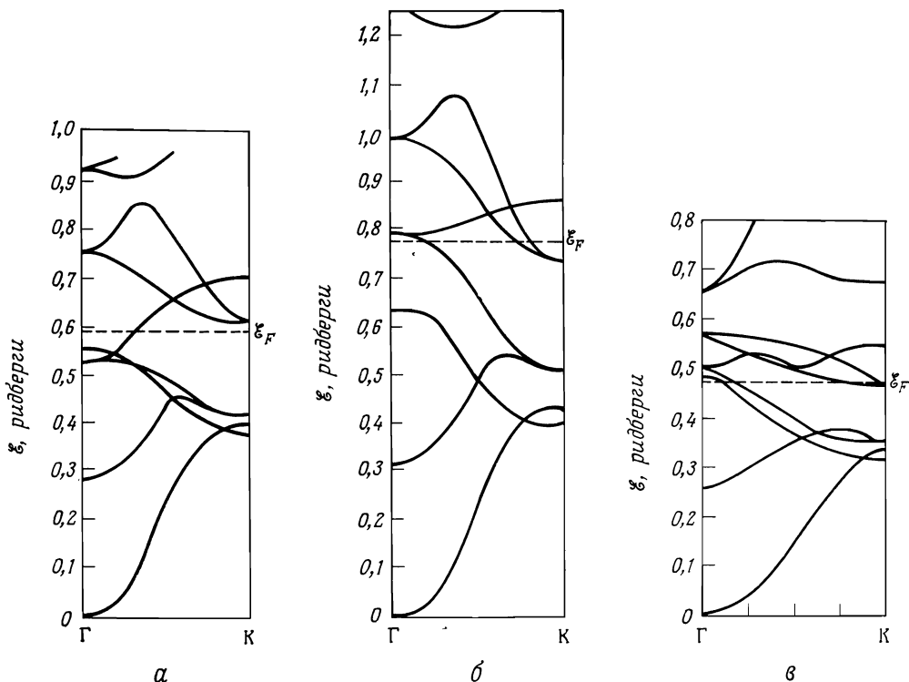
Фиг. 11.8. Три рассчитанные зонные структуры для титана.
