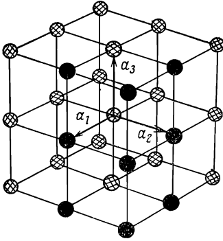
Фиг. 4.2. Трехмерная простая кубическая решетка Бравэ.
