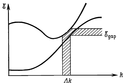
Фиг. K.1. К рассмотрению магнитного пробоя.
