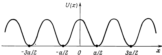
Фиг. 8.4. Одномерный периодический потенциал U(x) .
