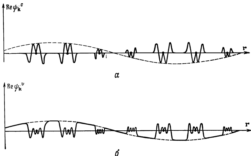
Фиг. 11.2. a — характерная пространственная зависимость волновой функции \psi_k^c(\mathbf{r}) электронов ионного остова.
