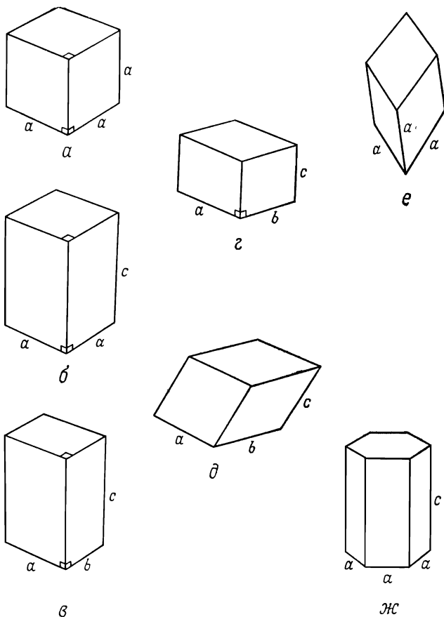
Фиг. 7.3. Объекты с симметриями точечных групп решеток Бравэ, принадлежащих семи кристаллическим системам: кубической (а), тетрагональной (б), ромбической (в), моноклинной (г), триклинной (д), тригональной (е), гексагональной (ж).
