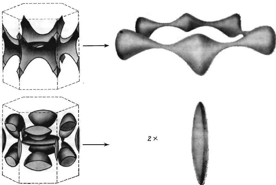
Фиг. 15.13. Найденная экспериментально поверхность Ферми бериллия. (Из работы [9].) «Монстр» свободных электронов (вверху слева) стягивается в «венки» (вверху справа), а все остальные куски поверхности Ферми свободных электронов (внизу слева), за исключением двух «сигар» (внизу справа), исчезают. В «венке» содержатся дырки, а в «сигарах» — электроны.
