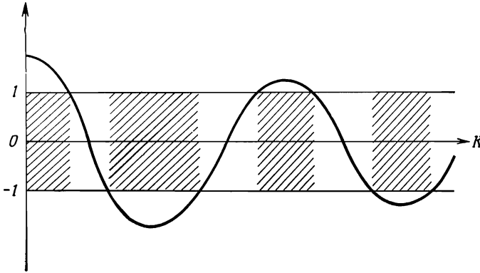
Фиг. 8.6. Характерный вид функции \cos(Ka + \delta)/|t| .
