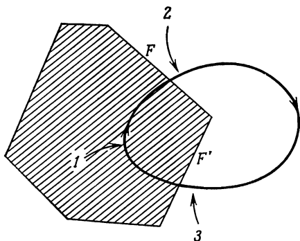
Фиг. 18.3. К рассмотрению работы выхода.
