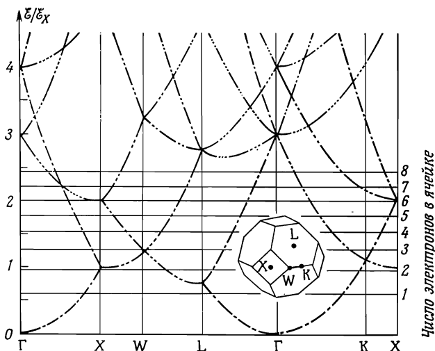
Фиг. 9.5. Энергетические уровни свободных электронов для г. ц. к. решетки Браве. (Из работы [2].)
