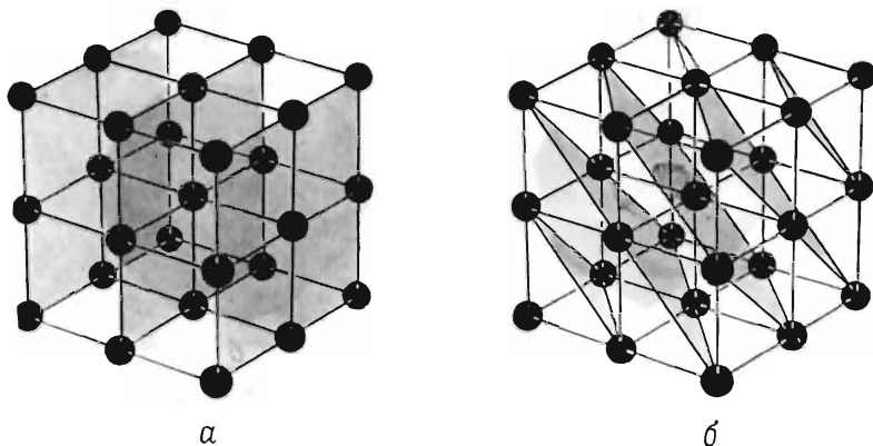
Фиг. 5.3. Некоторые атомные плоскости (темные) простой кубической решетки Бравэ. Показаны два различных способа (а и б) разбиения решетки на семейства атомных плоскостей.
