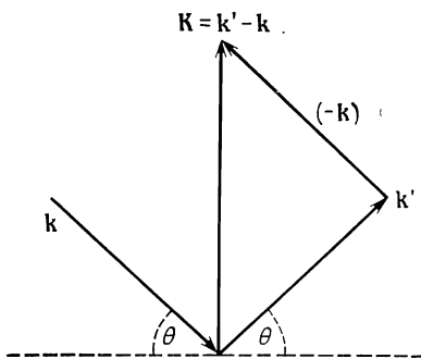
Фиг. 6.6. Волновой вектор \mathbf{k} падающего луча, волновой вектор \mathbf{k}' отраженного луча и вектор их разности \mathbf{K} = \mathbf{k}' - \mathbf{k} , удовлетворяющий условию Лауэ.
