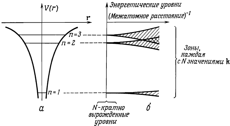
Фиг. 10.4. a — схематическое изображение невырожденных электронных уровней в атомном потенциале;
