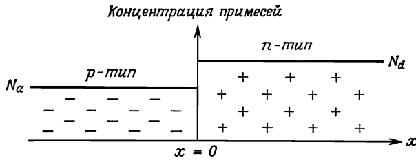
Фиг. 29.1. Распределение концентраций примесей вдоль p-n -перехода в случае «резкого перехода», в котором донорные примеси доминируют при положительных x , а акцепторные примеси — при отрицательных x .
