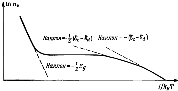
Фиг. 28.13. Температурная зависимость концентрации основных носителей тока (для случая N_d > N_a ).
