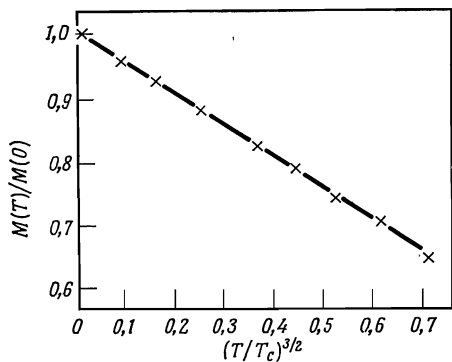
Фиг. 33.8. Зависимость отношения спонтанной намагниченности ферромагнитного гадолиния ( T_c = 293 К) при температуре T к намагниченности насыщения ( T = 0 ) от (T/T_c)^{3/2} . (Из работы [15].)
