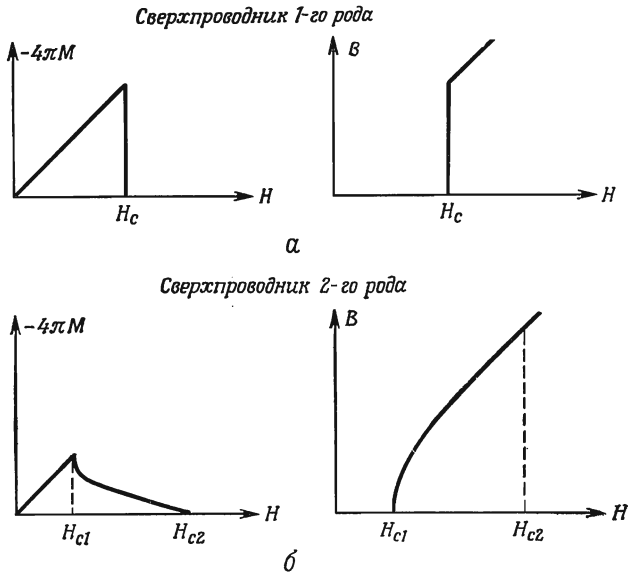
Фиг. 34.4. а — зависимость намагниченности от поля для сверхпроводника 1-го рода. Поле, меньшее H_c , не проникает в сверхпроводник, B = 0 (или M = -H/4\pi ) (см. примечание 1 на стр. 352 относительно различия между B и H в сверхпроводнике).
