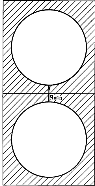
Фиг. 26.5. Схема расширенных зон для металла, поверхность Ферми которого целиком содержится в первой зоне Бриллюэна. Здесь q_{\min} — минимальный волновой вектор фонона, способного участвовать в процессе переброса. При температурах ниже той, которая отвечает энергии этого фонона, вклад процессов переброса должен падать по экспоненте.
