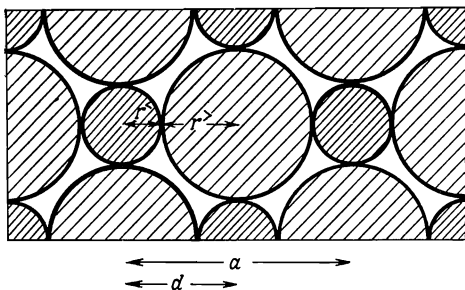
Фиг. 19.7. Плоскость (100) в структуре хлорида натрия, содержащая центры ионов. Каждый большой ион соприкасается лишь с соседними малыми ионами. Поэтому расстояние d между ближайшими соседями равно сумме ионных радиусов r^> + r^< . Это нормальная ситуация.
