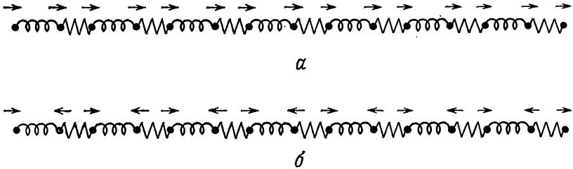
Фиг. 22.11. Длинноволновые акустическая (а) и оптическая (б) моды в двухатомной линейной цепочке.
