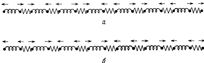
Фиг. 22.12. Акустическая (а) и оптическая (б) моды двухатомной линейной цепочки при k = \pm \pi/a , т. е. на краях зоны Бриллюэна.
