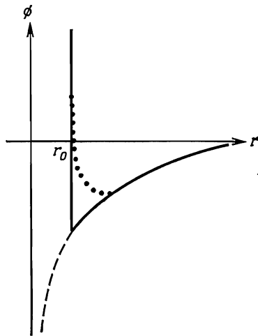
Фиг. 20.3. Пример парного потенциала.
