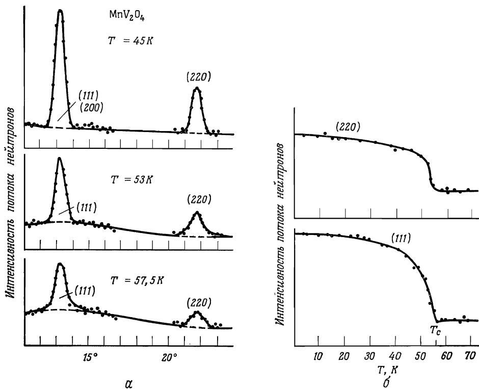
Фиг. 33.3. Результаты экспериментов по рассеянию нейтронов в антиферромагнетике. (Из работы [5].)
