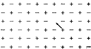
Фиг. 30.3. В идеальном кристалле движение положительного иона очень затруднено (а), однако при последовательном переходе положительного иона на соседние вакансии одиночный положительный заряд может сравнительно легко двигаться через кристалл (б — г).
