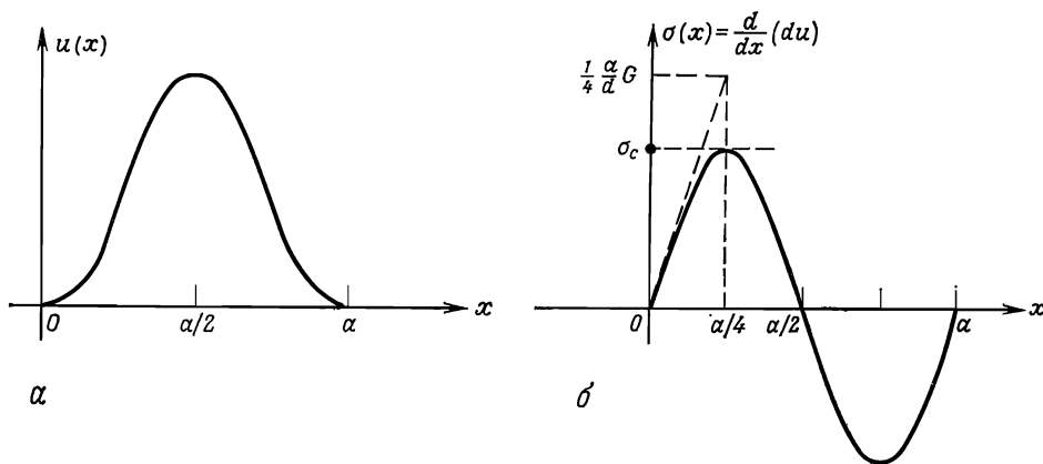
Фиг. 30.13. а — поведение дополнительной энергии (на единицу объема) u(x) , связанной со сдвиговой деформацией x .
