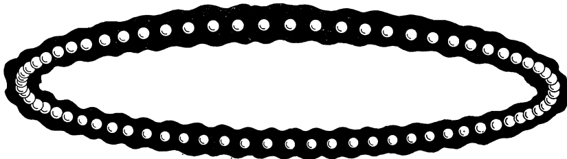
Фиг. 22.6. Граничное условие Борна — Кармана (или периодическое условие) для линейной цепочки.
