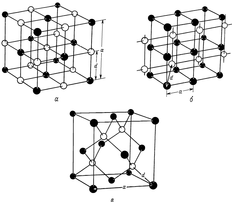
Фиг. 19.4. Структура хлорида натрия (а), хлорида цезия (б) и цинковой обманки (сфалерита) (в).
