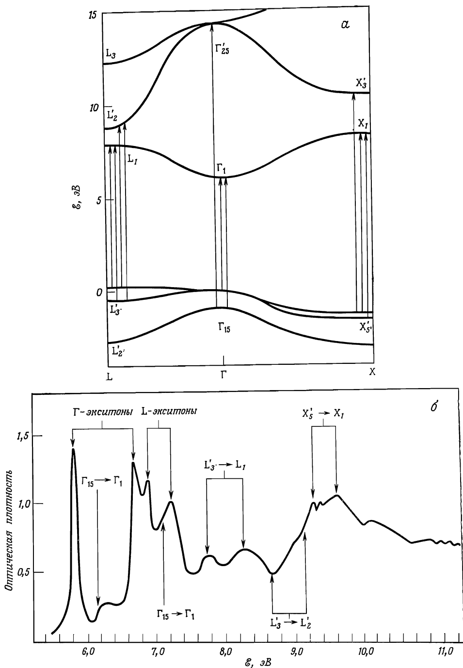
Фиг. 30.11. a — зонная структура KI, полученная Филлипсом [5] путем исследования оптического спектра поглощения этого вещества. б — спектр экситонных состояний, образовавшихся вблизи различных максимумов и минимумов валентной зоны и зоны проводимости (согласно результатам работы [6], приведенным в обзоре Филлипса [7]).
