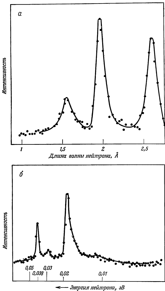
Фиг. 24.4. Типичные наблюдаемые в эксперименте группы нейтронов для меди (а) * и германия (б). (Из работ [2, 3].)
