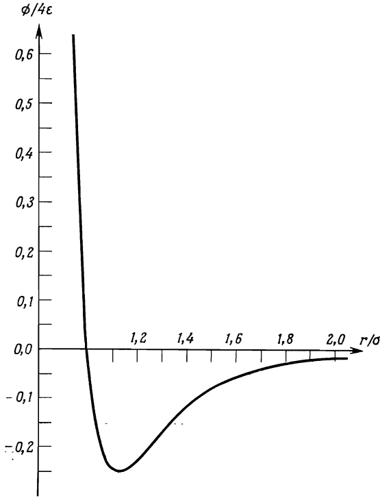
Фиг. 20.1. Потенциал «6—12» Леннарда-Джонса [формула (20.2)].
