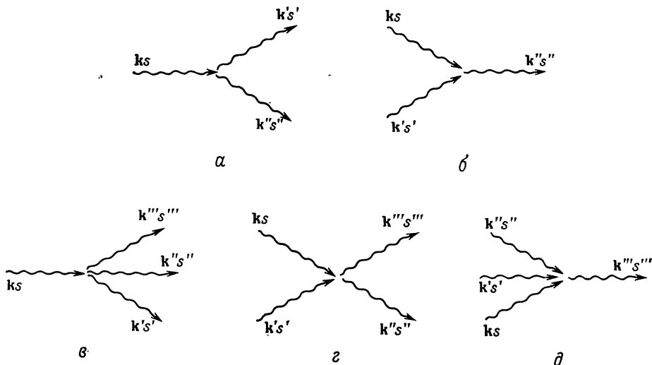
Фиг. 25.2. Процессы, отвечающие в низшем порядке теории возмущений анггармоническим членам третьего и четвертого порядка.
