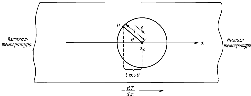
Фиг. 25.3. Перенос тепла фононами при наличии постоянного градиента температуры вдоль оси x .
