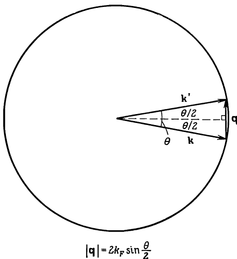
Фиг. 26.3. Рассеяние на малые углы на сферической поверхности Ферми.
