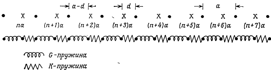
Фиг. 22.9. Двухатомная линейная цепочка одинаковых атомов, которые связаны пружинками с чередующейся жесткостью.
