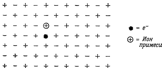
Фиг. 30.10. F_A -центр, в котором один из шести ближайших положительных ионов, окружающих вакансию в подрешетке отрицательных ионов, замещен примесным ионом.
