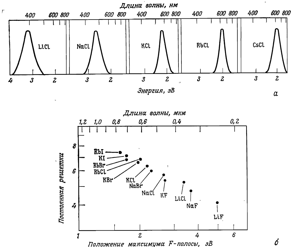
Фиг. 30.19. Полосы поглощения F -центров для некоторых хлоридов щелочных металлов (а) и зависимость положения максимума полосы поглощения F -центра от величины постоянной решетки (б). (Из работы [12].)
