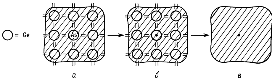
Фиг. 28.11. а — схематическое изображение донорной примеси (атом мышьяка с валентностью 5), замещающей в кристалле атом германия (валентность 4). б — атом мышьяка (As) можно представить как атом германия плюс добавочный единичный положительный заряд, закрепленный в узле решетки (точка в кружке). в — в полуклассическом приближении, в котором чистый полупроводник рассматривается как однородная среда, примесный атом мышьяка заменяется фиксированным точечным зарядом +e (точка).
