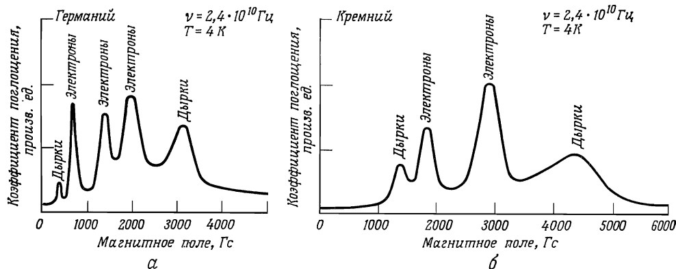
Фиг. 28.9. Типичные сигналы циклотронного резонанса в германии (а) и кремнии (б). (Из работы [6].)
