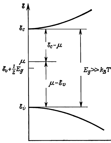
Фиг. 28.10. В собственном полупроводнике, у которого ширина запрещенной зоны E_g велика по сравнению с k_B T , химический потенциал \mu лежит в области шириной порядка k_B T вблизи середины запрещенной зоны, а следовательно, далеко (по сравнению с k_B T ) от обеих ее границ \mathcal{E}_c и \mathcal{E}_v .
