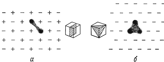
Фиг. 30.7. а — M -центр, в котором две соседние вакансии в подрешетке отрицательных ионов, находящиеся в плоскости (100), образуют связанное состояние двух электронов. б — R -центр, в котором три вакансии в подрешетке отрицательных ионов, находящиеся в плоскости (111), образуют связанное состояние трех электронов.
