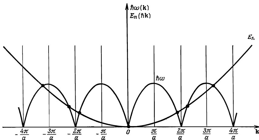
Фиг. 24.5. Одномерная иллюстрация того факта, что законы сохранения для однофононного поглощения могут всегда выполняться для падающих нейтронов с нулевой энергией.
