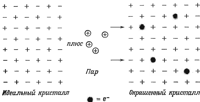
Фиг. 30.6. Возникновение дефектов в идеальном щелочно-галогидном кристалле при нагревании в атмосфере паров щелочного металла.
