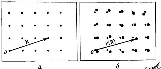
Фиг. 22.1. a — решетка Бравэ, точки которой задаются векторами \mathbf{R} . b — одно из мгновенных расположений ионов [ион, среднее положение которого есть \mathbf{R} , находится в точке \mathbf{r}(\mathbf{R}) ].
