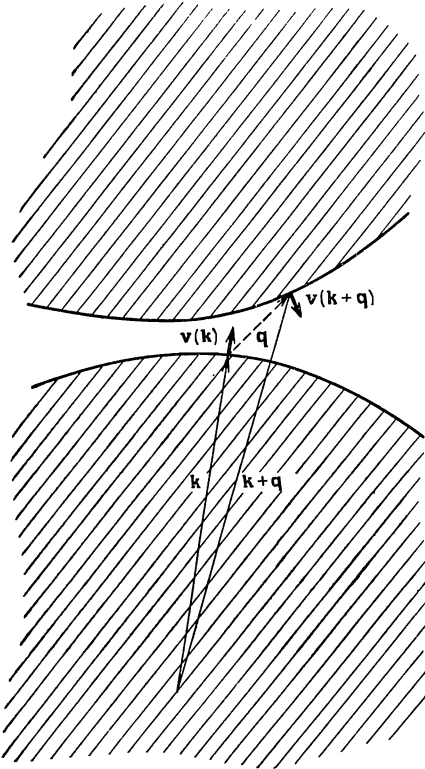
Фиг. 26.4. Простой процесс переброса. Волновые векторы \mathbf{k} и \mathbf{k} + \mathbf{q} отличаются на величину, малую по сравнению с k_F (или k_D ), но скорости \mathbf{v}(\mathbf{k}) и \mathbf{v}(\mathbf{k} + \mathbf{q}) не близки друг другу.
