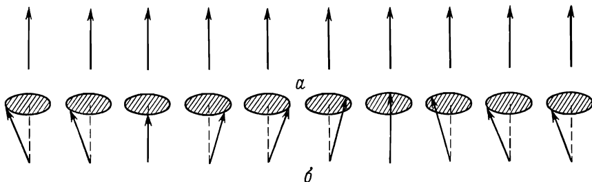
Фиг. 33.7. Схематическое представление цепочки спинов для ферромагнитного состояния (a) и состояния со спиновой волной (б).
