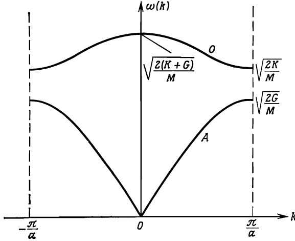
Фиг. 22.10. Закон дисперсии для двухатомной линейной цепочки.
