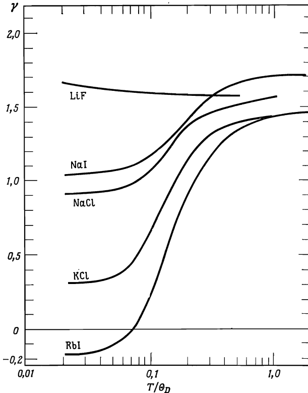
Фиг. 25.1. Зависимость параметра Грюнайзена от величины T/\Theta_D для некоторых щелочно-галогидных кристаллов. (Из работы [2].)
