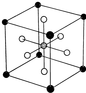
Фиг. 27.10. Структура перовскита, характерная для сегнетоэлектриков типа титаната бария ( \text{BaTiO}_3 ) в неполяризованной фазе.
