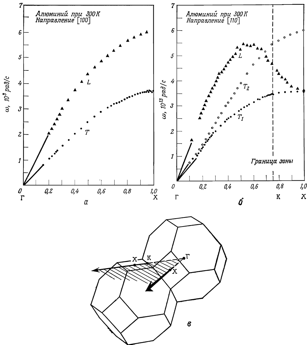
Фиг. 24.2. Определенный по рассеянию нейтронов фононный спектр алюминия вдоль линий ГХ и ГКХ в k -пространстве. (По работе [1].)
