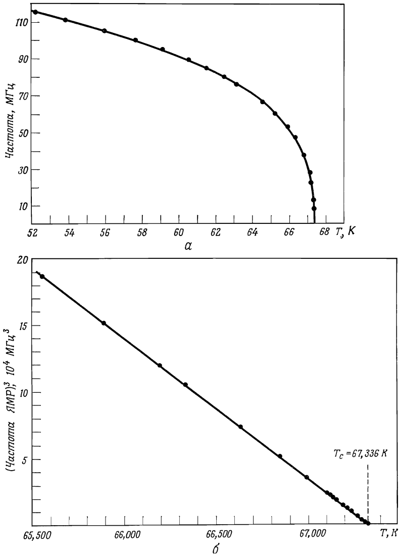
Фиг. 33.4. Результаты исследования антиферромагнетика методом ядерного магнитного резонанса.
