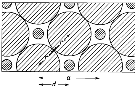
Фиг. 19.8. Та же плоскость, что и на фиг. 19.7, но теперь различие ионных радиусов очень велико и поэтому каждый большой ион касается лишь ближайшего большого иона.
