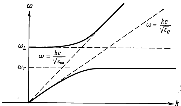
Фиг. 27.6. Решения дисперсионного уравнения \omega = kc/\sqrt{\varepsilon(\omega)} для поперечных электромагнитных мод, распространяющихся в двухатомном ионном кристалле.
