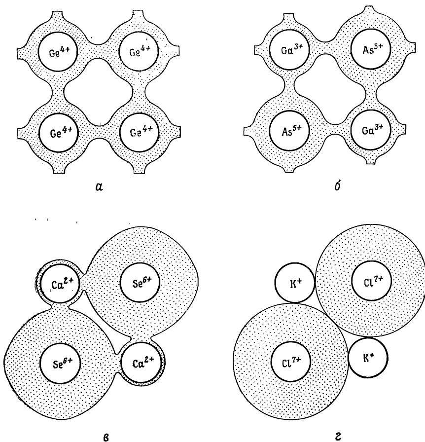
Фиг. 19.10. Сильно упрощенная картина непрерывного перехода от чисто ковалентных к чисто ионным кристаллам.
