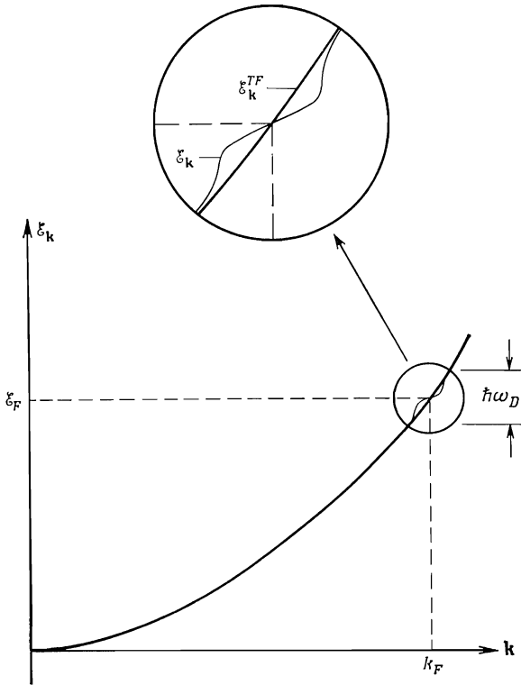
Фиг. 26.1. Поправка к зависимости \mathcal{E} от \mathbf{k} для электронов, учитывающая экранировку ионами (электрон-фононная поправка).
