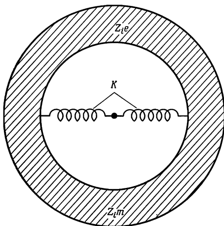
Фиг. 27.4. Грубая классическая модель, используемая при расчете атомной поляризуемости.
