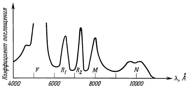
Фиг. 30.5. Пики в спектре поглощения KCl, обусловленные различными комбинациями F -центров, например самим F -центром, M -центром и R -центром. (Из работы [4].)
