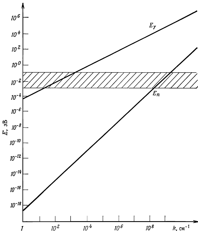
Фиг. 24.1. Соотношения между энергией и импульсом для нейтрона ( n ) и фотона ( \gamma ). При h = 10^n \text{ см}^{-1} эти энергии составляют E_n = 2,07 \cdot 10^{2n-19} эВ и E_\gamma = 1,97 \cdot 10^{n-5} эВ. Типичные тепловые энергии лежат в заштрихованной полосе или вблизи нее.
