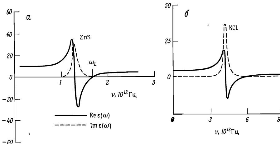
Фиг. 27.7. a — действительная (сплошная кривая) и мнимая (штриховая кривая) части диэлектрической проницаемости сульфида цинка. (Результат Абелеса и Матье [6], цитированный в работе [7].)
