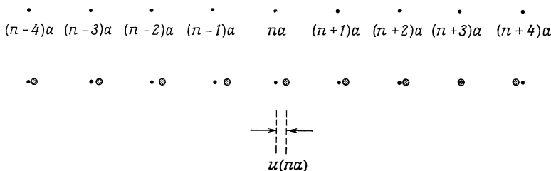
Фиг. 22.4. В произвольно выбранный момент времени ион, равновесное положение которого есть na , оказывается смещенным от этого положения на расстояние u(na) .
