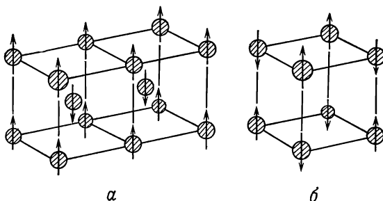
Фиг. 33.1. Некоторые простые антиферромагнитные структуры.
