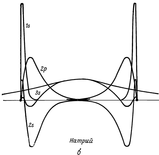
Фиг. 19.1. Рассчитанные радиальные волновые функции r\psi(r) для неона [1s^2 2s^2 2p^6] (а) и для натрия [1s^2 2s^2 2p^6 3s^1] (б). (Кривые построены по расчетам Д. Хартри и У. Хартри [1]). Волновые функции изображены для двух центров, расстояние между которыми взято равным наблюдаемому расстоянию между ближайшими соседями в твердом теле ( 3,1 \text{ \AA} в неоне, 3,7 \text{ \AA} в натрии). В неоне имеется очень слабое перекрытие 2s - и 2p -орбиталей. В натрии 2s - и 2p -орбитали перекрываются значительно меньше, но перекрытие 3s -волновых функций оказывается чрезвычайно сильным.
