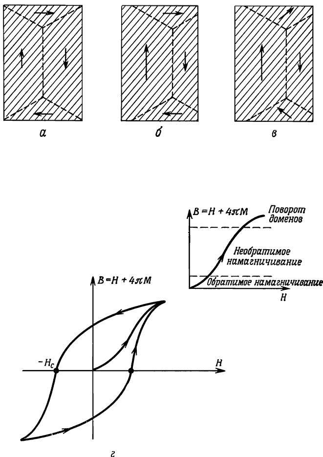
Фиг. 33.14. Процесс намагничивания.
