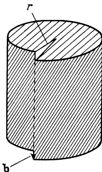
Фиг. 30.20. Винтовая дислокация с вектором Бюргерса \mathbf{b} .
