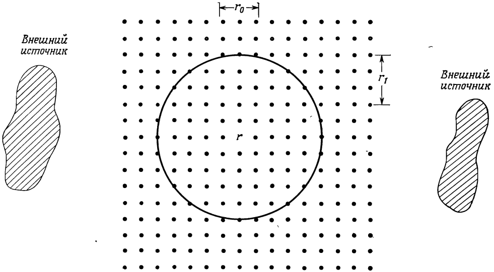
Фиг. 27.3. При расчете локального поля в точке \mathbf{r} удобно отдельно рассматривать вклад дальней области (к которой относится весь кристалл, за исключением сферы радиусом r_0 вокруг точки \mathbf{r} , а также внешние источники поля) и вклад ближней области (образованной всеми точками, лежащими внутри сферы с центром в \mathbf{r} ).
