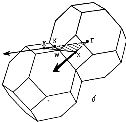
Фиг. 22.13. Типичные дисперсионные кривые (а) для частот нормальных мод в монокристаллической решетке Браве свинца, изображенные в схеме повторяющихся зон вдоль линий, являющихся сторонами заштрихованного треугольника (б). (По работе [2].)
