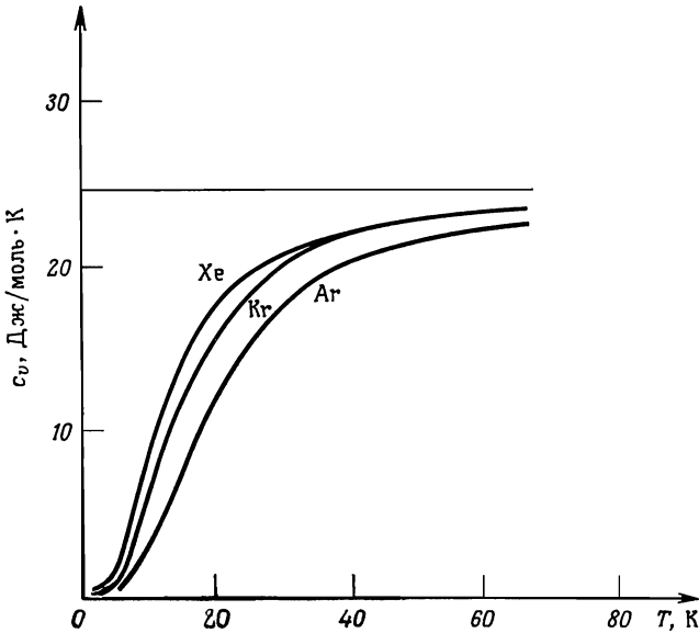
Фиг. 22.3. Измеренные удельные теплоемкости аргона, ксенона и криптона. (По работе [4]). Горизонтальная прямая — классический результат Дюлонга и Пти.
