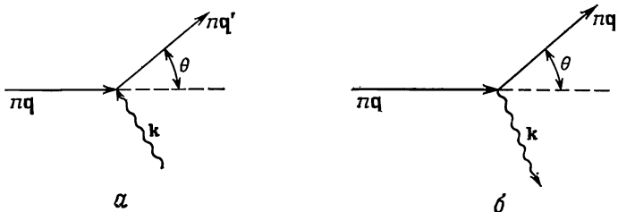
Фиг. 24.7. Рассеяние фотона на угол \theta , которое сопровождается поглощением фонона с волновым вектором \mathbf{k} (антистоксов процесс) (а) и испусканием фонона с волновым вектором \mathbf{k} (стоксов процесс) (б).
