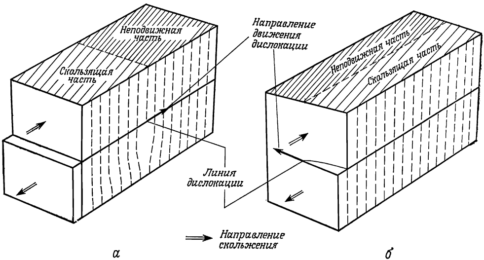
Фиг. 30.14. а — скольжение в кристалле, обусловленное движением краевой дислокации. б — скольжение в кристалле, обусловленное движением винтовой дислокации.
