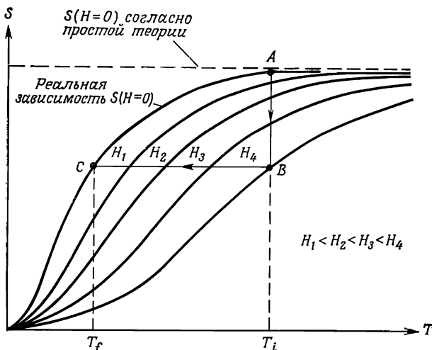
Фиг. 31.2. Температурная зависимость энтропии системы взаимодействующих спинов при различных значениях внешнего магнитного поля H .
