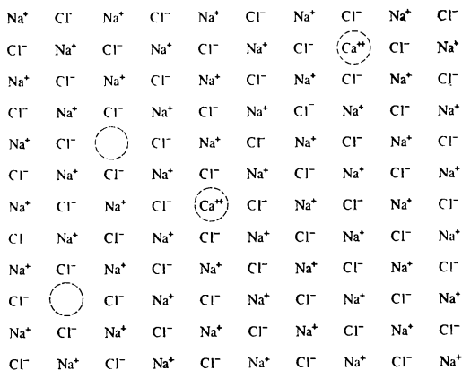
Фиг. 30.4. Внесение n ионов \text{Ca}^{++} в \text{NaCl} приводит к тому, что n ионов \text{Na}^+ замещаются ионами \text{Ca}^{++} ; при этом для сохранения электронейтральности образуются также n вакансий на местах ионов \text{Na}^+ .
