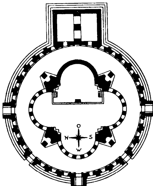
Չվարթնոց եկեղեցու հատակագիծը
