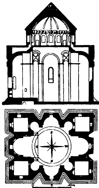
Հռիփսիմն եկեղեցին (ըստ Թ. Թորամանյանի)
