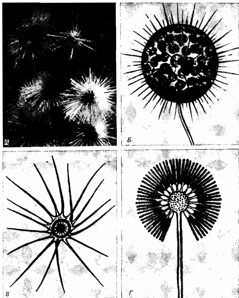
Рис. 12.16. Радиальная симметрия. А. Минерал: кристаллы водного мышьяково-кислого кальция — фармаколита (Medenbach, Sussiecke-Fornefeld, 1983). Б. Простейшее: солнечник Clathrulina elegans (Cabrera, 1936a). В. Растение: конидиеносец гриба Aspergillus niger (Hertwig, 1928). Г. Беспозвоночное: спермий рака (Guilliermond, Mangelot, 1941). Иллюстрация составлена автором.
