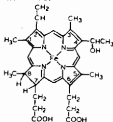
Рис. 11.1. Структурные формулы некоторых природных порфириновых производных (Margulis, 1981).
