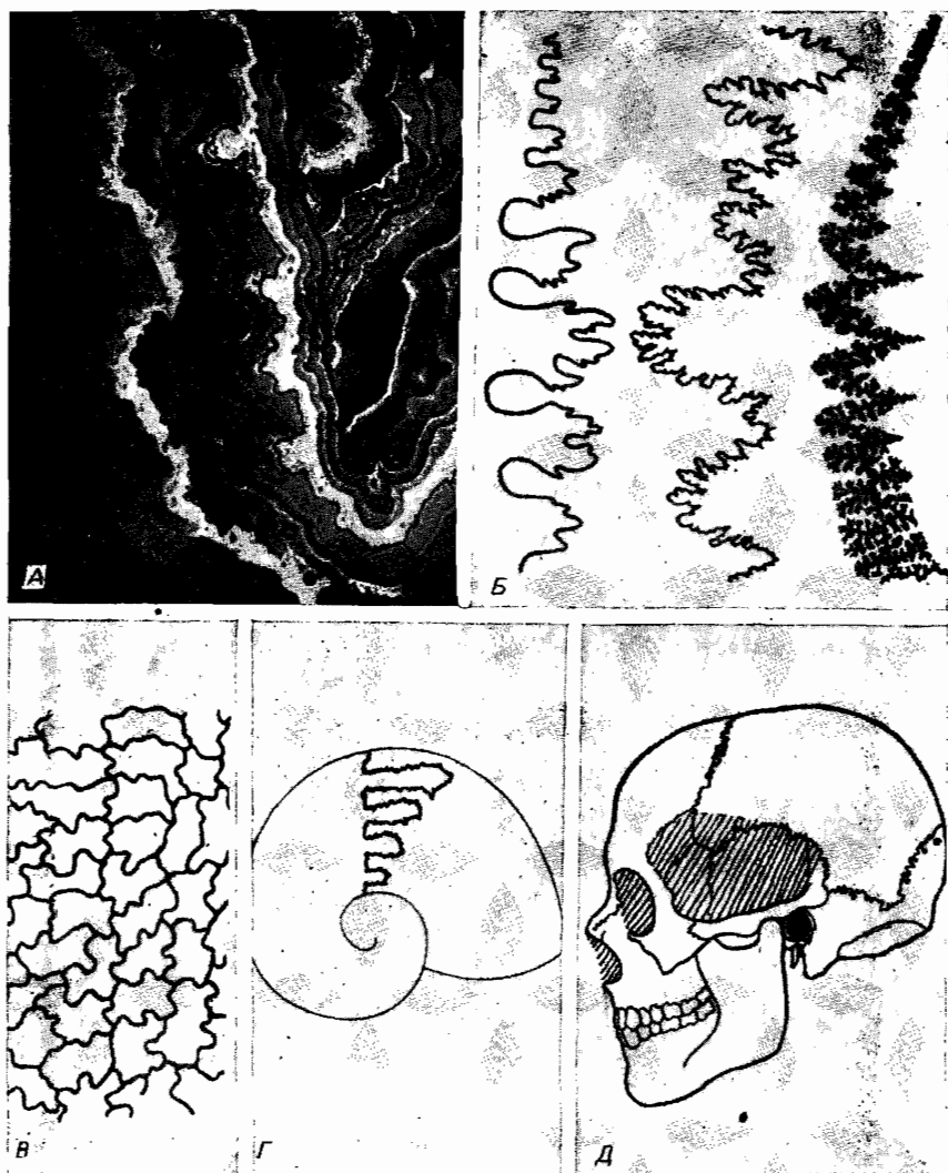
Рис. 9.18. Швы. А. Минерал: конкреция цинковой обманки — руды сульфида цинка, или сфалерита (Medenbach, Sussieck-Fornefeld, 1983). Б. Беспозвоночное: швы у аммонитов, имеющие разную величину зубцов (Shepherd, 1939). В. Растение: кутикула одного из видов Sagenopteris , папоротника юрского периода (Babin, 1980). Г. Беспозвоночное: у аммонитов, ископаемых головоногих, имеются швы различной степени сложности (Babin, 1980). Д. Позвоночное: швы в черепе Homo sapiens (Gregory, 1974). Иллюстрация составлена автором.
