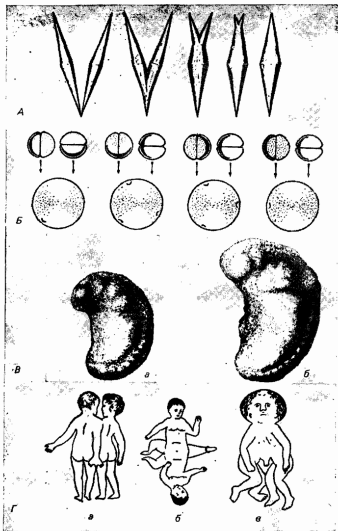
Рис. 10.5. Слияние кристаллов и слияние эмбрионов. А. Молекулярный процесс: слияние жидких кристаллов олеата аммония с образованием одного большого кристалла (Воннер, 1952, по Lehman). Б. Позвоночное: четыре способа слияния двух яиц тритона (на стадии двух клеток); показано положение blastopores в гастрюлах, образовавшихся из слившихся яиц (Weiss, 1939). В. Позвоночное: а — нормальный эмбрион Triton taeniatus ; б — крупный эмбрион, полученный путем слияния двух яиц (Weiss, 1939). Г. Позвоночное: три случая сросшихся близнецов человека. В случае в видна большая голова на сросшихся телах (Morgan, 1934, по Wilder).
