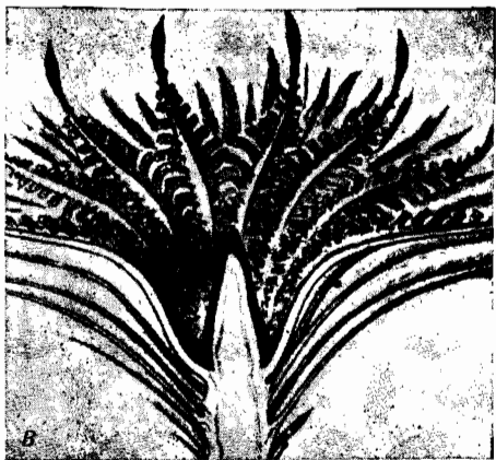
Рис. 9.14. Структуры, напоминающие цветок. А. Минерал: арагонит — карбонат кальция с большей плотностью, чем кальцит (Ehrhardt, 1939). Б. Беспозвоночное: актиния с ее «жалящими» щупальцами (Wheeler, 1940). В. Растение: продольный разрез цветка Cycadeoidea ingens (Strasburger, 1943). Г. Беспозвоночное: голотурия Cucumaria planci (Pierantoni, 1944). Иллюстрация составлена автором.
