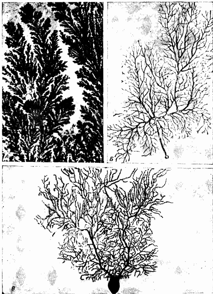
Рис. 10.7. Ветвистые структуры. А. Минерал: пиролюзит — черная окись марганца, — образующий ветвистые кристаллические дендриты в осадочных породах (Desautels, 1968). Б. Гриб: разветвленный мицелий (таллом), развивающийся из споры Mucor mucedo (Strasburger, 1924). В. Позвоночное: клетка Пуркинью из коры мозжечка (Costa, Chaves, 1937). Иллюстрация составлена автором.
