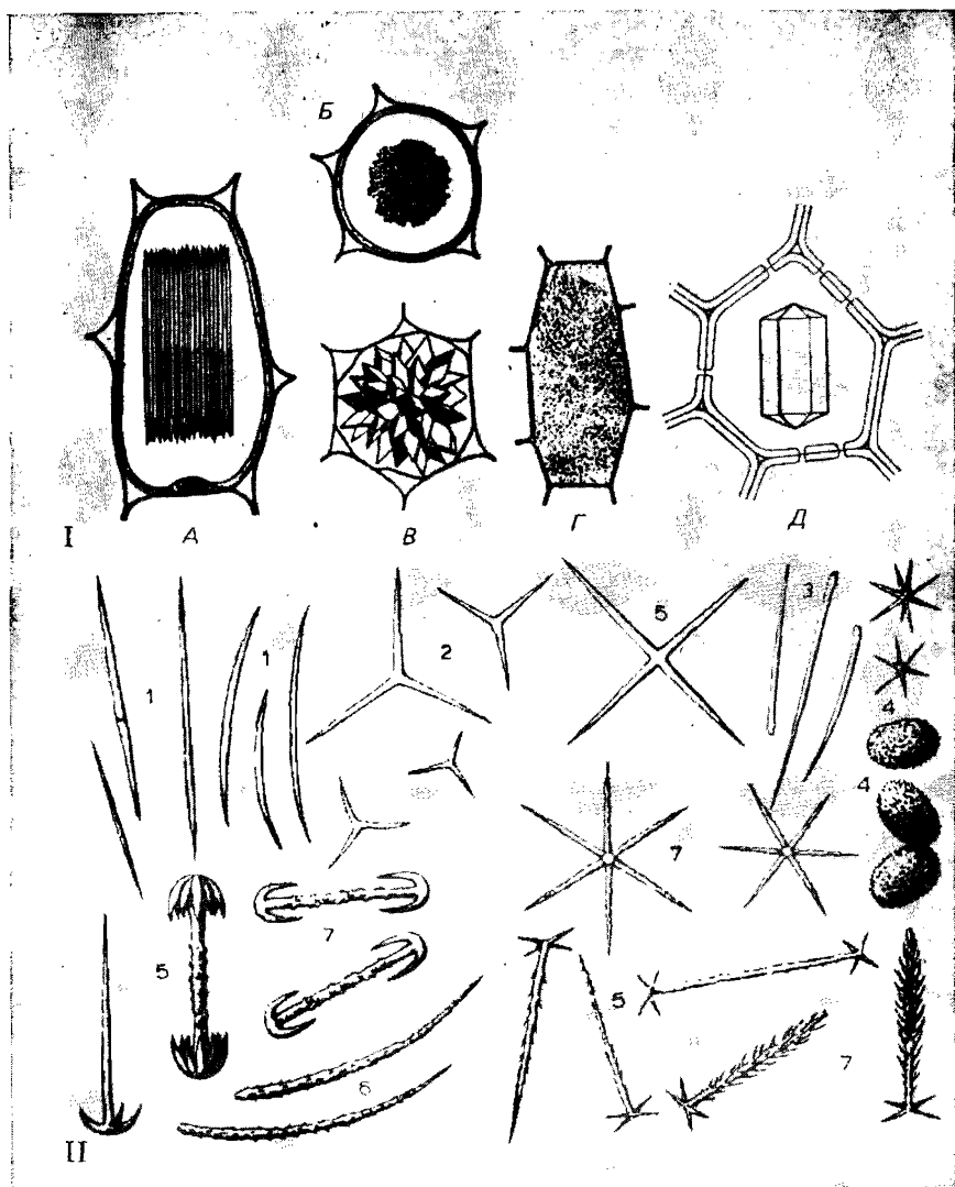
Рис. 9.6. Одно и то же химическое соединение принимает разные формы в разных клеточных средах. I. Моногидрат щавелевокислого кальция: различные формы кристаллов в клетках растений разных видов (Deniffer et al., 1971). А и Б — соответственно продольный и поперечный разрезы рафид в Impatiens ; В — друза в Opuntia ; Г — «кристаллический песок» в Solanum ; Д — тетрагональный кристалл дигидрата щавелевокислого кальция. II. Спиккулы губок (Sabrega, 1936a): 1 — кальцит, монорадиальные; 2 — кальцит, трирадиальные; 3—7 — кремнеземные спиккулы.
