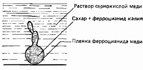
Рис. 10.14. А. Осмотическое набухание осадка ферроцианида меди (Leduc, 1911). Б. Осмотическое набухание капли раствора сахара и ферроцианида калия в растворе сернокислой меди. Образуется полупроницаемая пленка ферроцианида меди (Guilliermond, Mangelot, 1941).
