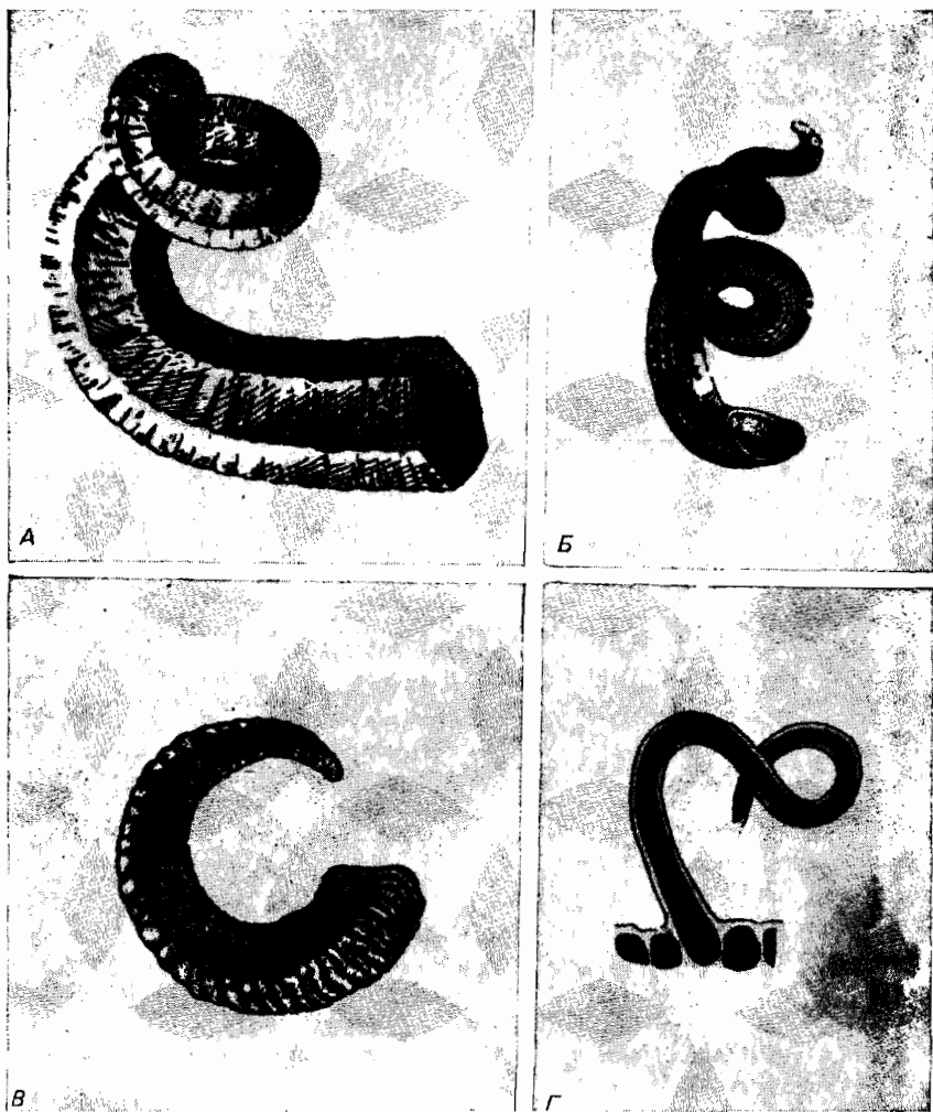
Рис. 9.21. Формирование роговидных структур. А. Минерал: изогнутые стопки кристаллов хлорита (Desautels, 1968). Б. Беспозвоночное: раковина моллюска Vermetus dentiferus (Hertwig, 1928). В. Позвоночное: рог дикого барана (муфлона) Ovis ammon (Reichholf, 1984). Г. Растение: одноклеточный волос Althaea rosea (сем. Malvaceae) (Coutinho, 1906). Иллюстрация составлена автором.
