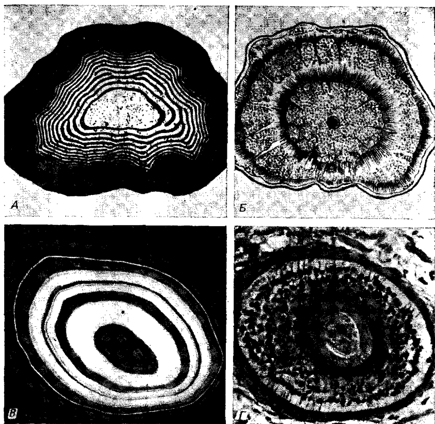
Рис. 9.12. Слоистые кольцевые структуры. А. Молекулярный процесс: кольца Лизеганга в смеси азотнокислого серебра и двухромовокислого калия в желатине (Rinne, 1928). Б. Растение: поперечный разрез стебля Mimosa altissima (сем. Papilionaceae) (Strasburger, 1943). В. Минерал: агат; растворенные минералы осаждаются слоями в тонкозернистом кварце (Desautels, 1968). Г. Позвоночное: поперечный разрез основания волоса в коже человека (Nachtigall, Kage, 1980). Иллюстрация составлена автором.
