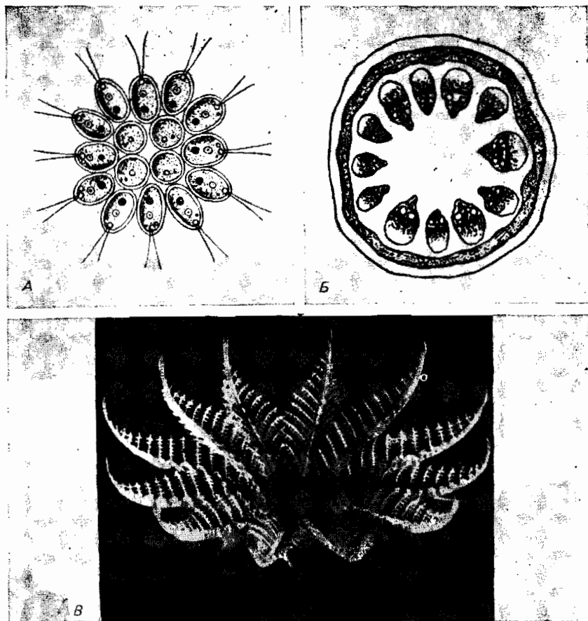
Рис. 12.11. Симметрия 12-го порядка. А. Простейшее: Gonium pectorale , вид сверху (Tieghem, Costantin, 1918). Б. Растение: Aristolochia sipho (сем. Aristolochiaceae), поперечный срез ветви (Strasburger, 1943). В. Растение: реконструкция цветка ископаемого растения Cycadoidea ingens (Cabrega, 1936b). Иллюстрация составлена автором.
