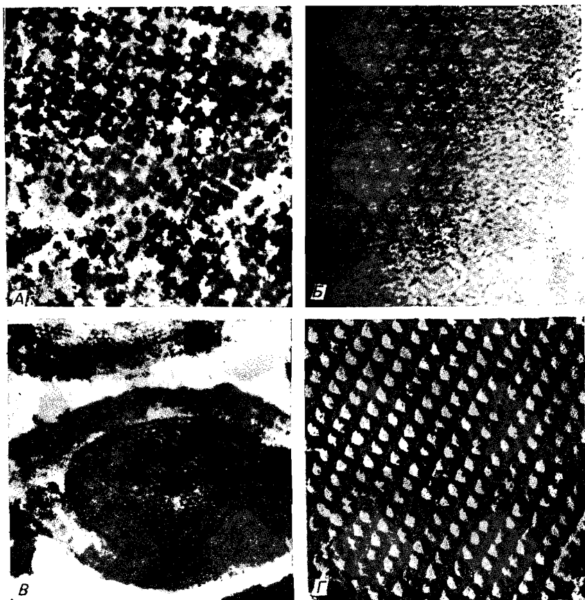
Рис. 9.5. Кристаллические формы клеточных органелл. А. Кристаллическая структура, образованная рибосомами в клетках курицы (Byers, 1967). Б. Кристалл из частиц сердцевины нуклеосом (Finch et al., 1977). В. Кристаллическая упаковка хромосом сперматиды насекомого Melanoplus (Gall, Bjork, 1958). Г. Правильная решетка из трансмембранных частиц в тилакоидных мембранах шпината (Stryer, 1981).
