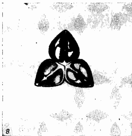
Рис. 12.2. Симметрия 3-го порядка. А. Минерал: кристалл тетраэдрита — сульфида меди и сурьмы, (\text{CuFe})_{12}(\text{SbAs})_4\text{S}_{13} (Medenbach, Sussieck-Fornefeld, 1983). Б. Минерал: кристалл борацита — природного борнокислого и хлористого магния (Medenbach, Sussieck-Fornefeld, 1983). В. Растение: плод Fumana procumbens (сем. Cistaceae) с тремя гнездами, содержащими семена (Heywood, 1978). Г. Беспозвоночное: передний конец нематоды (Barnes, 1980). Иллюстрация составлена автором.
