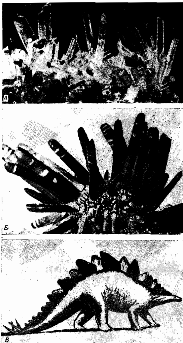
Рис. 9.23. Пластинчатые образования. А. Минерал: кристаллы гипса — селенита \text{CaSO}_4 \cdot 2\text{H}_2\text{O} (Cabrera, 1937). Б. Беспозвоночное: морской еж Heterocentrotus mamillatus , у которого иглы превратились в большие пластины (Cabrera, 1936a). В. Позвоночное: ископаемый ящер Stegosaurus с большими спинными пластинами и хвостовыми шипами (Colbert, 1980). Иллюстрация составлена автором.
