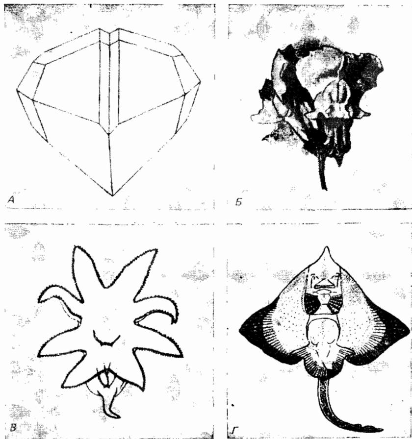
Рис. 12.1. Двусторонняя симметрия. А. Минерал: двойниковый кристалл кальцита \text{CaCO}_3 (ромбоэдрическая форма) (Саврега, 1937). Б. Растение: два цветка Antirrhinum majus , один изображен сбоку, другой — спереди (сем. Scrophulariaceae) (Бур, 1930). В. Беспозвоночное: глубоководный оболочник Ocyropsis ingolfi (Barnes, 1980). Г. Позвоночное: скат Raja alba (Luther, Fiedler, 1976). Иллюстрация составлена автором.
