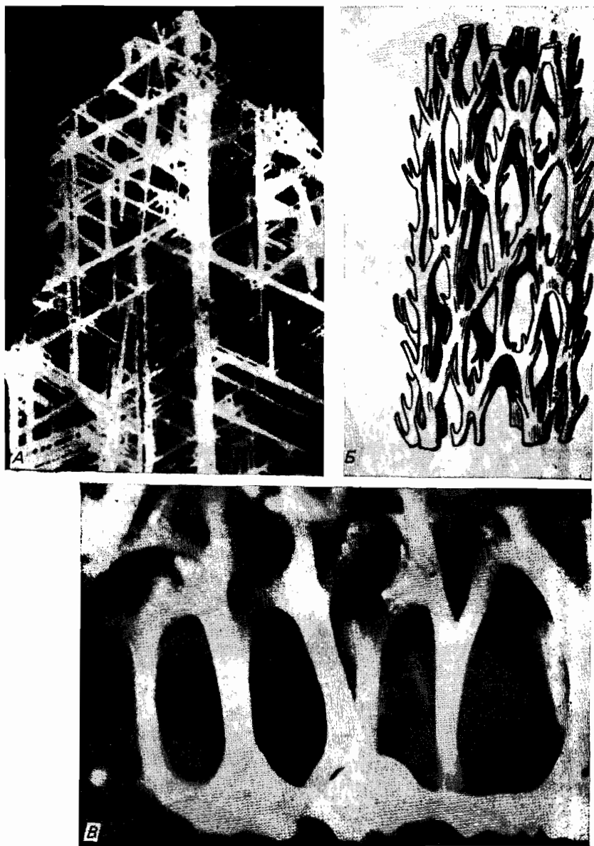
Рис. 10.17. Опорные структуры. А. Минерал: сетчатая структура церуссита \text{PbCO}_3 (Desautels, 1968). Б. Растение: сеть проводящих сосудов в стебле Aspidium filixmas (Strasburger, 1943). В. Беспозвоночное: скелет панциря мечехвоста (Feininger, 1956). Иллюстрация составлена автором.
