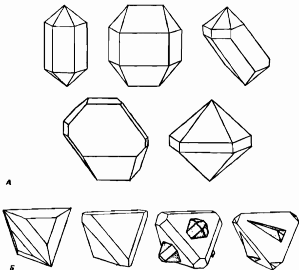
Рис. 8.4. Различные формы одного и того же минерала (Medenbach, Sussieck-Fornfeld, 1983). А. Пять разных кристаллов кварца \text{SiO}_2 . Углы между соответственными гранями всюду идентичны. Б. Четыре формы минерала тетраэдрита (\text{Cu, Fe})_{12}(\text{Sb, As})_4\text{S}_{13} ; на двух из них видны сrostки.
