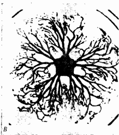
Рис. 9.9. Ветвящиеся фигуры, наблюдающиеся в ходе различных процессов и в разных биологических структурах. А. Физический процесс: электрический разряд (Feininger, 1956). Б. Растение: поперечный разрез молодого корешка (Denffer et al., 1971). В. Беспозвоночное: морская звезда Gorgonocephalus (Barnes, 1980). Г. Беспозвоночное: поперечный разрез щупальца Antedon (Pierantoni, 1944). Иллюстрация составлена автором.
