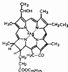
Хлорофилл а (фотосинтез у водорослей)
