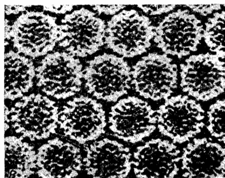
Рис. 9.3. Кристаллические формы вирусов. А. Октаэдрические кристаллы вируса желтой мозаики турнепса (Smith, Ritchie, 1980). Б. Кристаллы вируса кустистой карликовости томата (Luria, Darnell, 1967). В. Гексагональное расположение частиц вируса желтой мозаики вигны китайской (Horne, 1979).
