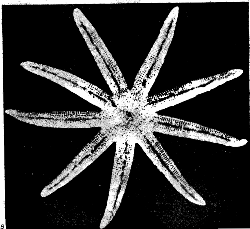
Рис. 12.8. Симметрия 9-го порядка. А. Растение: корень тыквы (сем. Cucurbitaceae) (Tieghem, Costantin, 1918). Б. Позвоночное: поперечный срез аксонемы жгутика (электронно-микроскопическая фотография); пару центральных одиночных микротрубочек окружают девять пар микротрубочек. Эта схема характерна для большинства жгутиков и ресничек эукариот (Stryer, 1981). В. Беспозвоночное: девятилучевая морская звезда (Stevens, 1981). Иллюстрация составлена автором.
