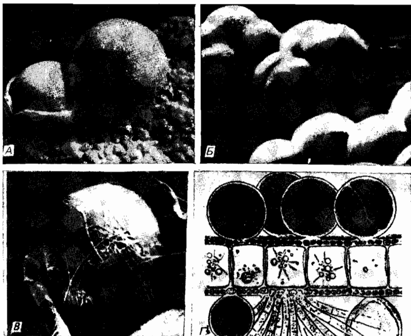
Рис. 3.7. Яйцевидные структуры. А. Минерал: глобулярные агрегаты фишериита \text{Al}_3(\text{OH})_3(\text{PO}_4)_2 \cdot 5\text{H}_2\text{O} (Medenbach, Sussieck-Fornefeld, 1983). Б. Бактерия: клетки Micrococcus radiodurans (микрофотография, полученная с помощью сканирующего электронного микроскопа; Margulis, Schwartz, 1982). В. Позвоночное: жировая клетка (микрофотография, полученная с помощью сканирующего электронного микроскопа; Strayer, 1981). Г. Растение: срез таллома водоросли Dictyota dichotoma с тетраспорангиями (Denffer et al., 1971). Иллюстрация составлена автором.
