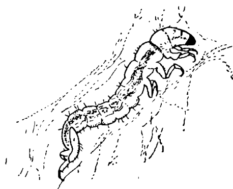
Рис. 9.20. А. Попад в кормовое пятно, личинка Plectrocnemia conspersa пятого возраста, которая встречает и съедает хирономиду, тотчас же прекращает поиск и начинает постройку ловчей сети. Хищники, которые не встретили жертву в течение 30 мин эксперимента, ведут более активный поиск, поэтому с большей вероятностью покинут пятно.
