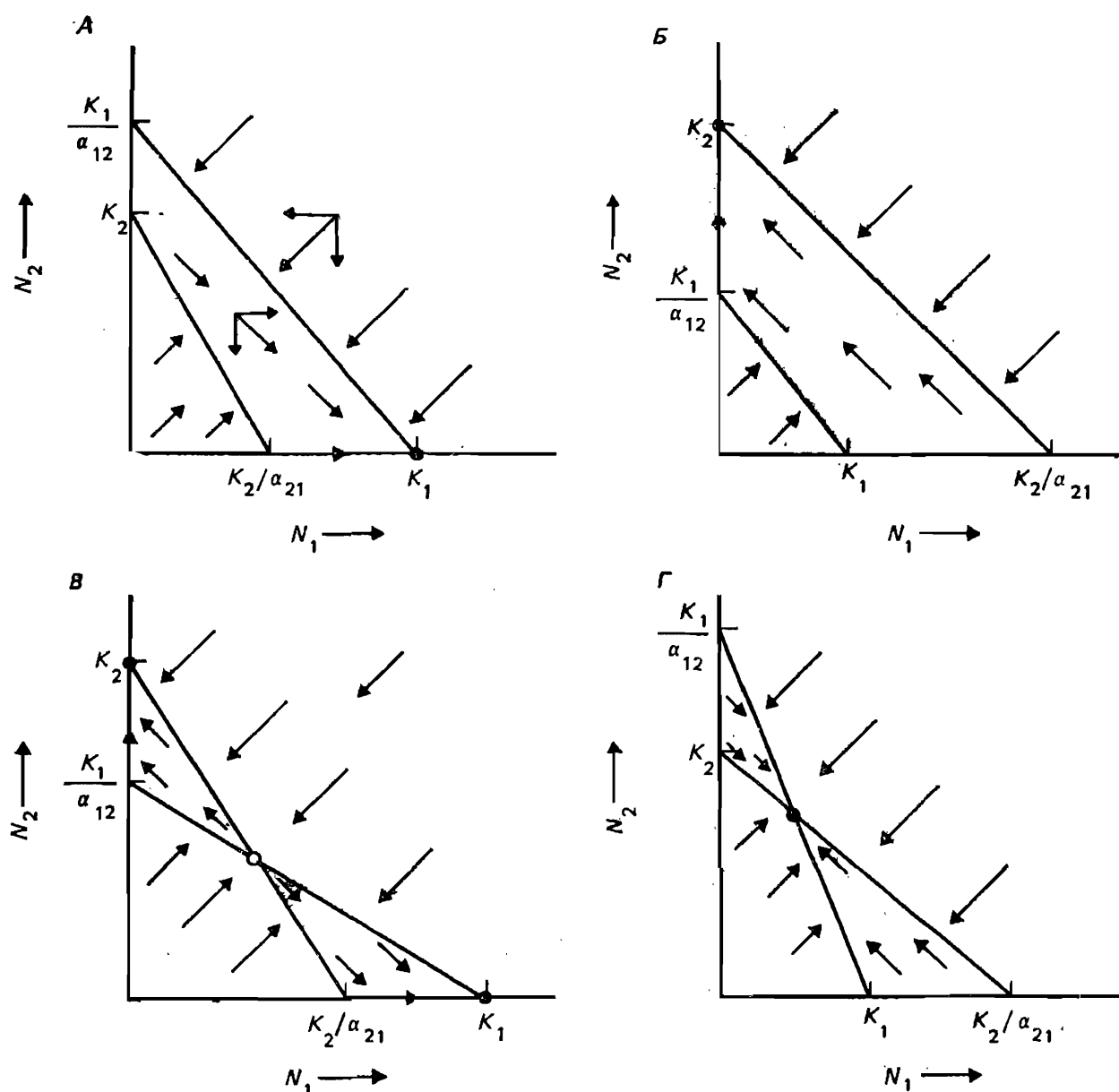
Рис. 7.8. Результаты конкуренции, полученные с помощью уравнений Лотки—Вольтерры для четырех возможных вариантов расположения изоклины для N_1 и N_2 . Векторы в большинстве случаев относятся к общей численности популяций и получены, как показано на рис. А. Черными кружками показаны точки устойчивого равновесия. Белый кружок на рис. В — точка неустойчивого равновесия. Более подробное обсуждение см. в тексте.
