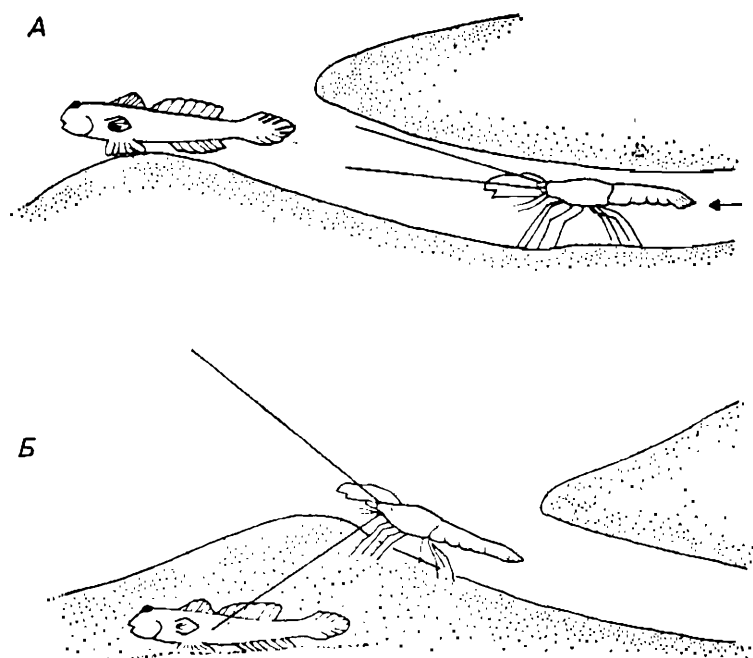
Рис. 13.2. Последовательность поведенческих актов в процессе выхода из норы при мутуализме креветки Alpheus djiboutensis и рыбы Cryptocentrus cryptocentrus . А. Креветка движется головой вперед к выходу из норы; антенны несколько приподняты и раздвинуты, так что их кончики отстоят друг от друга на 2—3 см. Б. Вне норы креветка одной антенной касается рыбы. (По Kag-plus et al., 1972.)
