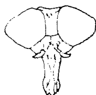
Слепень Tabanus atratus (отряд двукрылых) Кровосос. Мандибулы и максиллы уплощены
