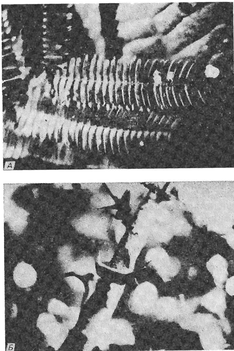
Фото 12. Отдельные структуры акации Acacia cornigera , которые привлекают муравьев-мутуалистов. А. Богатые белком тельца Белта на кончиках листьев. Б. Полые шипы, используемые муравьями для устройства гнезд. (Фотографии Gilbert.)
