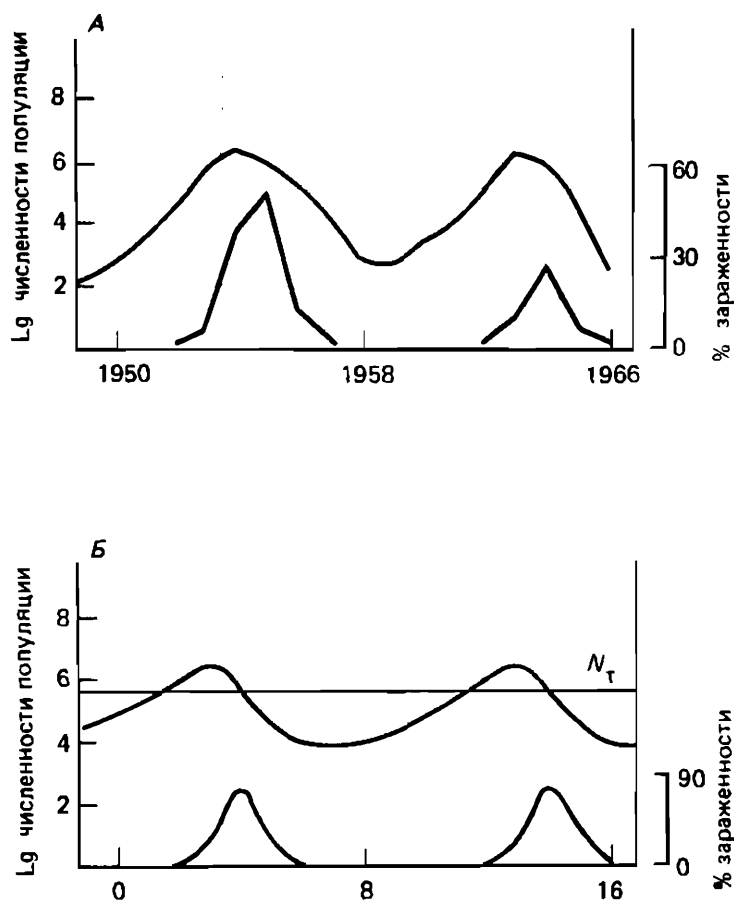
Рис. 12.25. А. Наблюдавшиеся изменения численности листовенничной моли Zeiraphera diniana в европейских Альпах (масштаб логарифмический) и распространение грануловирuсов (масштаб линейный, проценты). Б. Результаты, полученные на теоретической модели. (По Anderson, May, 1980.)
