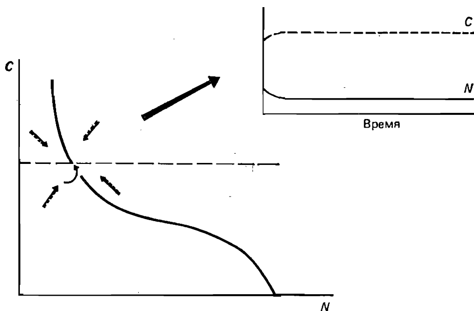
Рис. 10.10. Если функциональный ответ типа 3 возникает вследствие переключения хищника на другую жертву, то численность хищника может не зависеть от плотности жертвы любого типа ( основной рисунок ) и изоклина хищника может представлять собой горизонтальную линию (не изменяется в зависимости от плотности жертвы). Такая зависимость приводит к устойчивой динамике численности ( вверху справа ), когда плотность жертвы гораздо ниже предельной плотности насыщения
