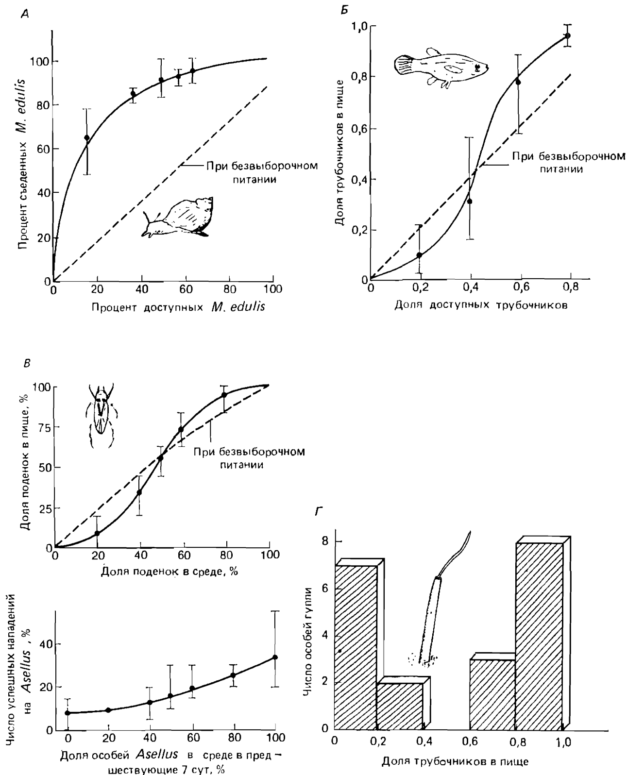
Рис. 9.2. Переключение. А. Отсутствие переключения: хищные моллюски, питаясь двусторчатыми моллюсками Mytilus edulis и M. californianus , проявляют постоянное предпочтение независимо от относительного обилия жертвы (среднее \pm стандартная ошибка). (По Murdoch, Oaten, 1975.) Б. Переключение у гуппи, питающихся червями-трубочниками и плодовыми мухами: рыбы поедают непропорционально большое количество той жертвы, которая более доступна (средние величины и крайние значения). (По Murdoch, Oaten, 1975.) В. Переключение у Notonecta , питающихся личинками поденок и раками Asellus (верхний рисунок). Причина переключения (нижний рисунок): Notonecta тем успешнее нападает на Asellus , чем больший опыт охоты на них она имеет (средние величины и крайние значения). (По Lawton et al., 1974.) Г. Предпочтение, проявляемое особями гуппи (на рис. Б), при равном количестве двух типов жертвы: отдельные рыбы в основном специализировались на одном из типов жертвы.
