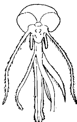
Комар Culex (отряд двукрылых) Ротовой аппарат колюще-сосущего типа
