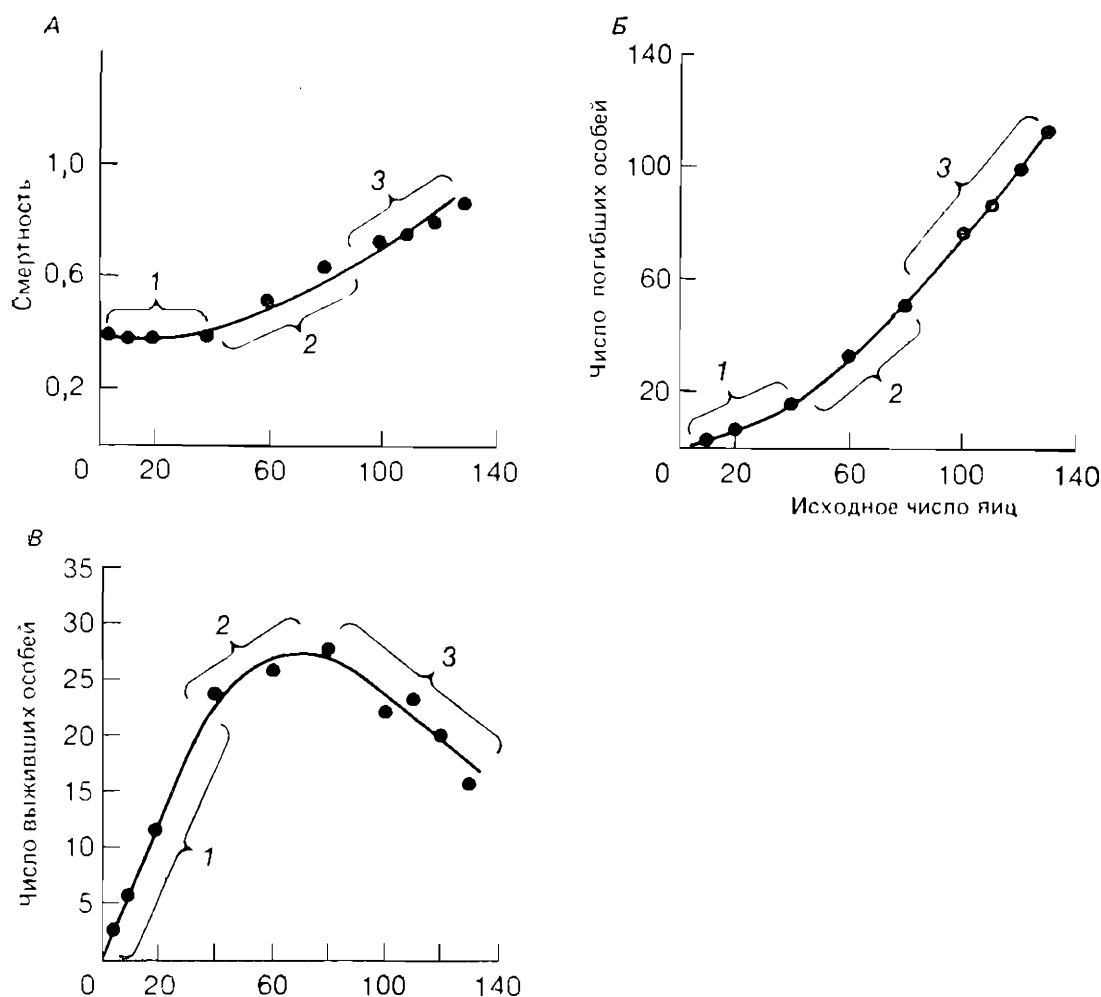
Рис. 6.1. Зависимость от плотности смертность в популяции малого мучного хрущака Tribolium confusum . А. Влияние плотности на смертность. Б. Влияние плотности на число погибших особей. В. Влияние плотности на число выживших особей. На участке 1 смертность не зависит от плотности; на участке 2 смертность не полностью компенсирует возрастание плотности; на участке 3 имеет место «сверхкомпенсация». (По Bellows, 1981.) (По оси абсцисс во всех случаях отложено исходное число яиц.)
