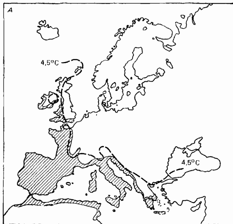
Рис. 2.16. А. Северная граница ареала марены чужеземной ( Rubia peregrina ) почти совпадает с январской изотермой 4,5^{\circ}\text{C} . (По Cox et al., 1976.) Б. Южная граница распространения морского желудя Balanus balanoides очень близка к изолинии минимального значения зимней температуры поверхностных вод, равного 8^{\circ}\text{C} . (По Barnes, 1957.)
