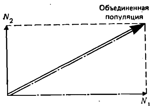
Рис. 7.7. Сложение векторов. Если численность видов 1 и 2 увеличивается, как показано векторам N_1 и N_2 , то возрастание численности объединенной популяции задается вектором, который представляет собой диагональ прямоугольника, образованного векторами N_1 и N_2 .
