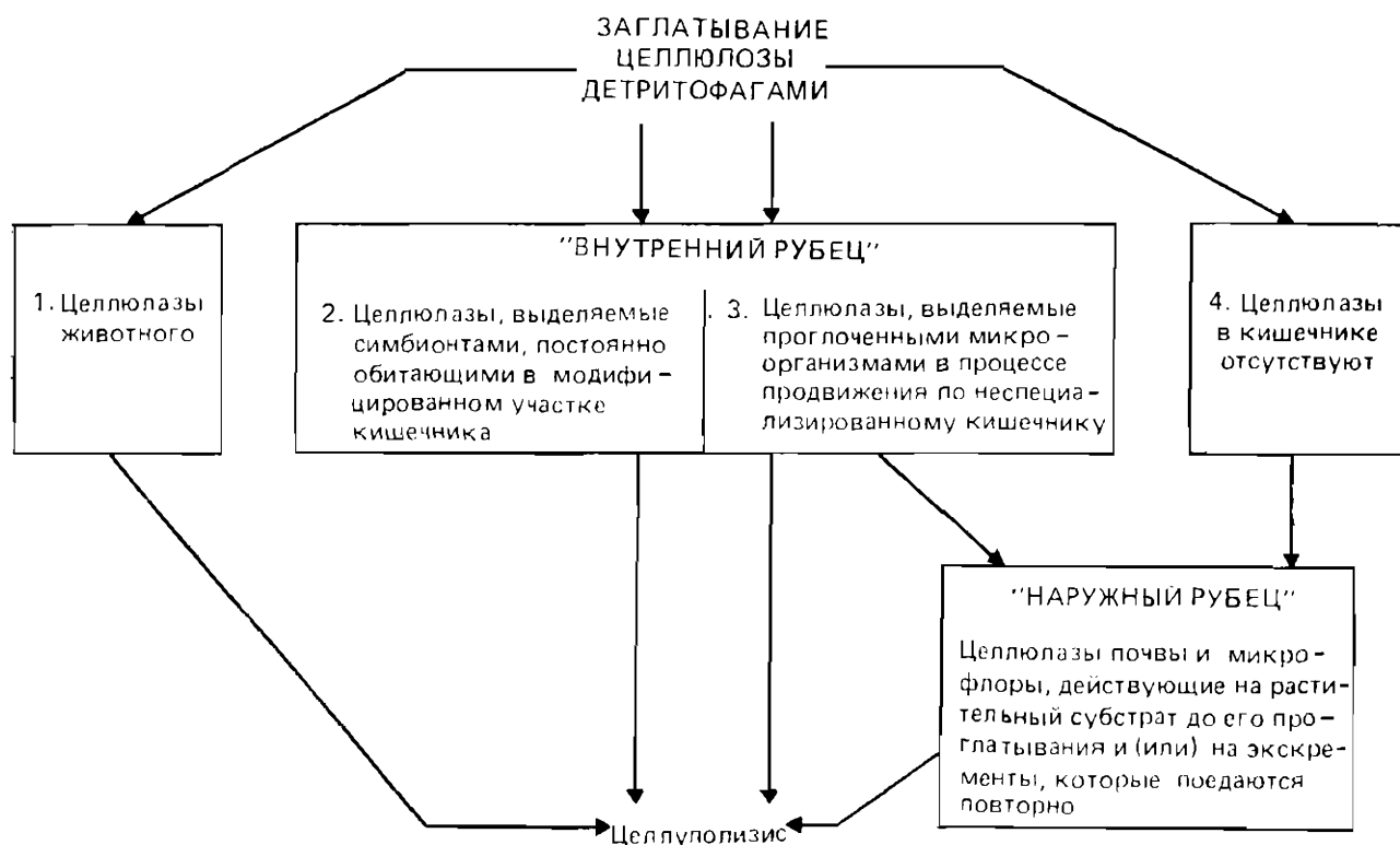
Рис. 11.13. Разнообразные механизмы для переваривания целлюлозы (целлюлолизис), выявленные у детритофагов. (По Swift et al., 1979.)
