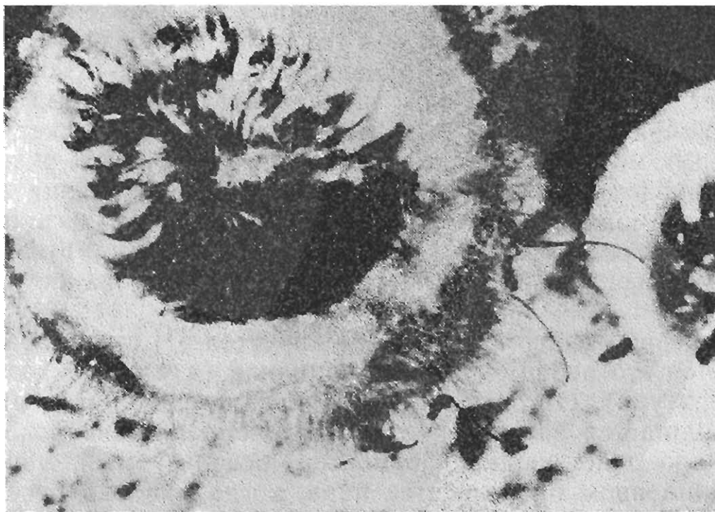
Фото 15. Осы blastofagi скапливаются на раскрытых соцветиях инжира и в них. Видны также паразитоиды (их можно узнать по длинным яйцекладам), которые поражают blastofaga. (Фотография W. D. Hamilton.)
