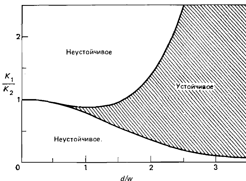
Рис. 7.10. Область благоприятных условий среды (обозначена величинами предельной плотности насыщения K_1 и K_2 , где K_1=K_3 , при которой возможно существование равновесного сообщества из трех видов с разной степенью перекрытия ниш ( d/w ). (По Мау, 1973.)
