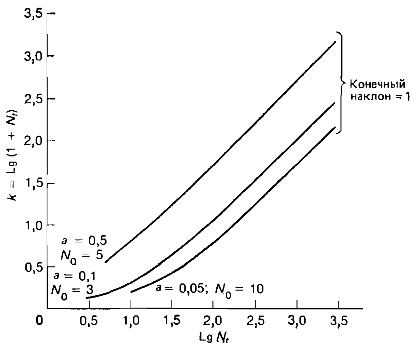
Рис. 6.20. Внутривидовая коикуренция, выраженная уравнением 6.3. Независимо от начальной плотности N_0 или константы a = (R-1)/K наклон линии, связывающей k с \lg N_t , становится равным 1 (точная компенсация)
