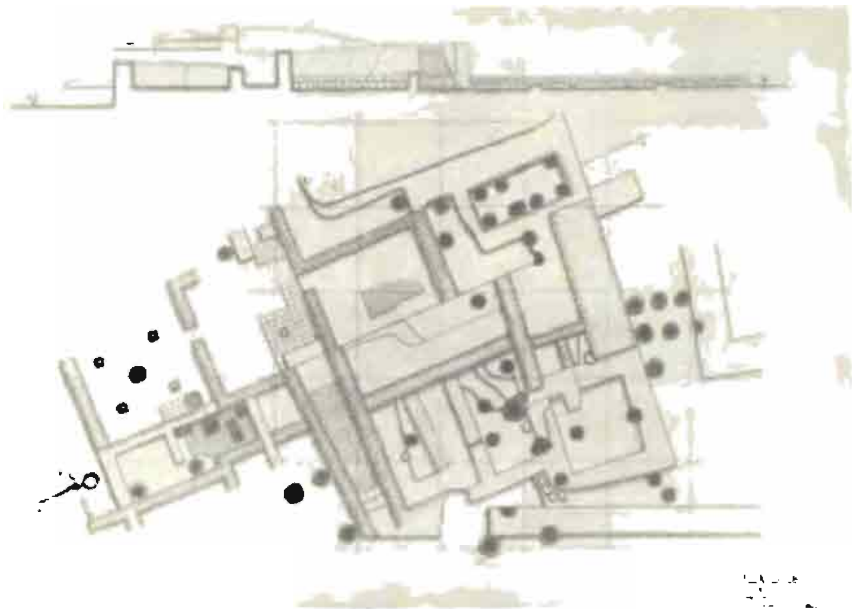
77 Միջնաբերդի հս ամ ծայրամասի վերին շերտի բնակելի չենքի հատակաձևը:
