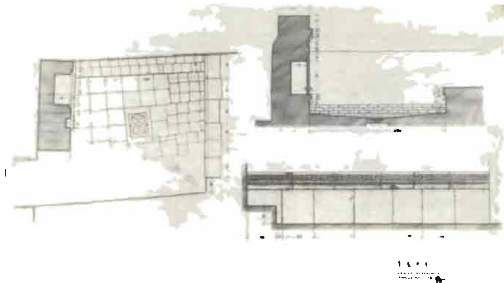
83. Ստորին բերդում պեղված բնակելի տան խորշավոր սենյակի հատակածը և կտրվածքները:
