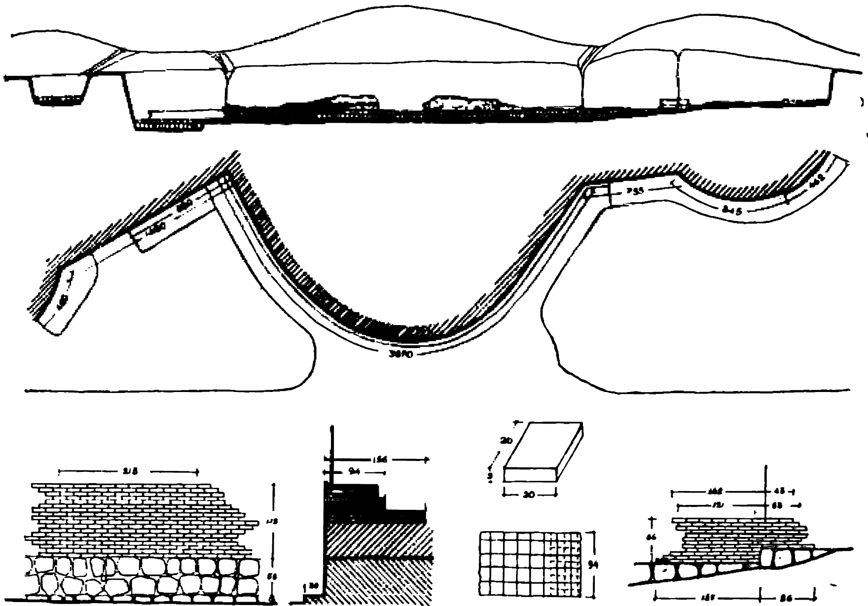
Ճ1. Միջնաբերդի հր-աւ բերդապարսպի բուրդերի հատակաձևերը (1963 թ.):
