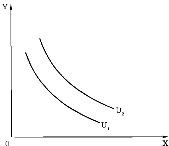
Рис. 4—21. Относительная взаимозаменяемость
