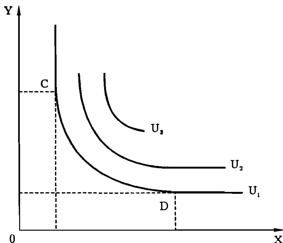
Рис. 4—19. Относительная взаимодополняемость
