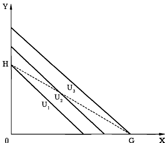
Рис. 4—20. Совершенная взаимозаменяемость
