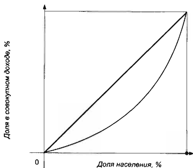
Рис. 16.1. Кривая Лоренца
