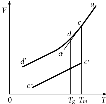
Նկ. 218. Նմուշի ծավալի կախումը ջերմաստիճանից. acc'' կորը համապատասխանում է հեղուկի բյուրեղացմանը, acd' կորը՝ ապակիացմանը:
