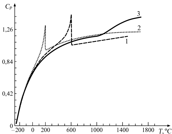
Նկ. 217. Բյուրեղային քվարցի տարատեսակների ջերմունակությունների ջերմաստիճանային կախման կորերը. քրիստոբալիտ (1), տրիդիմիտ (2), ամորֆ \text{SiO}_2 (3) ( C_p -ն չափված է կՋ/կգ· ^{\circ}\text{C} միավորով):
