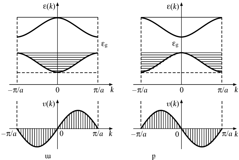
Նկ. 121. Լրիվ լրացված էներգիական գոտին և էլեկտրոնի արագությունը (ա. գույգ գոտի, բ. կենտ գոտի)
