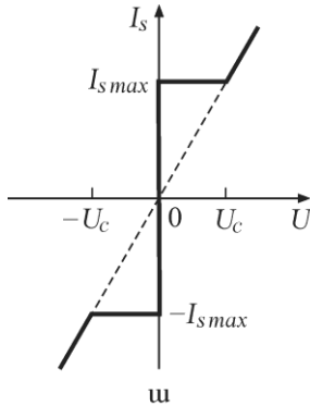
Նկ. 193. ա. Թույլ կապի վոլտ-ամպերային բնութագիծը, բ. հոսանքի աղբյուրն ապահովում է n_1 = \text{const} և n_2 = \text{const} պայմանների իրականացումը:
