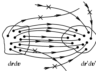
Նկ. 100. Բախումների հետևանքով d\mathbf{v} տիրությունը լրող (1-ով նշված գծեր) և d\mathbf{v} տիրությից մտնող (2-ով նշված գծեր) էլեկտրոններ (բախումները նշված են \times -ով):
