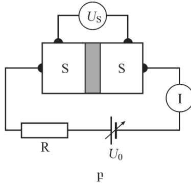
Նկ. 193. ա. Թույլ կապի վոլտ-ամպերային բնութագիծը, բ. հոսանքի աղբյուրն ապահովում է n_1 = \text{const} և n_2 = \text{const} պայմանների իրականացումը:
