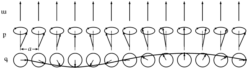
Նկ. 151. Ֆեռմոնագնիսի \omega հիմնական վիճակը, p գրգռված վիճակը (սպինային ալիքի առաջացումը), q սպինային ալիքը գծային շղթայում. ալիքը պատկերված է սպինային վեկտորների ծայրերով անցնող կորագծով:
