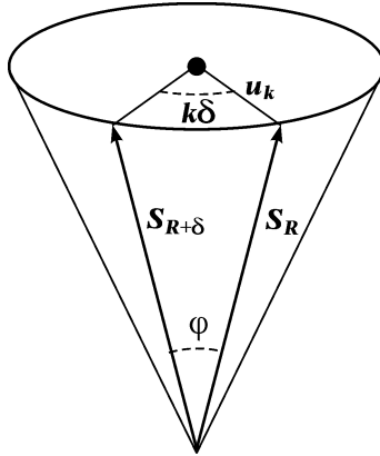
Նկ. 152. Սպինային ալիքում սպինի վեկտորի հաջորդական դիրքերը
