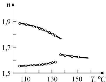
Նկ. 220. n -ազդակահանիզողի բեկման ցուցիչները
