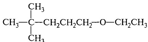
1-этоксн-4,4-днметнлпнтан
