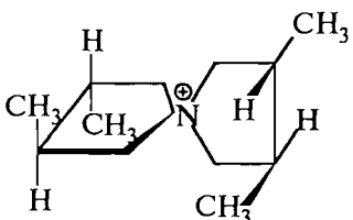
VIII ( S_4 )
