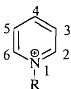
катион пиридиния
