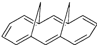
син -1,6-8,13-бисметано[14]-аннулен
