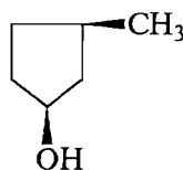
цис-3-метилциклопентанол
