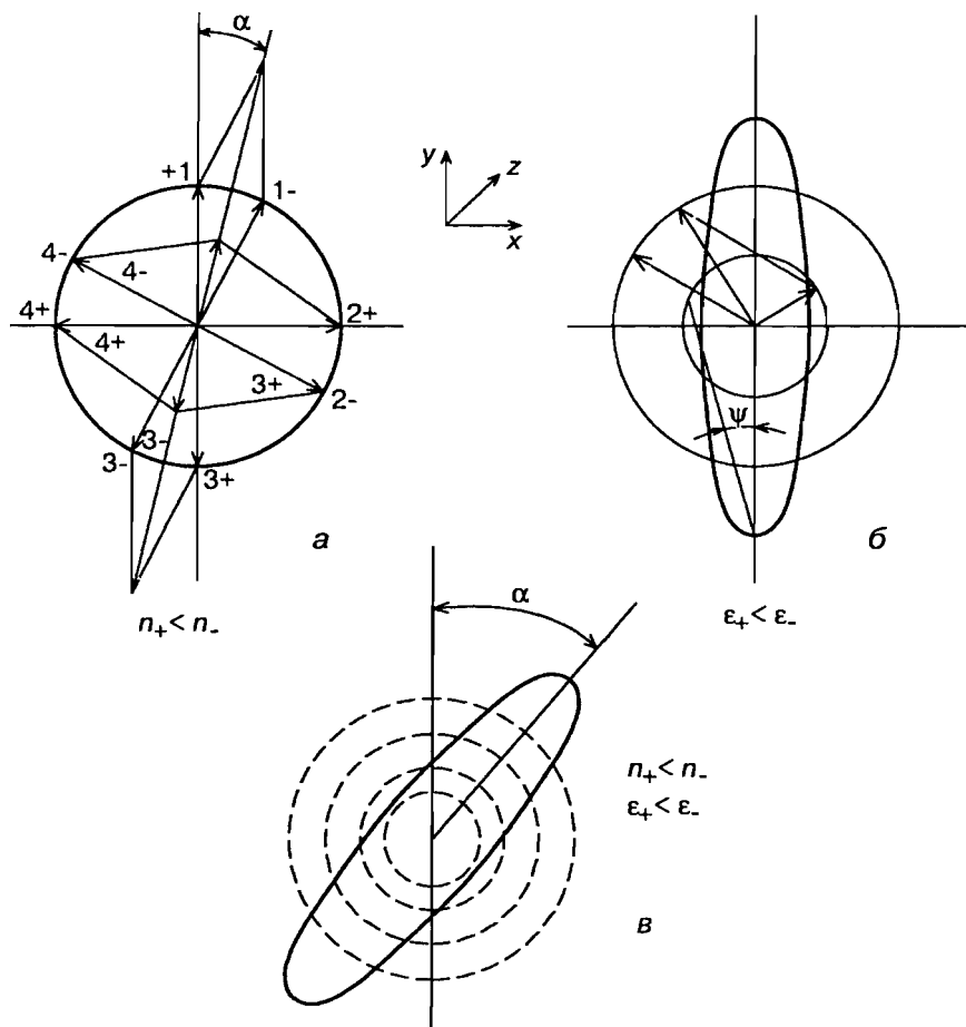
Рис. 8.2. a — Взаимодействие сдвинутых по фазе компонент равной амплитуды; б — взаимодействие находящихся в фазе компонентов разной амплитуды; в — суммарный результат сдвига по фазе. Точки 1, 2, 3, 4 соответствуют точкам на рис. 8.1, б и в . Знак «плюс» для правого луча, знак «минус» для левого «отстающего» и более сильно поглощаемого луча
