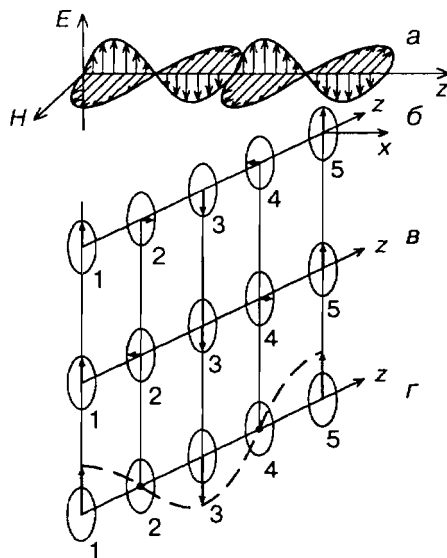
Рис. 8.1. Плоско (линейно) поляризованный световой луч (а), правый (б) и левый (в) циркулярно поляризованные лучи (показаны только векторы электрического поля). г — Результат взаимодействия электрических векторов лучей (б) и (в), находящихся в фазе
