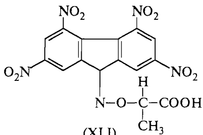
(XLI)
