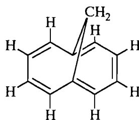
1,6-метаноциклодека- пентаен
