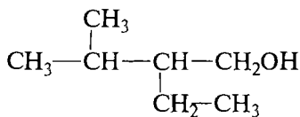
2-этил-3-метилбутанол-1
