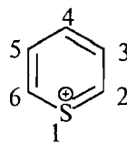
катион тиопирилия
