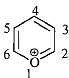
катион пирилия
