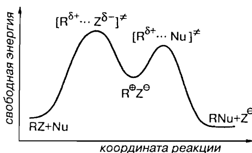
Рис. 9.6. Первая стадия ионизации \text{RZ}
