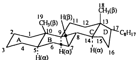
5α-холестан
