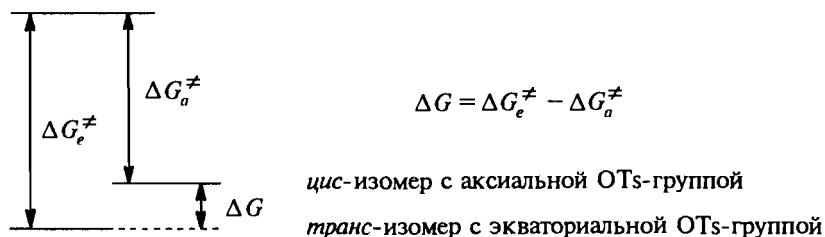
Рис. 22.4. Соотношение энергий активации сольволиза цис - и транс -изомеров тозилатов 4- трет -бутилциклогексанола соответственно с аксиальной и экваториальной тозилосигруппой
