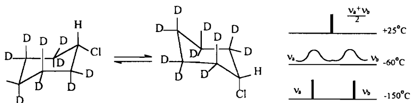
Рис. 22.3. ПМР спектр декадейтерохлорциклогексана при +25°; -60° и -150°С
