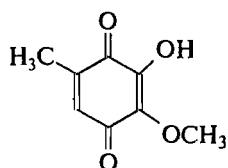
3-гидрокси-2-метокси- 5-метил-1,4-бензохинон (антибиотик фумигатин)
