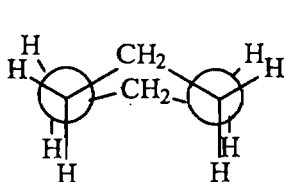
проекция Ньюмена для формы ванны
