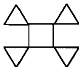
4-ротан
