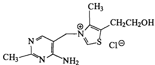
тиаминхлорид (витамин В 1 )
