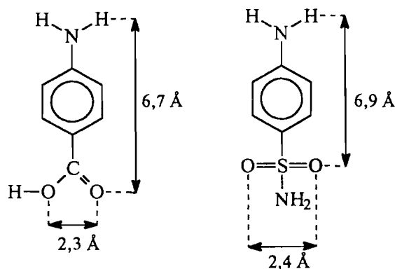
Рис. 19.1. Структурное подобие para -аминобензойной кислоты и сульфаниламида
