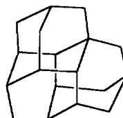
триамантан
