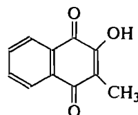
фтиокол (антибиотик) 2-гидрокси-3-метил- 1,4-нафтохинон
