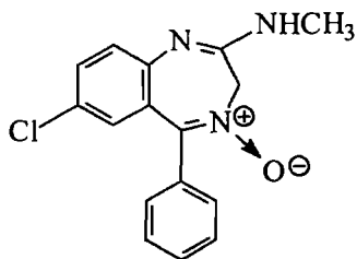
элениум
