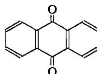
9,10-антрахинон
