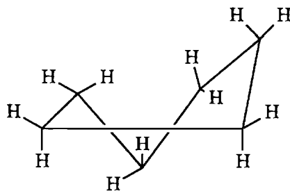
твист-форма
