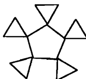
5-ротан
