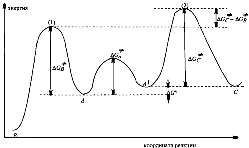
Рис. 22.5. Влияние конформационного равновесия на соотношение продуктов реакции
