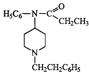
фентанил
