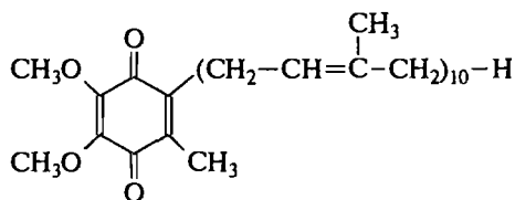
убихинон (коэнзим Q 10 )
