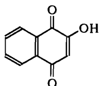
2-гидрокси-1,4-нафтохинон (действующее начало хны)
