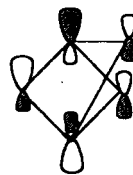
НСМО
