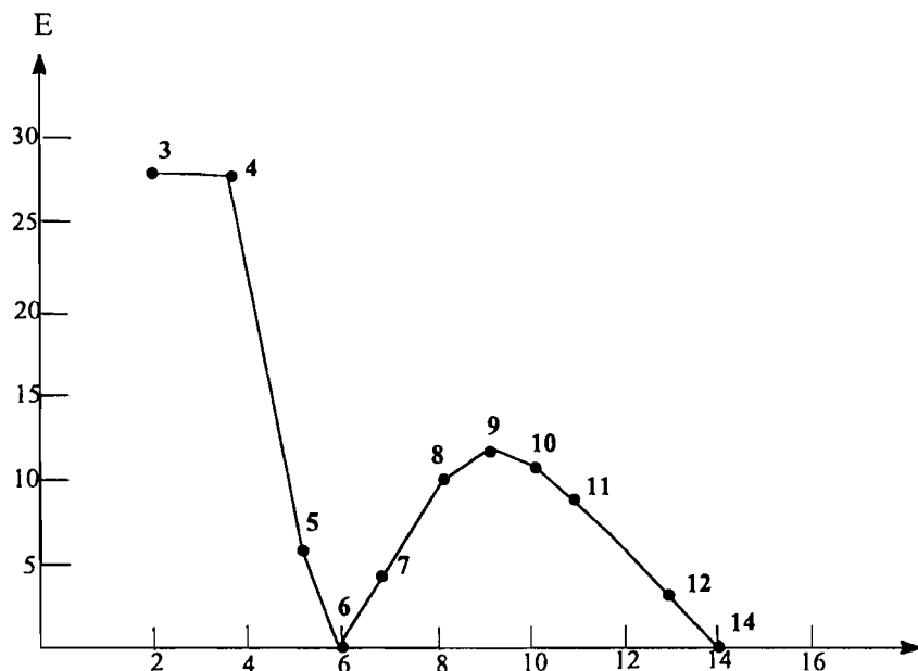
Рис. 22.1. Изменение энергии напряжения циклоалканов в зависимости от размера цикла
