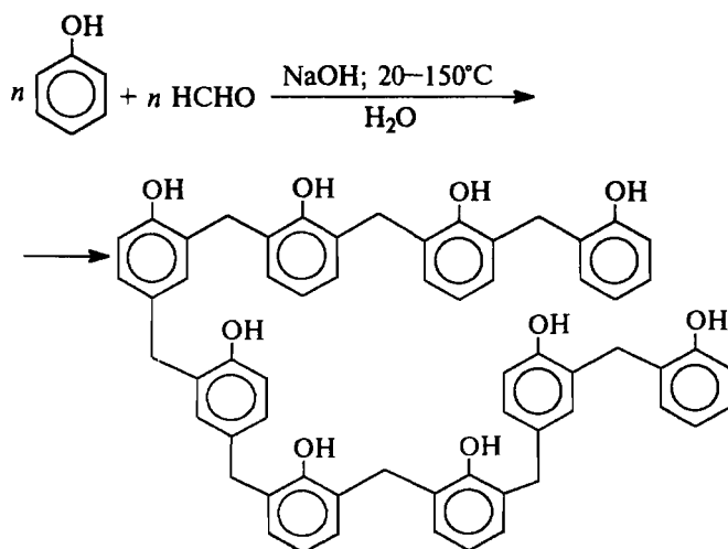
Структура феноло-формальдегидной смолы
