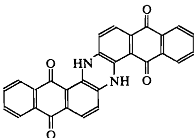
индантреновый синий Р для хлопка (индантрен)
