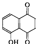
юглон (5-гидро- кси-1,4-нафтохинон)
