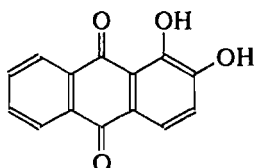
ализарин (протравной краситель) 1,2-дигидро- кси-9,10-антрахинон
