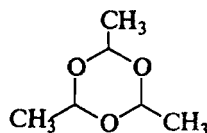
паральдегид
