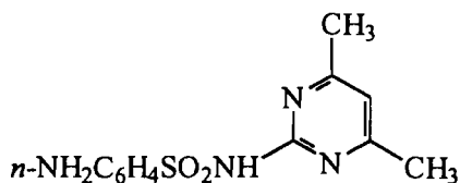
сульфадимезин
