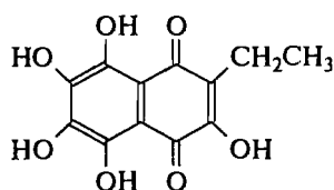
эхинохром А (пигмент морского ежа)
