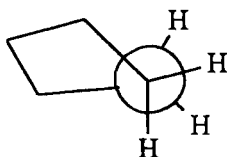
проекция Ньюмена
