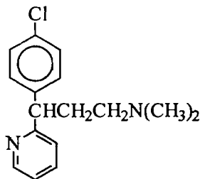
хлорфенирамин
