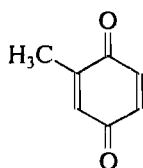
2-метил-1,4-бензо- хинон (толухинон)
