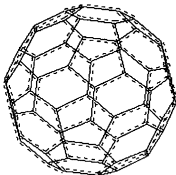
фуллерен C 60
