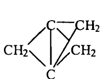
[1.1.1]-пропеллан
