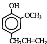
4-аллил-2-метоксифенол, (эвгенол)
