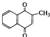
2-метил-1,4-нафтохинон
