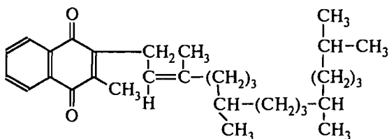
витамин K 1 (филлохинон)
