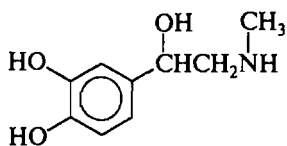
адреналин
