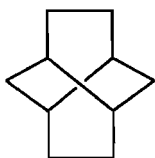
твистан
