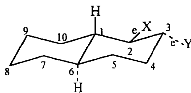
экваториальный ( 2\beta ; 3\alpha )*
