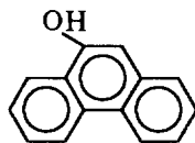
9-фенантрол
