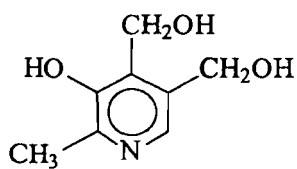
пиридоксин (витамин В 6 )
