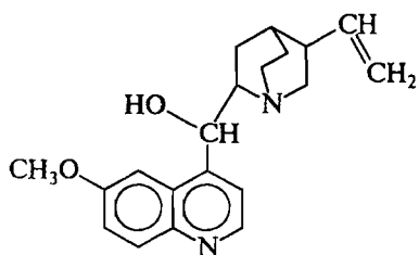
хинин
