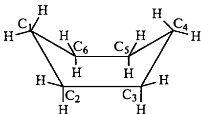
конформация ванны
