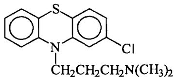
хлорпромазин
