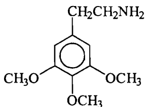
мескалин
