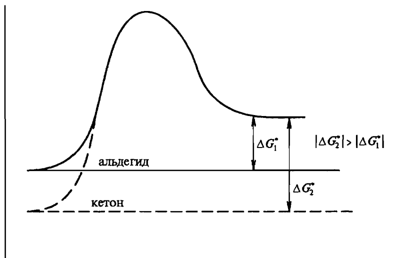
Рис. 16.1. Энергетическая диаграмма для обратимого присоединения нуклеофильного агента NuH к альдегидам и кетонам
