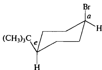
цис -4-бром-1- трет -бутил циклогексан
