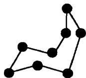
ванна-кресло
