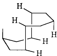
циклодекан (ванна-кресло-ванна)
