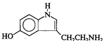
серотонин
