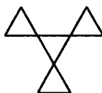
3-ротан
