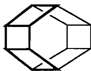
тетрастиран
