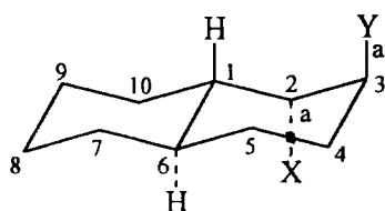
аксиальный ( 2\alpha ; 3\beta )*
