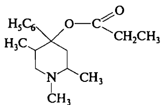
промедол
