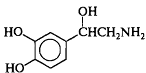
норадреналин
