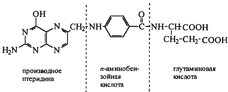
Фолиевая кислота
