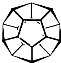
додекаэдран, т. пл. 430°C
