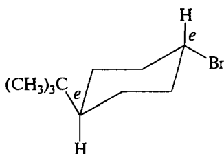
транс -4-бром-1- трет -бутил циклогексан
