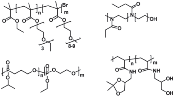
Նկ. 9. Զերմաստիճանի փոփոխությանը արձագանքող որոշ պոլիմերների կառուցվածքներ:
