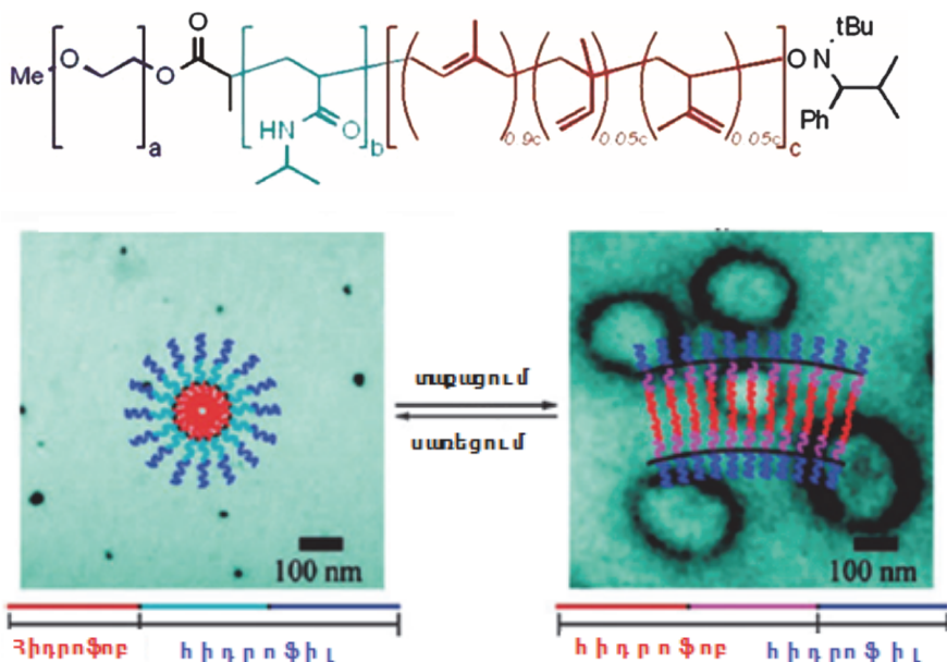
Նկ. 8. NIPA բլոկ պարունակող տրիբլոկ պոլիմեր:
