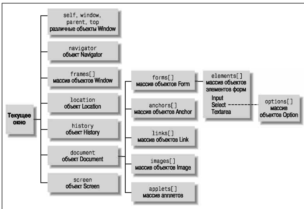
Рис. 13.1. Иерархия объектов клиентского JavaScript и нулевой уровень модели DOM
