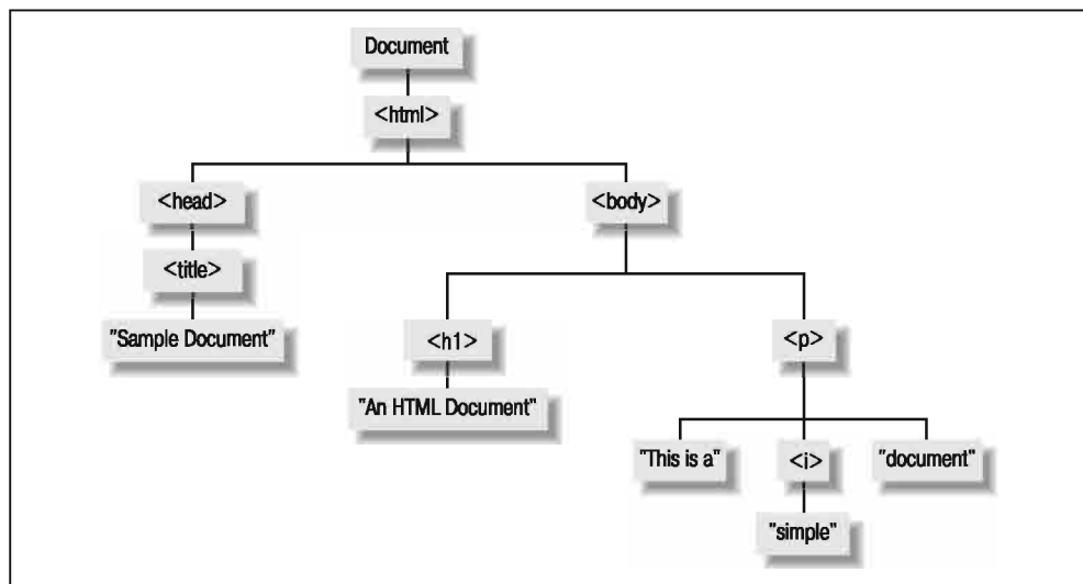
Рис. 15.1. Древовидное представление HTML-документа
