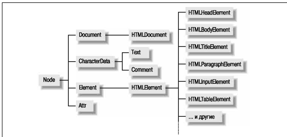
Рис. 15.2. Неполная иерархия классов DOM API
