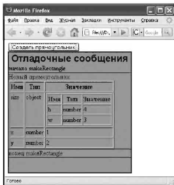
Рис. 15.4. Результат исполнения функции log()
