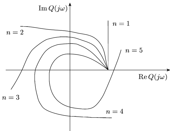
Рис. 3.2. Кривые Михайлова устойчивых систем
