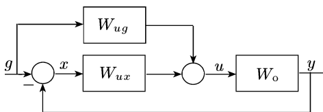
Рис. 5.2. Структурная схема (к примеру 5.10)
