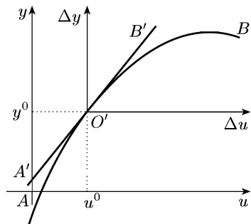
Рис. 2.1. Линейризация
