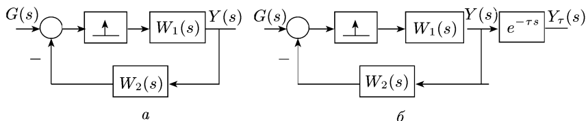
Рис. 8.2. Структурные схемы (к определению переходной функции h_\tau[lT] ): а — исходная схема; б — преобразованная схема
