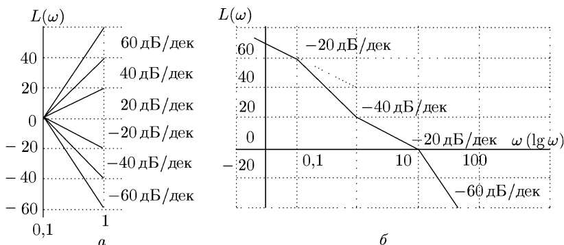
Рис. 2.6. К построению асимптотических ЛАЧХ: a — наклоны асимптот; б — асимптотическая ЛАЧХ
