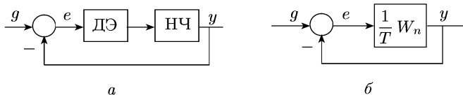
Рис. 6.25. Дискретная система (а) и ее непрерывная модель (б)
