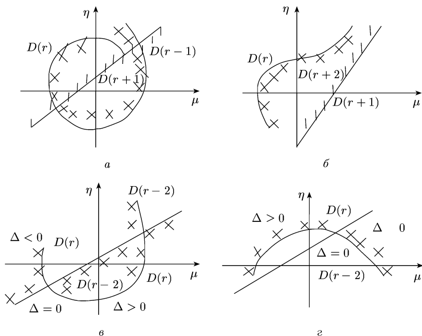
Рис. 3.9. Штриховка особых прямых: a - \omega = 0 ; b - \omega = \pm\infty ; c - \omega = \omega_k ; d - \omega = \omega_k
