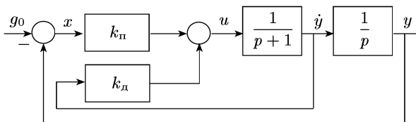
Рис. 5.3. Структурная схема (к вопросу о реализуемости)
