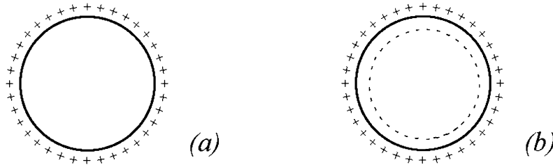
Рис. 12.1: Потенциалы простого (a) и двойного (b) слоя.
