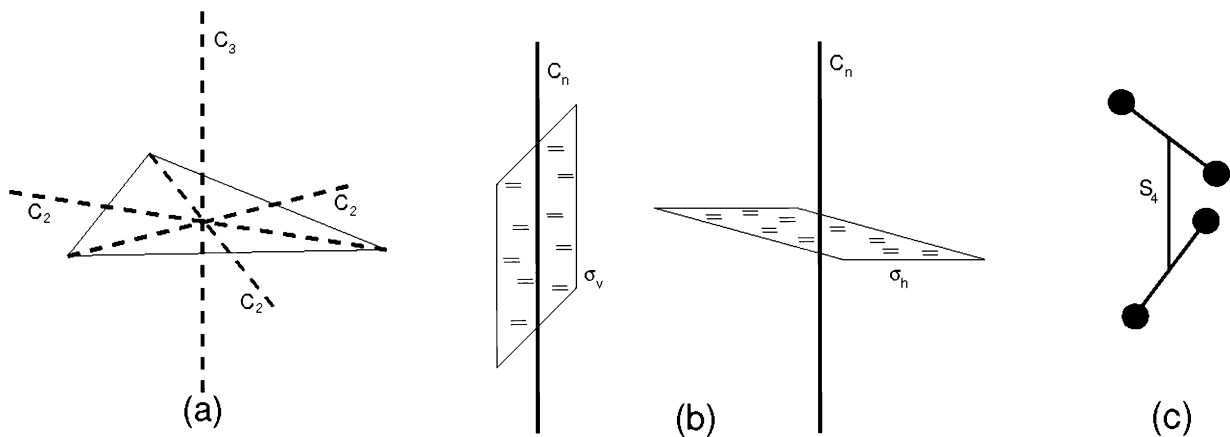
Рис. 1.1: (a) Группа вращений правильного треугольника включает в себя ось третьего порядка C_3 и три оси второго порядка C_2 . (b) Вертикальная зеркальная плоскость \sigma_v и горизонтальная \sigma_h . (c) “Молекула”, имеющая зеркально-поворотную ось четвертого порядка S_4 .
