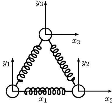
Рис. 4.1: Координаты ядер трехатомной молекулы с симметрией C_{3v} . Оси z_{1,2,3} направлены на читателя из плоскости рисунка и не изображены.
