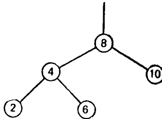
Рис 4.31. Сбалансированное дерево.
