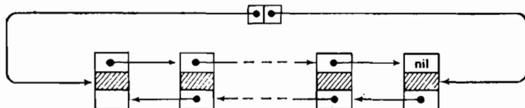
Рис. 4.55. Двунаправленный список.
