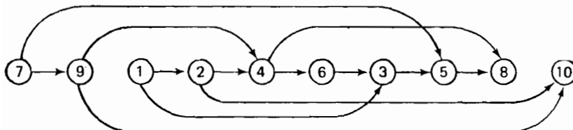
Рис. 4.14. Линейное расположение частично упорядоченного множества, приведенного на рис. 4.13.
