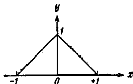
Рис. 5. y = 1 - |x| , |x| \leq 1 .
