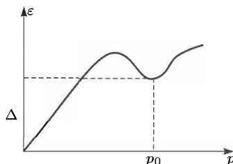
Рис. 19.1. Зависимость энергии фононов-ронов от импульса
