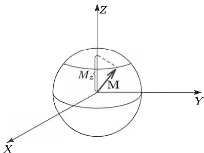
Рис. 7.2. Вектор момента количества движения M
