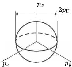
Рис. 17.1 Сфера Ферми
