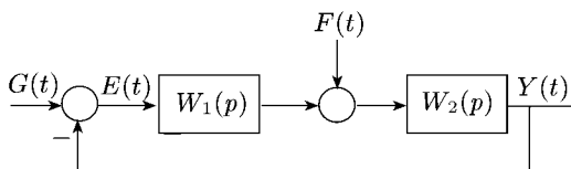
Рис. 10.2. К анализу систем при случайных воздействиях
