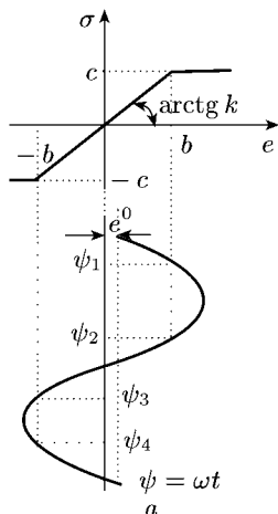
Рис. 3.10. Несимметричные колебания на входе и выходе НЗ с кусочно линейной характеристикой с насыщением
