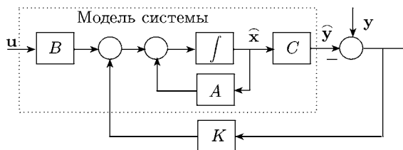
Рис. 9.3. Структурная схема наблюдателя
