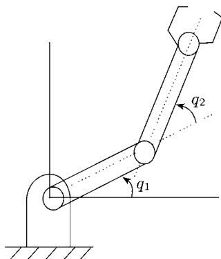
Рис. 8.5. Двухзвенный робот
