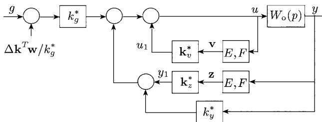
Рис. 11.8. Эквивалентная структурная схема основного контура
