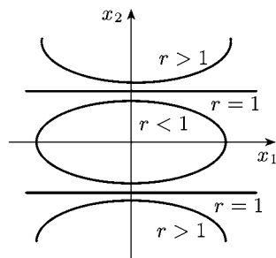
Рис. 4.1. Кривые уравнения (1-r^2)x_1^2 + x_2^2 = r^2
