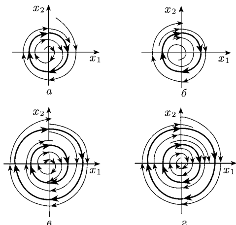
2.8. Предельные циклы
