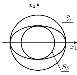
Рис. 2.6. К определению устойчивости особой точки типа центр
