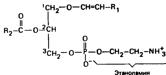
Рис. 15.17. Плазмалоген (фосфатидальтаноламин).
