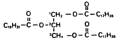
Рис. 15.7. 1,3-Дистеаропальмитин.
