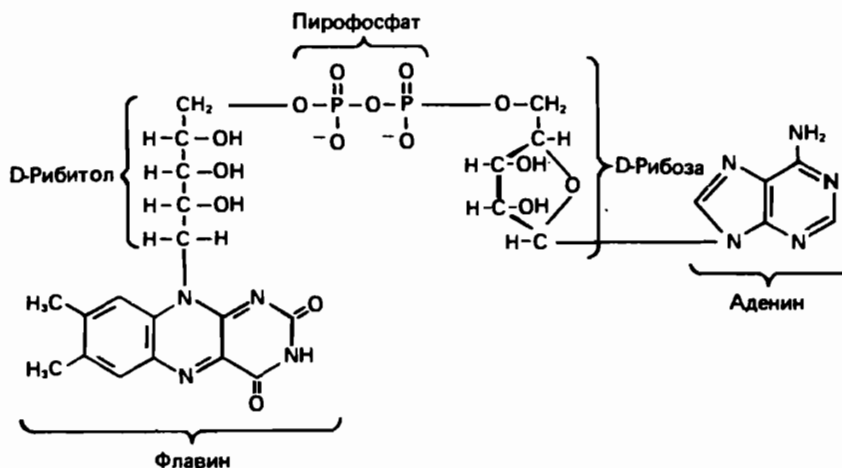
Рис. 12.7. Флавинадениндинуклеотид (FAD).
