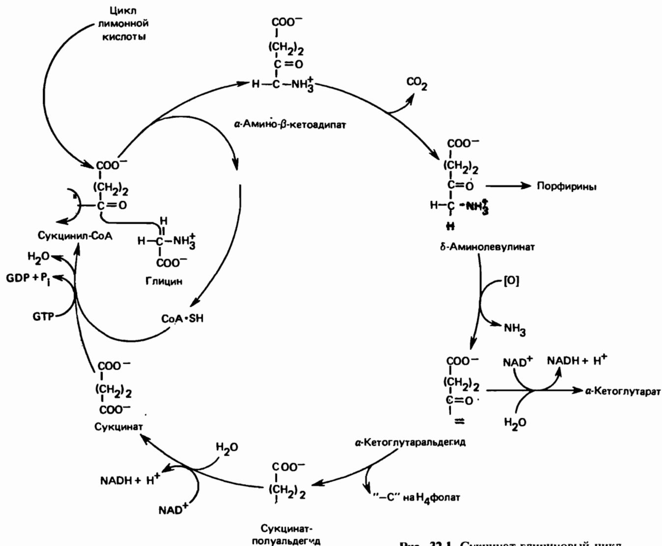
Рис. 32.1. Сукцинат-глициновый цикл.
