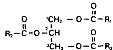
Рис. 15.6. Триацилглицерол.
