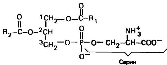
Рис. 15.15. 3-Фосфатидилсерин.
