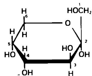
α-D-Фруктопираноза
