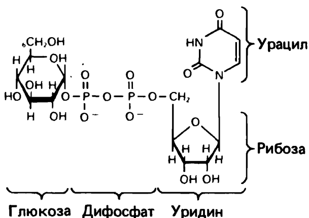
Рис. 19.2. Уридиндифосфатглюкоза (UDPGlc).
