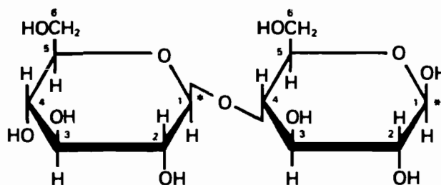
Целлобиоза
