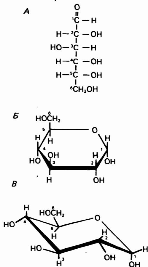
Рис. 14.1. \alpha -D-глюкоза.
