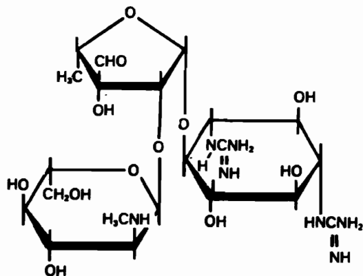
Рис. 14.10. Стрептомицин (слева) и убаин (справа).
