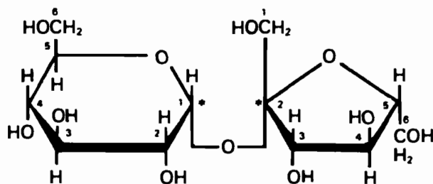
Сахароза
