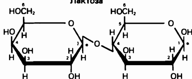
Лактоза
