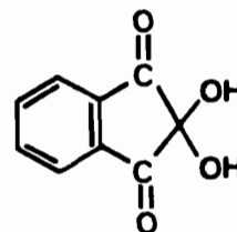
Рис. 3.5. Нингидрин.
