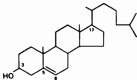
Рис. 15.24. Холестерол.
