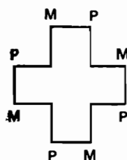
Копропорфирин III
