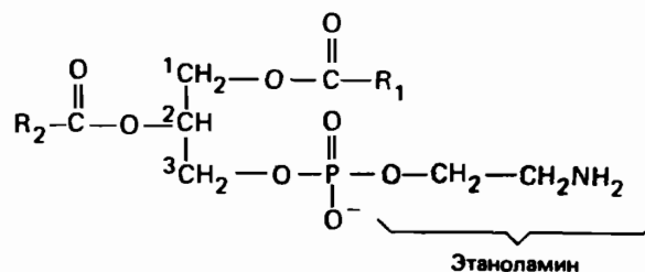
Рис. 15.13. 3-Фосфатидилэтанолламин.
