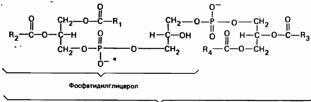
Рис. 15.11. Дифосфатидилглицерол (кардиолипин).
