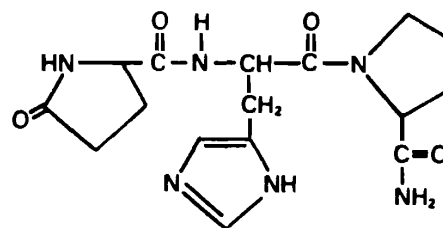
Рис. 4.5. Тиреолиберин (пироглутамилгистидилпролин-амид).
