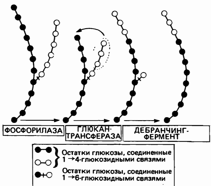
Рис. 19.4. Стадии гликогенолиза.
