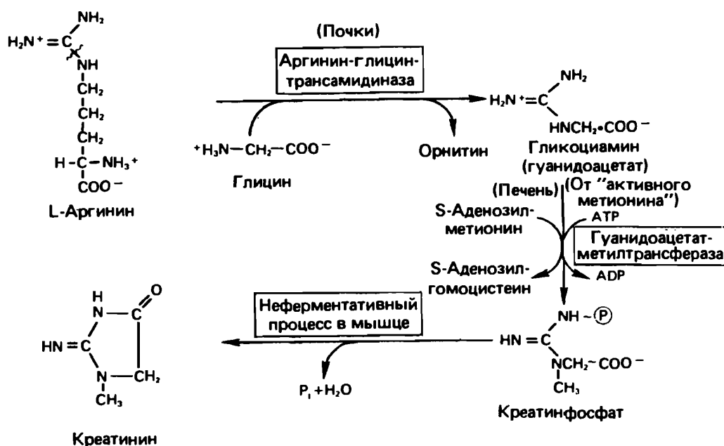
Рис. 32.11. Биосинтез креатина и креатинина.
