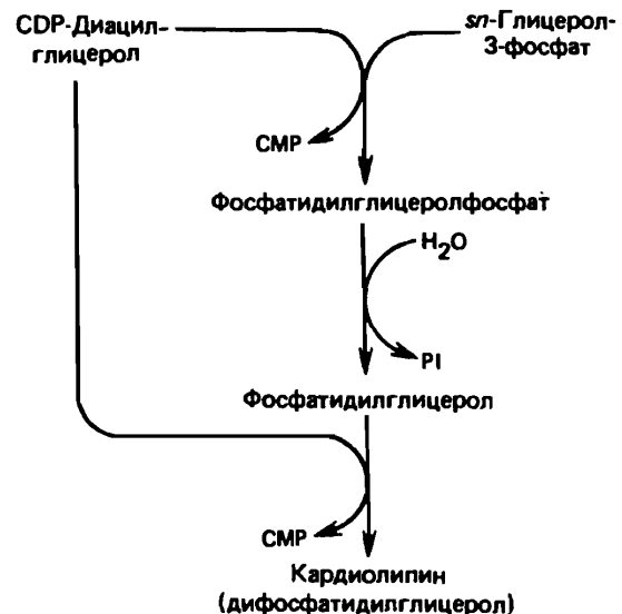
Рис. 25.2. Биосинтез кардиолипина.
