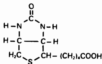
Рис. 20.3. Биотин.
