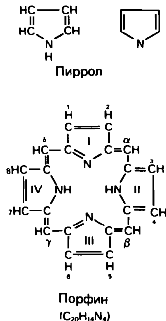
Рис. 33.1. Молекула порфина. Кольца обозначены цифрами I, II, III и IV. Места присоединения замещающих групп обозначены номерами 1, 2, 3, 4, 5, 6, 7, 8. Метенильные мостики обозначены буквами \alpha , \beta , \gamma и \delta .
