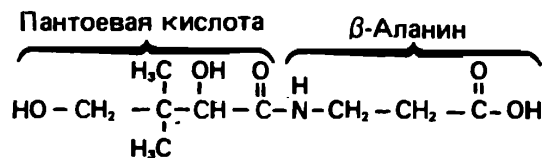
Рис. 17.5. Пантотеновая кислота.
