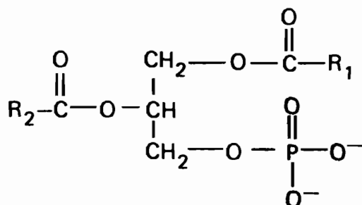
Рис. 15.10. Фосфатидная кислота.
