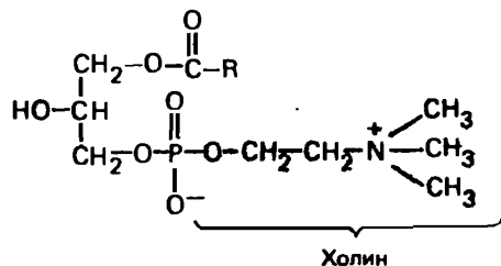
Рис. 15.16. Лизолецитин.
