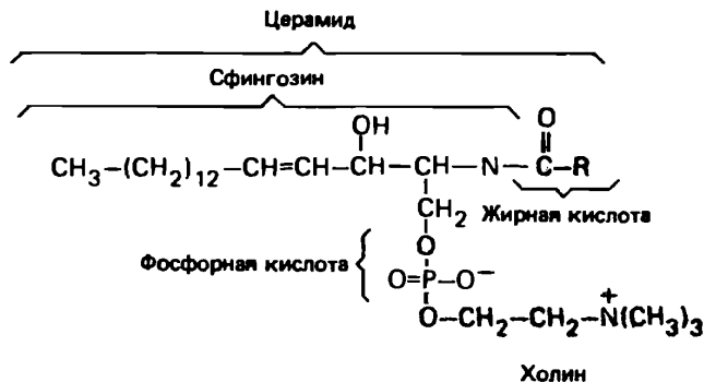
Рис. 15.18. Сфингомиелин.
