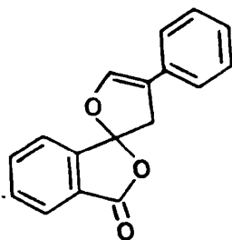
Рис. 3.6. Флуорескамин.
