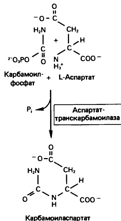
Рис. 10.7. Реакция, катализируемая аспартат-транскарбамоилазой (АТКазой).
