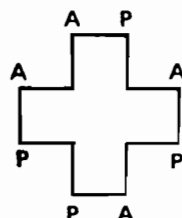
Уропорфирин I
