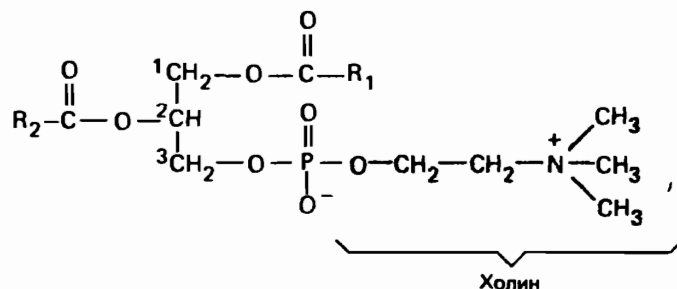
Рис. 15.12. 3-Фосфатидилхолин.
