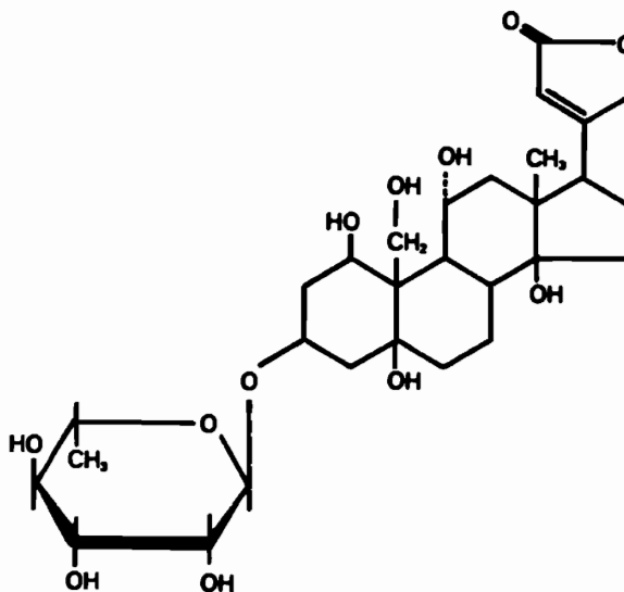
Рис. 14.10. Стрептомицин (слева) и убаин (справа).
