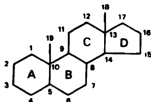
Рис. 15.21. Стероидное ядро.
