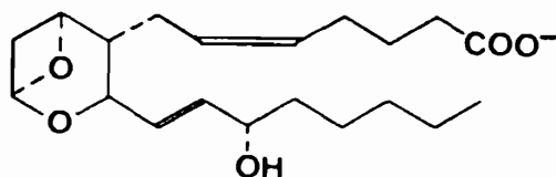
Рис. 15.3. Тромбоксан A_2 .
