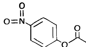
Рис. 9.1. n -Нитрофенилацетат.
