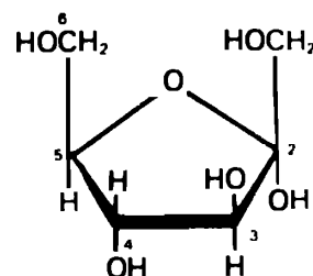
α-D-Фруктофураноза
