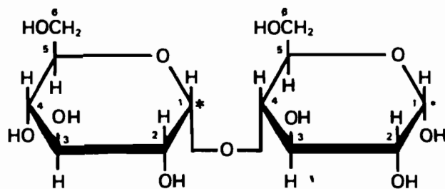
Мальтоза
