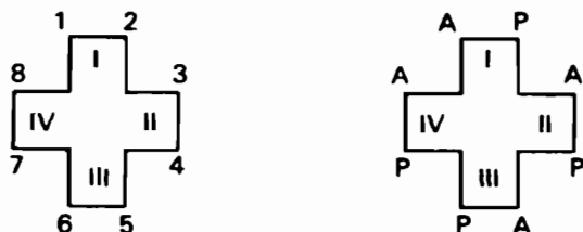
Рис. 33.2. Уропорфирин III.
