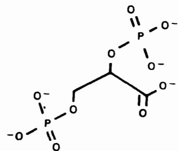
Рис. 6.16. Структура 2,3-бисфосфоглицерата.
