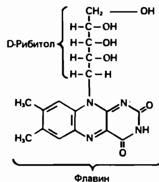
Рис. 12.5. Рибофлавин.
