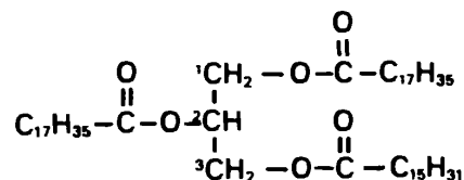
Рис. 15.8. 1,2-Дистеаропальмитин.
