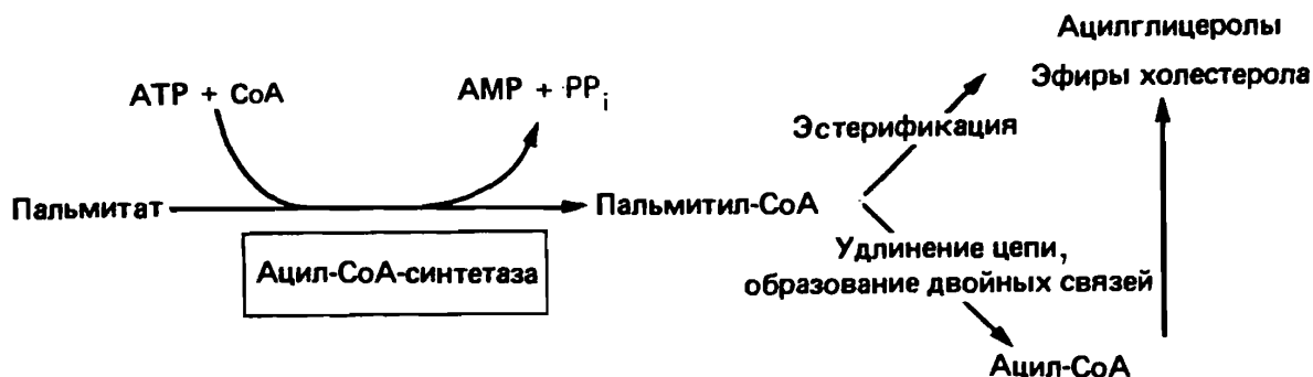
Рис. 23.8. Судьба пальмитата.
