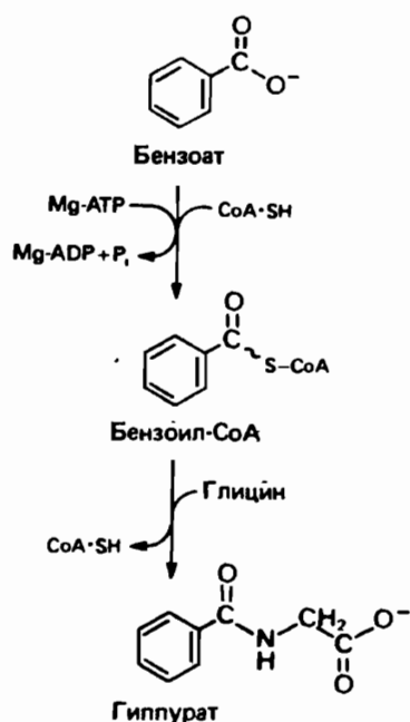
Рис. 32.2. Биосинтез гиппурата.
