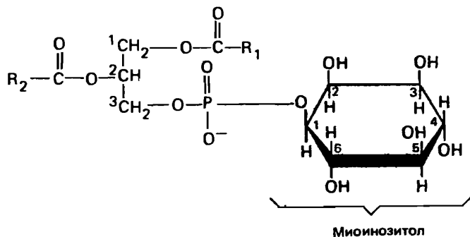
Рис. 15.14. 3-Фосфатидилинозитол.
