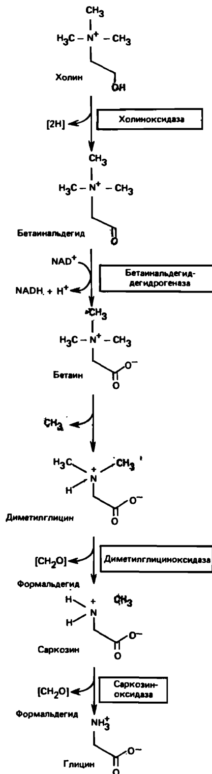
Рис. 29.6. Образование глицина из холина.
