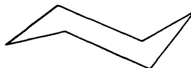
Конформация «кресла»
