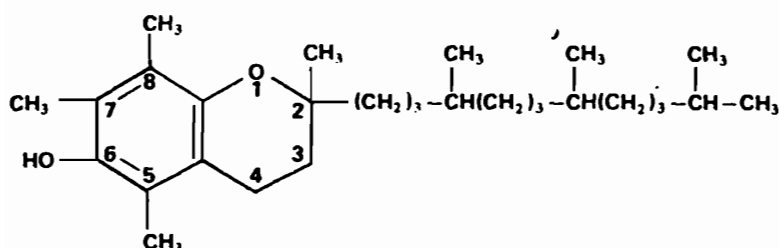
Рис. 15.29. \alpha -Токоферол.
