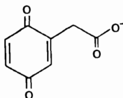
Бензо хинонацетат
