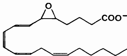
Рис. 15.4. Лейкотриен A_4 .
