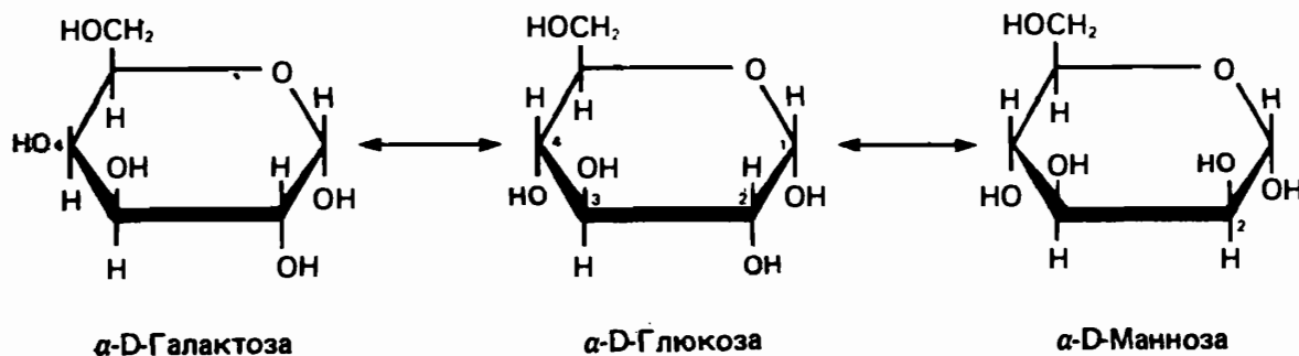
Рис. 14.6. Эпимеризация глюкозы.
