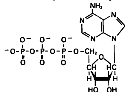
Рис. 11.5. Аденозинтрифосфат (АТР).
