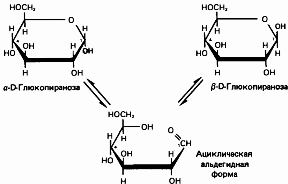
Рис. 14.5. Мутаротация глюкозы.
