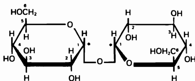
Трегалоза
