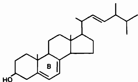
Рис. 15.25. Эргостерол.
