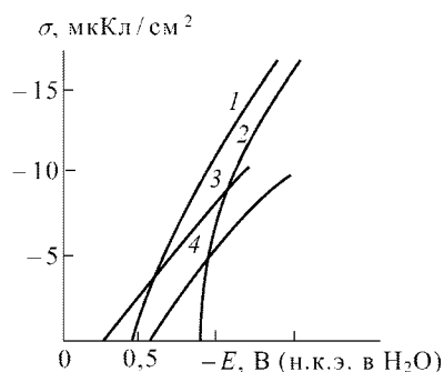
Рис. 11.13. Зависимость заряда поверхности ртути (1, 3) и галлия (2, 4) в 1 M \text{Na}_2\text{SO}_4 в воде (1, 2) и в 0,1 н. \text{LiClO}_4 в ацетонитриле (3, 4) от потенциала
