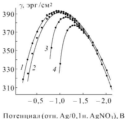
Рис. 11.11. Электрокапиллярные кривые Hg в метаноле при 8 °C: 1 — 0,1 M \text{NH}_4\text{NO}_3 ; 2 — 1 M \text{NH}_4\text{NO}_3 ; 3 — 1 M NaBr; 4 — 1 M NaI
