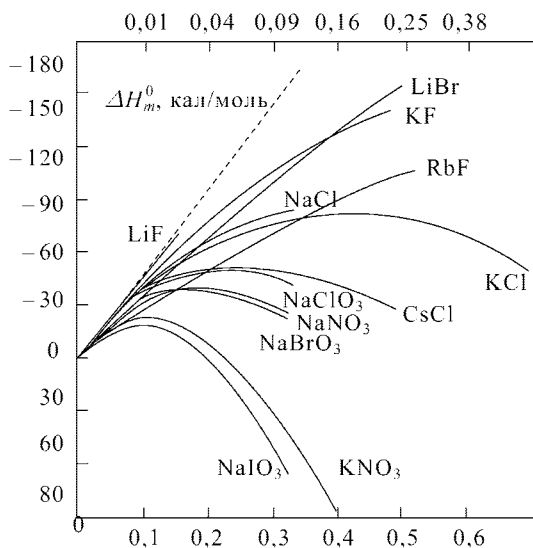
Рис. 7.1. Зависимость интегральных теплот разведения 1–1 валентных солей в воде при 24 °C
