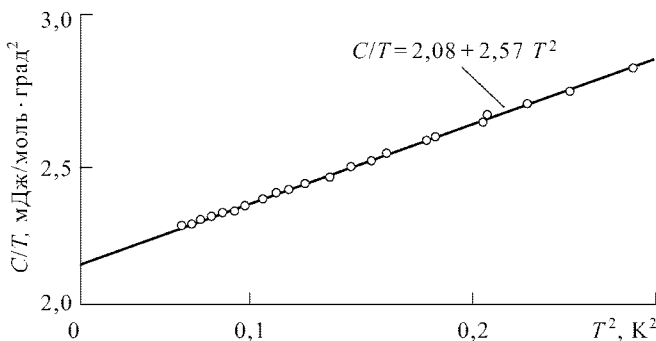
Рис. 1.2. Зависимость C/T от T^2 для калия
