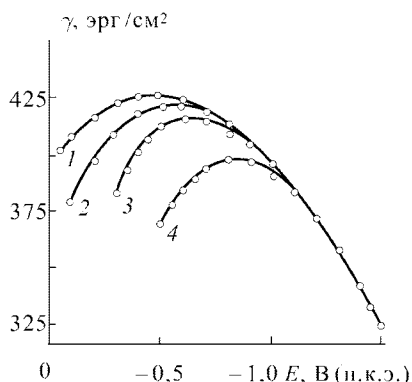
Рис. 11.10. Электрокапиллярные кривые Hg-электрода в водных растворах солей: 1 — 0,9 M NaF; 2 — 0,9 M NaCl; 3 — 0,9 M NaBr; 4 — 0,9 M NaI
