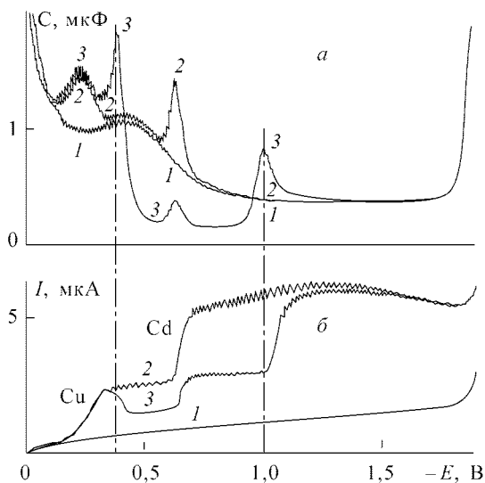
Рис. 15.9. Вольтфарадные (а) и вольтамперные (б) зависимости Hg-электрода в растворе, содержащем \text{Cu}^{2+} , \text{Cd}^{2+} и триэтилфосфат на фоне 1 \text{ M KCl} : 1 — раствор \text{KCl} ; 2 — \text{Cu}^{2+} ( 1,0 \cdot 10^{-4} \text{ M} ) + \text{Cd}^{2+} ( 1,6 \cdot 10^{-4} \text{ M} ); 3 — \text{Cu}^{2+} ( 1,0 \cdot 10^{-4} \text{ M} ) + \text{Cd}^{2+} ( 1,6 \cdot 10^{-4} \text{ M} ) + триэтилфосфат ( 2,5 \cdot 10^{-3} \text{ M} )
