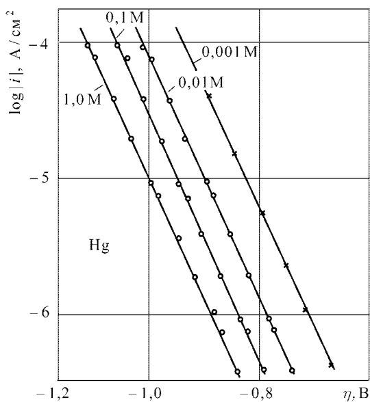
Рис. 15.6. Зависимость перенапряжения выделения водорода на \text{Hg} в водных растворах 0,991н. \text{HCl} при добавках \text{KCl}
