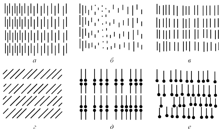
Рис. 10.1. Структура различных форм жидких кристаллов: а — нематическая; б — холестерическая; в — смектическая; г — скошенная смектическая; д — смектическая с двойными связями; е — смектическая с полярным порядком
