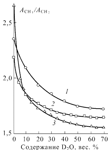
Рис. 7.5. Зависимость относительного уширения линий спектра ЯМР ( A_{CH_3} / A_{CH_2} ) от содержания D_2O в смешанном растворителе C_2H_5OD - D_2O для растворов парамагнитных солей. 1 — CuCl_2 (0,1 моль/л); 2 — CuCl_2 (0,05 моль/л); 3 — Cu(NO_3)_2 \times 3H_2O (0,05 моль/л)
