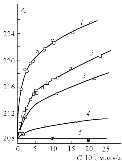
Рис. 7.4. Зависимость величины химического сдвига для иона Bu_4N^+ от концентрации различных солей его в нитробензоле при 35,9^\circ C . 1 — Bu_4NCl ; 2 — Bu_4NBr ; 3 — Bu_4NI ; 4 — Bu_4NClO_4 ; 5 — Bu_4NPic
