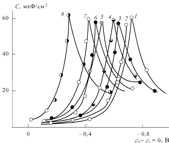
Рис. 15.11. Катодные участки зависимости дифференциальной емкости двойного слоя от относительного потенциала в растворе 0,1 М \text{H-C}_5\text{H}_{11}\text{OH} на металлах: 1 — Hg; 2 — Bi; 3 — Pb; 4 — Sn; 5 — Cd; 6 — In; 7 — In-Ga; 8 — Ga
