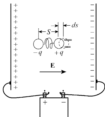
Рис. 11.5. Модель поляризуемой молекулы
