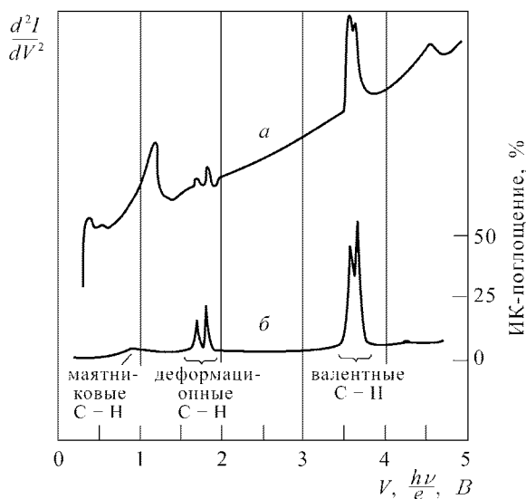
Рис. 15.8. Туннельный (а) и инфракрасный (б) спектры углеводорода с большим молекулярным весом при T = 4, 2 \text{ K}
