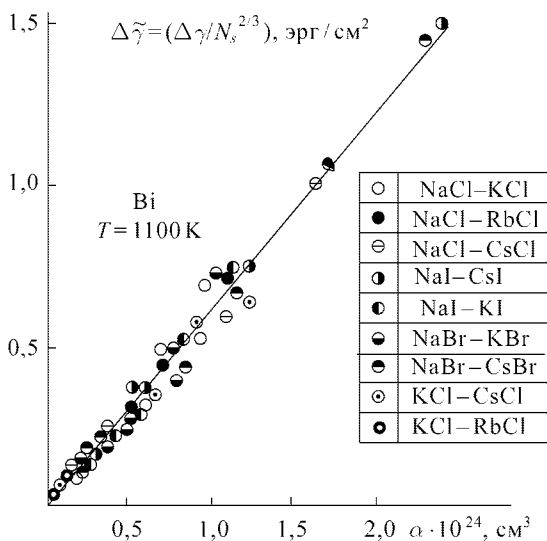
Рис. 11.8. Зависимость изменения мольного поверхностного натяжения \gamma N_{0i}^{-2/3} висмута от поляризуемости расплавленных щелочногалогенидных солей
