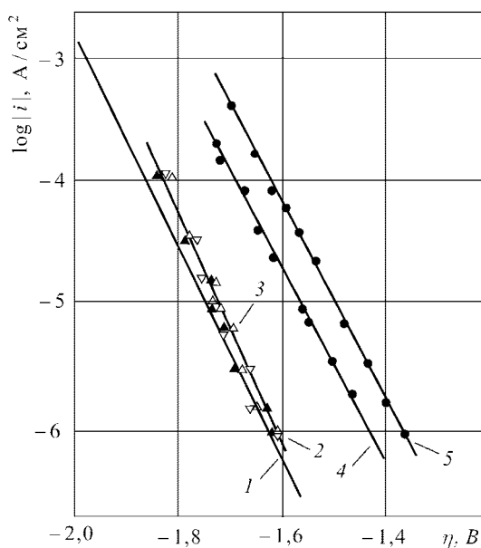
Рис. 15.5. Перенапряжение выделения водорода на ртути в водных растворах \text{HCl} при разных \text{pH} : 1 — 13,3, 2 — 12,8, 3 — 11,1, 4 — 6,9, 5 — 6,3
