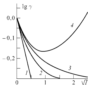
Рис. 7.7. Средний рациональный коэффициент активности NaCl при 20 °С как функция ионной силы раствора (рассчитан по уравнениям (7.64) (кривая 1), по (7.63) при Ba = 1 (кривая 2), по (7.63) при a = 4 \cdot 10^{-8} см (кривая 3) и кривая 4 — эксперимент
