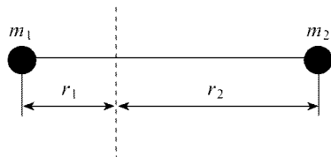
Рис. 5.3. Модель колебательного движения двухатомной молекулы
