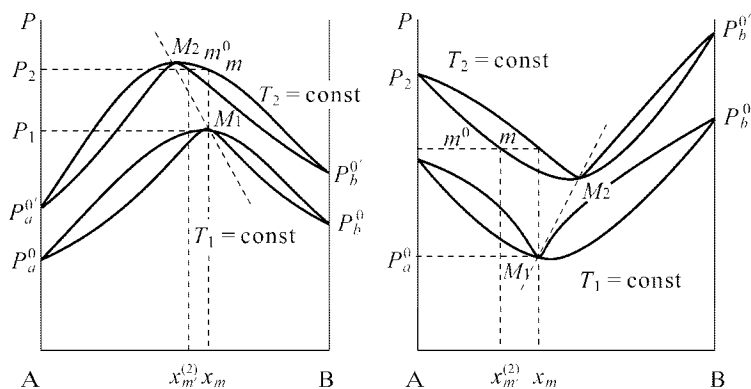
Рис. 8.5. Влияние температуры на состав пара и состав азеотропной смеси при закрепленном составе жидкости
