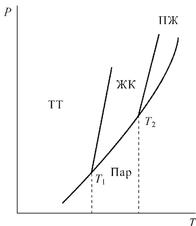
Рис. 10.3. Фазовая диаграмма ЖК
