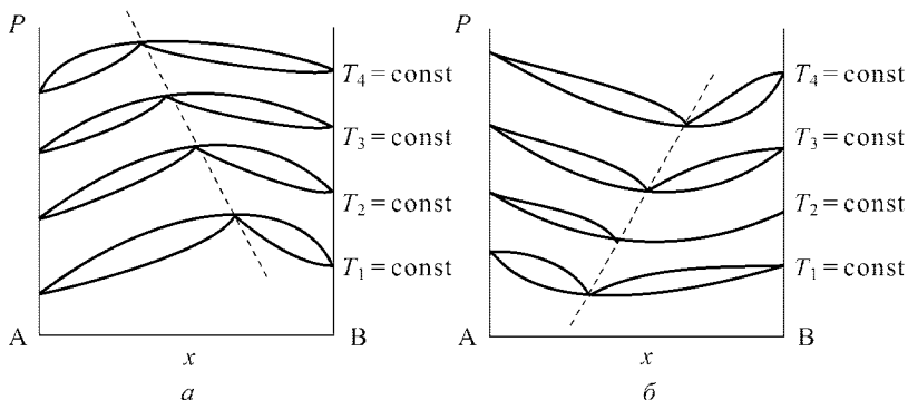
Рис. 8.7. Влияние температуры на состав азеотропной смеси
