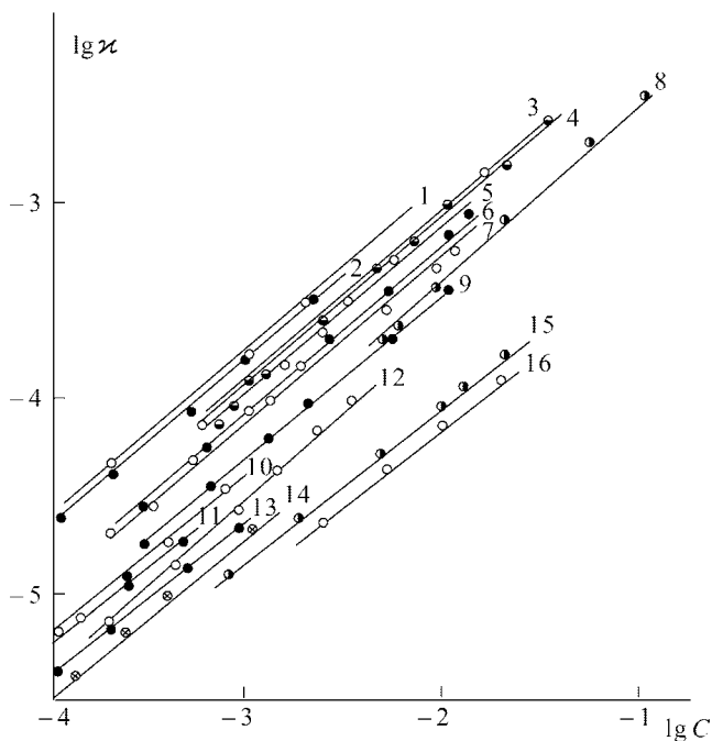
Рис. 7.18. Зависимость \lg \kappa (C_2H_5)_4NI от \lg c в неводных растворителях: 1 — ацетонитрил, 2 — ацетон, 3 — пропионитрил, 4 — метанол, 5 — вода, 6 — метилроданид, 7 — ацетилбромид, 8 — метилформаид, 9 — эпихлоргидрин, 10 — этанол, 11 — хлористый метил, 12 — диметилсульфоксид, 13 — этиленхлорид, 14 — n -пропанол, 15 — метиленхлорид, 16 — пропиональдегид
