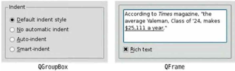
Рис. 2.18. Виджеты одностраничных контейнеров Qt
