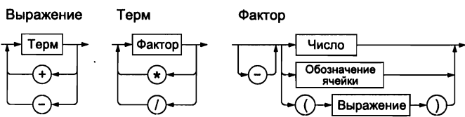
Рис. 4.10. Блок-схема синтаксического анализа выражений электронной таблицы
