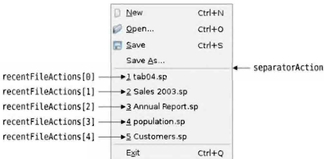
Рис. 3.11. Меню File со списком файлов, которые открывались недавно
