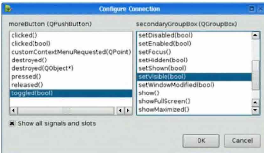
Рис. 2.16. Редактор соединений в Qt Designer
