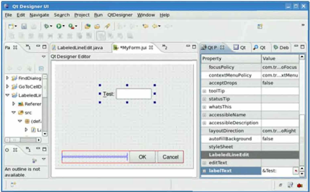
Рис. В.3. Форма с пользовательским виджетом LabeledLineEdit
