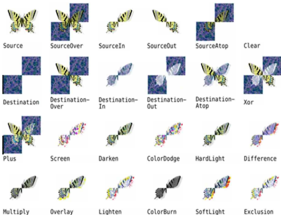
Рис. 8.13. Режимы композиции QPainter
