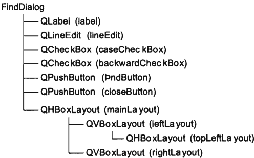
Рис. 2.3. Родословная объектов диалогового окна поиска данных
