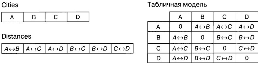
Рис. 10.13. Структуры данных cities и distances и табличная модель
