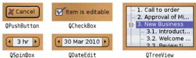
Рис. 19.17. Виджеты в стиле Bronze
