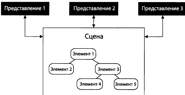
Рис. 8.14. Одна сцена может быть связана с несколькими представлениями
