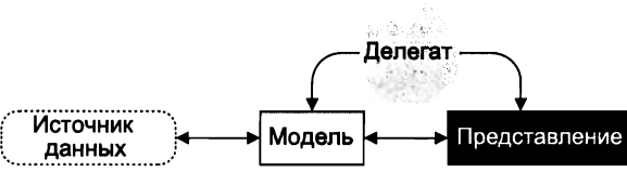
Рис. 10.1. Архитектура модель/представление в Qt
