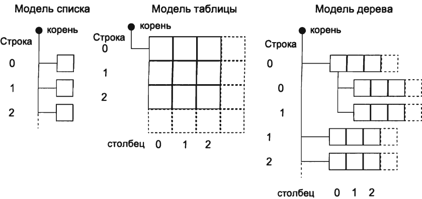
Рис. 10.9. Схематическое представление моделей Qt
