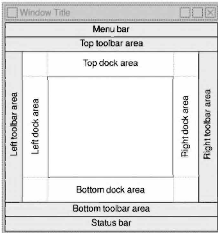
Рис. 6.14. Области крепления виджетов и области панелей инструментов QMainWindow
