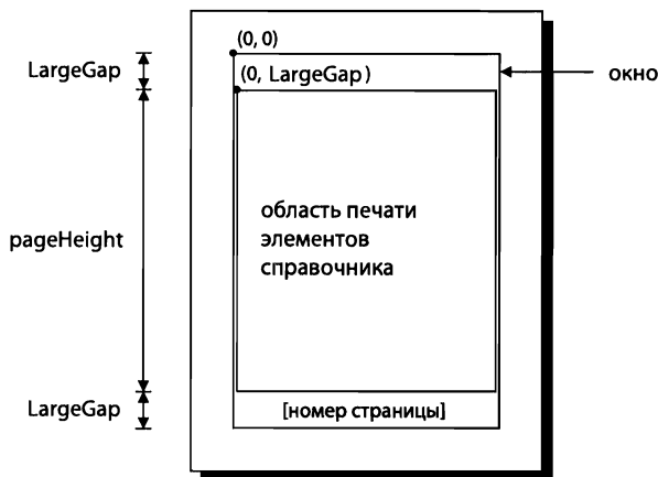
Рис. 8.22. Компоновка страницы справочника по цветам
