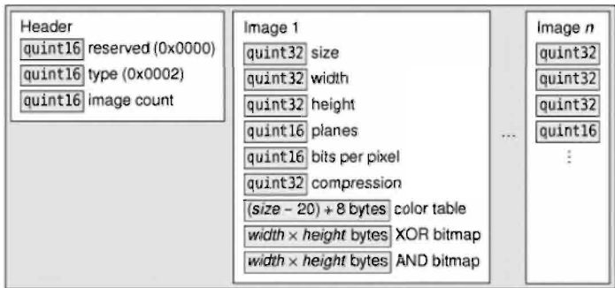
Рис. 21.2. Формат файла .cur
