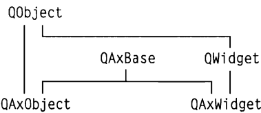
Рис. 23.4. Дерево наследования для модуля QAxContainer
