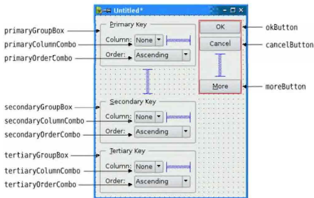
Рис. 2.14. Имена виджетов формы
