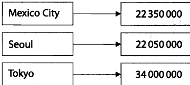
Рис. 11.6. Ассоциативный массив, связывающий QString с int
