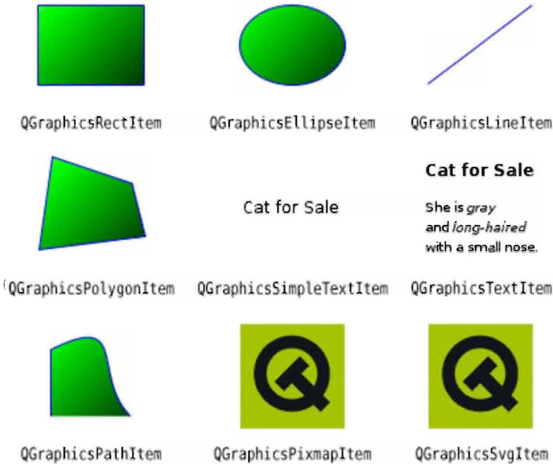
Рис. 8.15. Элементы графических представлений, имеющиеся в Qt 4.3
