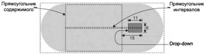
Рис. 19.13. Структура поля QComboBox, доступного только для чтения
