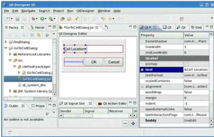
Рис. В.2. Диалоговое окно Go to Cell в Eclipse
