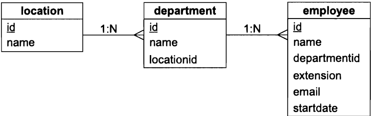
Рис. 13.2. Таблицы приложения Менеджер персонала
