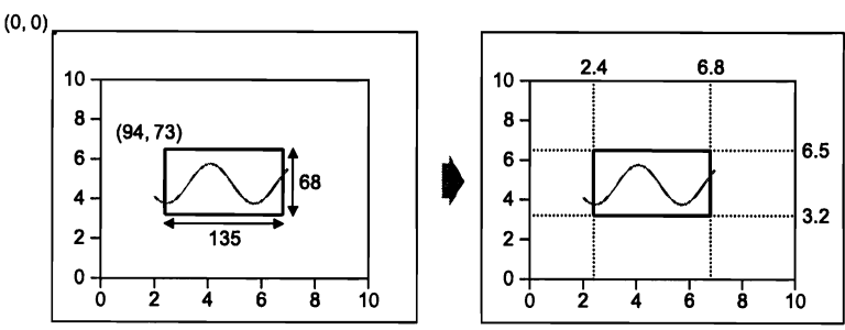
Рис. 5.10. Преобразование прямоугольника резиновой ленты из системы координат виджета в систему координат построителя графиков
