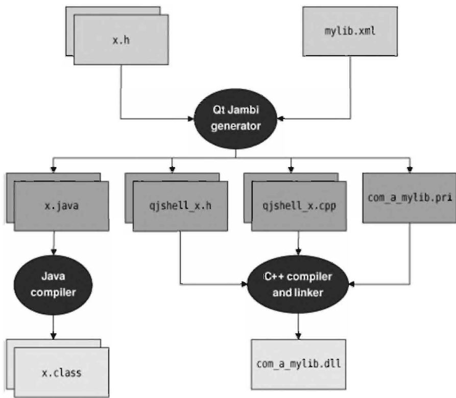
Рис. В.4. Создание классов C++, доступных в Qt Jambi
