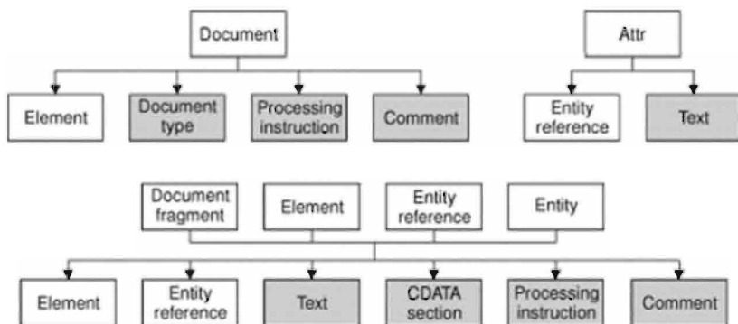
Рис. 16.3. Родственные связи между узлами DOM
