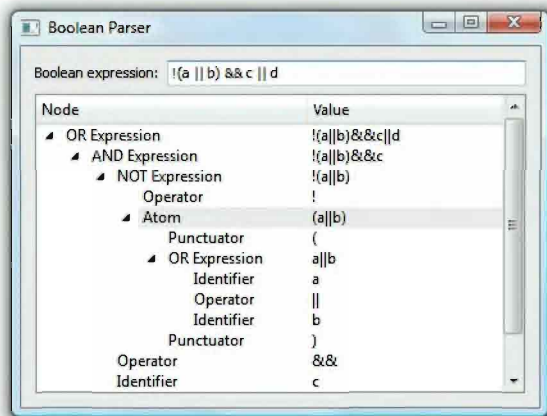
Рис. 10.14. Приложение Парсер булевых выражений
