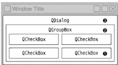
Рис. 7.2. Передача события в диалоговом окне
