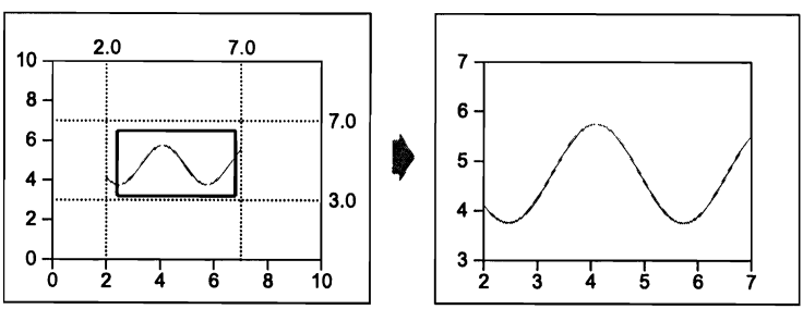
Рис. 5.11. Настройка прямоугольника резиновой ленты в системе координат построителя графиков и увеличение изображения
