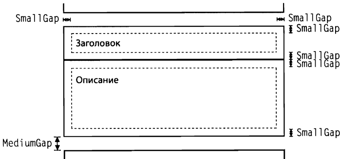
Рис. 8.20. Компоновка элементов справочника цветов на странице
