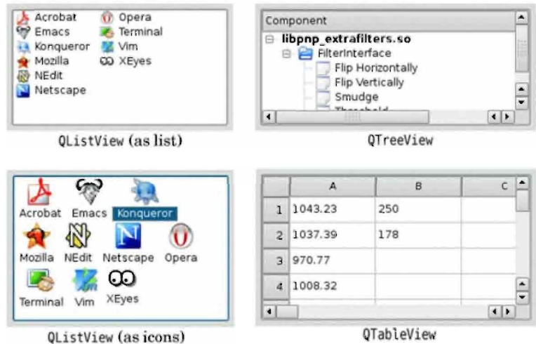
Рис. 2.20. Виджеты для просмотра списков объектов
