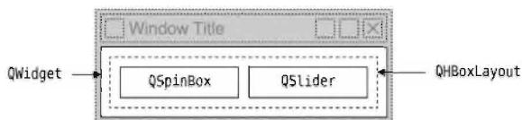
Рис. 1.7. Виджеты приложения Age и компоновка
