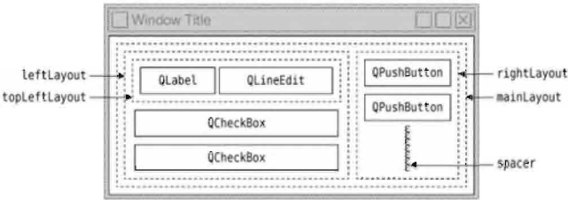
Рис. 2.2. Менеджеры компоновки диалогового окна поиска данных
