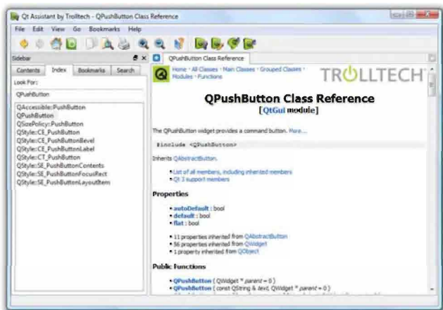
Рис. 1.8. Просмотр документации Qt программой Qt Assistant в системе Windows Vista
