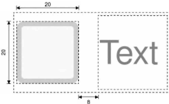
Рис. 19.3. Задание размера индикатора QCheckBox
