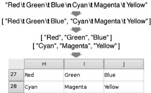
Рис. 4.6. Вставка текста из буфера обмена в электронную таблицу
