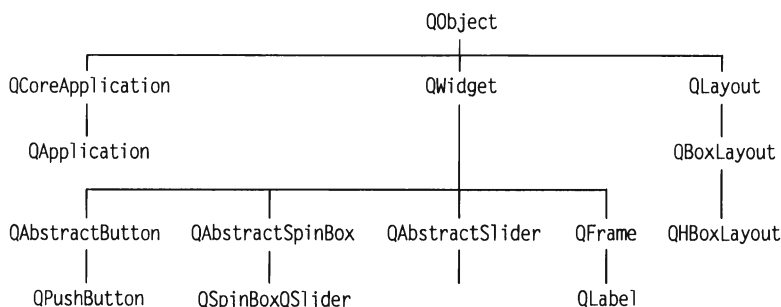
Рис. 1.9. Дерево наследования для классов, используемых в данной главе
