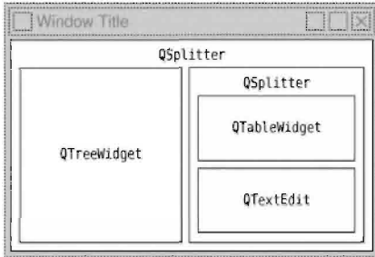
Рис. 6.10. Компоновка разделителя в приложении Mail Client
