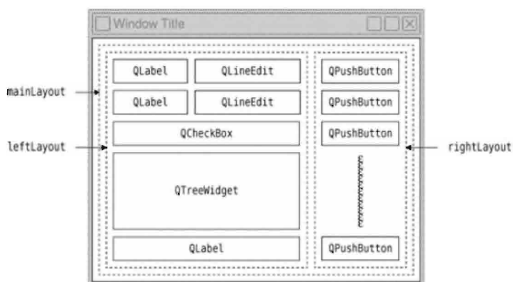
Рис. 6.3. Компоновка диалогового окна Find File
