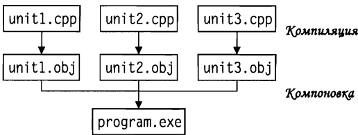
Рис. Г.1. Процесс компиляции программы на C++ (в Windows)
