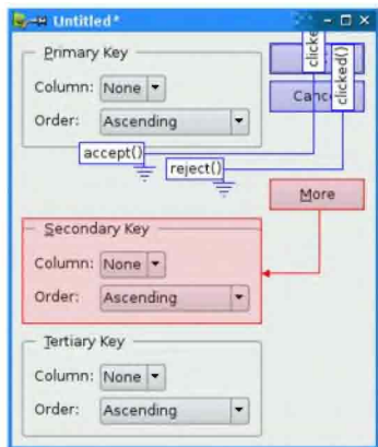
Рис. 2.15. Соединение виджетов формы
