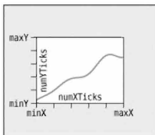
Рис. 5.8. Переменные-члены настроек графика PlotSettings
