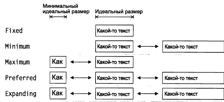
Рис. 6.4. Смысл различных политик размеров
