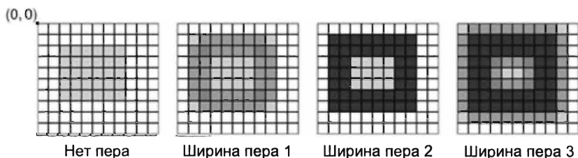
Рис. 8.8. Результат выполнения команды drawRect(2, 2, 6, 5) с включенным режимом сглаживания линий
