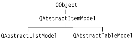
Рис. 10.11. Дерево наследования для абстрактных классов моделей
