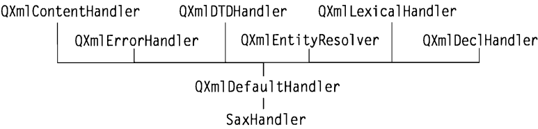
Рис. 16.4. Дерево наследования SaxHandler
