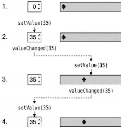
Рис. 1.5. Изменение значения в одном из виджетов приводит к изменению значения в другом виджете
