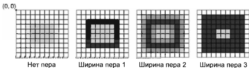
Рис. 8.9. Результат выполнения команды drawRect(2.5, 2.5, 6, 5) с включенным режимом сглаживания линий
