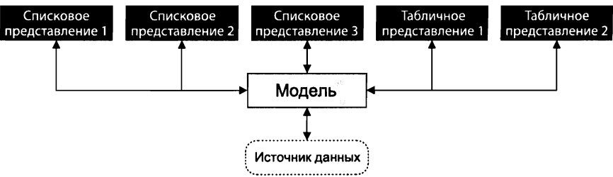
Рис. 10.2. Одна модель может обслуживать несколько представлений
