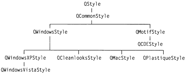
Рис. 19.16. Дерево наследования для встроенных стилей Qt
