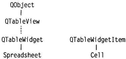
Рис. 4.1. Деревья наследования для классов Spreadsheet и Cell
