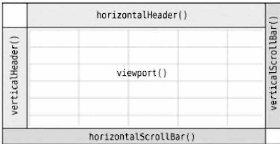
Рис. 4.2. Виджеты, составляющие QTableWidget
