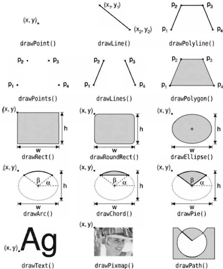
Рис. 8.1. Часто используемые функции draw...() рисовальщика QPainter
