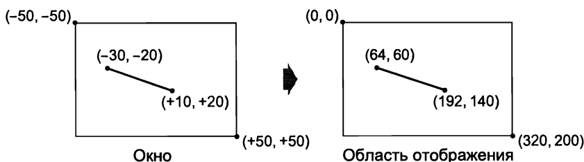
Рис. 8.10. Преобразование логических координат в физические
