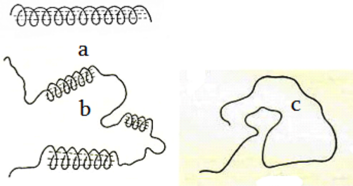
5.6. Պարույր- կծիկ անցումների եզրային կոնֆիգուրացիոն վիճակները: a -հղեալական \alpha -պարույր, b -միջանկյալ վիճակ, c -վիճակագրական կծիկ
