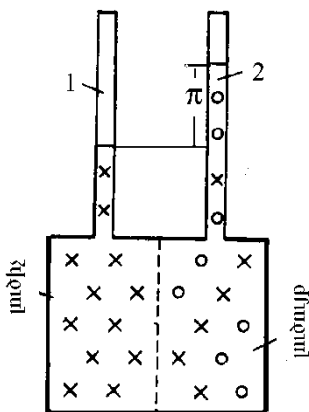
4.2. Օսմոսաչափի սկզբունքային սխեման
