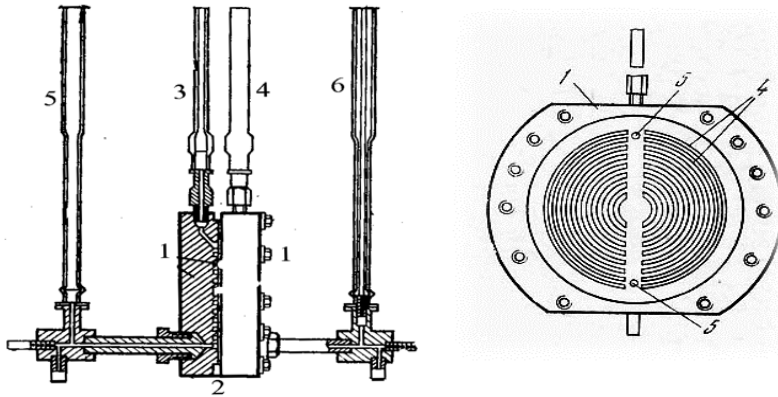
4. 6. Ֆուսսի և Միդդի օսմոսաչափի սխեման
