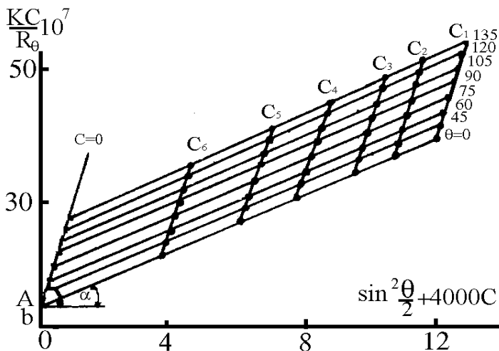
6.10. Ձխմի դիագրամը պոլիստիրոլի բենզոլային լուծույթի համար
