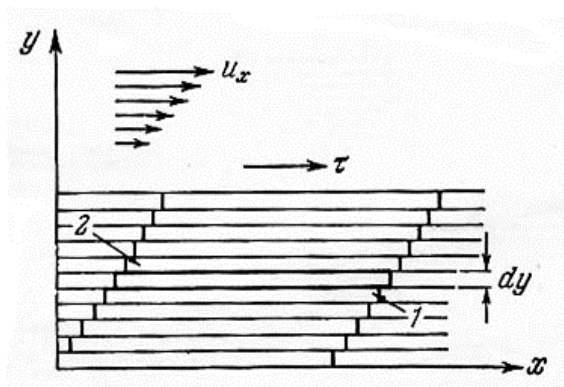
5.1. Հեղուկի լամինար հոսքը
