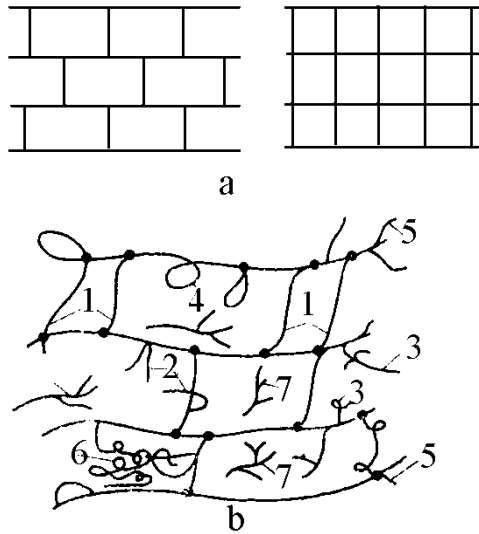
7.2. Կարված կառուցվածքների տեսակները. a -կատարյալ ցանցեր; b -իրական ցանցեր; 1-ակտիվ շղթաներ; 2-ոչ ակտիվ շղթաներ; 3-փոքր ճյուղավորումներ; 4-օղակներ; 5-կարճ ազատ ծայրեր; 6-խճճումներ; 7-զուլ ֆրակցիա
