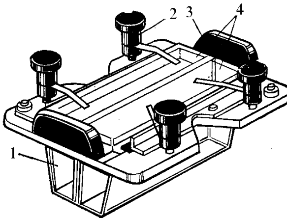
8.6. ИТП-2 ինտերֆերոմետրի կյուվետը
