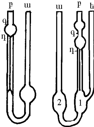
5.9. Օստվալդի (ձախում) և Ուբբեղդեի (աջում) մածուցիկաչափերը
