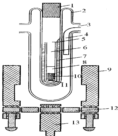
5.10. Ջիմմի մածուցիկաչափի սխեման: 1-խցան, 2-ջերմակայունացնող շապիկ, 3-ջերմակայունացնող հեղուկ, 4. Ջերմակայունացնող հեղուկի մուտք, 5-մագանթ, 6-ռոտոր, 7-ստատոր, 8-կարգավորման գիծ, 9-բևեռ, 10-խճողակ, 11-պողպատե ձողիկ, 12-մագնիս, 13-խառնիչի շարժիչ
