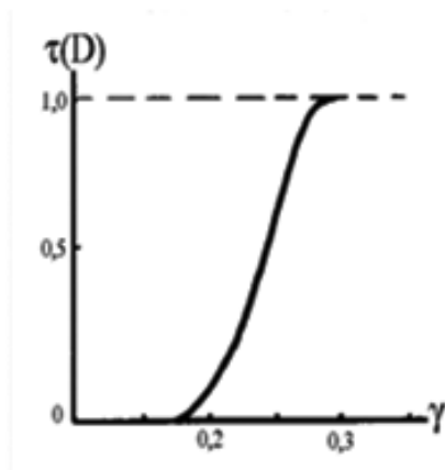
3.2. Պոտորաչաձական տիտրման կորը
