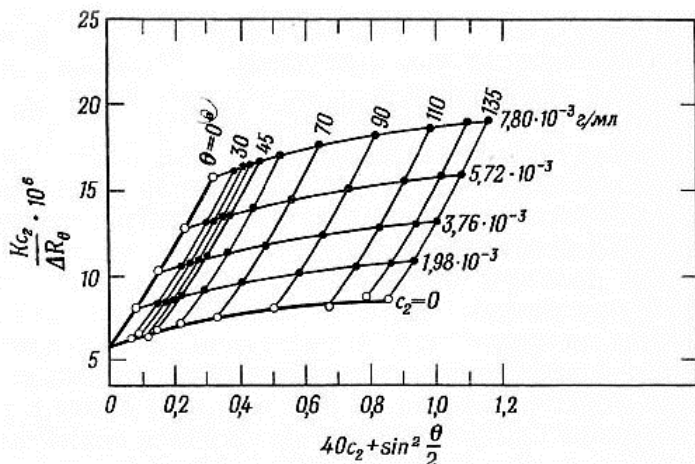
6.6 Կրկնակի էքստապոլացման գրաֆիկը պոլիստիրոլի համար բենզոլում
