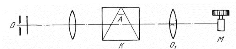
6.7. Լուծույթի բեկման ցուցիչի ինկրեմենտի ճշգրիտ որոշումը «հեղուկ պրիզմայի» օգտագործմամբ
