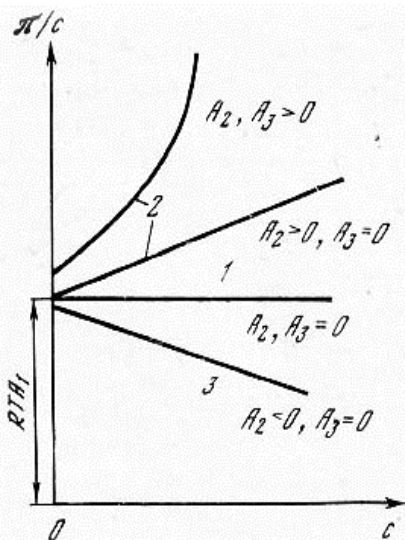
4.3. \pi / C = f(C) կախումը A_2 -ի և A_3 -ի տարբեր արժեքների դեպքում:
