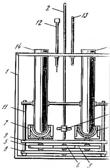
Նկ 4.9. Կաշալսկու կրիոսկոպը
