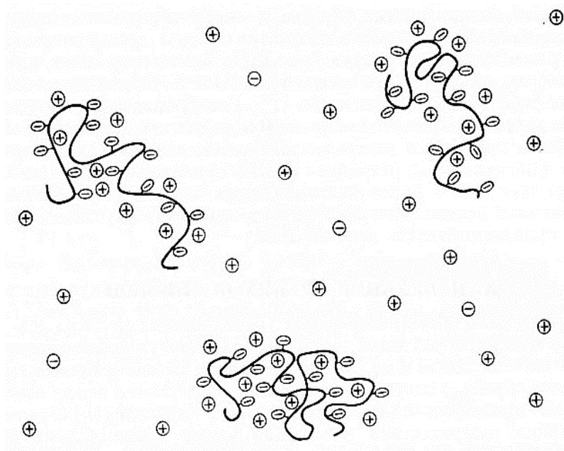
5.5. Իոնների բաշխման սխեմա ճկուն շղթայական մակրոմոլեկուլներ և քիչ քանակող 1:1 էլեկտրոլիտ պարունակող պոլիթթվային լուծույթում
