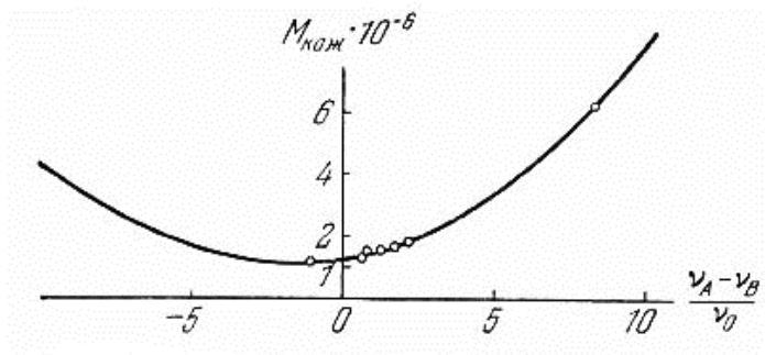
6.12. Ստիքոլ – մեթիլմետակրիլատ սոպոլիմերի չափված մոլեկուլային զանգվածի կախումը (\mathbf{v}_A - \mathbf{v}_B) / \mathbf{v}_0 -ի արժեքից
