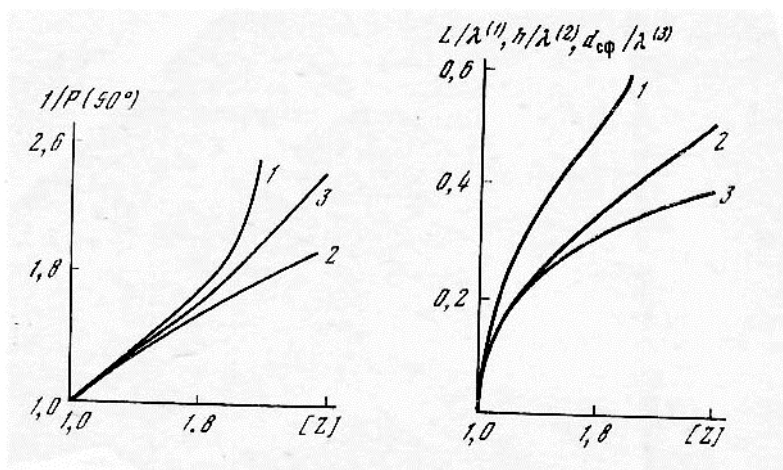
6.5. Ներքին ինտերֆերենցիայի ֆակտորի կախումը լուսացրման ասիմետրիայից ձողաձև (1) գնդաձև (2) և կծիկաձև (3) մասնիկների համար
