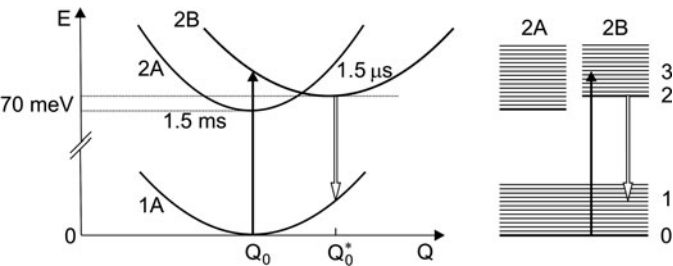
Fig. 15.4 Alexandrite laser
