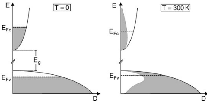
Fig. 21.5 Quasi-Fermi energies
