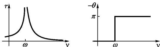
Рис. 185. Амплитуда и фаза маятника без трения как функция частоты внешней силы
