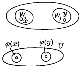
Рис. 234. Отделимость
