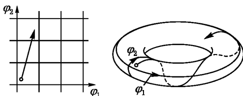
Рис. 174. Обмотка тора
