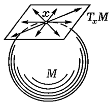
Рис. 49. Касательное пространство
