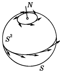
Рис. 258. Поле скоростей
