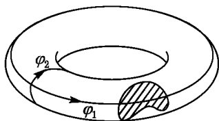
Рис. 172. Тор
