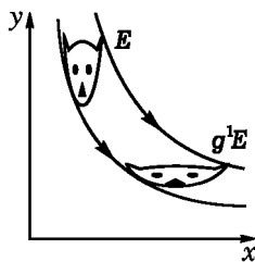
Рис. 47. Гиперболический поворот
