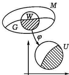
Рис. 239. Открытое подмножество
