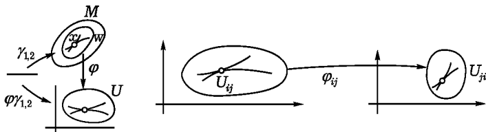
Рис. 248. Касательный вектор
