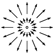
Рис. 61. Эйлерово поле
