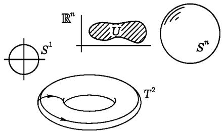
Рис. 231. Примеры многообразий
