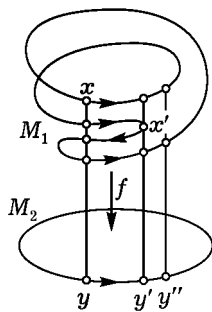
Рис. 271. Отображение степени 2
