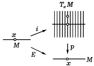
Рис. 251. Касательное расслоение
