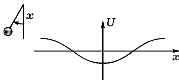
Рис. 92. Потенциальная энергия маятника
