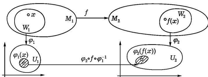
Рис. 242. Дифференцируемое отображение
