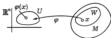
Рис. 232. Карта
