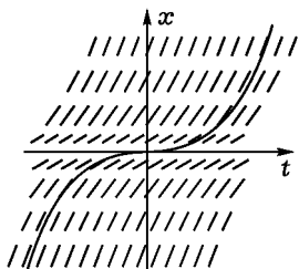
Рис. 27. Пример неединственности
