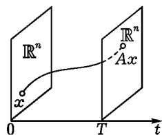
Рис. 205. Отображение монодромии
