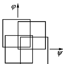
Рис. 236. Атлас тора
