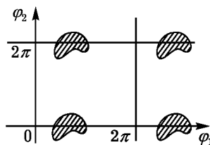
Рис. 173. Карта тора
