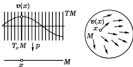
Рис. 257. Векторное поле
