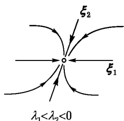
Рис. 133. Устойчивые узлы
