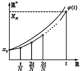
Рис. 111. Ломаная Эйлера
