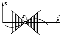
Рис. 29. Условие Липшица
