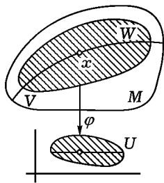
Рис. 246. Подмногообразие
