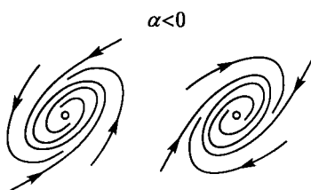
Рис. 136. Устойчивые фокусы
