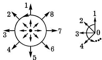
Рис. 262. Кривая индекса 1
