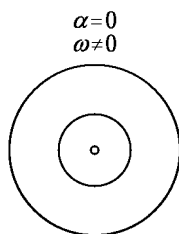
Рис. 125. Центр
