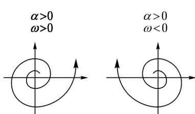
Рис. 124. Неустойчивые фокусы
