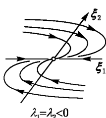
Рис. 133. Устойчивые узлы
