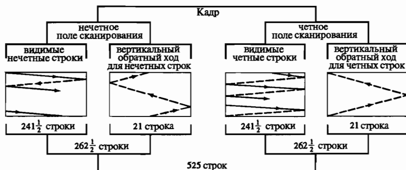
Рис. 1-35 Схема 525-строчного стандартного кадра.
