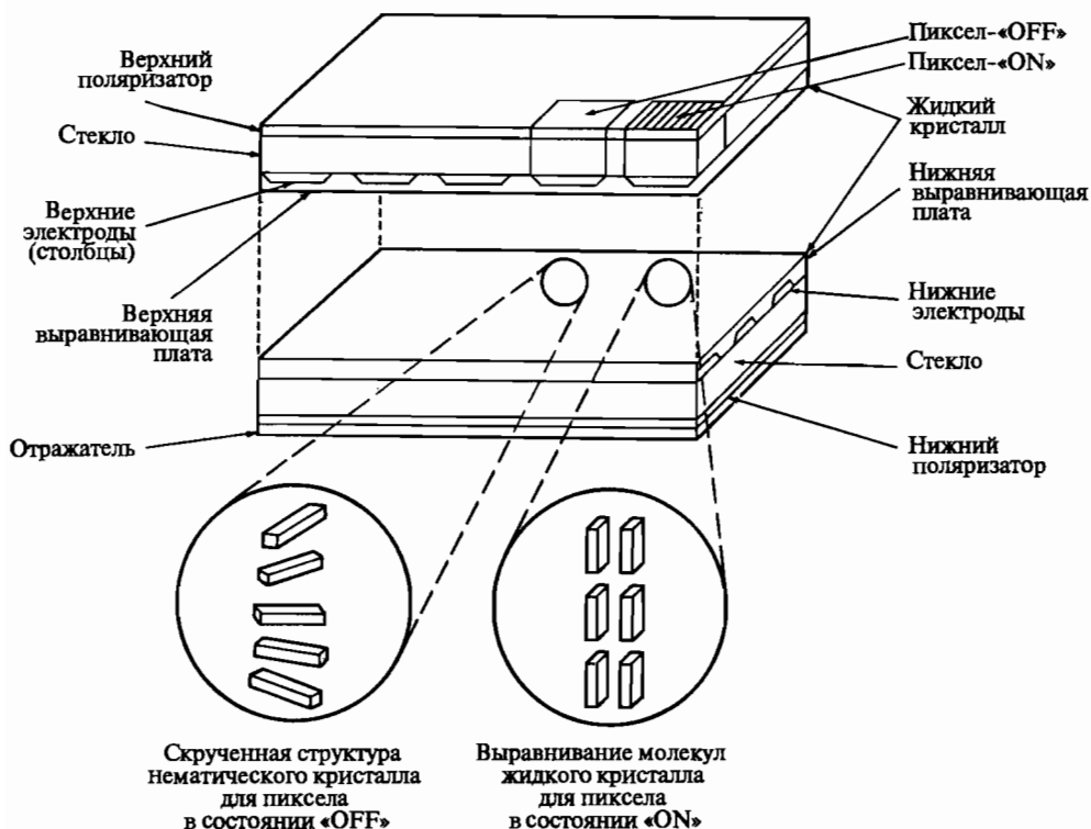
Рис. 1-42 Принципиальная схема дисплея на скрученных нематических жидких кристаллах.
