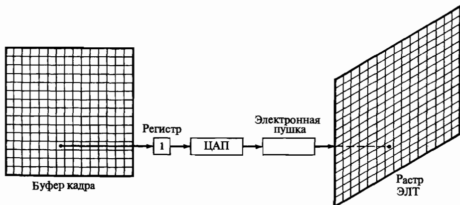
Рис. 1-24 Черно-белый буфер кадра (с одной битовой плоскостью) для растрового графического устройства.
