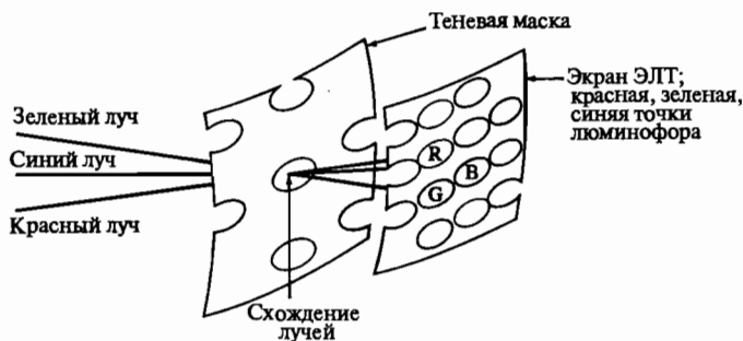
Рис. 1-33 Расположение электронной пушки и теневой маски цветной ЭЛТ.
