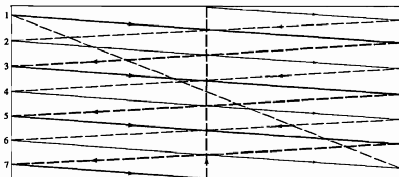
Рис. 1-34 Схема чересстрочной развертки для раstra из семи строк. Нечетное поле начинается со строки 1. Штриховой линией обозначен горизонтальный обратный ход луча. Вертикальный обратный ход луча для нечетного поля начинается внизу в центре, а для четного поля — внизу справа.
