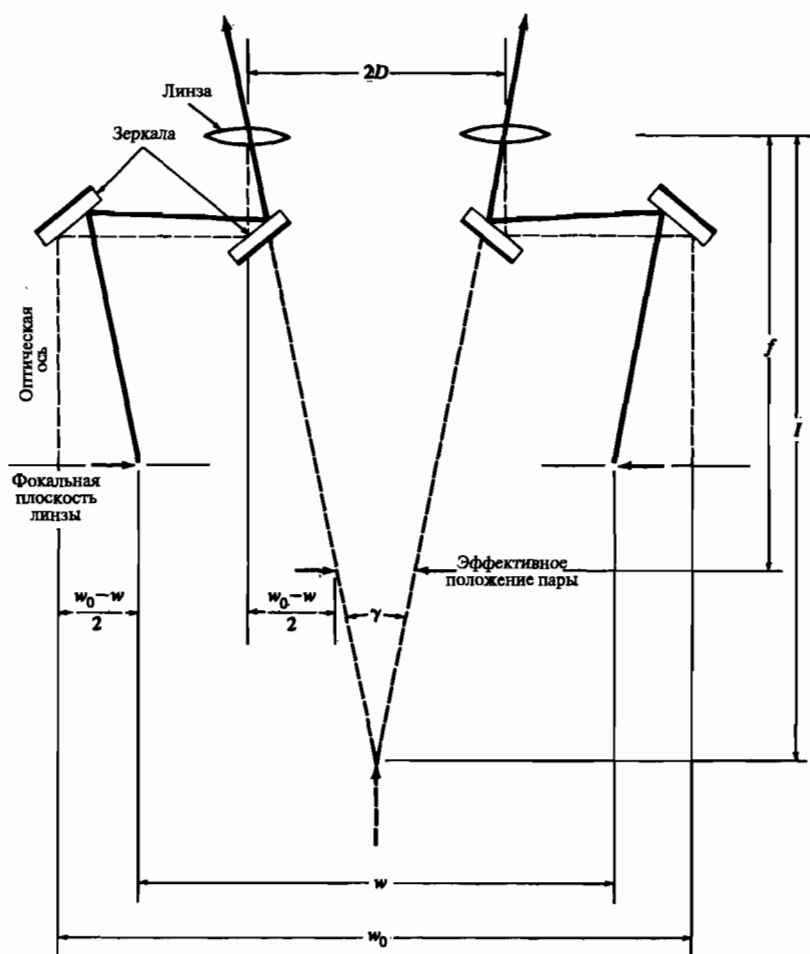
Рис. 3-46 Схема зеркального стереоскопа.
