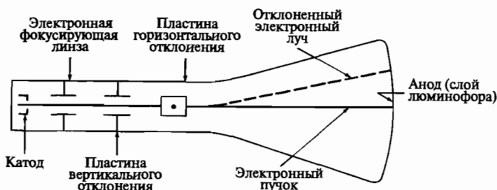
Рис. 1-31 Электронно-лучевая трубка.
