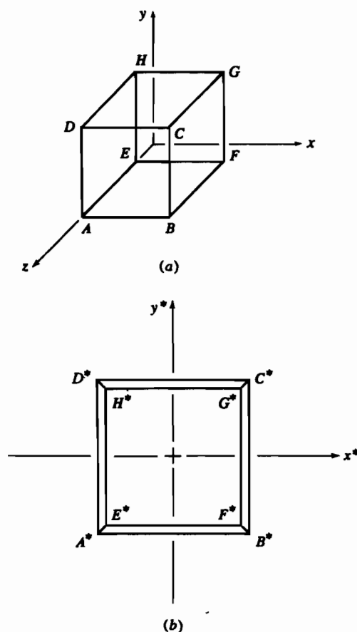
Рис. 3-29 Одноточечная перспективная проекция центрированного единичного куба.
