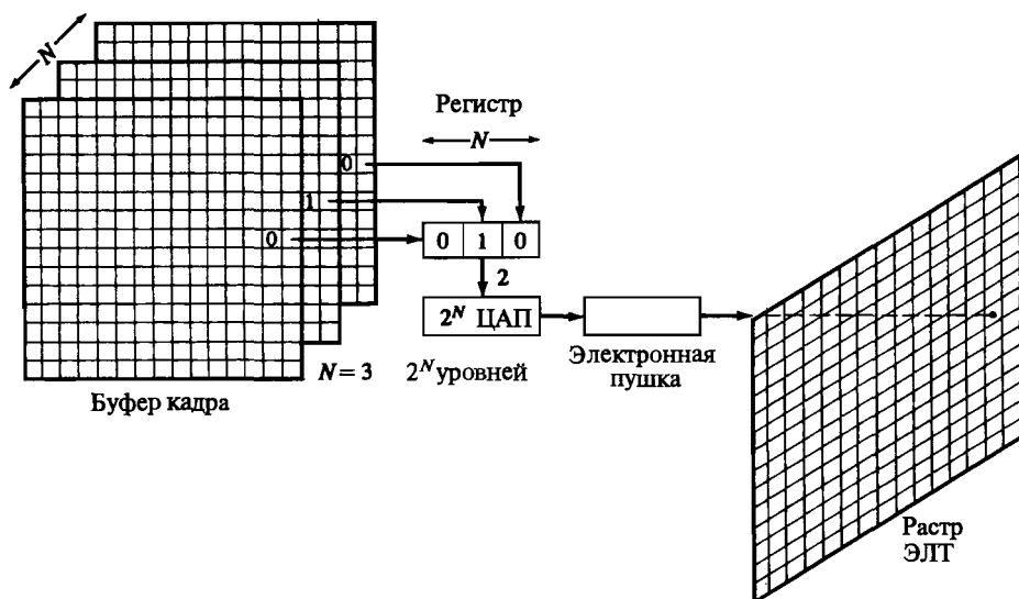
Рис. 1-25 Полутонный черно-белый буфер кадра с N битовыми плоскостями.
