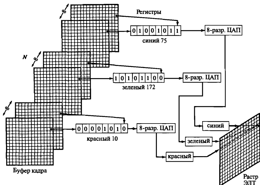
Рис. 1-28 Цветовой буфер кадра с 24 битовыми плоскостями.
