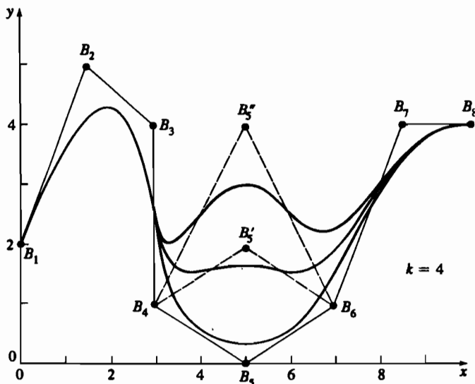
Рис. 5-43 Локальная коррекция В-сплайна.
