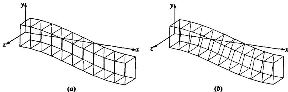
Рис. 6-17 Прямоугольник перемещается вдоль направляющей кривой. (а) Нормаль направлена как ось x ; (б) нормаль направлена так же, как касательная к направляющей кривой.
