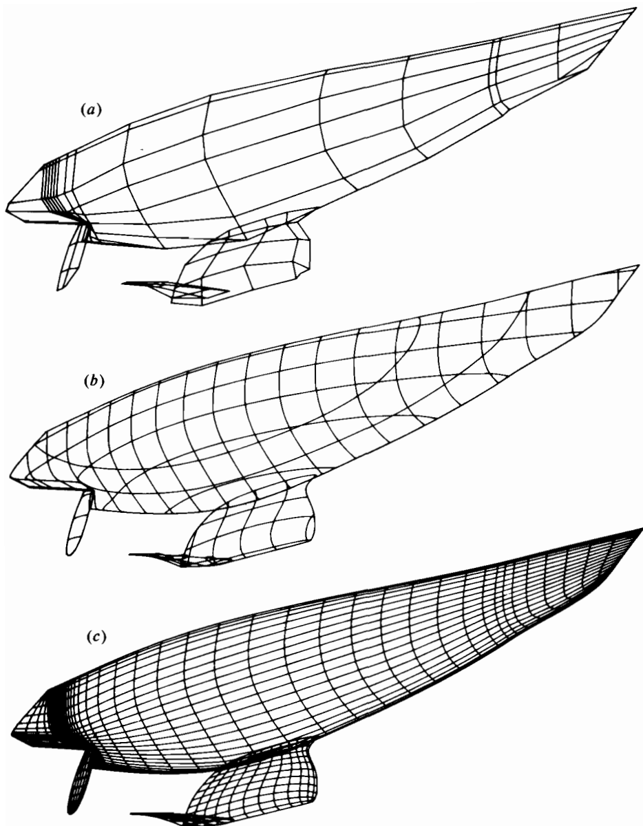
Рис. 1. Американская яхта класса Stars & Strips в форме В-сплайн поверхности, определяемой (а) сеткой многоугольников; (б) телом корпуса, хвостовой частью и ватерлинией; (с) параметрической сеткой. (С разрешения Джорджа Хейзена.)
