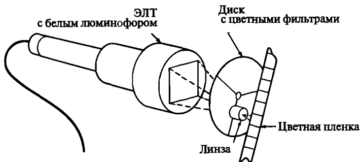
Рис. 1-62 Принципиальная схема цветной камеры.
