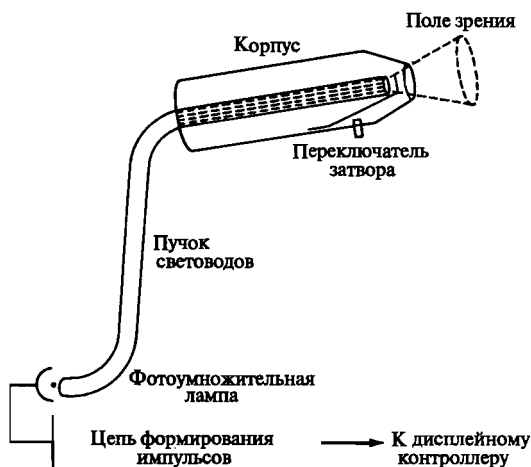
Рис. 1-14 Схема светового пера.
