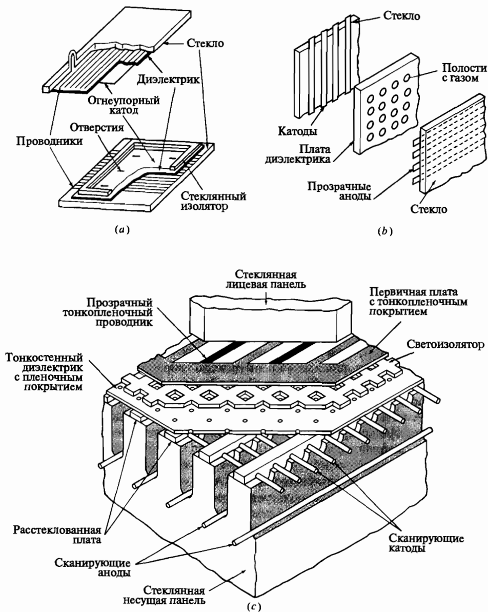
Рис. 1-38 Принципиальная схема плазменного газоразрядного дисплея: а) АС тип; б) DC тип; в) АС/DC тип.
