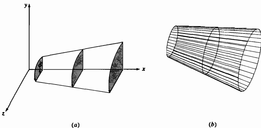
Рис. 6-2 Коническая поверхность вращения. (a) Схема построения; (b) результат.
