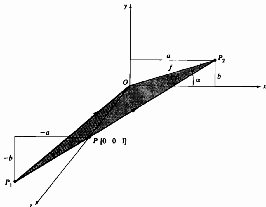
Рис. 3-21 Построение косоугольной проекции.
