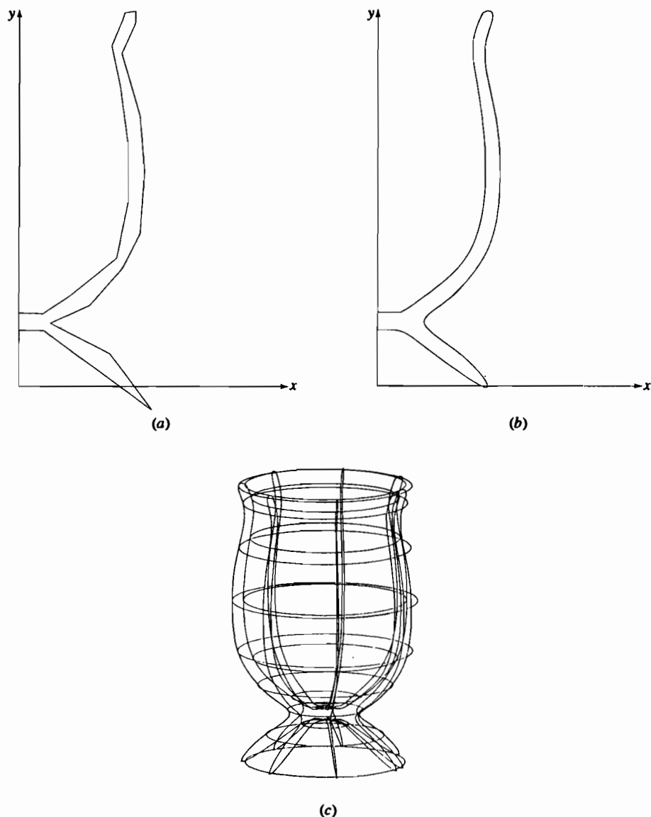
Рис. 6-10 В-сплайн поверхность вращения. (a) Вершины ломаной; (b) В-сплайн; (c) поверхность.
