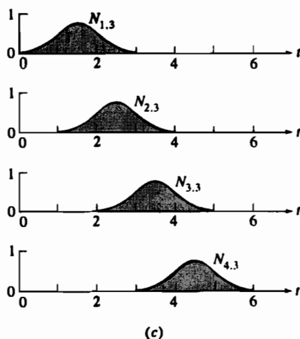
Рис. 5-39 Построение периодических базисных функций n+1=4 . (a) k=1 ; (b) k=2 ; (c) k=3 .
