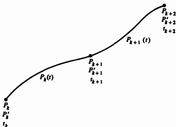
Рис. 5-7 Обозначения множества кусочно кубических сегментов сплайна.
