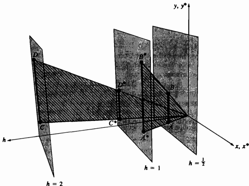
Рис. 2-15 Геометрическая интерпретация пропорционального масштабирования.
