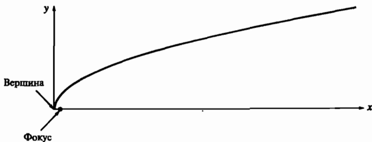
Рис. 4-9 Парабола.
