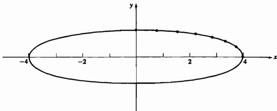
Рис. 4-7 Параметрическое представление эллипса.
