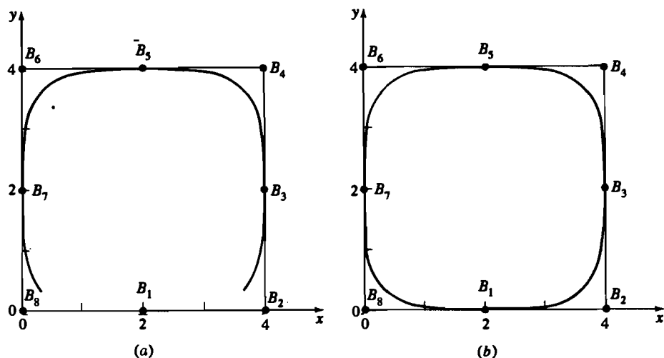
Рис. 5-46 Замкнутый периодический В-сплайн. (а) B_1 B_2 B_3 B_4 B_5 B_6 B_7 B_8 B_1 — определяющий многоугольник; (б) B_8 B_1 B_2 B_3 B_4 B_5 B_6 B_7 B_8 B_1 B_2 — определяющий многоугольник.
