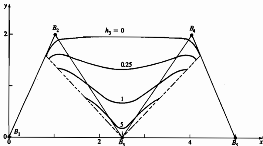
Рис. 5-64 Рациональные В-сплайны для n+1=5 , k=4 с периодическим узловым вектором [X] = [0 \ 1 \ 2 \ 3 \ 4 \ 5 \ 6 \ 7 \ 8] , [H] = [1 \ 1 \ h_3 \ 1 \ 1] .
