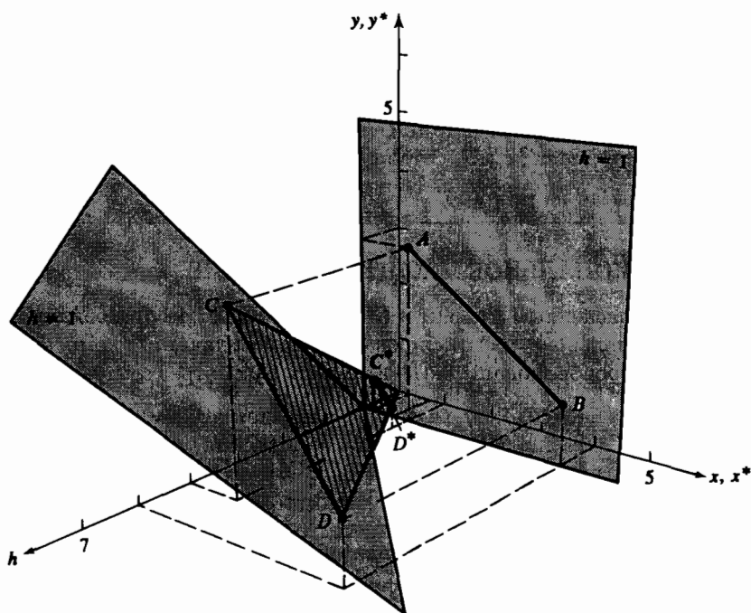
Рис. 2-14 Преобразование из физической плоскости ( h = 1 ) на плоскость h \neq 1 и проецирование обратно на физическую плоскость.
