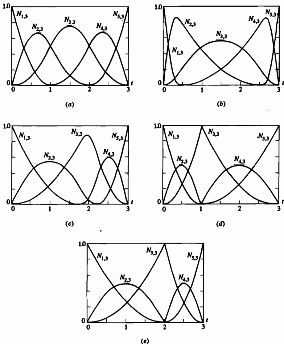
Рис. 5-38 Функции неравномерного базиса для n+1=5 , k=3 .
