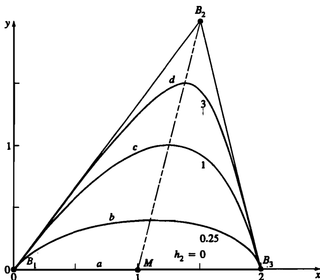
Рис. 5-67 Конические сечения, заданные рациональными В-сплайнами (кривыми Безье); (а) прямая линия, h_2 = 0 ; (б) эллипс, h_2 = 0.25 ; (с) парабола, h_2 = 1 ; (д) гипербола, h_2 = 3 .
