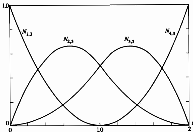
Рис. 5-37 Базисные функции открытого равномерного В-сплайна, [X] = [0 \ 0 \ 0 \ 1 \ 2 \ 2 \ 2] , k=3 , n+1=4 .
