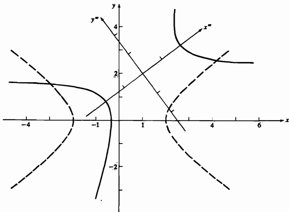
Рис. 4-16 Гипербола 2x^2 - 72xy + 23y^2 + 140x - 20y + 50 = 0 . Сплошная линия — заданная ориентация. Пунктир — стандартная ориентация.
