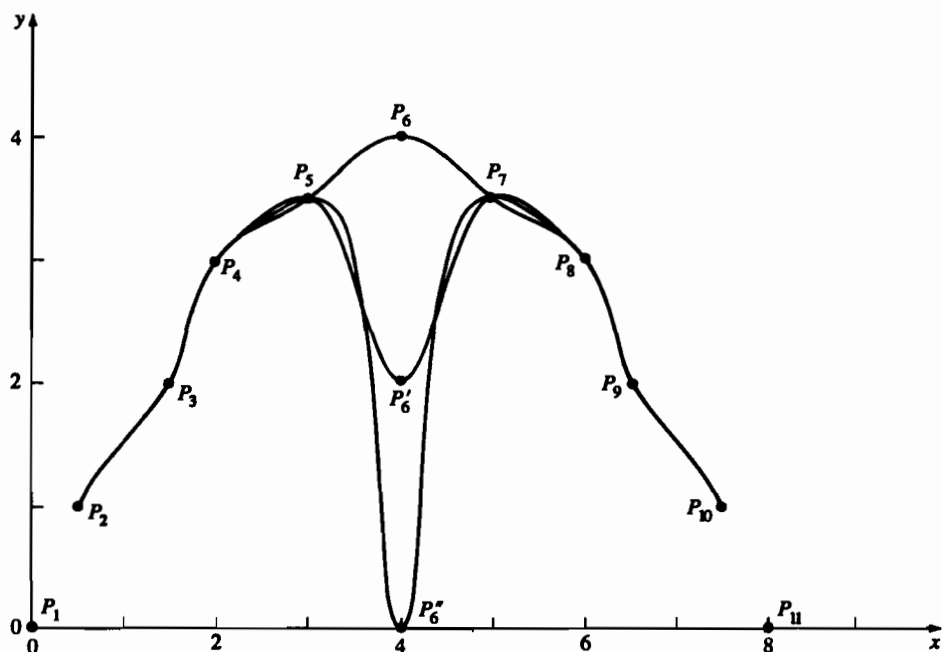
Рис. 5-24 Локальная коррекция параболически интерполированных кривых.
