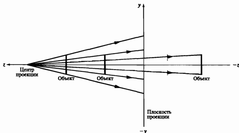
Рис. 3-33 Эффект масштабирования при перемещениях вдоль оси z для одноточечной перспективной проекции.
