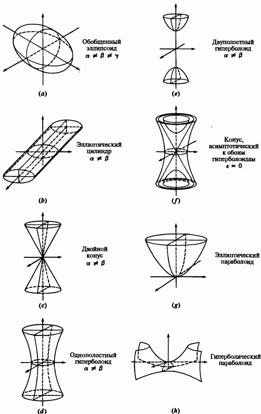
Рис. 6-18 Квадратичные поверхности. (a) Обобщенный эллипсоид \alpha \neq \beta \neq \gamma ; (b) эллиптический цилиндр \alpha \neq \beta ; (c) двойной конус \alpha \neq \beta ; (d) однополостный гиперболюд \alpha \neq \beta ; (e) двуполостный гиперболюд \alpha \neq \beta ; (f) конус, асимптотический к обоим гиперболюдам \kappa = 0 ; (g) эллиптический параболоид; (h) гиперболический параболоид.
