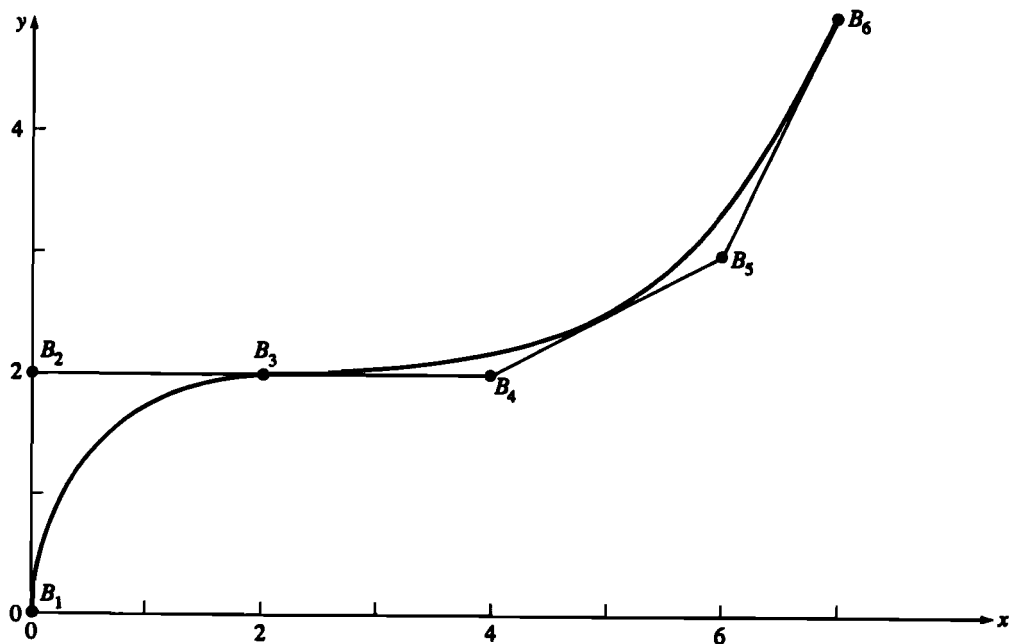
Рис. 5-70 Сопряжение рациональных В-сплайнов.
