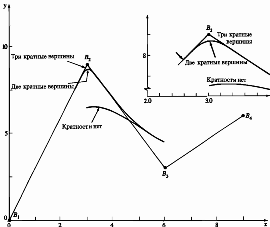
Рис. 5-45 Влияние кратности вершины на форму периодического В-сплайна, k = 4 .
