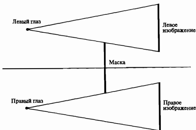
Рис. 3-42 Простой метод просмотра стереопар.
