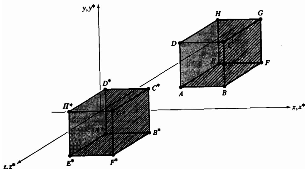
Рис. 3-4 Трехмерное отражение относительно плоскости xy .
