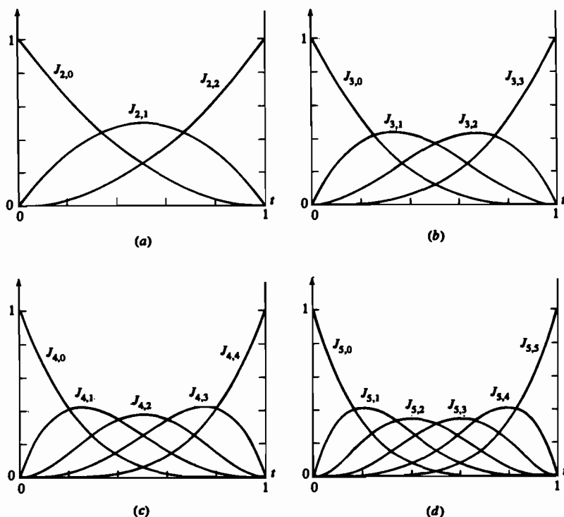
Рис. 5-27 Весовые функции Безье/Бернштейна. (а) Многоугольник из трех точек, n = 2 ; (б) из четырех точек, n = 3 ; (с) из пяти точек, n = 4 ; (д) из шести точек, n = 5 .
