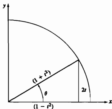
Рис. 4-4 Связь между параметрическими представлениями.
