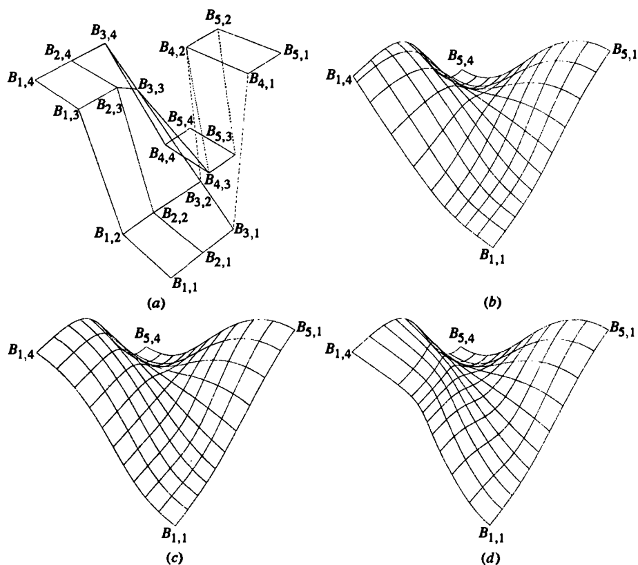
Рис. 6-53 Рациональные В-сплайн поверхности с n + 1 = 5 , m + 1 = 4 , k = l = 4 . (a) Характеристический многогранник; (b) h_{1,3} = h_{2,3} = 0 ; (c) h_{1,3} = h_{2,3} = 1 ; (d) h_{1,3} = h_{2,3} = 5 .
