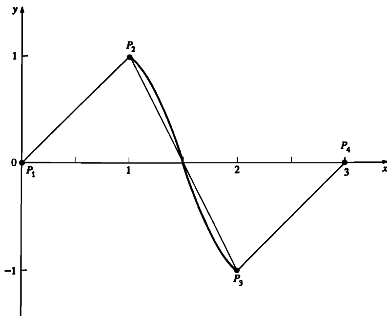
Рис. 5-21 Параболически интерполированная кривая для примера 5-5.
