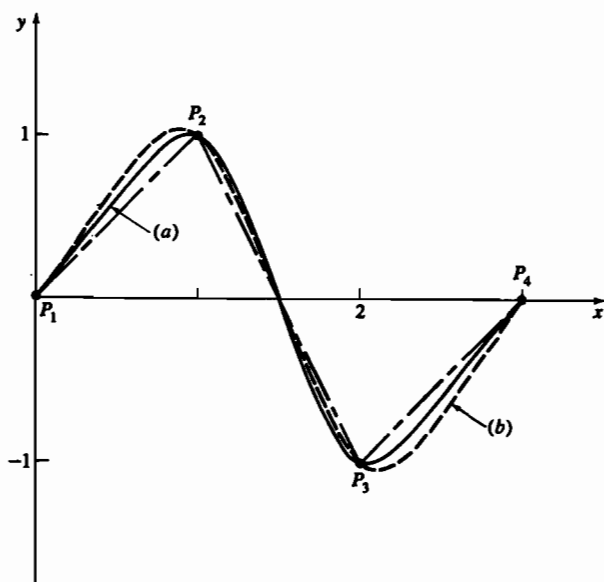
Рис. 5-9 Кусочный кубический сплайн. (а) t_k вычислены с помощью хордовой аппроксимации; (б) t_k нормализованы к 1.
