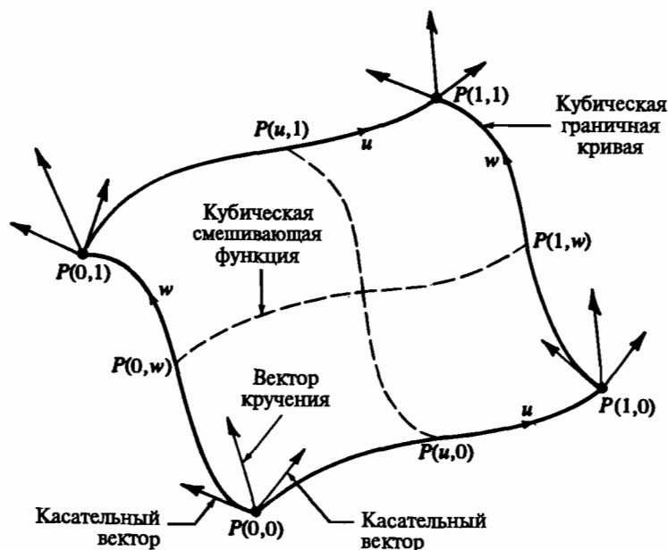
Рис. 6-31 Геометрия для куска бикубической поверхности Кунса.
