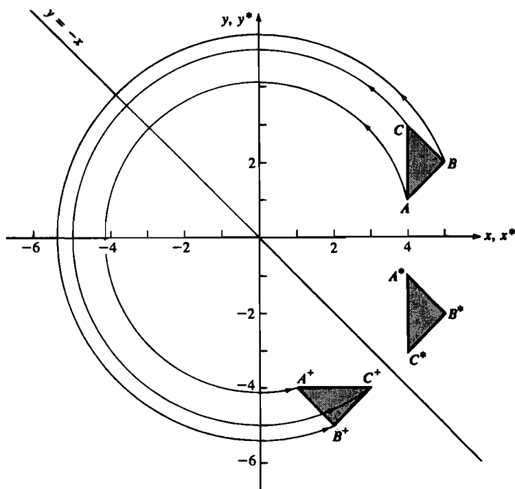
Рис. 2-7 Выполнение отражения путем поворота.
