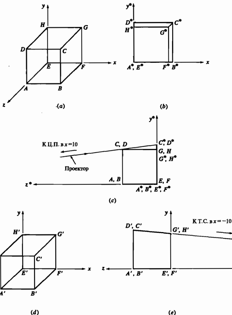
Рис. 3-28 Одноточечная перспективная проекция единичного куба.
