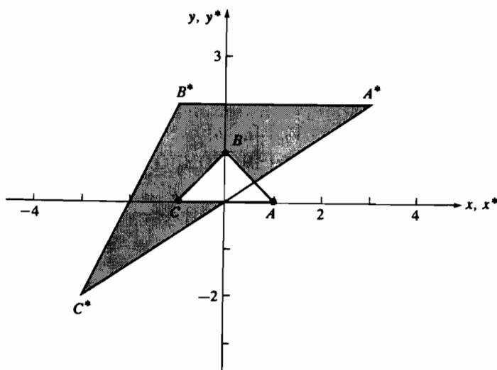
Рис. 2-12 Масштабирование области.
