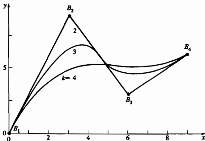
Рис. 5-41 Зависимость формы В-сплайна от его порядка.
