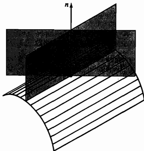
Рис. 6-27 Свойства линейчатой поверхности.
