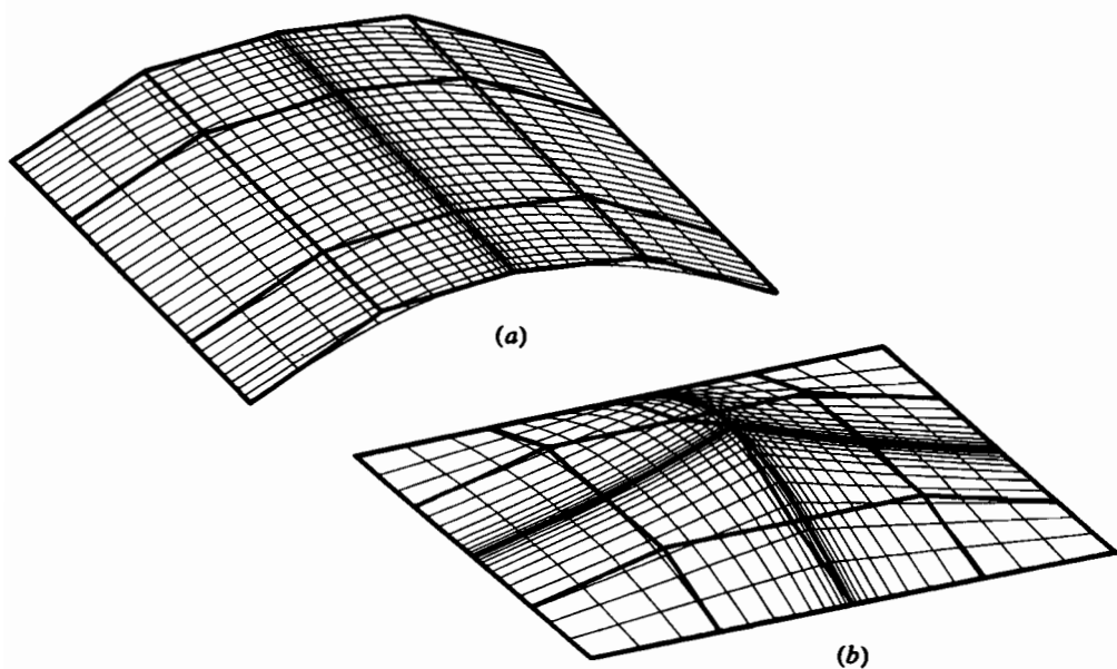
Рис. 6-43 В-сплайн поверхности четвертого порядка с несколькими совпадающими линиями сетки.
