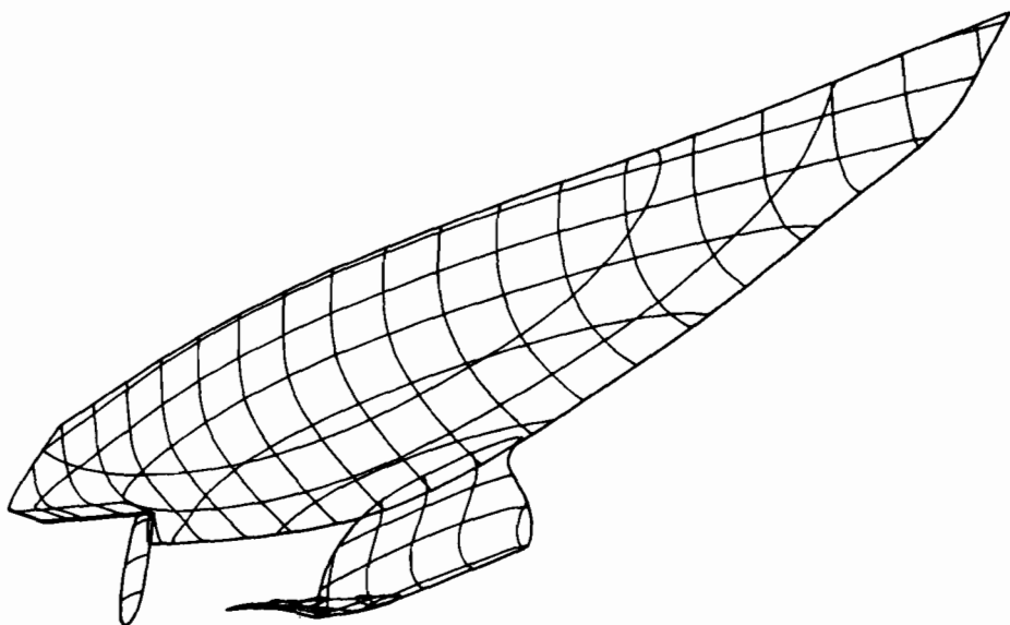
Рис. 5-1 Поверхность в виде сети ортогональных плоских кривых (Дж. Хейзен)
