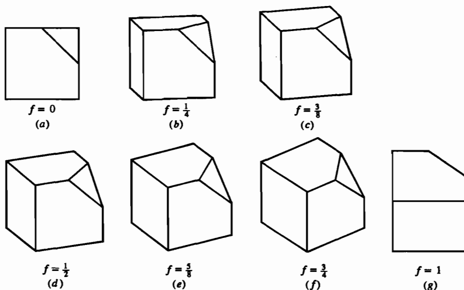
Рис. 3-17 Диметрические проекции для разных значений коэффициента искажения. (a) 0; (b) 1/4 ; (c) 3/8 ; (d) 1/2 ; (e) 5/8 ; (f) 3/4 ; (g) 1.
