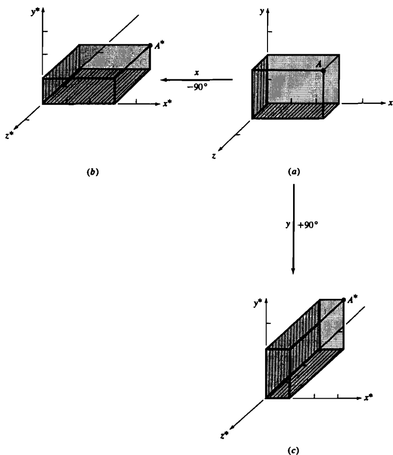
Рис. 3-2 Трехмерные повороты.
