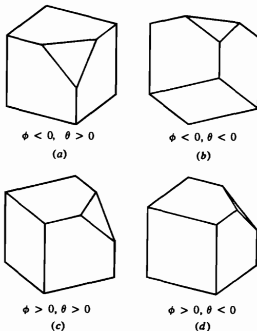
Рис. 3-18 Четыре возможных диметрических проекции для коэффициента искажения 5/8 и углов поворотов \phi = \pm 29.52^\circ, \theta = \pm 26.23^\circ . (a) \phi = -29.52^\circ, \theta = +26.23^\circ ; (b) \phi = -29.52^\circ, \theta = -26.23^\circ ; (c) \phi = +29.52^\circ, \theta = +26.23^\circ ; (d) \phi = +29.52^\circ, \theta = -26.23^\circ .
