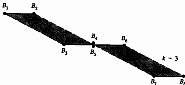
Рис. 5-34 Выпуклая оболочка для кратных вершин, k=3 .
