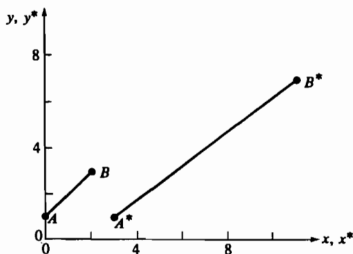
Рис. 2-2 Преобразование отрезков.
