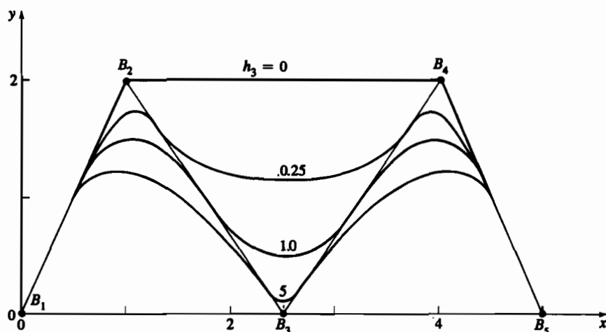
Рис. 5-62 Рациональные В-сплайны для n+1=5 , k=4 с периодическим узловым вектором [X] = [0 \ 1 \ 2 \ 3 \ 4 \ 5 \ 6 \ 7] , [H] = [1 \ 1 \ h_3 \ 1 \ 1] .
