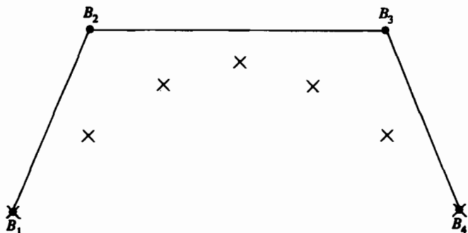
Рис. 5-55 Построение многоугольника В-сплайна для заданного множества точек.
