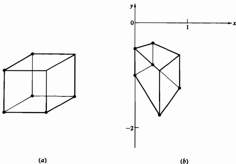
Рис. 3-50 Восстановление преобразования по перспективной проекции.
