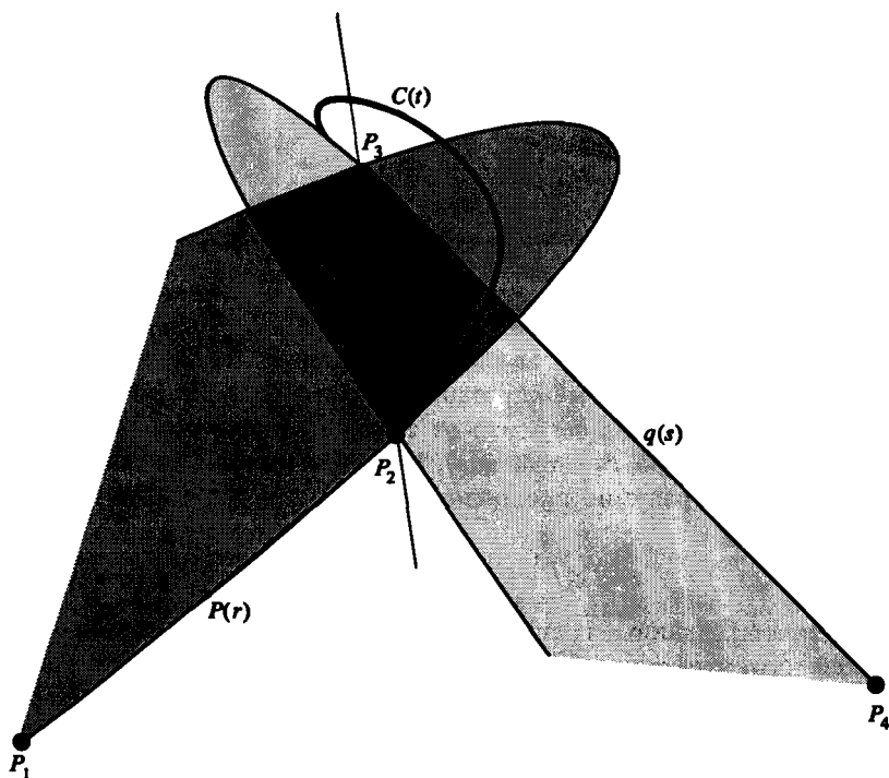
Рис. 5-18 Параболическая интерполяция.
