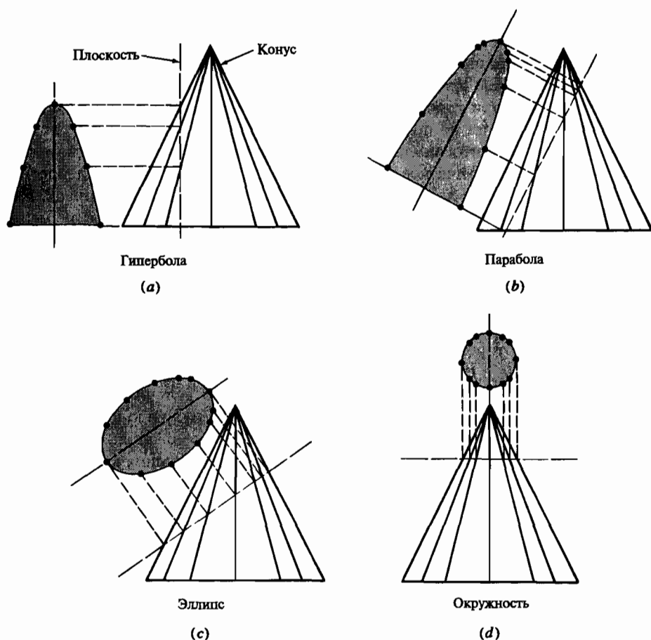
Рис. 4-2 Конические сечения.
