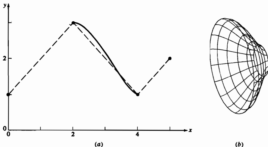
Рис. 6-9 Поверхность вращения из параболически интерполированной кривой. (а) Создание кривой; (b) поверхность.
