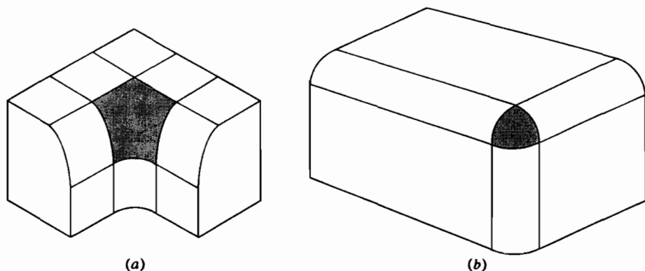
Рис. 6-36 Нечетырехугольные куски. (а) Пятиугольный; (б) треугольный.
