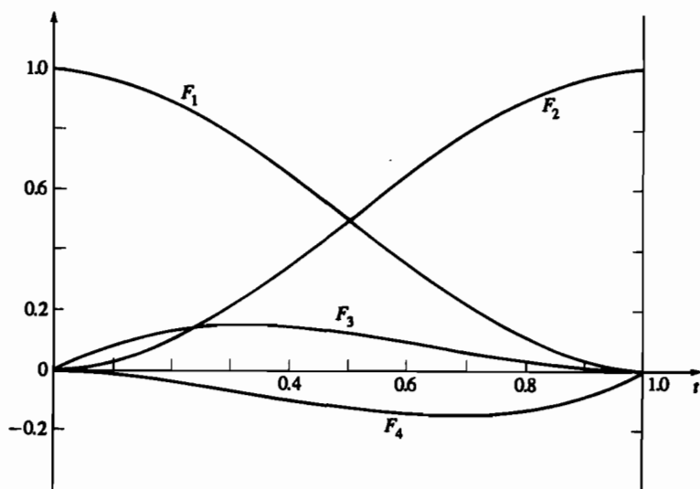
Рис. 5-8 Весовые функции кубического сплайна для t_{k+1} = 1.0
