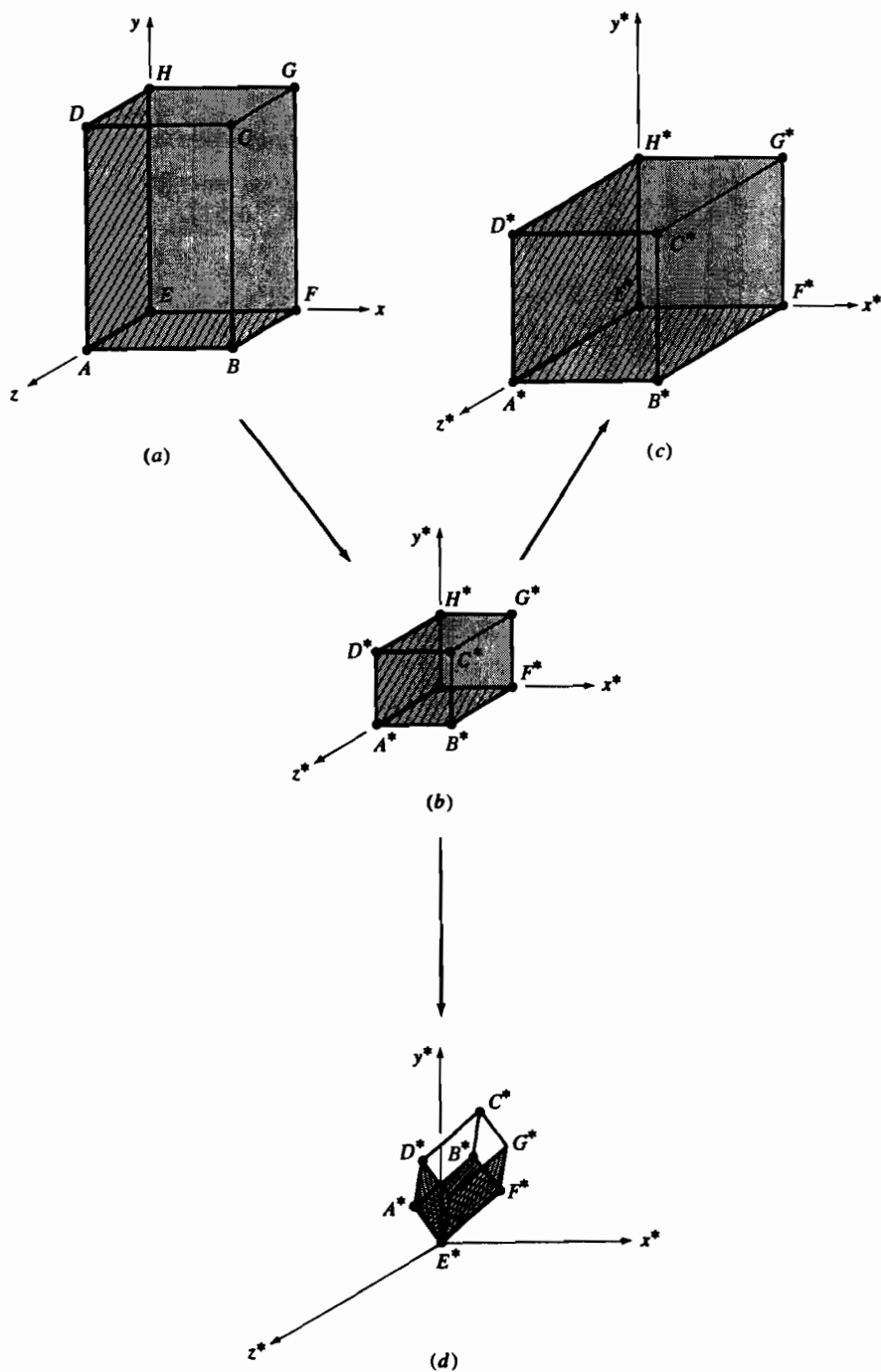
Рис. 3-1 Трехмерные масштабирования.
