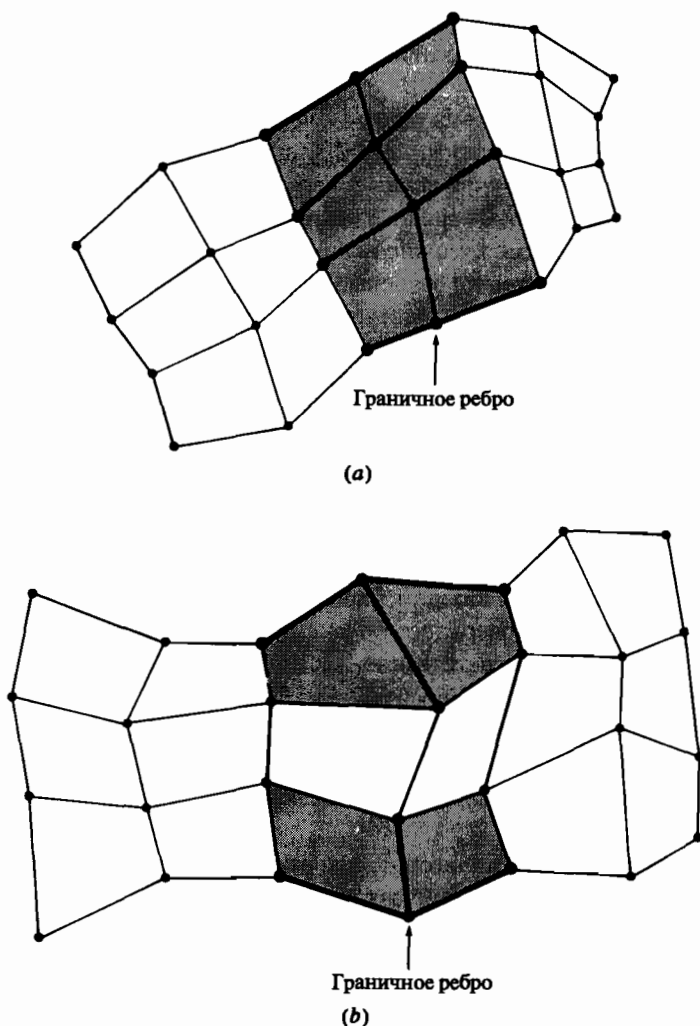
Рис. 6-41 Гладкость стыковки кусков поверхности Безье. (a) Линии сетки коллинеарны; (b) ребра ломаных некомпланарны.
