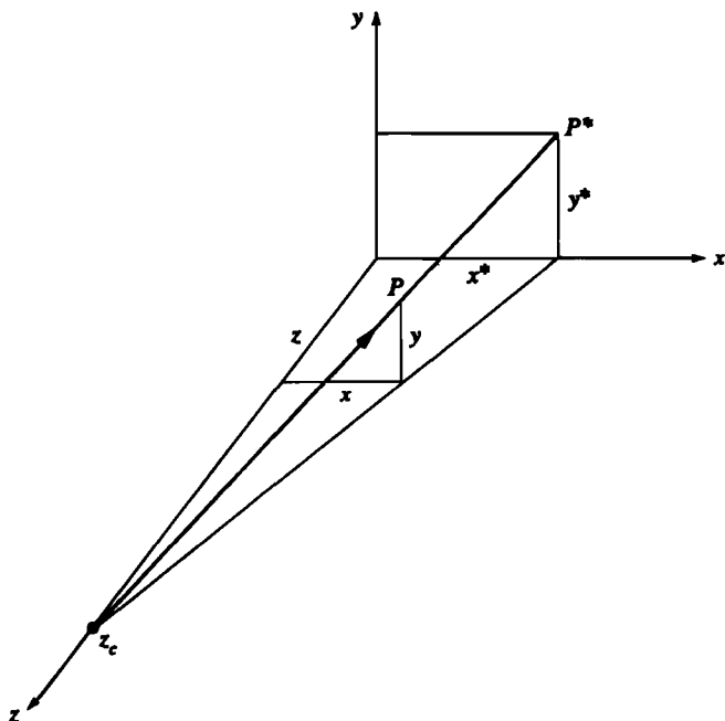
Рис. 3-26 Перспективная проекция точки.
