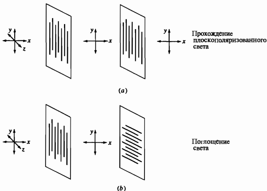
Рис. 1-41 Поляризация света: а) прохождение плоскополяризованного света; б) поглощение света.
