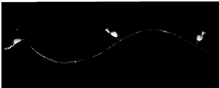
Рис. 5-4 Физические отвесы и сплайн.
