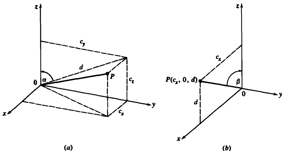
Рис. 3-7 Повороты, необходимые для совмещения с осью z единичного вектора OP . (а) Поворот вокруг x ; (б) поворот вокруг y .
