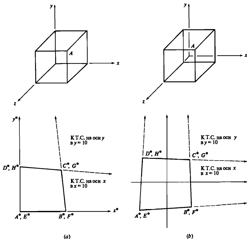
Рис. 3-30 Двухточечные перспективные проекции. (а) Нецентрированного куба; (б) центрированного куба.
