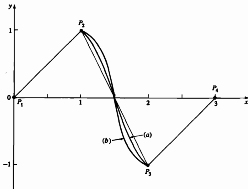
Рис. 5-23 Сравнение результатов параболической интерполяции. (a) Пример 5-5, \alpha = \beta = 1/2 ; (b) Пример 5-6, \alpha = 1 - \beta .
