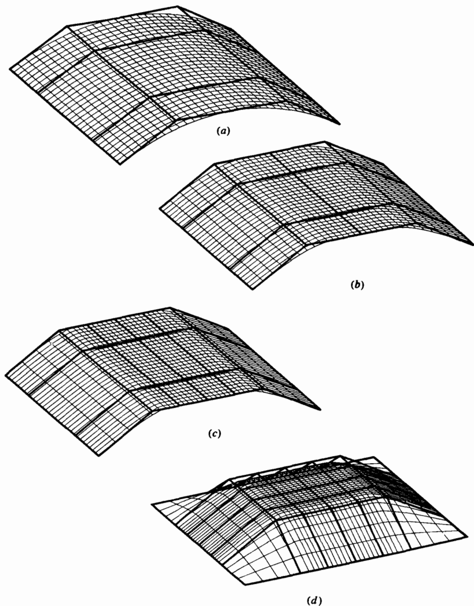
Рис. 6-42 В-сплайн поверхности третьего порядка. (а) Гладкая линейчатая поверхность; (б) небольшая внутренняя плоская область, вызванная коллинеарностью трех вершин сетки в u направлении; (с) обширная внутренняя плоская область, вызванная коллинеарностью пяти вершин сетки в u направлении; (д) плоская область внутри скульптурной поверхности.
