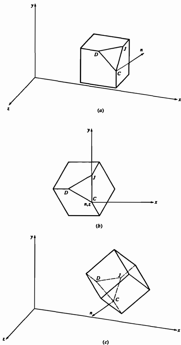
Рис. 3-9 Отражение относительно произвольной плоскости.
