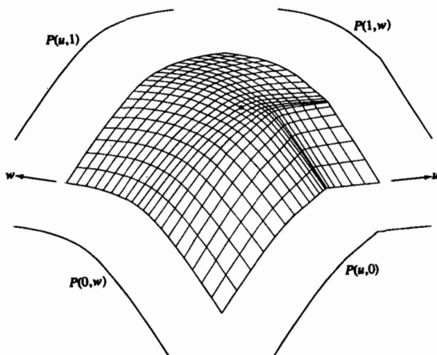
Рис. 6-30 Линейная поверхность Кунса.
