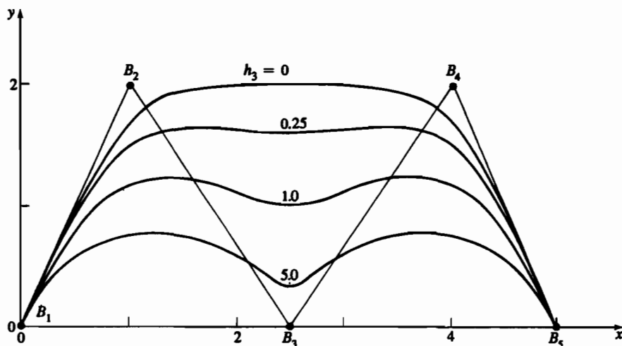
Рис. 5-60 Рациональные В-сплайны для n+1=5 , k=4 с открытым узловым вектором [X] = [0 \ 0 \ 0 \ 0 \ 1 \ 2 \ 2 \ 2 \ 2] , [H] = [1 \ 1 \ h_3 \ 1 \ 1] .
