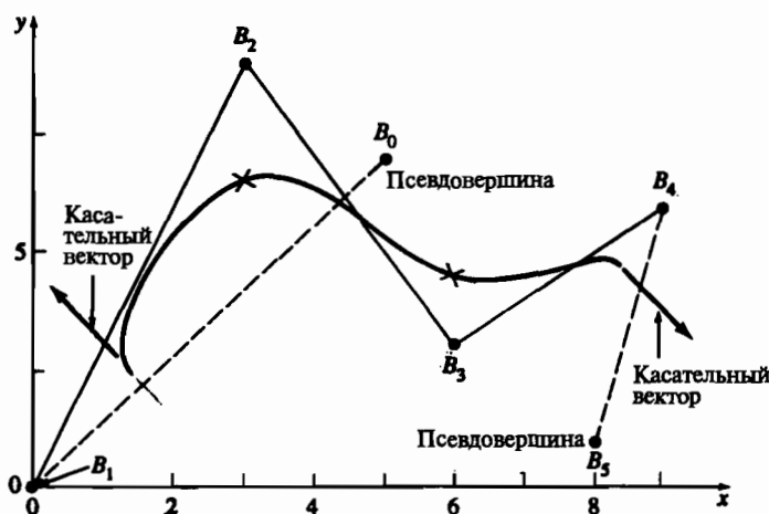
Рис. 5-54 Управление касательным вектором для периодического В-сплайна, k = 4 .
