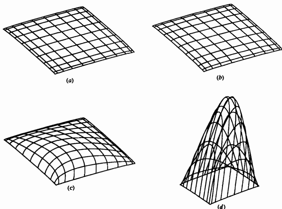
Рис. 6-35 Влияние вектора кручения на кусок бикубической поверхности. Значение компоненты вектора кручения в точке P(0,0) равно (a) 10; (b) 100; (c) 1000; (d) 10000.
