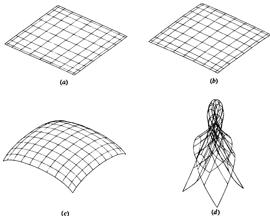
Рис. 6-33 Действие на кусок бикубической поверхности варьирования величины касательного вектора. Значения компонент касательного вектора равны (a) 1; (b) 10; (c) 100; (d) 1000.
