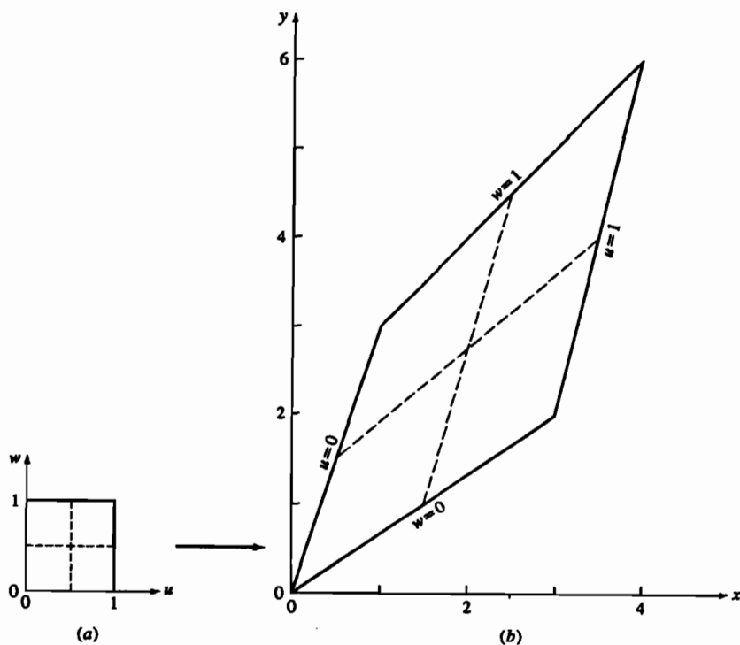
Рис. 6-23 Двумерное отображение поверхности. (а) Параметрическое пространство; (б) объектное пространство.
