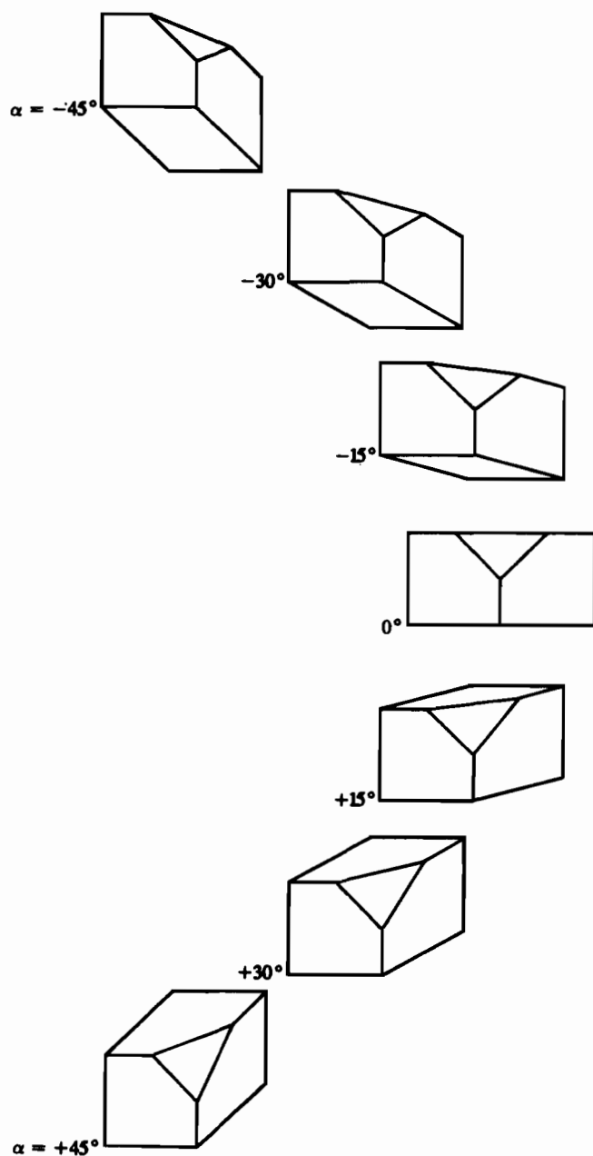
Рис. 3-22 Проекция кавалье. Сверху вниз угол \alpha изменяется от -45^\circ до +45^\circ с интервалом 15^\circ , угол \beta = 45^\circ .
