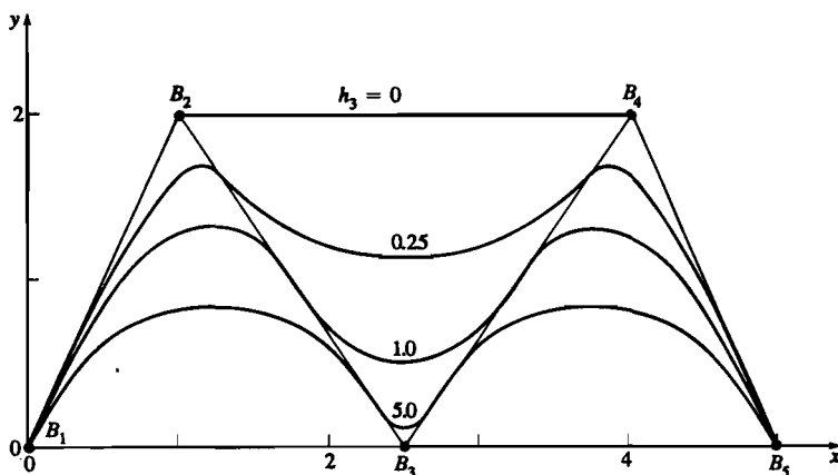
Рис. 5-58 Рациональные В-сплайны для n+1=5 , k=3 с открытым узловым вектором [X] = [0 \ 0 \ 0 \ 1 \ 2 \ 3 \ 3 \ 3] , [H] = [1 \ 1 \ h_3 \ 1 \ 1] .
