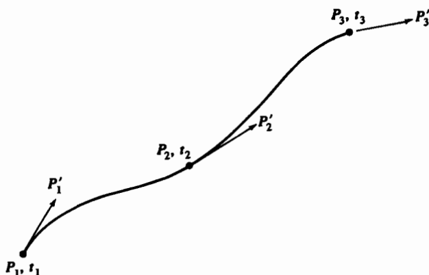
Рис. 5-6 Два кусочно кубических сегмента сплайна.
