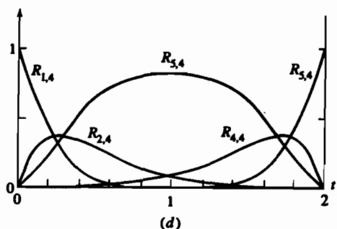
Рис. 5-59 Базисные функции рационального В-сплайна для n+1 = 5 , k = 4 с открытым узловым вектором [X] = [0 \ 0 \ 0 \ 0 \ 1 \ 2 \ 2 \ 2 \ 2] , [H] = [1 \ 1 \ h_3 \ 1 \ 1] . (a) h_3 = 0 ; (b) h_3 = 0.25 ; (c) h_3 = 1.0 ; (d) h_3 = 5.0 .
