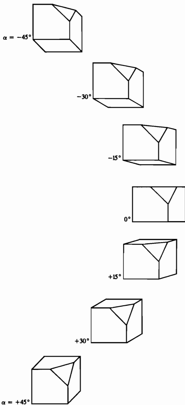
Рис. 3-23 Проекция кабины. Сверху вниз угол \alpha изменяется от -45^\circ до +45^\circ с интервалом 15^\circ , коэффициент искажения f = 0.5 .
