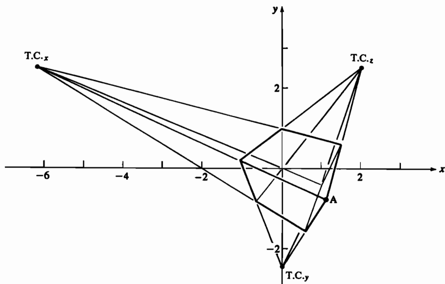
Рис. 3-36 Трехточечная перспективная проекция с поворотом вокруг двух осей.
