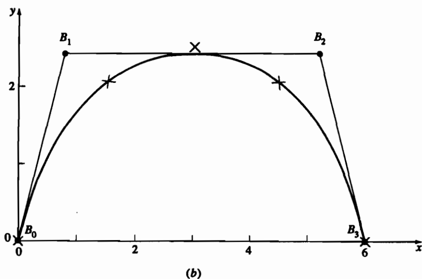
Рис. 5-56 Результаты для примера 5-17. (a) Пятиугольник; (b) четырехугольник.
