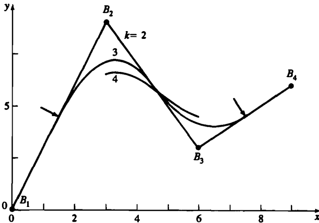
Рис. 5-44 Зависимость формы периодического В-сплайна от его порядка.
