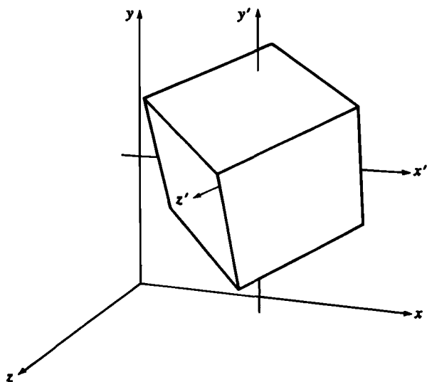
Рис. 3-6 Несколько поворотов относительно локальной системы координат.
