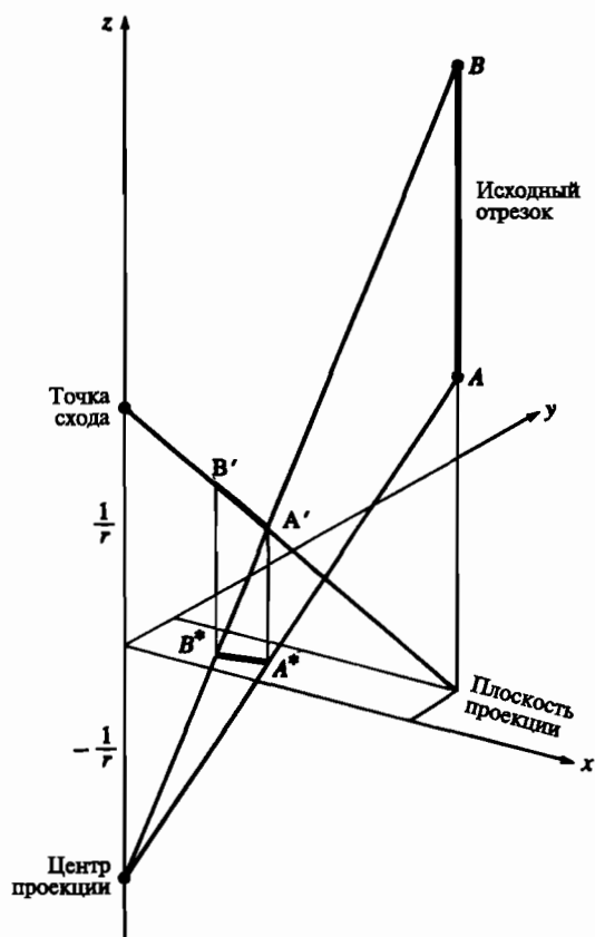
Рис. 3-27 Проекция прямой, параллельной оси z .
