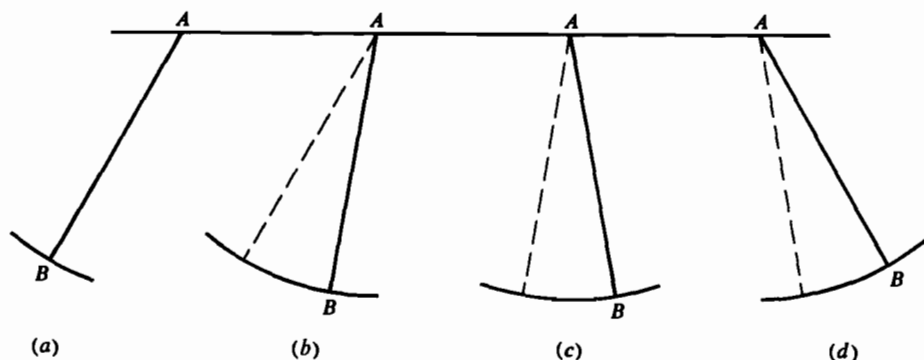
Рис. 1-19 Динамическое движение.
