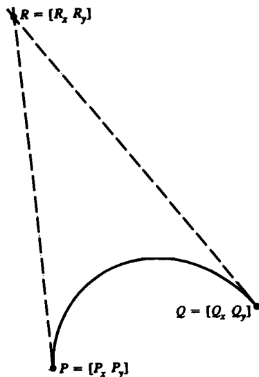
Рис. 4-12 Задание параметрической параболы вершинами.
