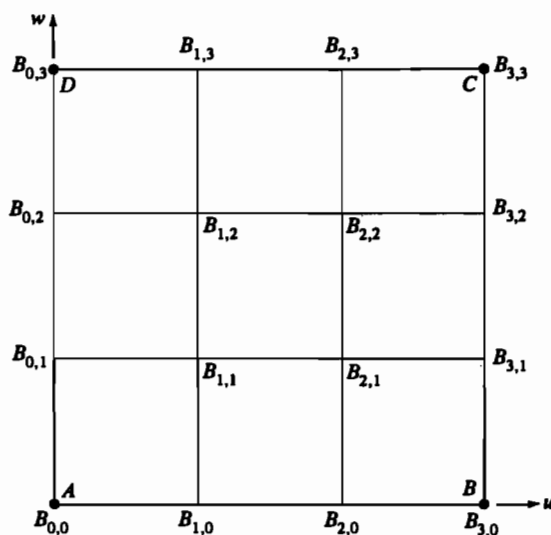
Рис. 6-38 Схема задающей полигональной сетки 4 \times 4 для поверхности Безье.
