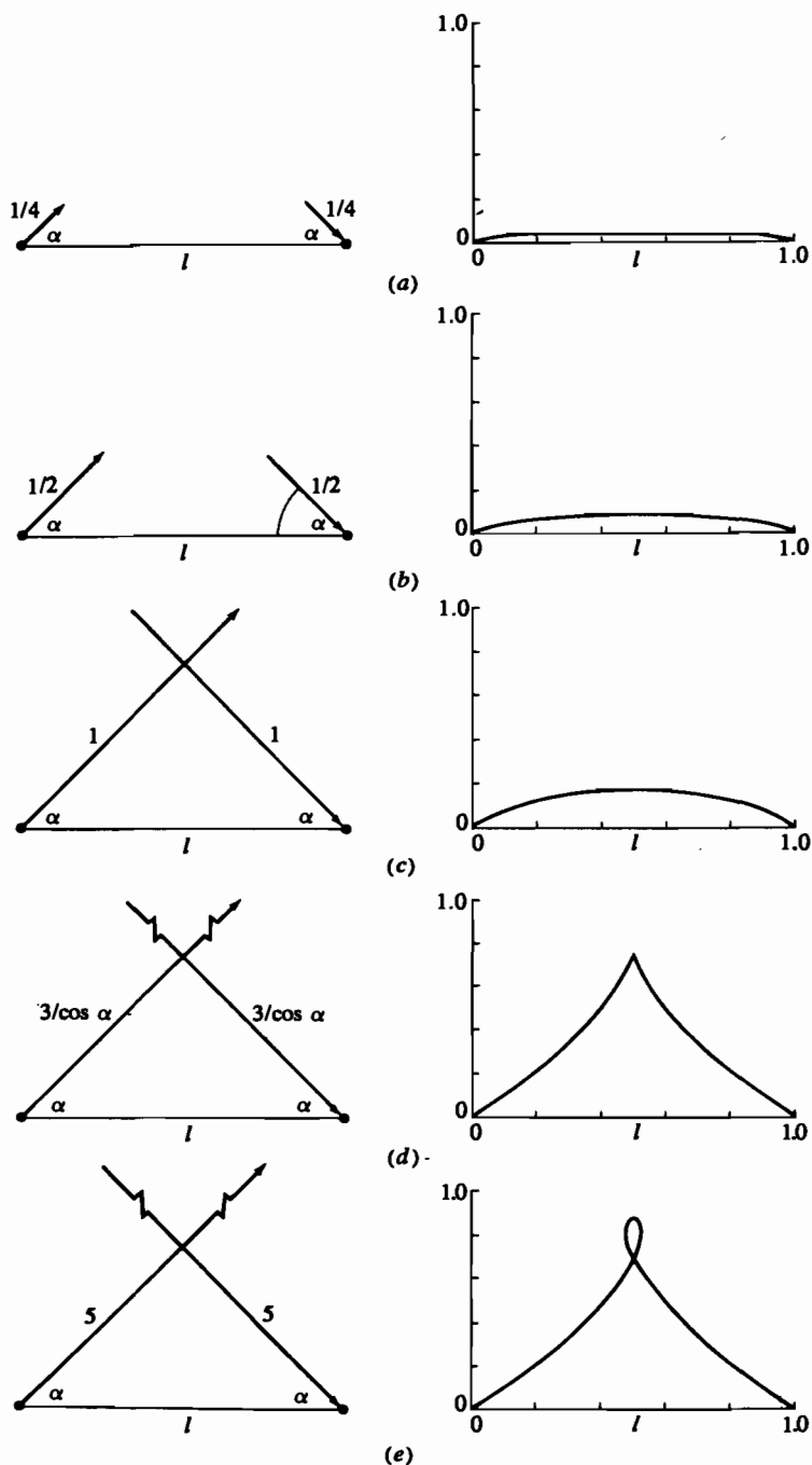
Рис. 5-10 Влияние величины касательного вектора на форму сегмента кубического сплайна, \alpha = \pi/4 . (a) 1/4 ; (b) 1/2 ; (c) 1; (d) 3/\cos \alpha ; (e) 5.
