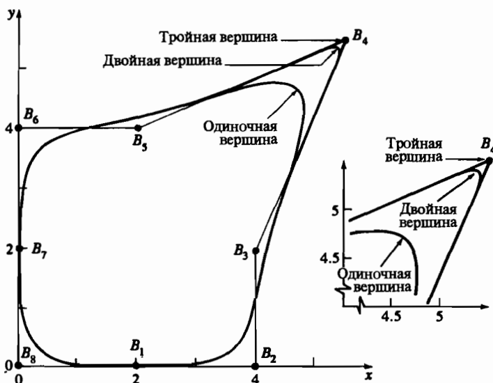
Рис. 5-48 Влияние кратных вершин на форму замкнутого периодического В-сплайна.
