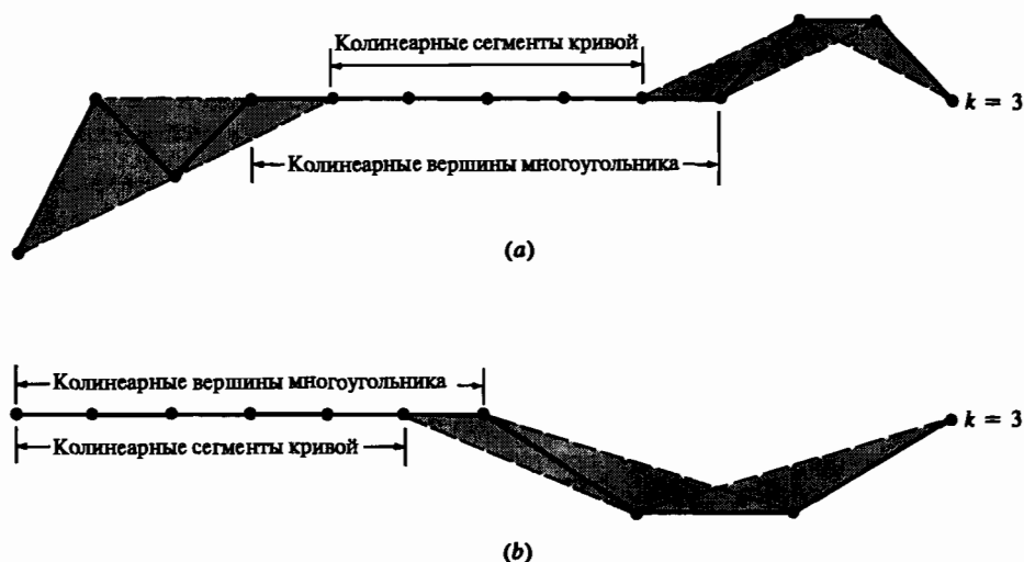
Рис. 5-33 Свойства выпуклой оболочки В-сплайнов для коллинеарных сегментов кривой. (а) Внутренние вершины определяющего многоугольника; (б) вершины в конце определяющего многоугольника.
