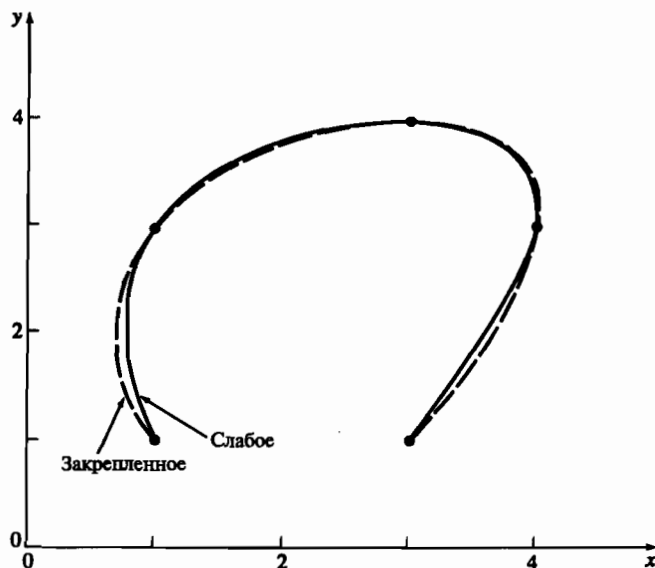
Рис. 5-13 Сравнение закрепленного и слабого граничных условий для нормализованного кусочно кубического сплайна.
