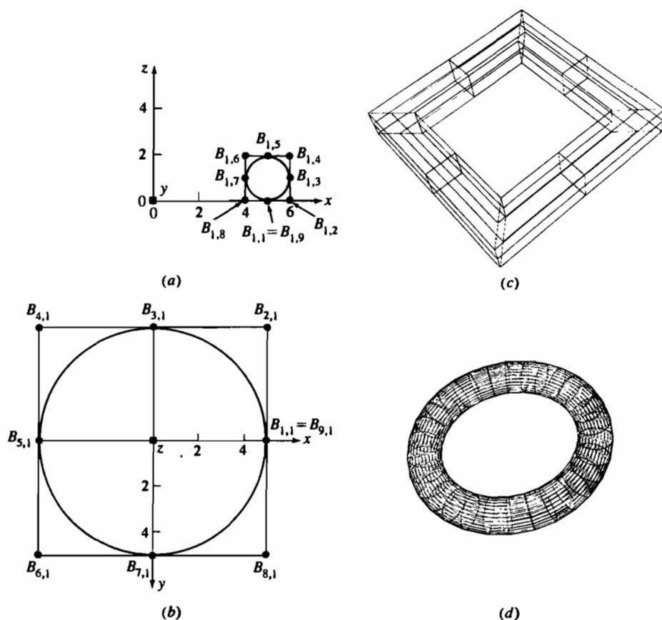
Рис. 6-58 Тор, сгенерированный как рациональная В-сплайн поверхность. (а) Смещенная окружность и задающий многоугольник; (б) окружность вращения и задающий многоугольник; (с) характеристический многогранник для тора; (д) тор.
