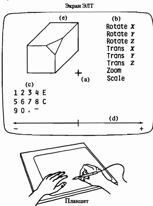
Рис. 1-16 Использование планшета для моделирования всех логических интерактивных функций: (а) локатора, (б) кнопки, (с) клавиатуры, (д) валюатора, (е) селектора.
