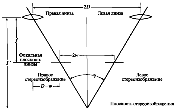
Рис. 3-44 Схема фокусного плоского стереоскопа.
