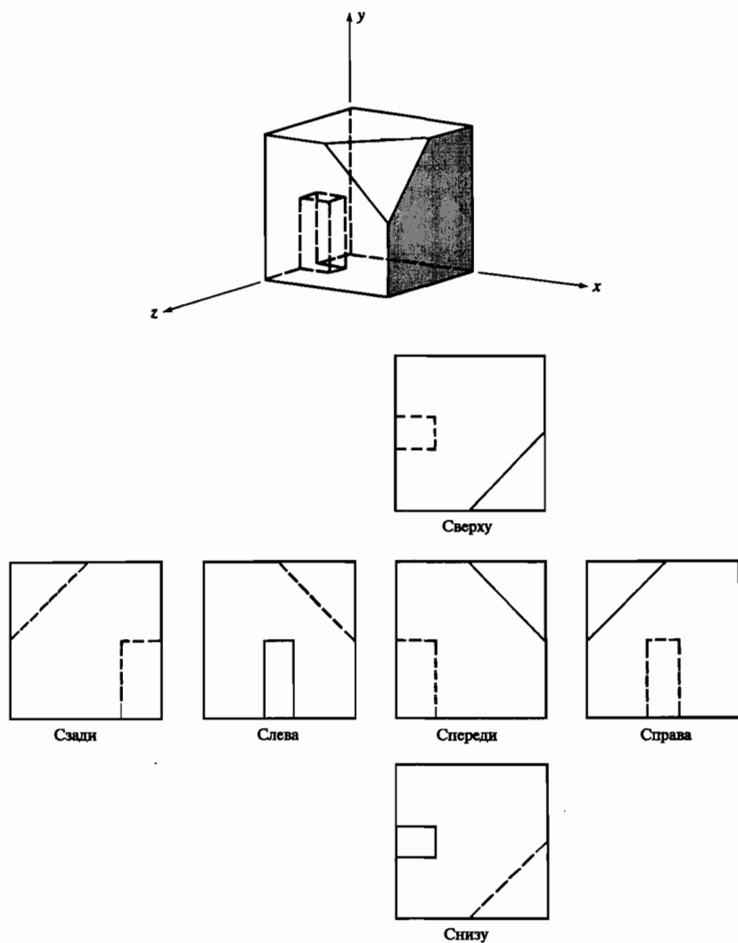
Рис. 3-13 Многовидовая ортогографическая проекция.
