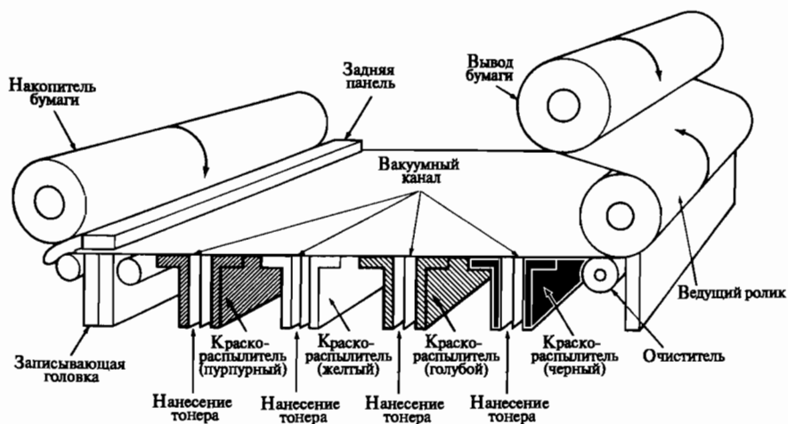
Рис. 1-44 Принципиальная схема цветного электростатического графопостроителя.
