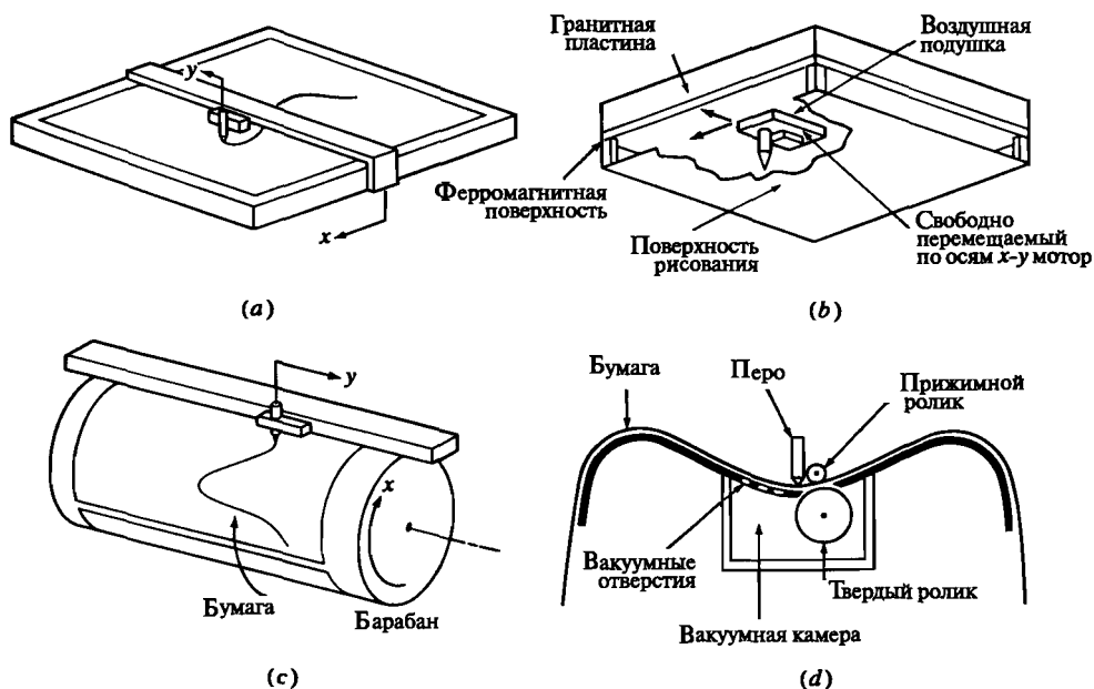
Рис. 1-56 Схемы действия перьевых графопостроителей разных типов: а) планшетный с подвижным кронштейном; б) планшетный с подвижным пишущим узлом; в) барабанный; д) с нажимным роликом.
