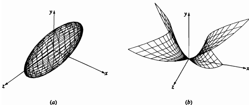
Рис. 6-19 Параметрические квадратичные поверхности. (а) Эллипсоид; (b) гиперболический параболоид.
