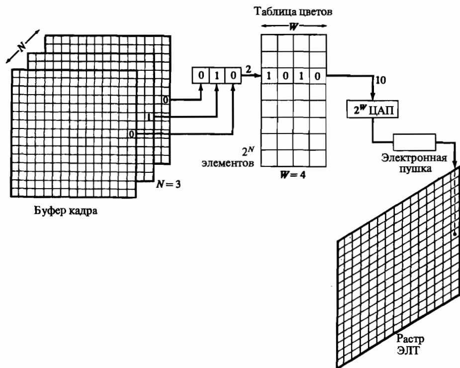
Рис. 1-26 Полутонный черно-белый буфер кадра с N битовыми плоскостями и W -разрядной таблицей цветов.
