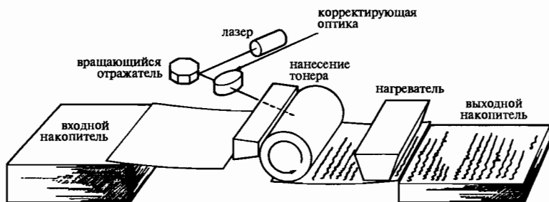
Рис. 1-48 Схема устройства лазерного принтера.
