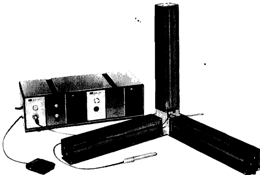
Рис. 1-8 Трехмерный звуковой планшет. (С разрешения фирмы Science Accessories Corp.)
