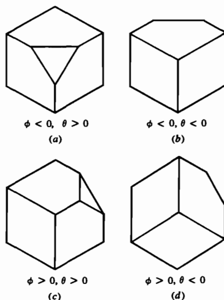
Рис. 3-19 Четыре возможных изометрических проекции с углами поворотов \phi = \pm 45^\circ , \theta = \pm 35, 26^\circ . (a) \phi = -45^\circ , \theta = +35, 26^\circ ; (b) \phi = -45^\circ , \theta = -35, 26^\circ ; (c) \phi = +45^\circ , \theta = +35, 26^\circ ; (d) \phi = +45^\circ , \theta = -35, 26^\circ .
