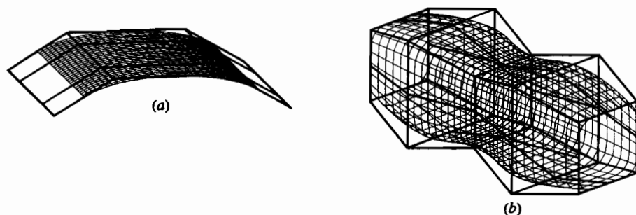
Рис. 6-47 Объединенные В-сплайн поверхности третьего порядка. (а) Незамкнутый характеристический многогранник; (b) замкнутый характеристический многогранник.
