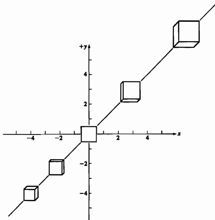
Рис. 3-34 Одноточечная перспективная проекция, объединенная с переносами в x , y , z направлениях.
