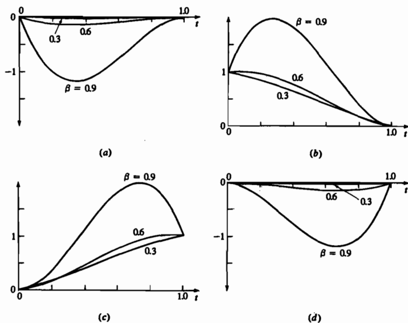
Рис. 5-22 Обобщенные параболические весовые функции, \alpha = 1 - \beta . (a) F_1 ; (b) F_2 ; (c) F_3 ; (d) F_4 .
