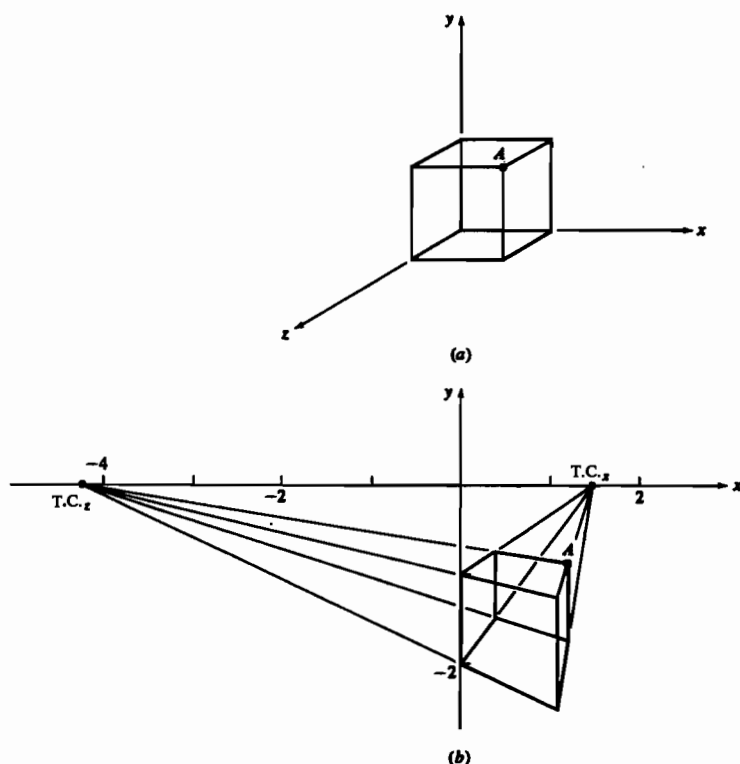
Рис. 3-35 Двухточечная перспективная проекция с поворотом вокруг одной оси.
