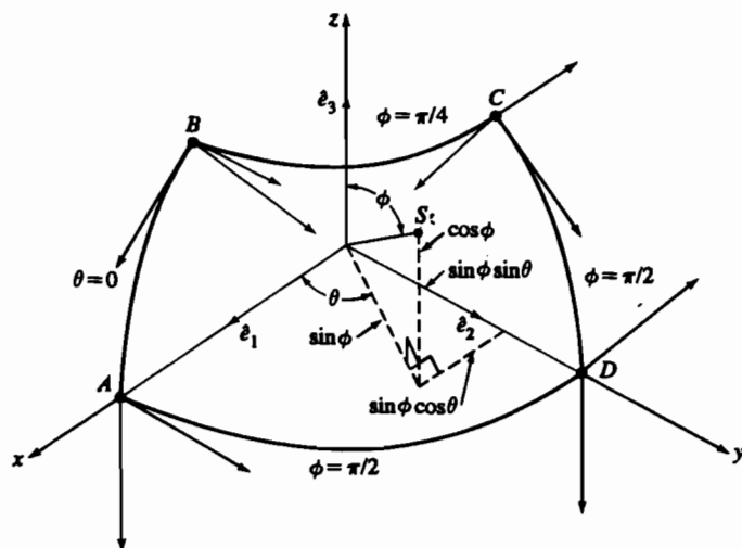
Рис. 6-21 Кусок сферической поверхности.
