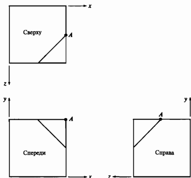
Рис. 3-49 Восстановление трехмерной формы по ортогографическим проекциям.
