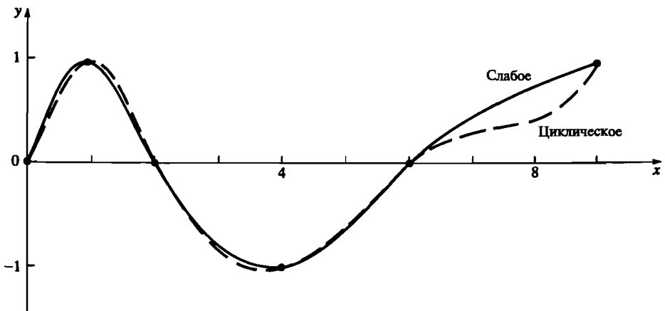
Рис. 5-16 Сравнение слабого и циклического граничных условий для открытых кривых.
