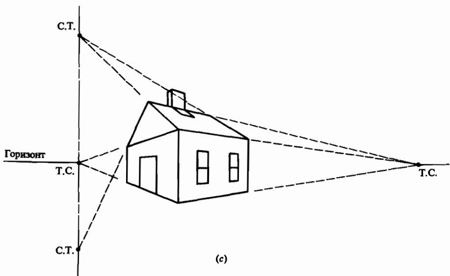
Рис. 3-37 Следы точек и точки схода.
