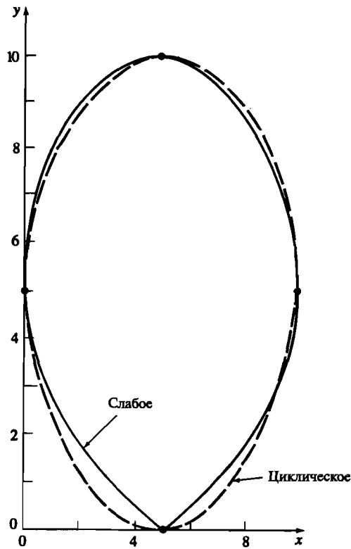
Рис. 5-15 Сравнение слабого и циклического граничных условий для нормализованного кусочно кубического сплайна.
