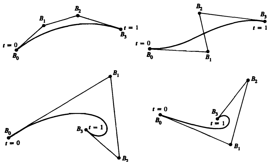
Рис. 5-26 Многоугольники Безье для кубических кривых.
