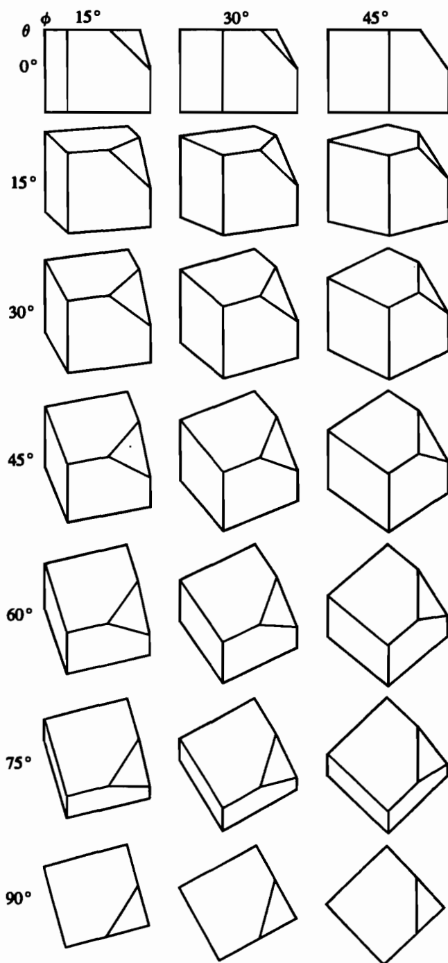
Рис. 3-16 Триметрические проекции.
