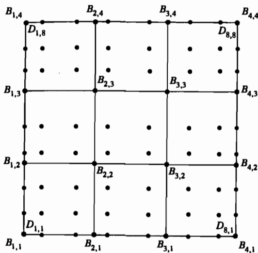
Рис. 6-49 Определение В-сплайн поверхности по известному набору данных.
