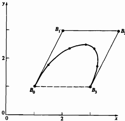
Рис. 5-28 Сегмент кривой Безье, пример 5-7.
