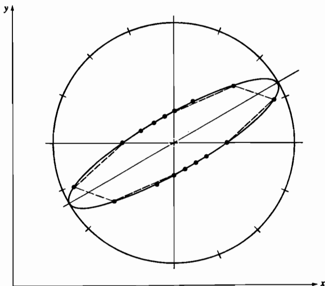
Рис. 4-6 Равноугольное представление сильно вытянутого эллипса.
