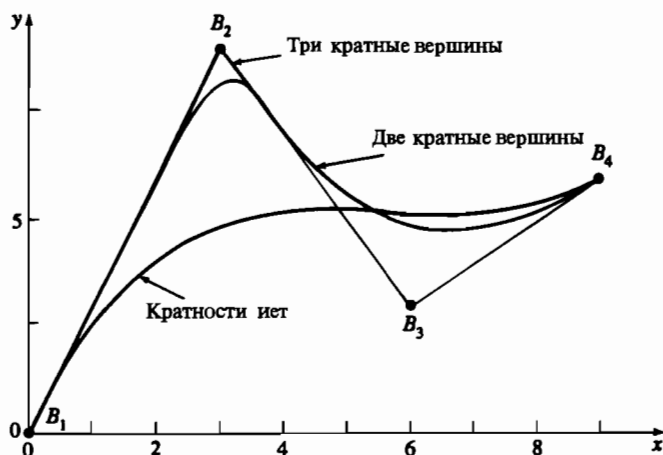
Рис. 5-42 Влияние кратности вершины на форму В-сплайна, k = 4 .
