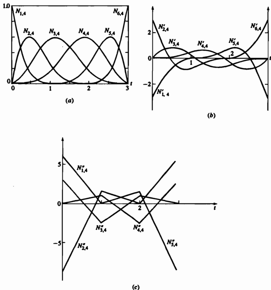
Рис. 5-51 Базисные функции В-сплайна и их первые и вторые производные, k = 4 , n = 6 . (a) Базисные функции; (b) первая производная; (c) вторая производная.
