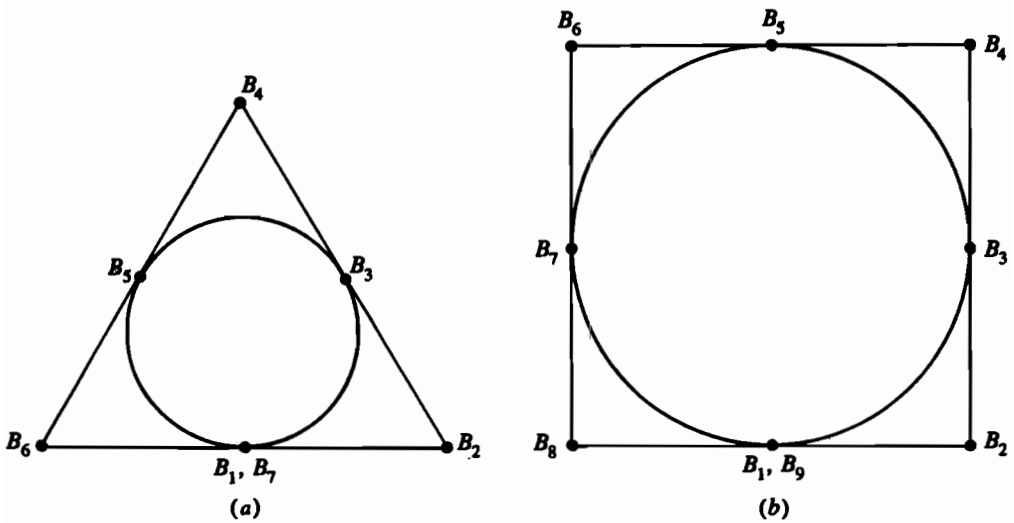
Рис. 5-69 Рациональные В-сплайны — окружности. (а) Три сегмента по 120^\circ ; (б) четыре сегмента по 90^\circ .
