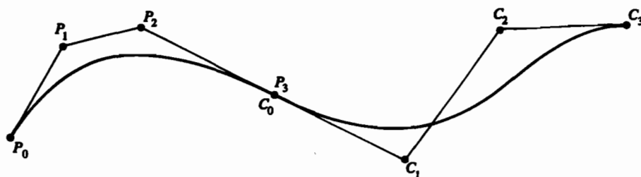
Рис. 5-30 Непрерывность первой производной для кубических кривых Безье.
