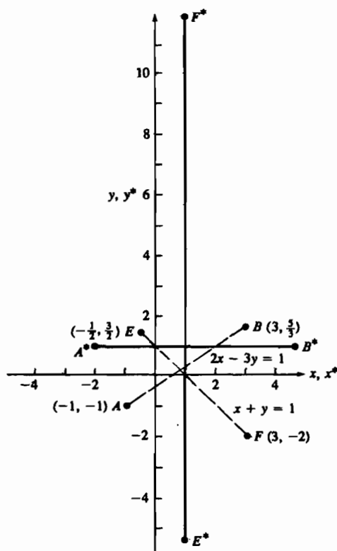
Рис. 2-3 Преобразование пересекающихся прямых.
