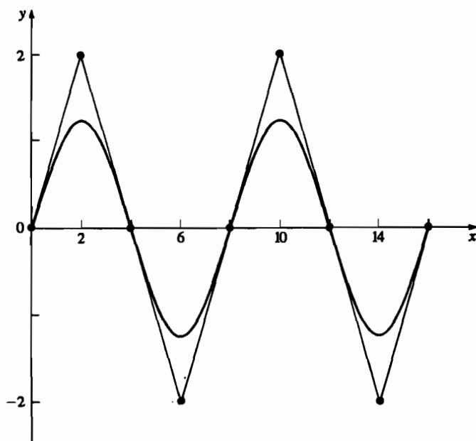
Рис. 5-31 Непрерывность второй производной для кривых Безье четвертой степени.
