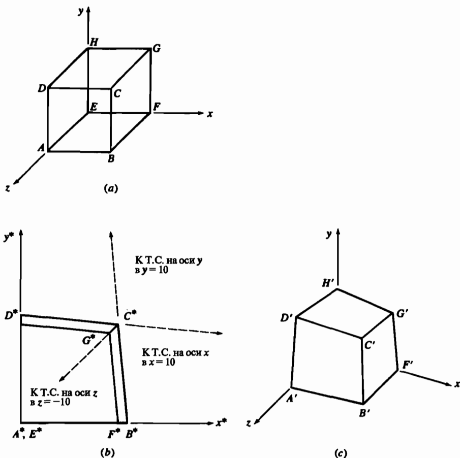
Рис. 3-31 Трехточечная перспектива. (а) Исходный куб; (б) перспективная проекция на плоскость z = 0 ; (с) искаженный куб.
