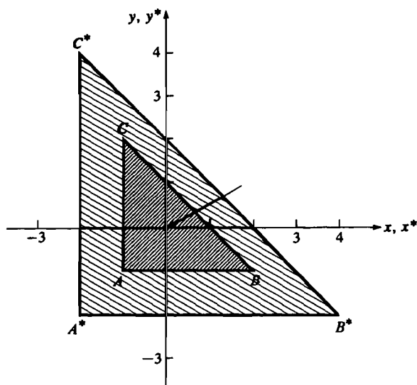
Рис. 2-9 Пропорциональное масштабирование без явного перемещения.
