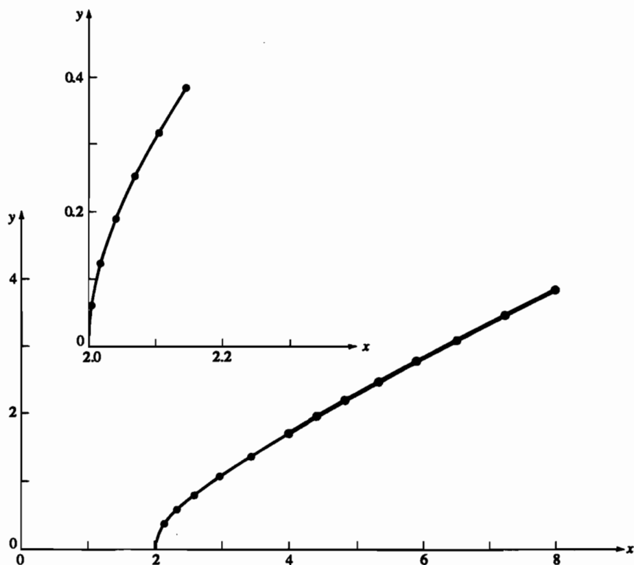
Рис. 4-13 Параметрическая гипербола.
