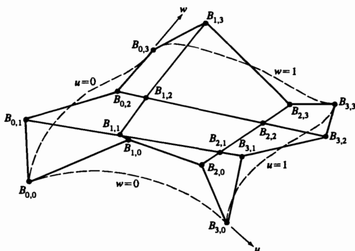
Рис. 6-37 Поверхность Безье и вершины характеристического многогранника.
