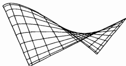
Рис. 6-32 Кусок бикубической поверхности Кунса.
