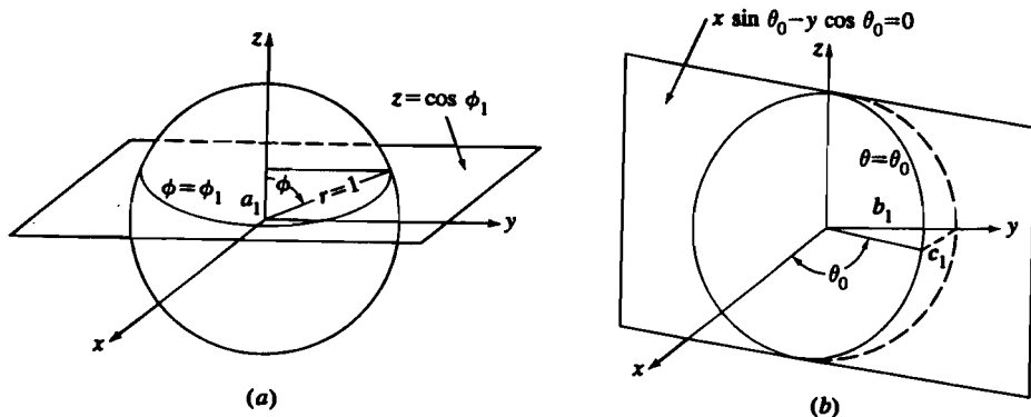
Рис. 6-20 Пересечение плоскости и сферы. (а) Параллель широты; (б) меридиан долготы.
