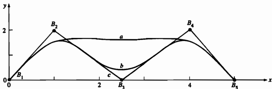
Рис. 5-66 Влияние кратной вершины многоугольника B_3 на рациональный В-сплайн n+1=5 , k=4 . (а) Одна вершина [H] = [1 \ 1 \ 0.25 \ 1 \ 1] ; (б) двойная вершина [H] = [1 \ 1 \ 0.25 \ 0.25 \ 1 \ 1] ; (с) тройная вершина [H] = [1 \ 1 \ 0.25 \ 0.25 \ 0.25 \ 1 \ 1] .
