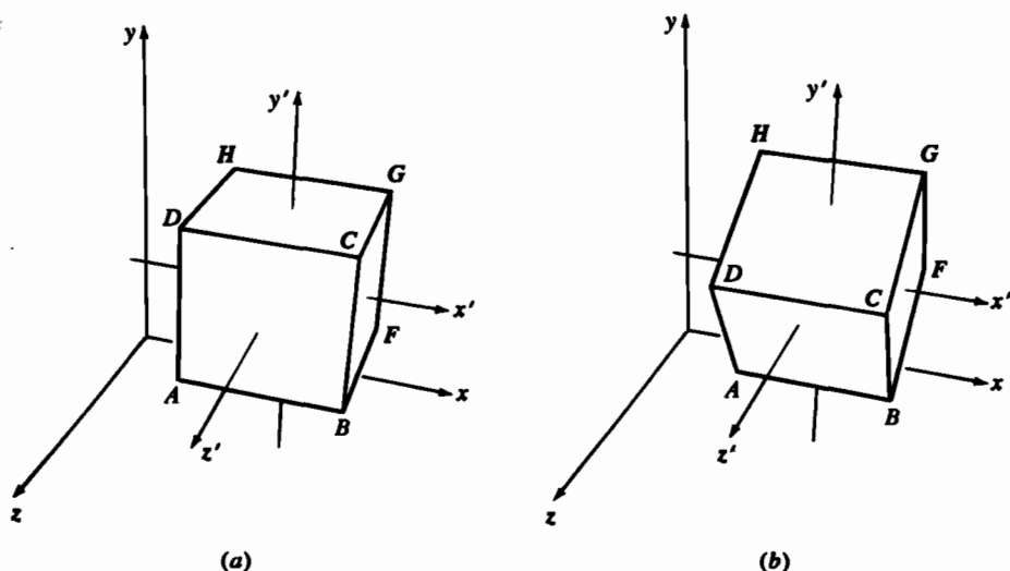
Рис. 3-5 Поворот вокруг оси, параллельной одной из координатных осей.
