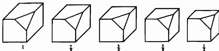
Рис. 3-24 Косоугольные проекции. Слева направо f = 1, 7/8, 3/4, 5/8, 1/2 при \alpha = 45^\circ .
