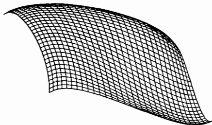
Рис. 6-34 Действие на кусок бикубической поверхности изменения направления касательного вектора.
