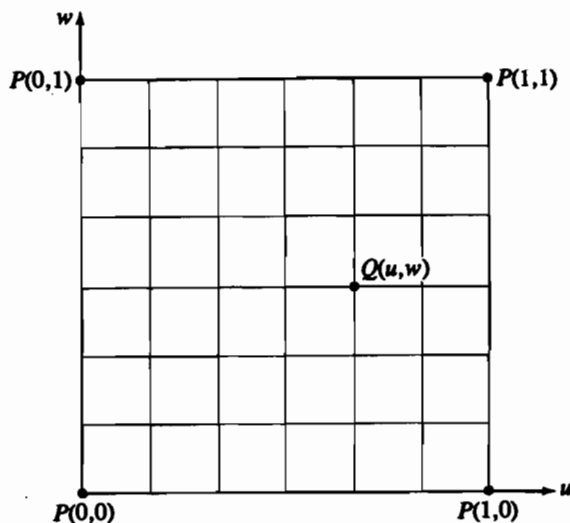
Рис. 6-25 Билинейная интерполяция в параметрическом пространстве.
