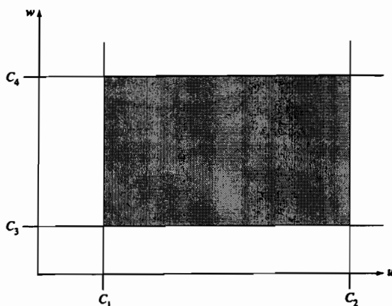
Рис. 6-22 Прямоугольная параметрическая плоская поверхность.
