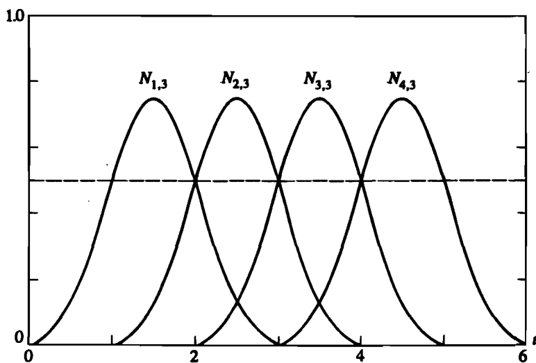
Рис. 5-36 Базисные функции периодического равномерного В-сплайна, [X] = [0 \ 1 \ 2 \ 3 \ 4 \ 5 \ 6] , n+1=4 , k=3 .
