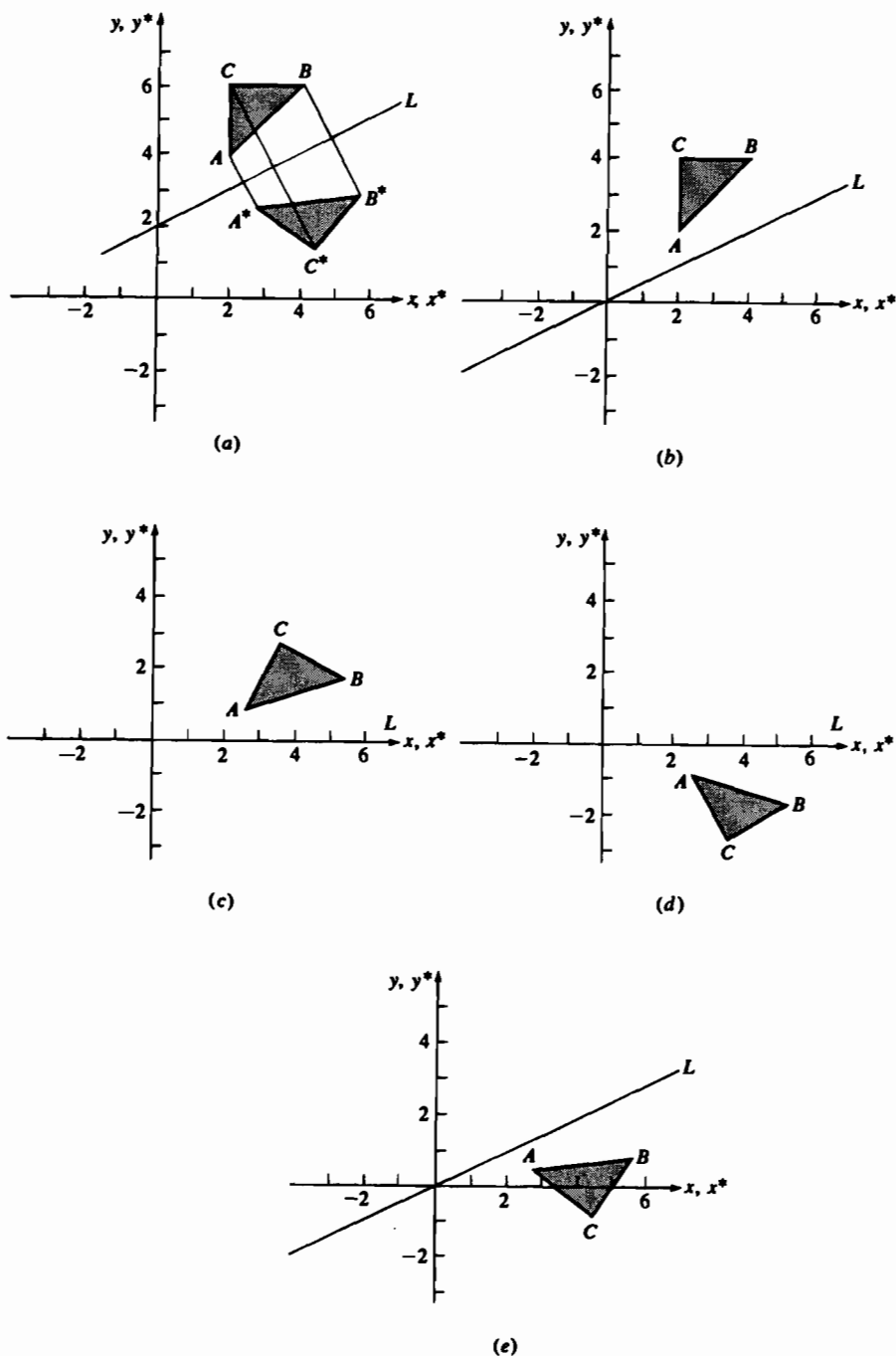
Рис. 2-13 Отражение относительно произвольной прямой: а) исходное и конечное положение; б) перенос прямой в начало координат; в) поворот до совпадения с осью x ; д) отражение относительно оси x ; е) обратный поворот; а) обратный перенос.
