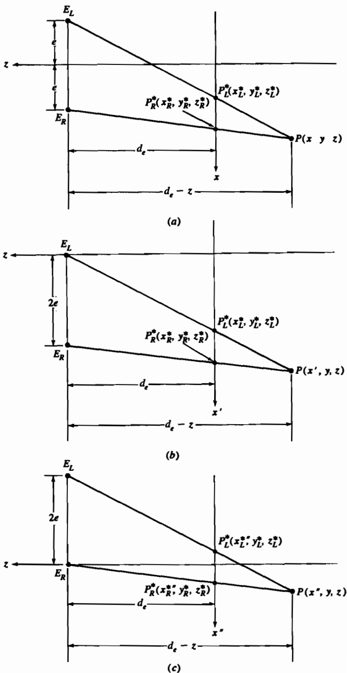
Рис. 3-41 Стереогрaфическая проекция на плоскость z = 0 .
