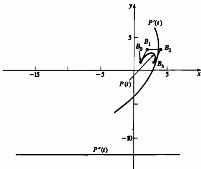
Рис. 5-29 Кривая Безье и ее производные: P(t) ; P'(t) ; P''(t) .
