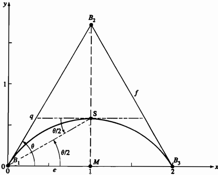
Рис. 5-68 Дуга окружности, построенная как рациональный В-сплайн.
