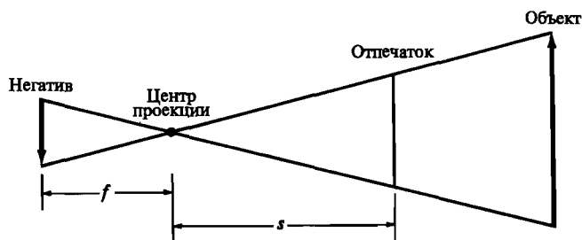
Рис. 3-39 Фотография как перспективная проекция.
