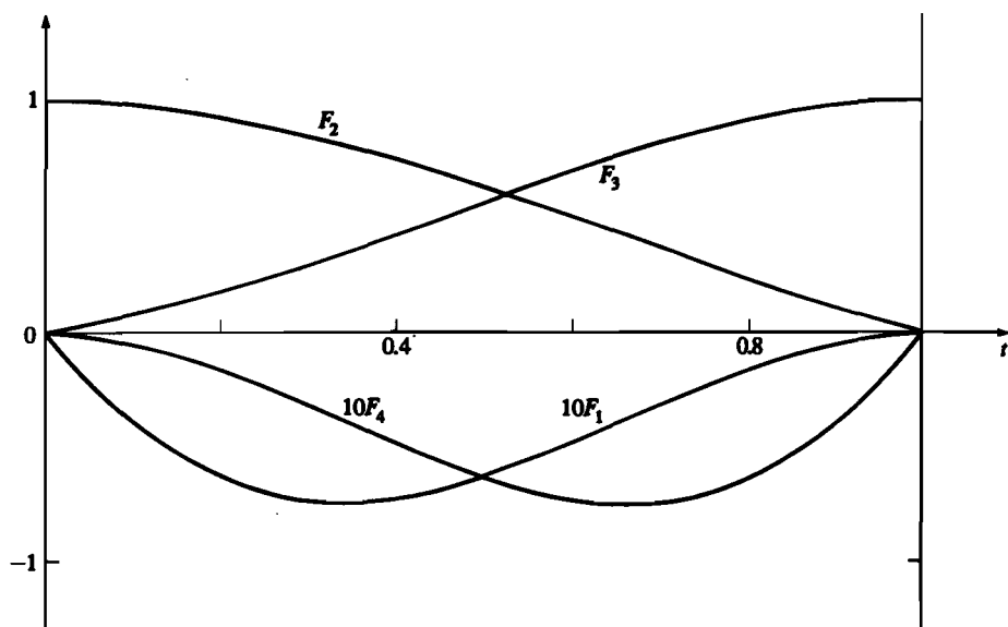
Рис. 5-20 Весовые функции для параболически интерполированных кривых в случае \alpha = \beta = 0.5 .
