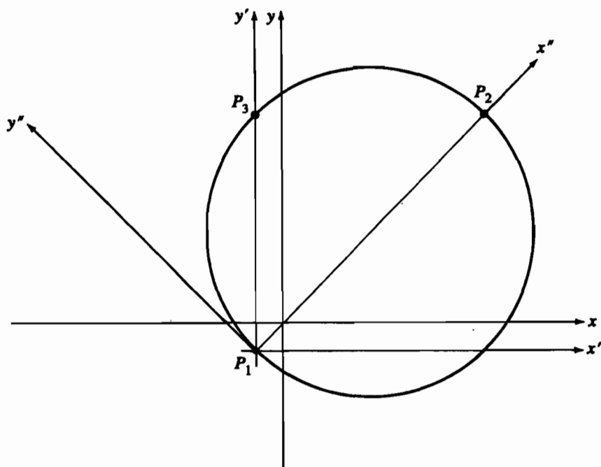
Рис. 4-14 Окружность, проходящая через три заданные точки.
