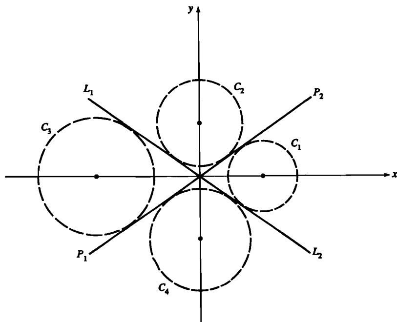
Рис. 4-15 Окружности, касающиеся двух пересекающихся прямых.
