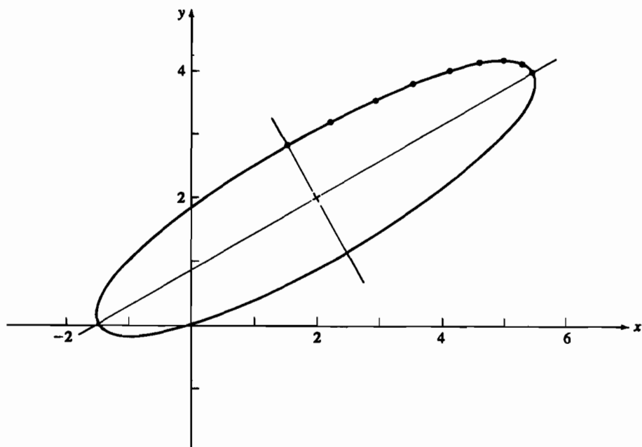
Рис. 4-8 Эллипс после поворота и переноса.
