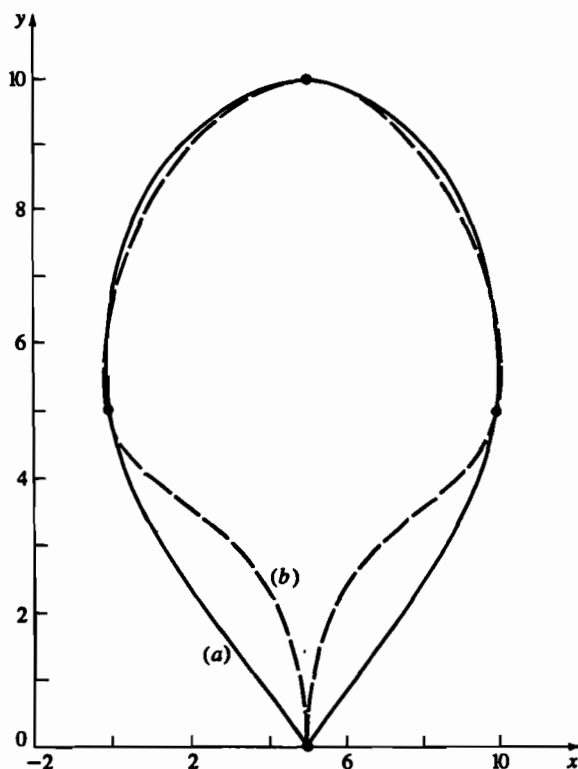
Рис. 5-14 Влияние величины касательного вектора на форму нормализованного кусочно кубического сплайна. (a) P_1'[0 \ 1] , P_2'[0 \ -1] ; (b) P_1'[0 \ 10] , P_2'[0 \ -10] .
