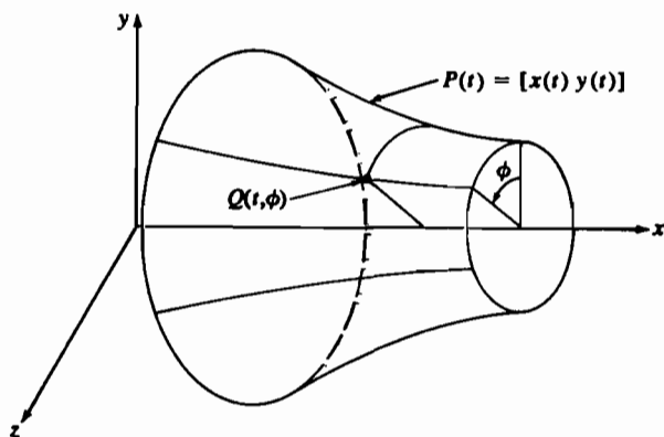
Рис. 6-5 Бипараметрическая поверхность вращения.
