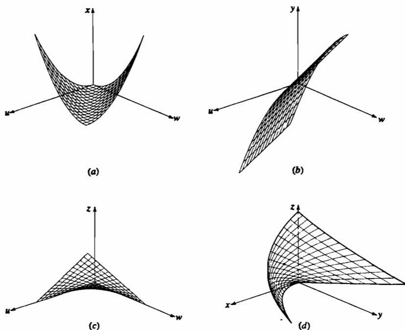
Рис. 6-24 Трехмерное отображение поверхности. (a) x компонента; (b) y компонента; (c) z компонента; (d) результат.
