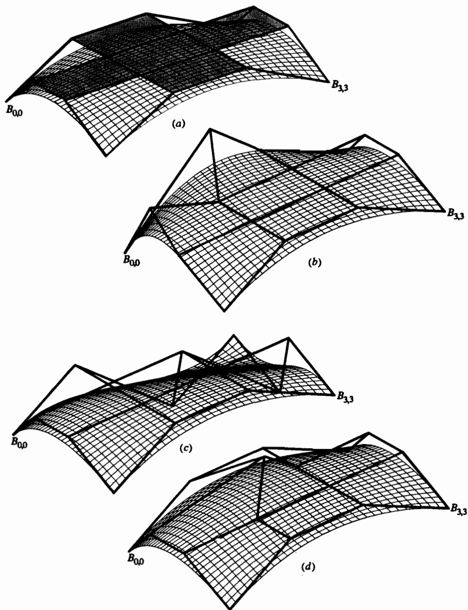
Рис. 6-39 Бикубические поверхности Безье. (а) Основная поверхность; (б) эффект изменения величины обоих касательных векторов в B_{0,0} ; (с) эффект изменения направления касательного вектора в B_{0,3} ; (д) эффект изменения величины вектора кручения в B_{0,0} .
