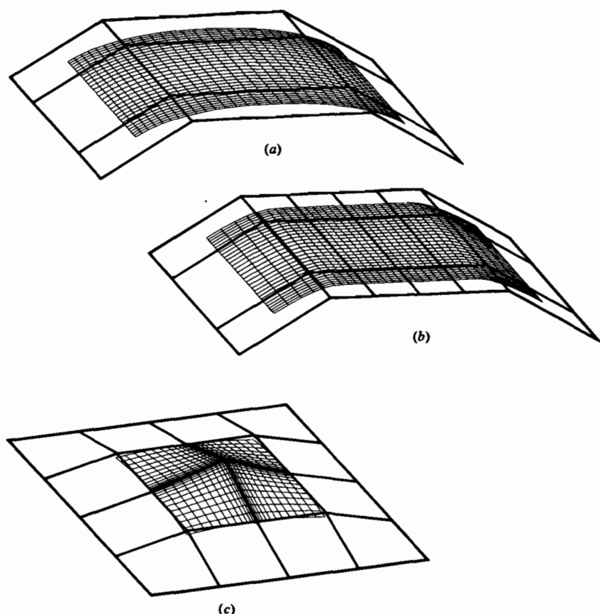
Рис. 6-45 Периодические В-сплайн поверхности для незамкнутых характеристических многогранников. (а) Гладкая линейчатая поверхность третьего порядка; (б) большая внутренняя плоская область третьего порядка, вызванная коллинеарностью пяти вершин сетки в u направлении; (с) острый выступ на поверхности четвертого порядка, вызванный пересечением нескольких совпадающих линий сетки.
