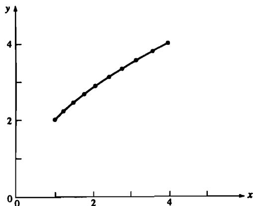
Рис. 4-11 Сегмент параболы.
