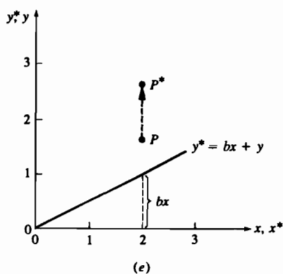
Рис. 2-1 Преобразование точек.
