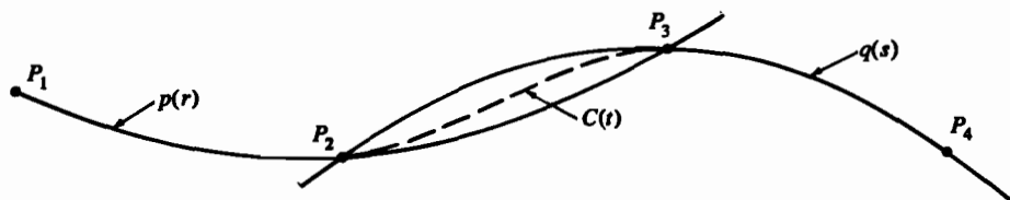
Рис. 5-19 Обозначение для параболической интерполяции.
