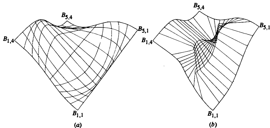
Рис. 6-54 Рациональные В-сплайн поверхности с n + 1 = 5 , m + 1 = 4 , k + l = 4 . (a) Все внутренние h_{i,j} - e = 0 ; (b) все внутренние h_{i,j} - e = 500 .
