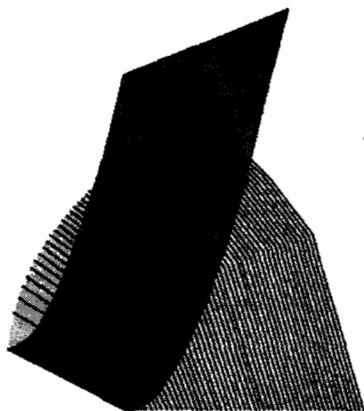
Рис. 5-2 Пересечение кривых второго порядка.
