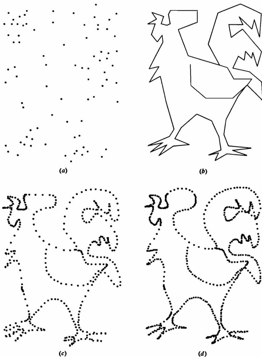
Рис. 5-11 Сравнение кубических сплайновых аппроксимаций. (a) Данные; (b) соединения прямыми; (c) нормализованная аппроксимация t_k ; (d) хордовая аппроксимация t_k .
