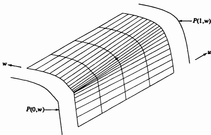
Рис. 6-28 Пример линейчатой поверхности.
