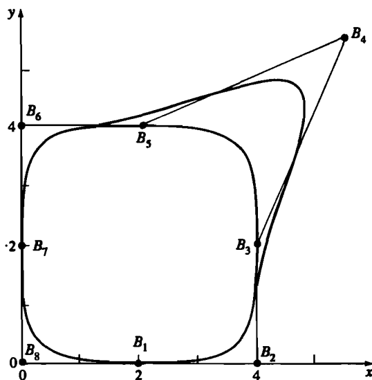
Рис. 5-47 Изменение формы В-сплайна после перемещения одной вершины многоугольника.
