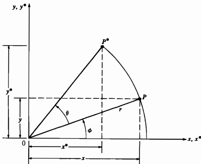
Рис. 2-5 Поворот координатного вектора.
