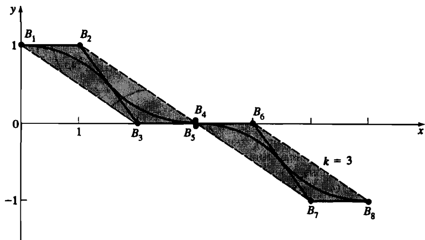
Рис. 5-35 Плавное ( C^{k-2} ) превращение в отрезки прямой.
