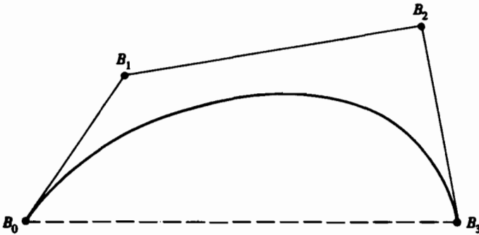
Рис. 5-25 Кривая Безье и определяющие ее точки.
