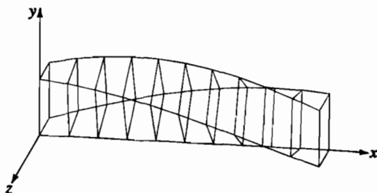
Рис. 6-16 Заметающая поверхность, образованная квадратом, перемещаемым вдоль оси x и одновременно вращаемым вокруг нее.
