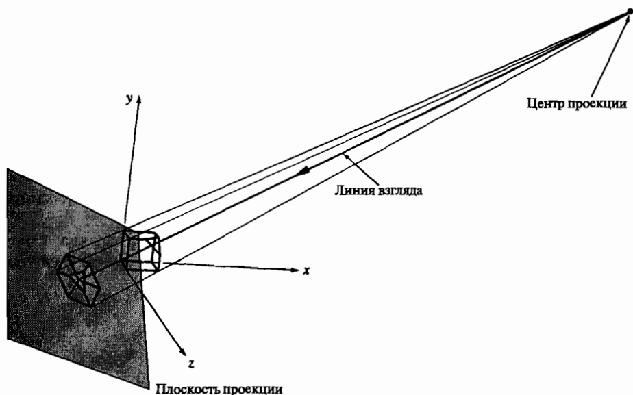
Рис. 3-47 Перспективное проецирование с перемещающимся центром проекции.
