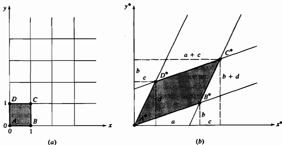
Рис. 2-11 Общее преобразование единичного квадрата: а) до преобразования; б) после преобразования.
