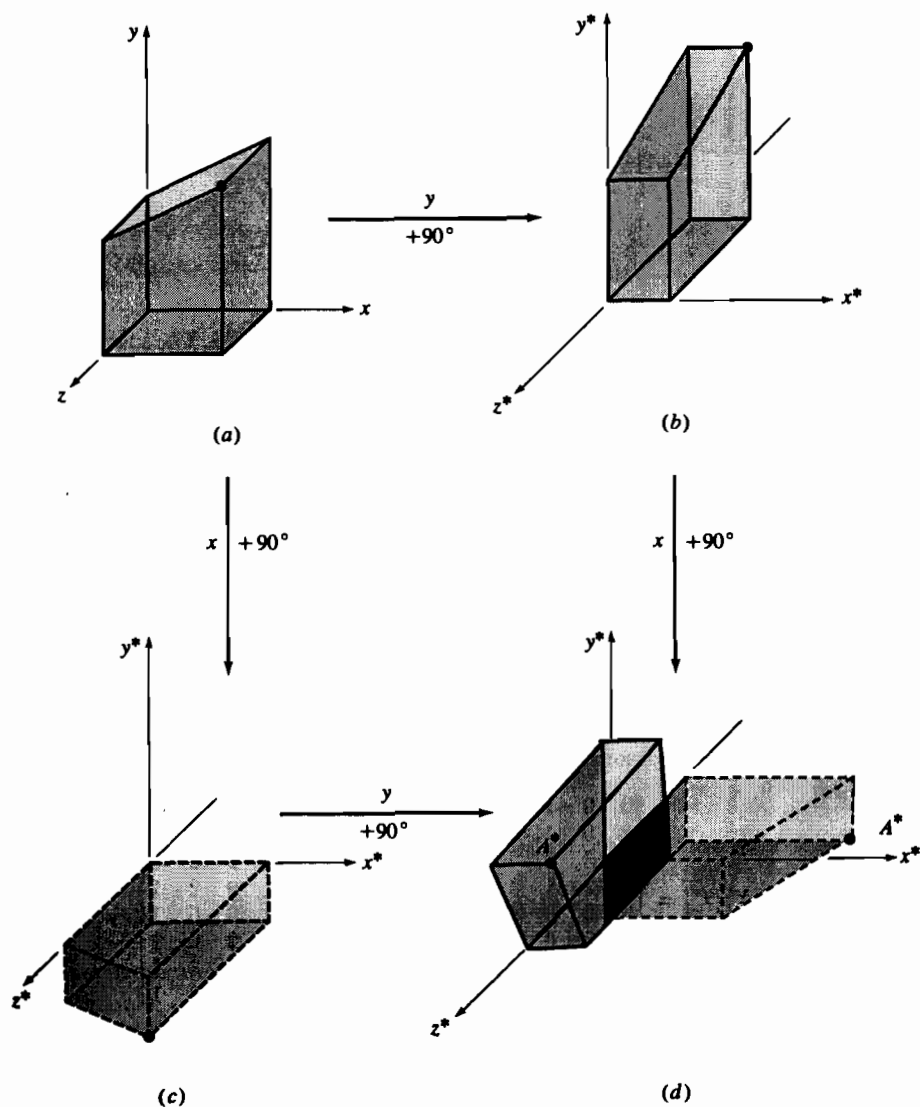
Рис. 3-3 Некоммутативность трехмерных поворотов.
