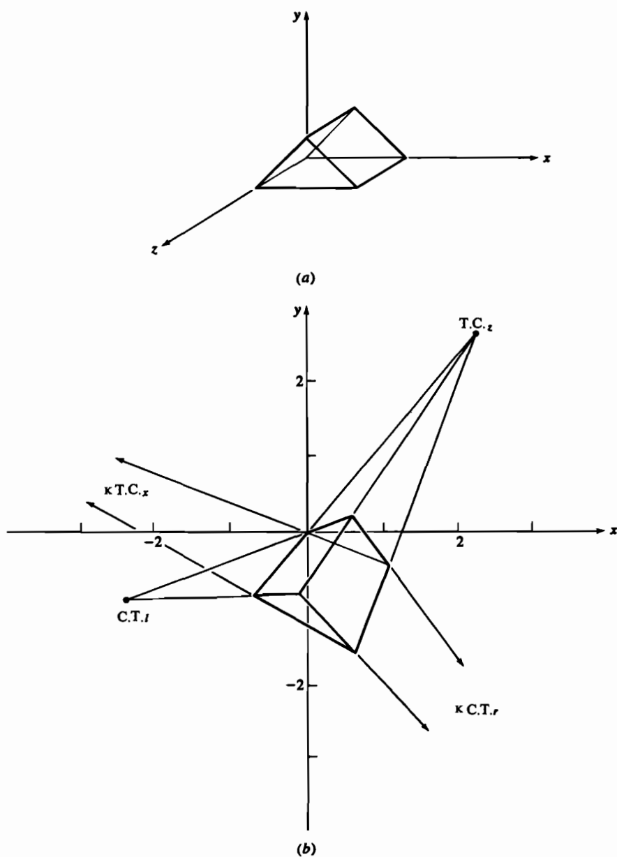
Рис. 3-38 Следы точек.
