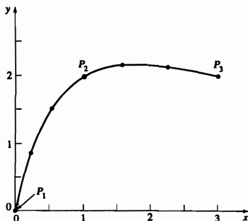
Рис. 5-12 Кубический сплайн для примера 5-4.
