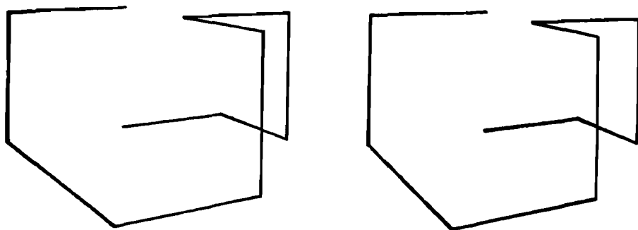
Рис. 3-45 Стереопара.
