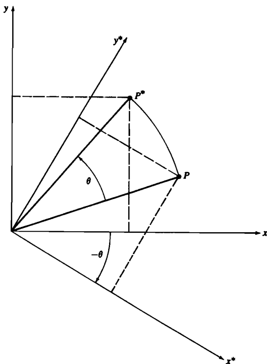
Рис. 2-16 Эквивалентность преобразования координатных векторов и систем координат.
