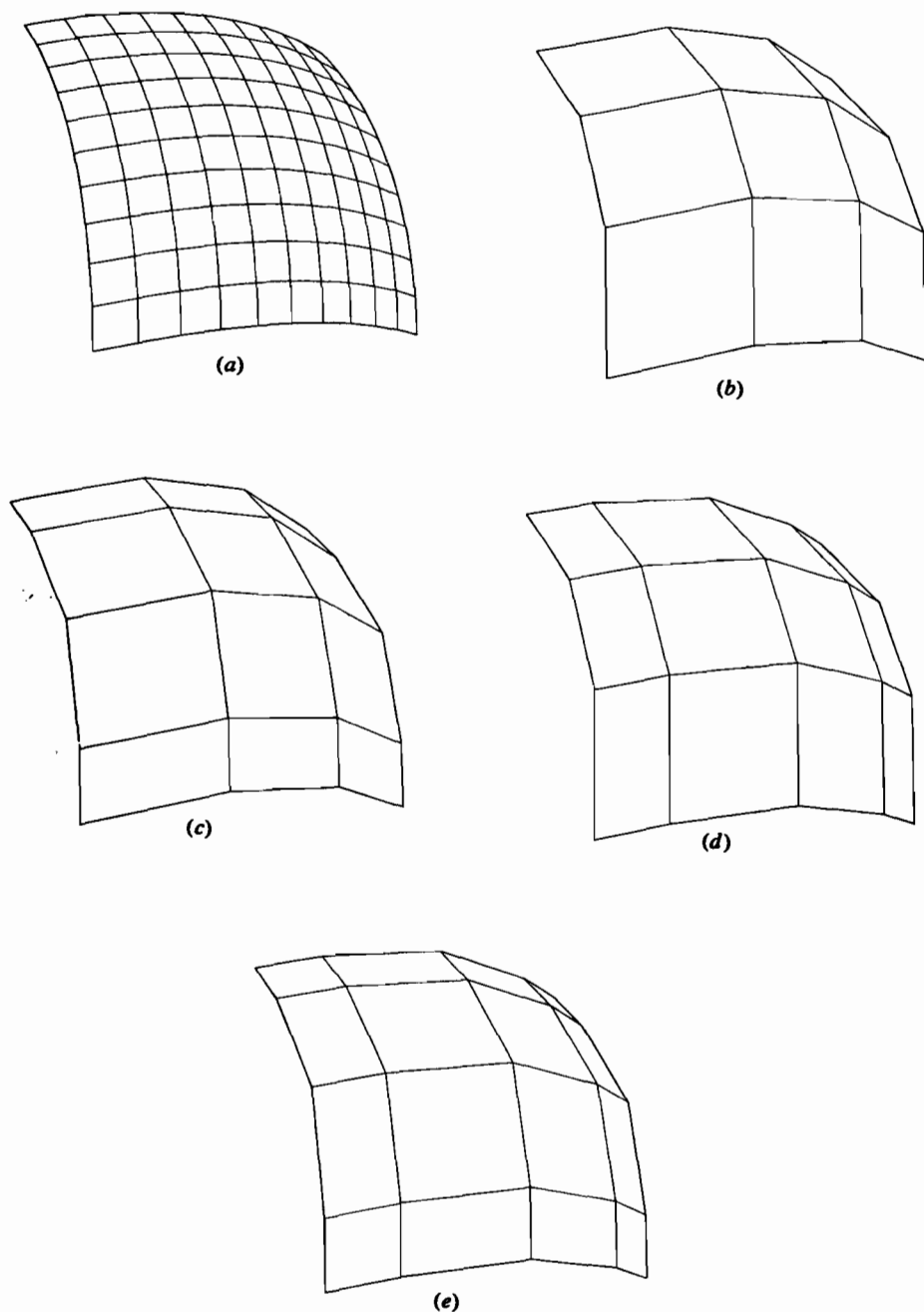
Рис. 6-51 Разбиение В-сплайн поверхности. (a) Поверхность; (b) исходная задающая полигональная сетка; (c) сетка, разбитая в w направлении; (d) сетка, разбитая в u направлении; (e) сетка, разбитая в обоих направлениях.
