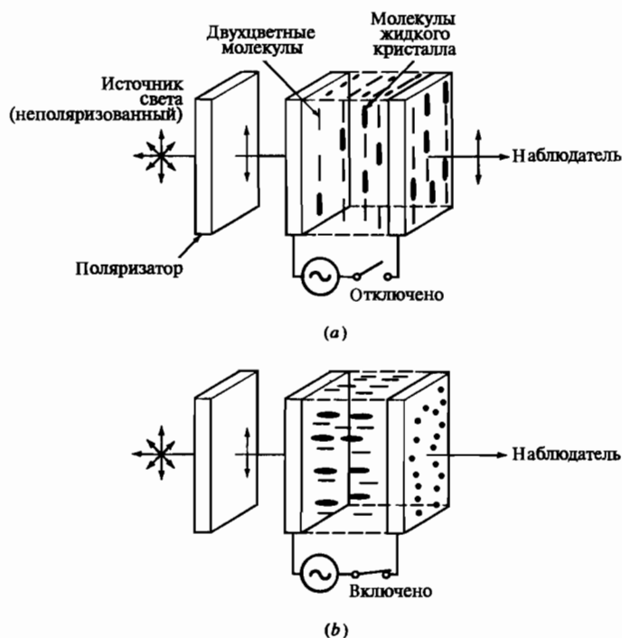
Рис. 1-43 Жидкие кристаллы типа гость-хозяин (закрашены). Молекулы ориентированы для блокировки (а) и для свободного прохождения (б).
