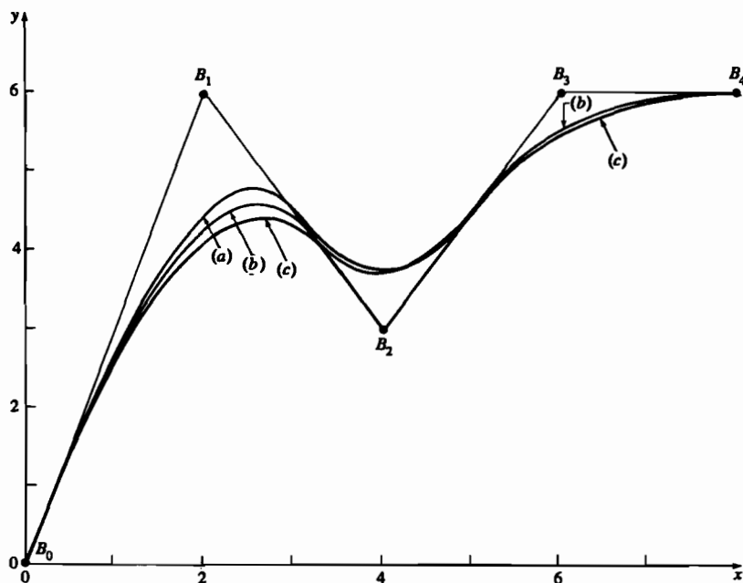
Рис. 5-50 Сравнение открытых неравных В-сплайнов: (a) равномерный узловый вектор; (b) неравномерный узловый вектор, пропорциональный длинам хорд; (c) неравномерный узловый вектор, пропорциональный длинам хорд, с двойной вершиной в B_2 .
