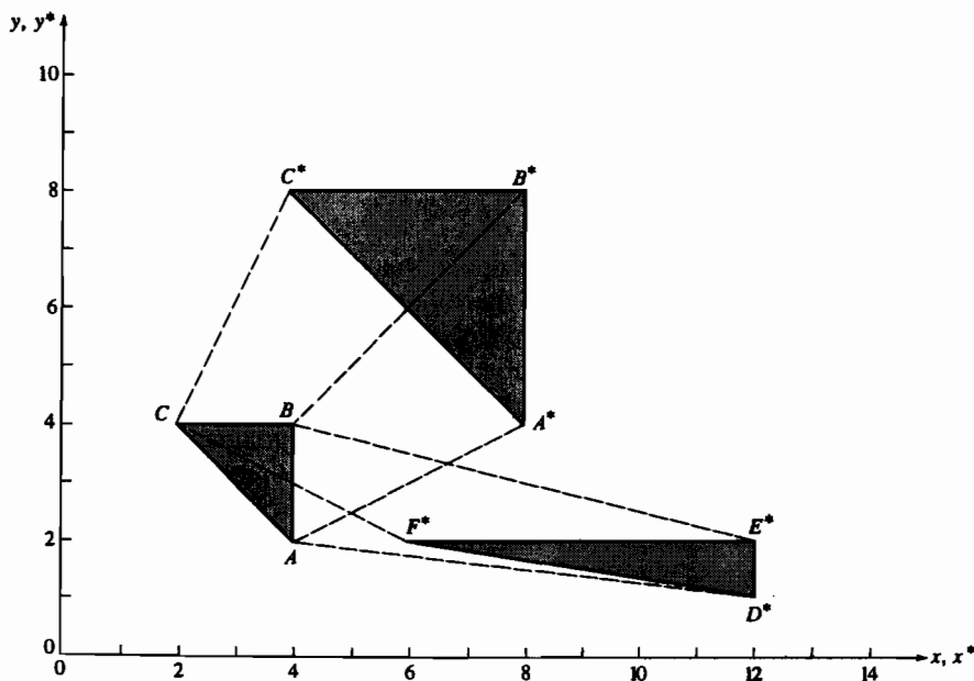
Рис. 2-8 Пропорциональное и непропорциональное масштабирование (искажение).
