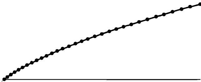
Рис. 4-10 Параметрически сгенерированная парабола.
