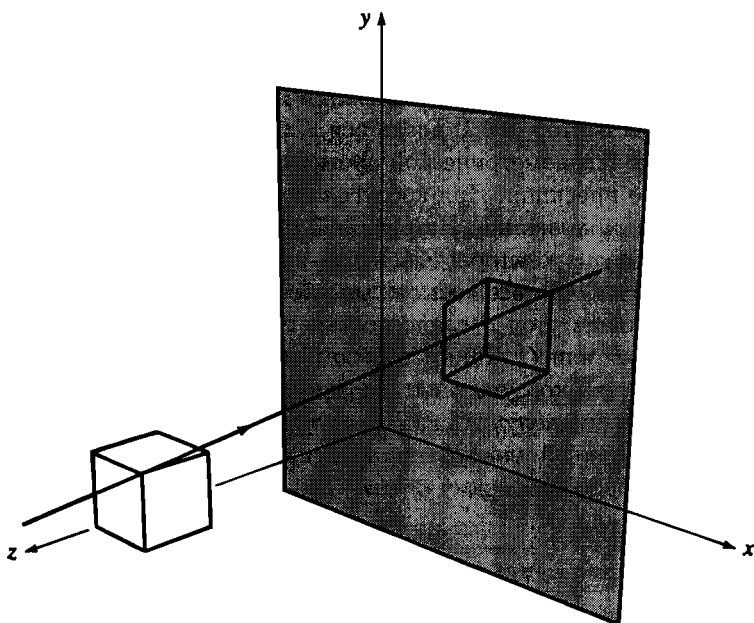
Рис. 3-20 Косоугольная проекция.
