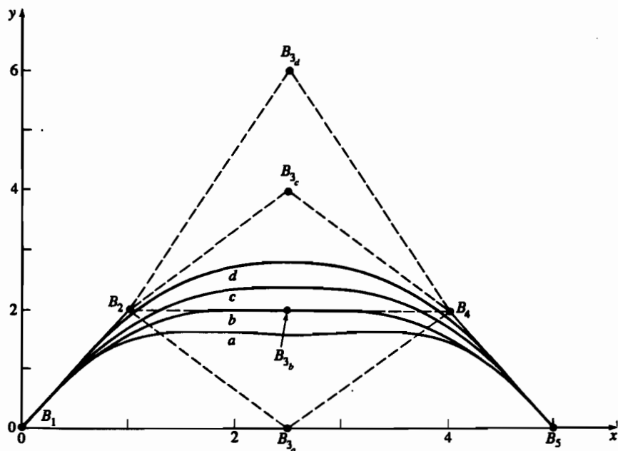
Рис. 5-65 Влияние перемещения одной вершины многоугольника на рациональный В-сплайн n+1=5 , k=4 , [H] = [1 \ 1 \ 0.25 \ 1 \ 1] .
