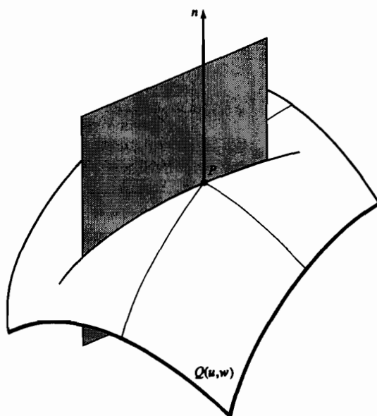
Рис. 6-29 Кривизна бипараметрической поверхности.
