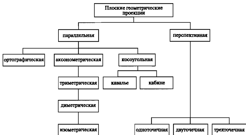
Рис. 3-10 Иерархия плоских геометрических проекций.
