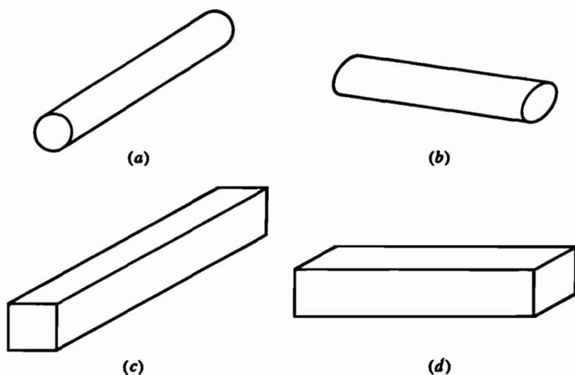
Рис. 3-25 Искажение, возникающее в косоугольных проекциях, f = 5/8 , \alpha = 45^\circ . (a) Круглая грань параллельна плоскости проекции; (b) круглая грань перпендикулярна плоскости проекции; (c) длинная сторона перпендикулярна плоскости проекции; (d) длинная сторона параллельна плоскости проекции.
