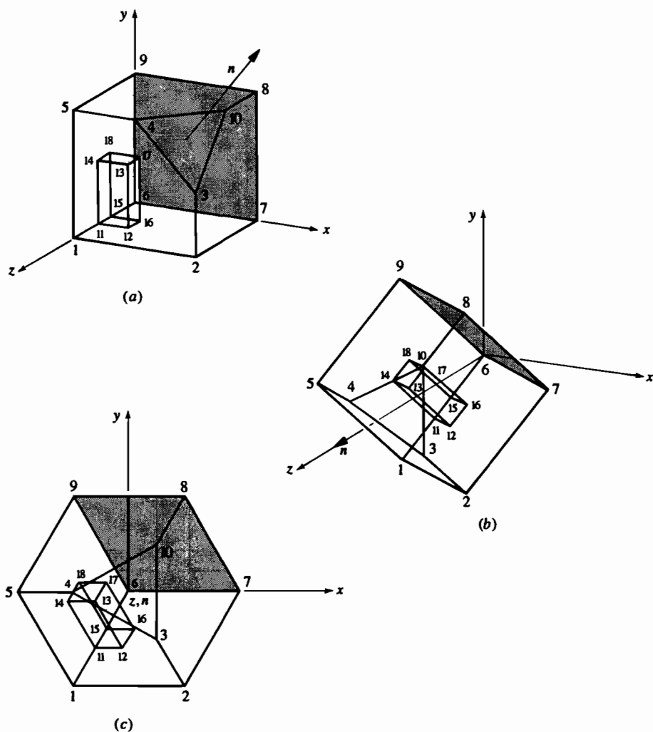
Рис. 3-14 Построение вспомогательного вида. (а) Триметрический вид; (б) нормаль совмещена с осью z ; (с) спроецировано на плоскость z = 0 .
