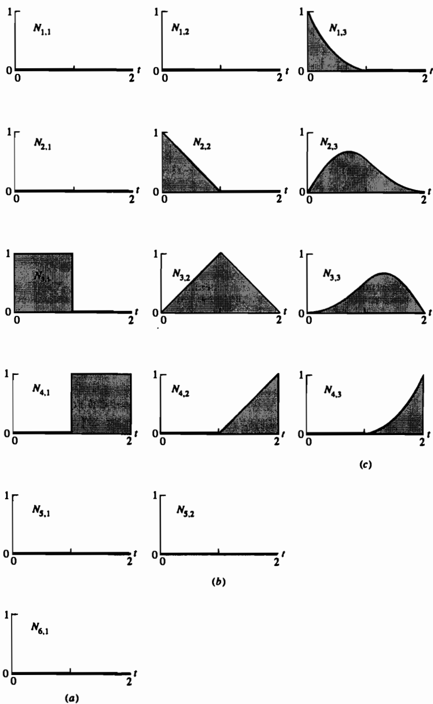
Рис. 5-40 Построение открытых базисных функций n + 1 = 4 . (a) k = 1 ; (b) k = 2 ; (c) k = 3 .
