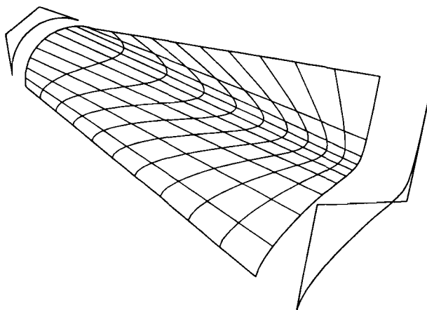
Рис. 6-56 Рациональная В-сплайн линейчатая поверхность.
