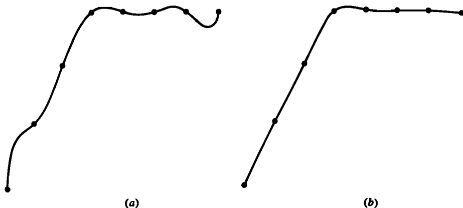
Рис. 5-17 Эффект напряжения кусочно кубического сплайна. (a) Без напряжения; (b) с напряжением.
