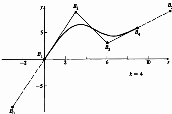
Рис. 5-53 Псевдовершины определяют начальную и конечную точки периодического В-сплайна.
