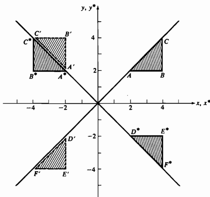
Рис. 2-10 Комбинированное преобразование на плоскости.
