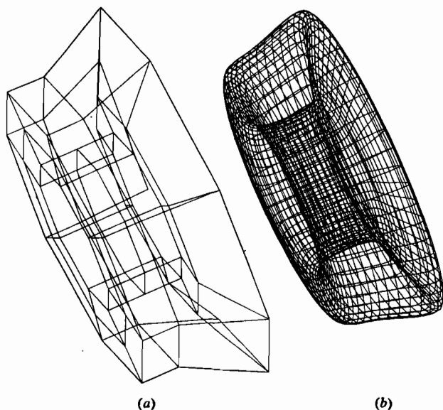
Рис. 6-48 Замкнутая тороидальная бикубическая ( k = l = 4 ) В-сплайн поверхность. (а) Характеристический многогранник; (б) поверхность.
