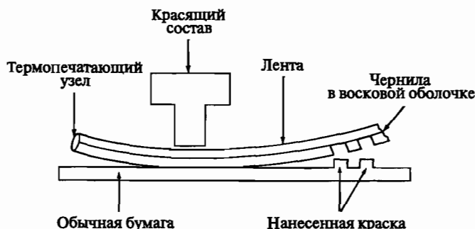
Рис. 1-55 Технология с косвенным тепловым воздействием.
