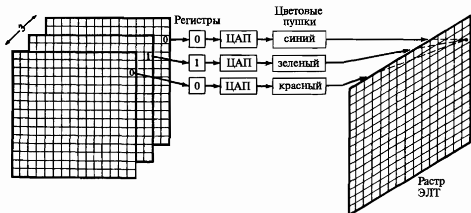
Рис. 1-27 Простой цветовой буфер кадра.
