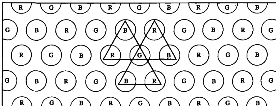
Рис. 1-32 Точечный люминофорный растр для ЭЛТ с теньевой маской.
