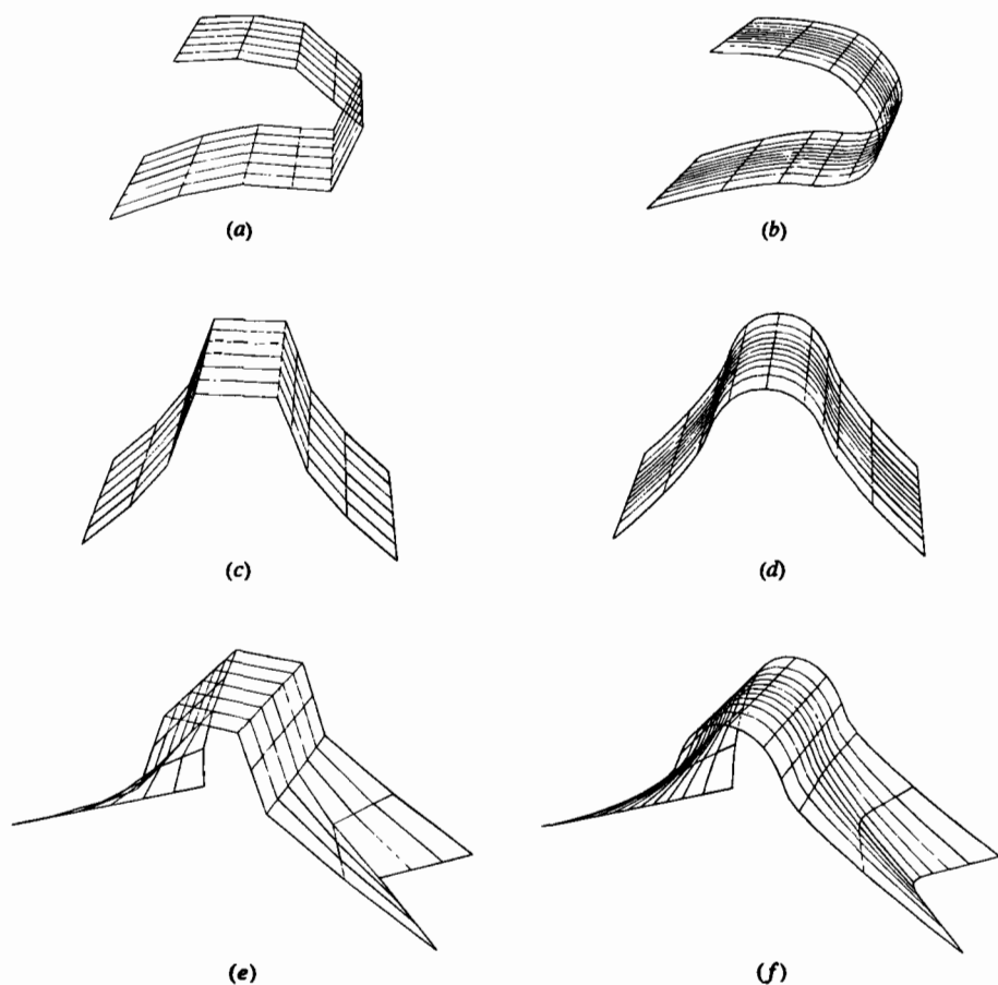
Рис. 6-60 Элемент квадратичной поверхности внутри более общей рациональной В-сплайн поверхности. Передняя кромка крыла. (а) Характеристический многогранник; (b) поверхность. Корма корабля. (с) Характеристический многогранник; (d) поверхность. Цилиндр как часть более общей поверхности. (e) Характеристический многогранник; (f) поверхность.
