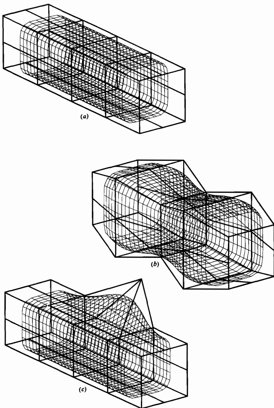
Рис. 6-46 Замкнутые периодические В-сплайн поверхности. (а) Прямая цилиндрическая поверхность; (b) возмущенная волнистая цилиндрическая поверхность; (с) эффект возмущения одной вершины сетки.
