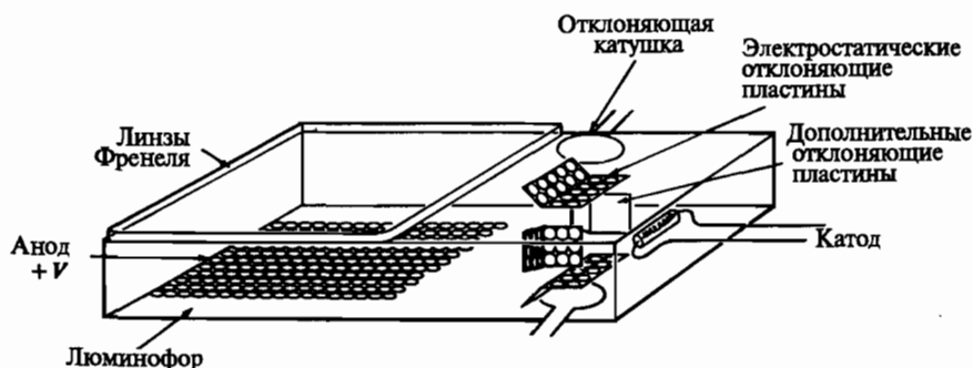
Рис. 1-36 Схема ЭЛТ.
