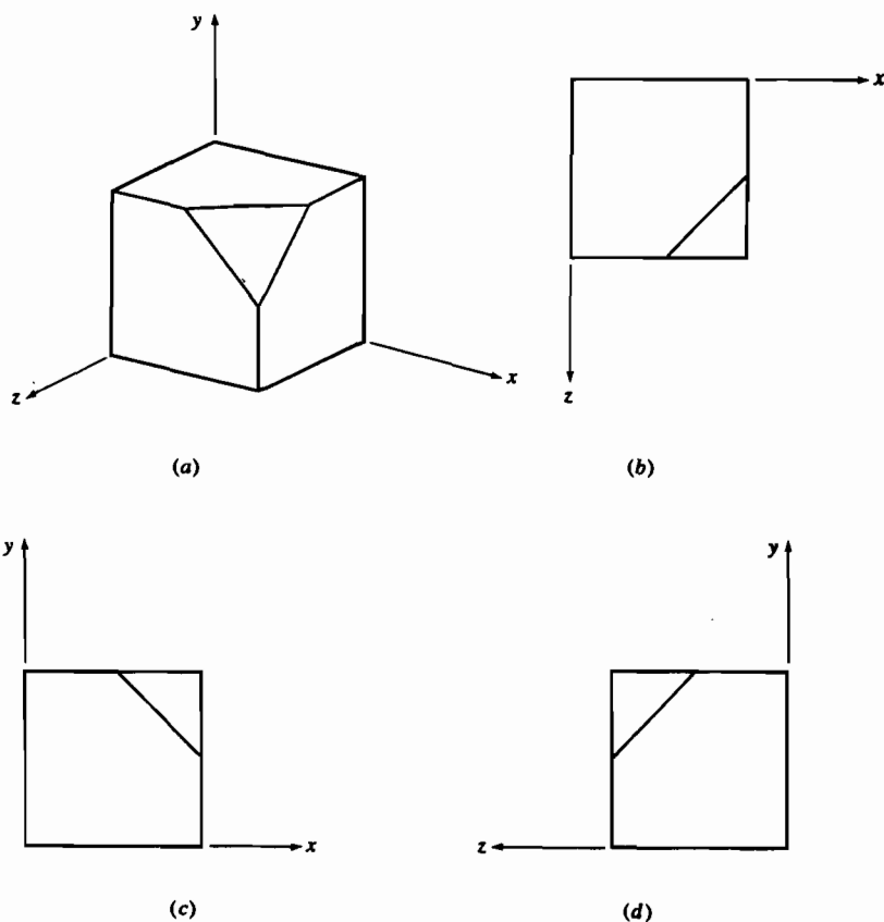
Рис. 3-12 Ортогографические проекции объекта на рис. 3-12а на плоскости: (b) y = 0 , (c) z = 0 и (d) x = 0 .
