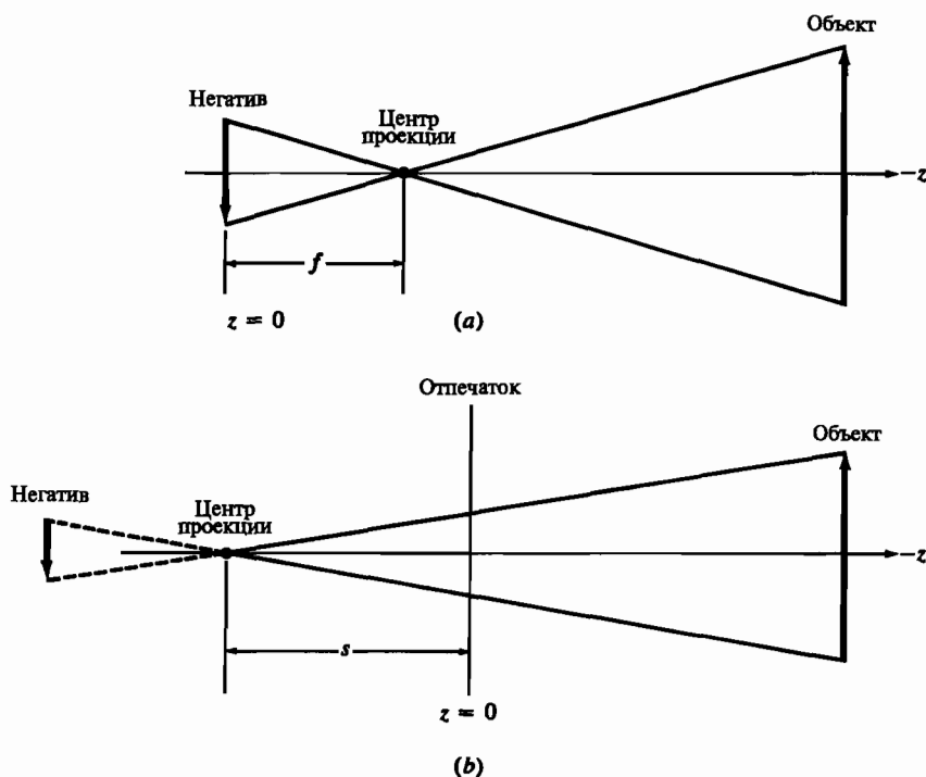
Рис. 3-40 Схема фотографической перспективы. (а) Создание исходного негатива; (б) создание оттиска.
