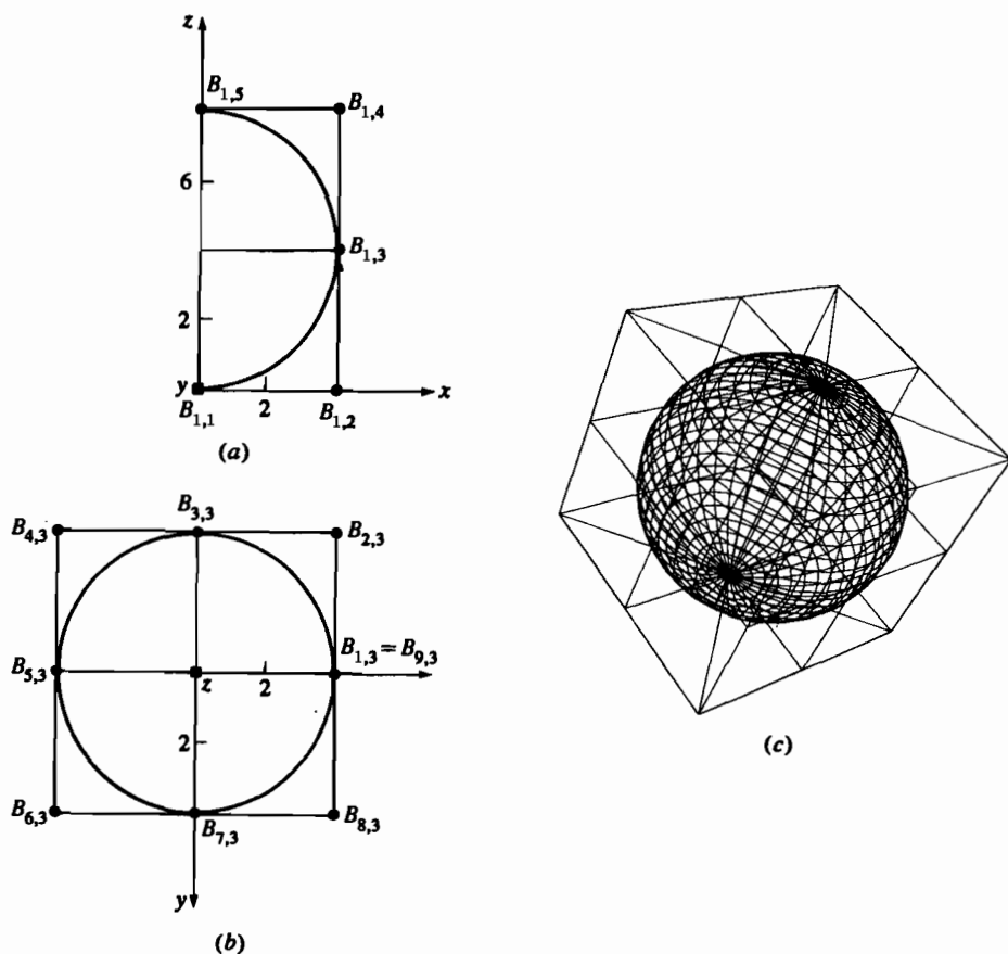
Рис. 6-59 Сфера, сгенерированная как рациональная В-сплайн поверхность. (а) Сместенная окружность и задающий многоугольник; (б) окружность вращения и задающий многоугольник; (в) характеристический многогранник и сфера.
