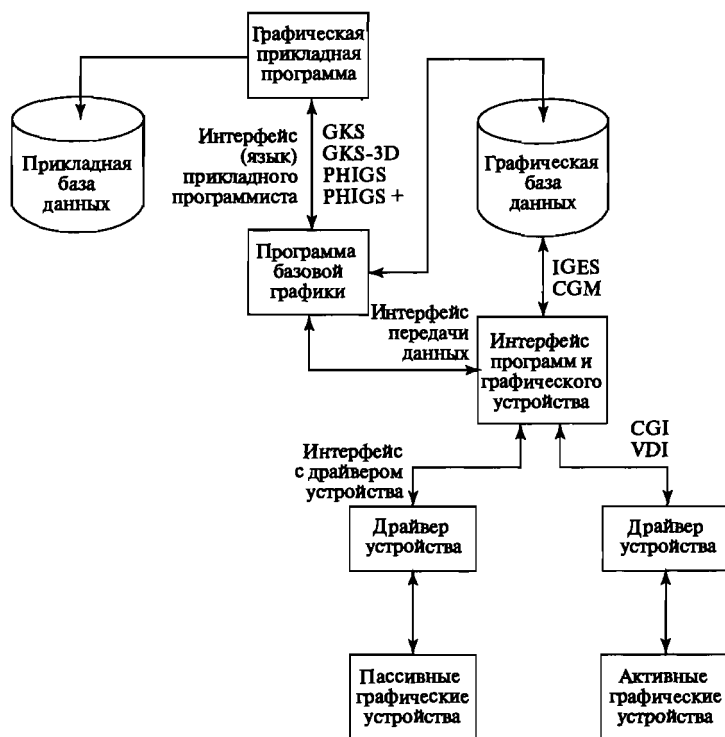
Рис. 1-63 Структура программного обеспечения машинной графики.
