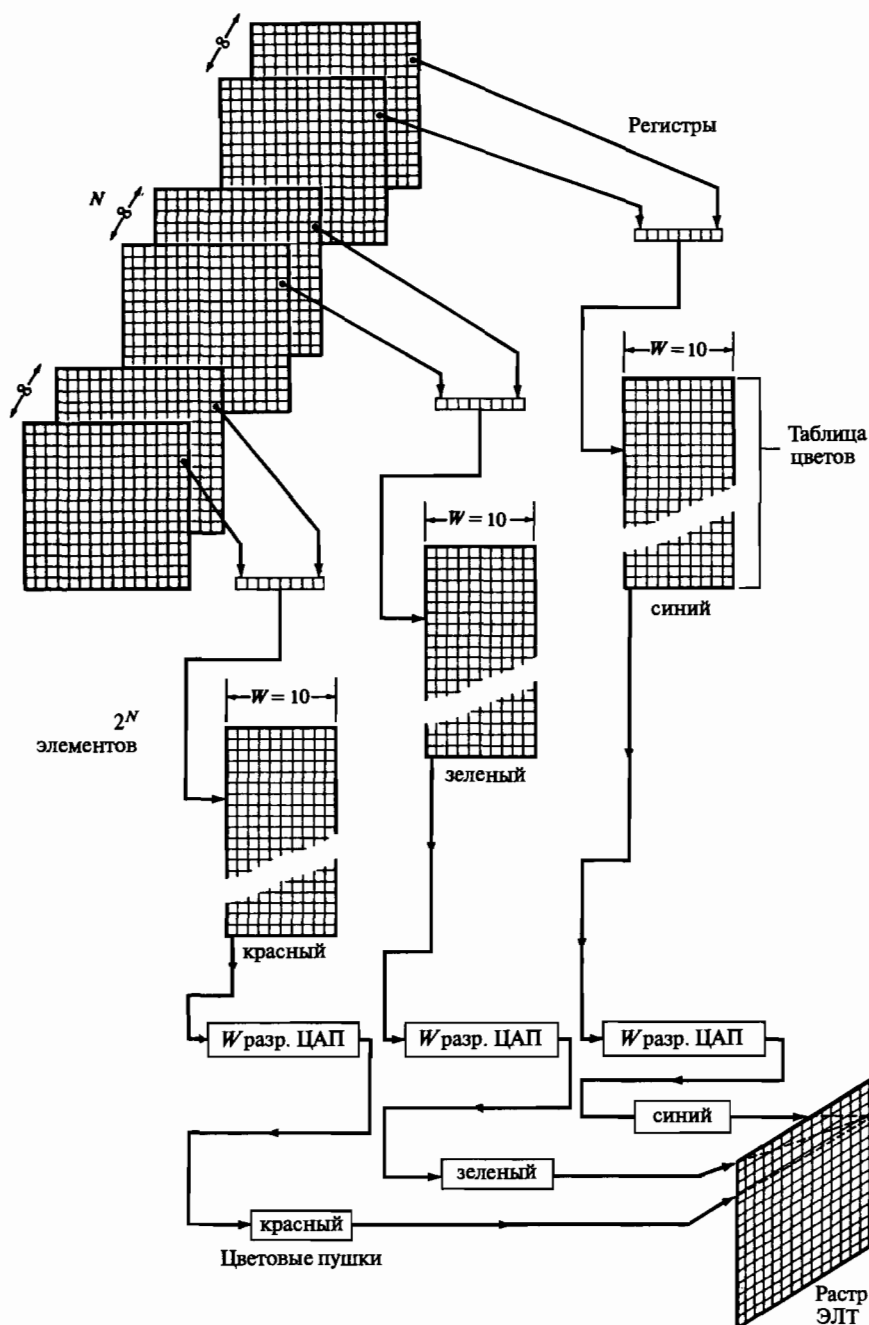
Рис. 1-29 Цветовой буфер кадра с 24 битовыми плоскостями и 10-разрядной таблицей цветов.
