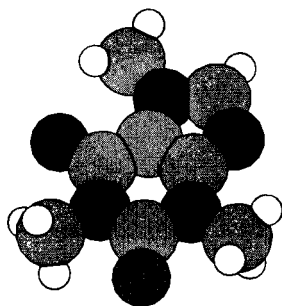
caffeine
