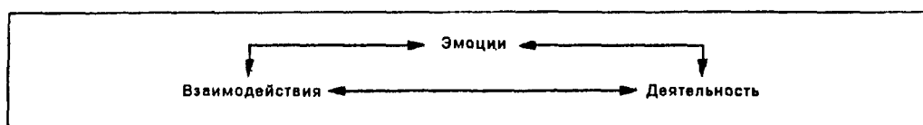
Рис. 15.2. Модель Хоманса.
