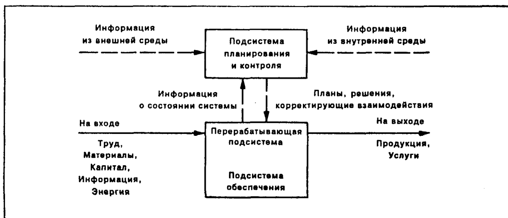
Рис. 20.1. Операционная система.
