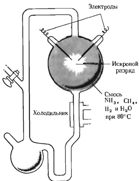
Рис. 3-16. Искроэлектрический аппарат, предназначенный для демонстрации абиотического образования органических соединений в условиях первичной атмосферы.
