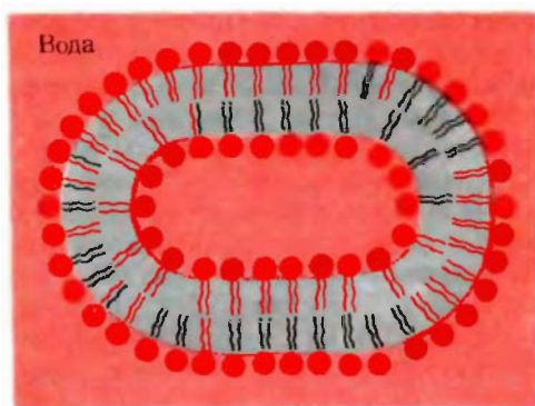
Липосома
