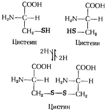
Рис. 5-7. Цистеин и цистин. Тиоловые ( -\text{SH} ) группы двух молекул цистеина легко окисляются и, соединяясь друг с другом, образуют дисульфидную группу цистина. В белках встречаются как цистеин, так и цистин.
