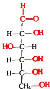
Глюкоза (сахар)
