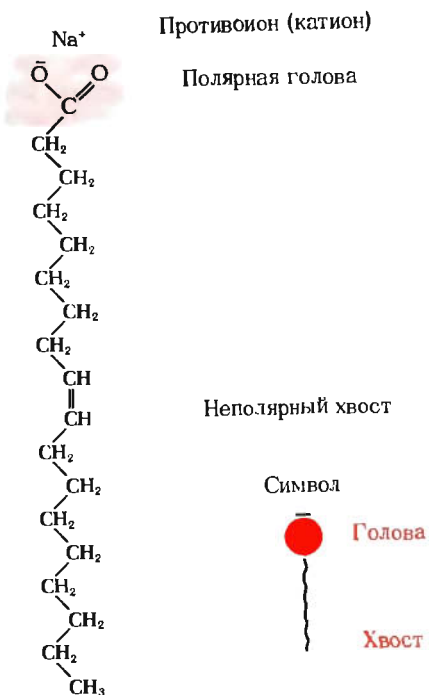
Олеат натрия
