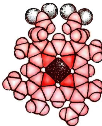
Пространственная модель гема
