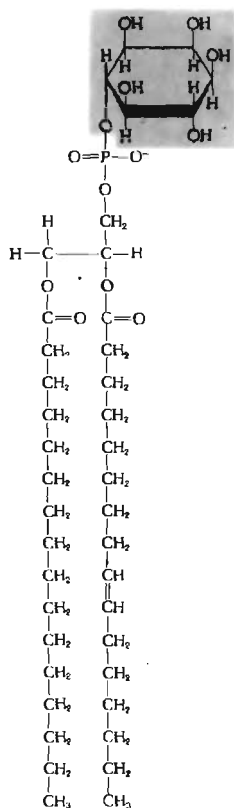
Фосфатидилинозитол
