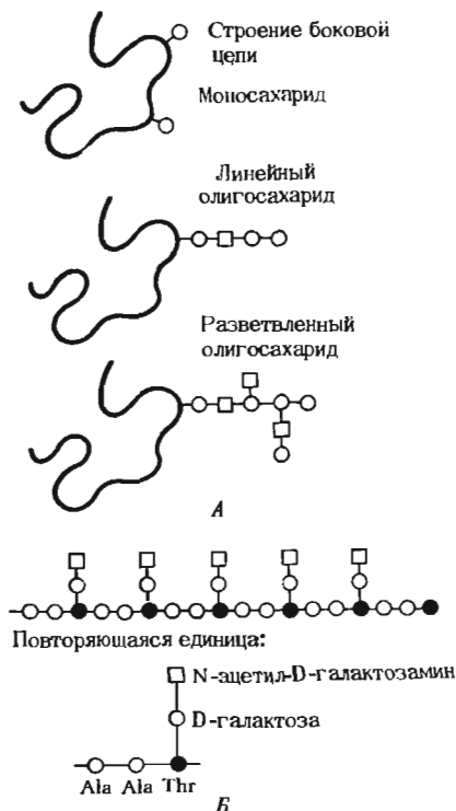
Рис. 11-22. Структура некоторых гликопротеинов и протеогликана. А. Три типа гликопротеинов, различающиеся размером и составом боковых углеводных цепей. Б. Повторяющаяся структурная единица антифризного гликопротеина, встречающегося у некоторых видов полярных рыб. Этот фрагмент повторяется много раз. Красные квадратики – N-ацетил-D-галактозамин, красные кружки – D-галактоза.
