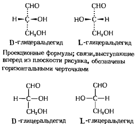
Рис. 11-5. Стереизомеры глицеральдегида.
