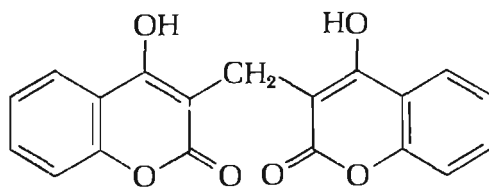
Дикумарол
