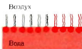
Фосфолипидный монослой
