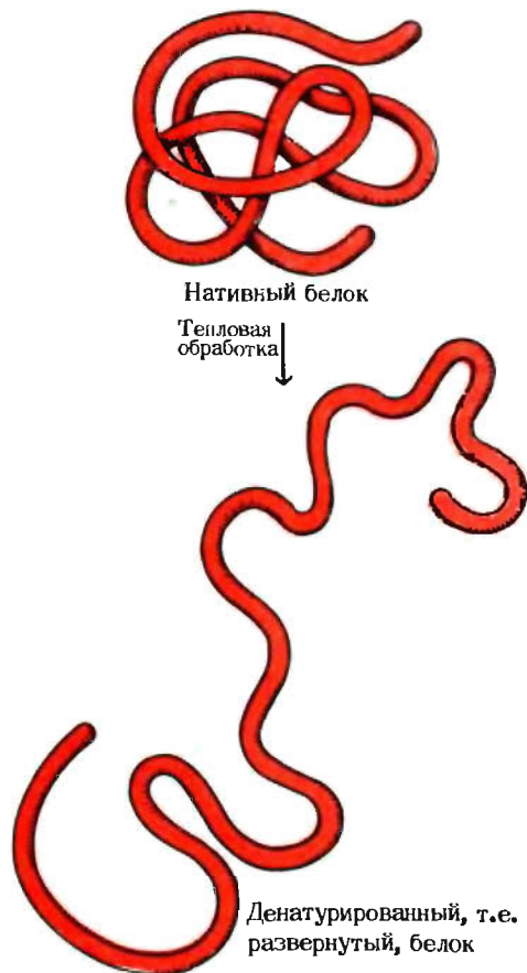
Рис. 6-16. Тепловая обработка нативных глобулярных белков, а также некоторые другие виды воздействия приводят к денатурации этих белков, т. е. к разворачиванию цепей без разрушения их ковалентной структуры. Денатурированный белок может принимать множество случайных конформаций и обычно не обладает биологической активностью.
