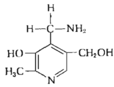
Пиридоксамин
