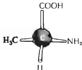
D-аланин
