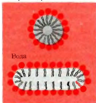
Фосфолипидный монослой
