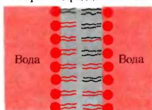
Липосома
