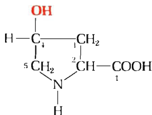
4-гидроксипролин
