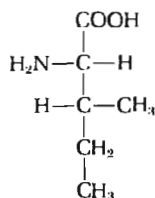
Изолейцин
