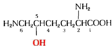
5-гидроксилизин
