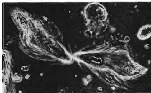
Рис. 11-17. Две клетки Trichonympha . Эти простейшие живут в кишечнике термитов и секретируют целлюлазу. Не будь этих паразитов, термиты не смогли бы переваривать целлюлозу.
