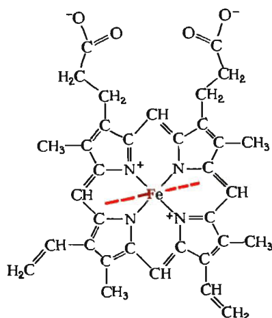
Структура гема
