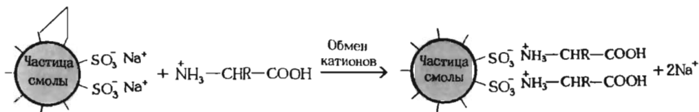
Анионные центры
