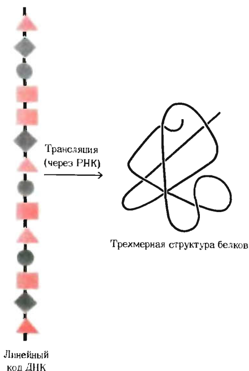
Рис. 1-11. Информация, записанная в виде линейной последовательности нуклеотидов в ДНК, транслируется (т. е. переводится) в трехмерную структуру белков.
