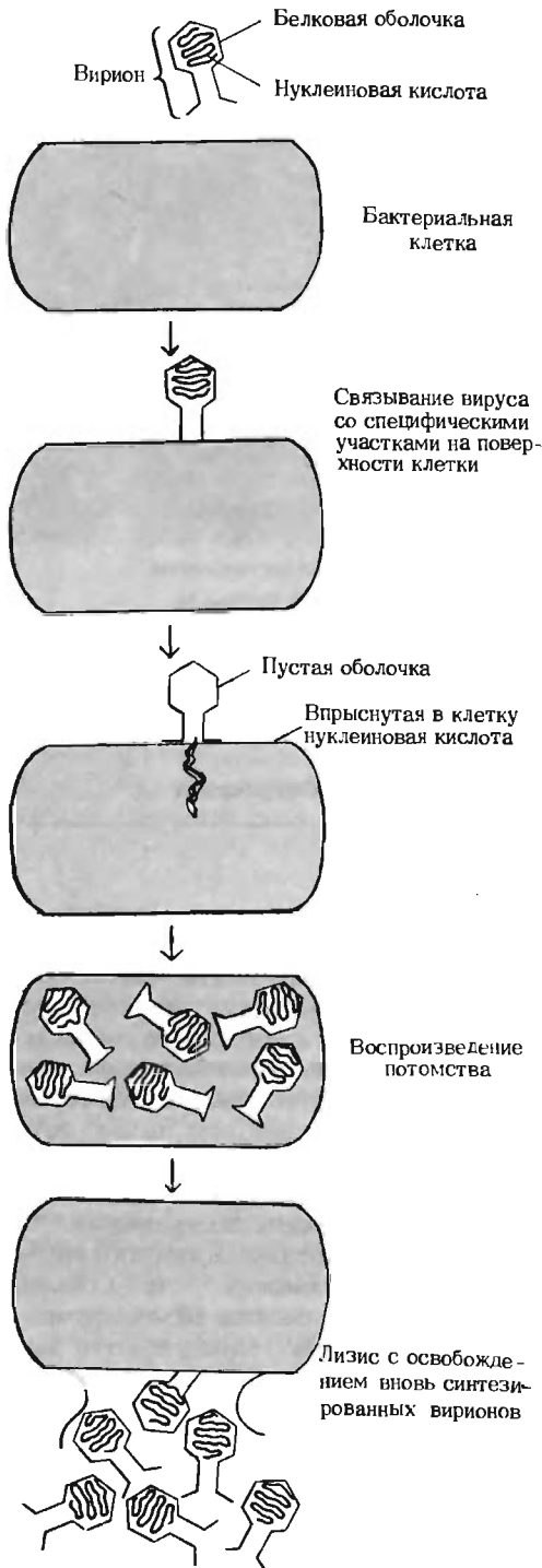
Рис. 2-24. Репликация бактериофага в клетке-хозяине.
