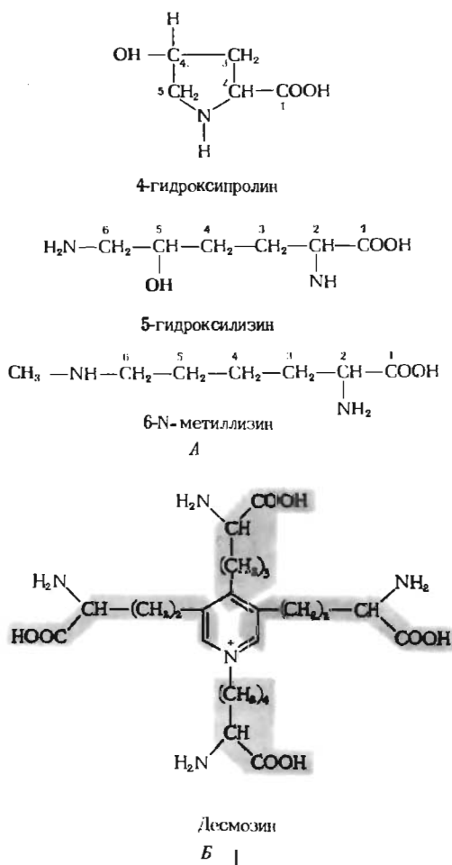
Рис. 5-8. А. Некоторые нестандартные аминокислоты, встречающиеся в белках. Цветом выделены дополнительные функциональные группы, присоединенные к молекулам стандартных аминокислот пролина и лизина. Б. Десмозин, обнаруженный в белке эластине, образуется из четырех молекул лизина, углеродные скелеты которых выделены жирным шрифтом и затенены.
