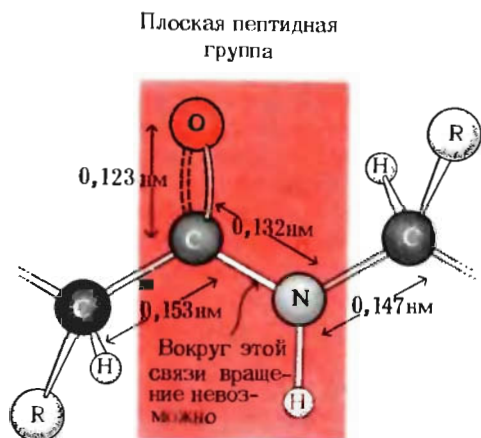
Рис. 7-4. Плоская пептидная группа. С—N-связь частично имеет характер двойной связи и поэтому вокруг нее свободное вращение невозможно. Обратите внимание, что атомы кислорода и водорода лежат в этой плоскости по разные стороны от С—N-связи. Это соответствует транс -конфигурации пептидной связи.
