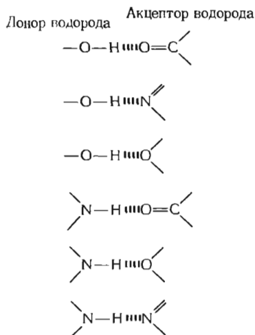
Рис. 4-3. Водородные связи. В связях этого типа атом водорода неравномерно распределен между двумя электроотрицательными атомами. Атом, с которым водород связан ковалентно, служит донором водорода, а электроотрицательный атом другой молекулы – акцептором. В биологических системах электроотрицательными атомами, участвующими в образовании водородных связей, являются кислород и азот; атомы углерода принимают участие в образовании водородных связей только в редких случаях. Расстояние между двумя электроотрицательными атомами, соединенными водородной связью, варьирует от 0,26 до 0,31 нм. Ниже показаны обычные типы водородных связей.
