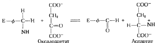
Оксалоацетат
