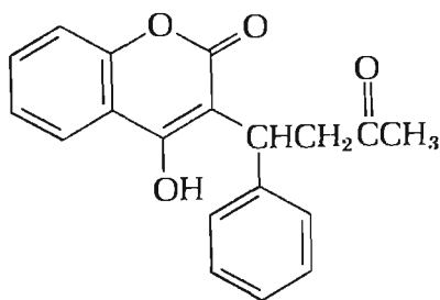
Варфарин
