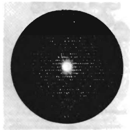
Рис. 8-3. Фотоотпечаток рентгенограммы кристаллического миоглобина кашалота. По расположению и интенсивности дифракционных пятен, возникающих в результате взаимодействия рентгеновского пучка с атомами миоглобина в кристалле, была рассчитана точная трехмерная структура миоглобина.
