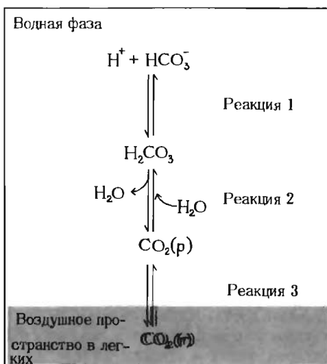
Рис. 1. Между \text{CO}_2 в воздушном пространстве легких и бикарбонатным буфером в плазме крови, протекающей через капилляры легких, устанавливается равновесие. Так как концентрация растворенной \text{CO}_2 может быть быстро отрегулирована путем изменений скорости дыхания, бикарбонатная буферная система крови находится почти в равновесии с обширным потенциальными резервуаром \text{CO}_2 .
