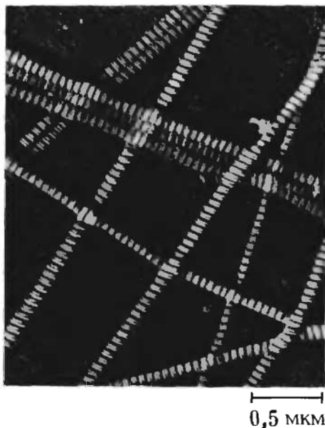
Рис. 7-12. Электронная микрофотография коллагеновых фибрилл соединительной ткани. Обратите внимание на периодичность поперечных полос в фибриллах. В коллагенах многих тканей эти полосы повторяются примерно через каждые 64 нм.
