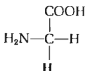
Рис. 5-3. Глицин, единственная аминокислота, у которой нет асимметрического атома углерода. R-группа, представляющая собой атом водорода, выделена красным цветом.
