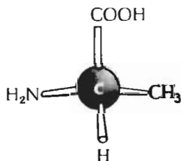
L-аланин
