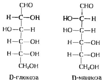
Рис. 11-7. Эпимеры D-глюкозы.
