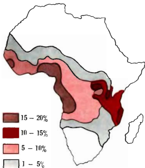
Рис. 8-24. Относительная частота распространения гена серповидноклеточности в различных частях Африки. Зоны, соответствующие наибольшему распространению этого гена, находятся в тех областях, где когда-то основной причиной смертности была малярия.
