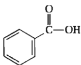
Бензойная кислота pK' \sim 5 нерастворима в воде
