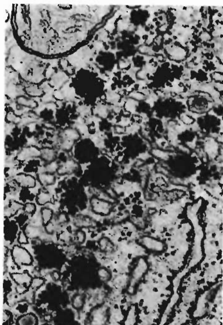
Рис. 2-19. Гранулы гликогена (интенсивно окрашенные) в цитоплазме клетки печени хомяка. Гранулы состоят из больших групп, образуемых молекулами гликогена. По своим размерам они значительно превышают рибосомы, которые видны на поверхности эндоплазматического ретикулума в нижнем правом углу.
