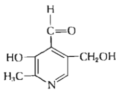
Пиридоксаль
