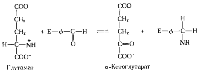
Глутамат
