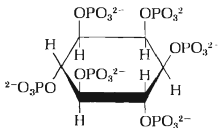
Фитиновая кислота
