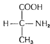
D-аланин
