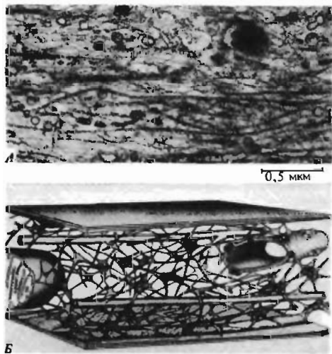
Рис. 2-17. А. Электронная микрофотография воложистого цитоскелета фибробласта. Б. Схематическое изображение цитоскелета фибробласта. Длинные трубки – это микротрубочки, а более тонкие элементы – микрофиламенты различных типов.
