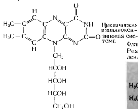
Рибофлавин
